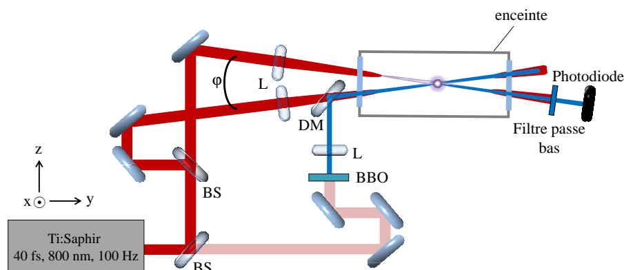
FIGURE 4.6: Montage expérimental pour mesurer la durée de vie du réseau. Les deux filaments se croisent avec un angle \varphi de 7, 14 ou 90 degrés. La sonde est doublée en fréquence par un cristal de BBO. L'intensité de la sonde diffractée par le réseau est enregistrée par une photodiode. Les mesures ont été réalisées dans huit gaz : air, O 2 , N 2 , CO 2 et Ne, Ar, Kr, Xe.
