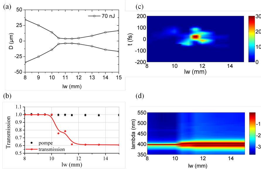
FIGURE 2.20: (a) Diamètre du faisceau, (b) transmission, (c) profil temporel de la distribution d'intensité et (d) suivi spectral en fonction de la longueur de propagation l_w . E_i = 70 nJ, L_1 : 50 mm.
