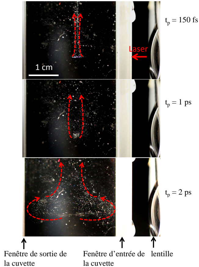
FIGURE 3.8: Photographies de la zone d'interaction prises avec un appareil photo numérique Canon équipé d'un objectif Macro 100 mm f/2,8 . t_p \approx 150 fs, 1 ps, 2 ps. f = 20 mm. \lambda = 800 nm. E_i = 600 \mu J.
