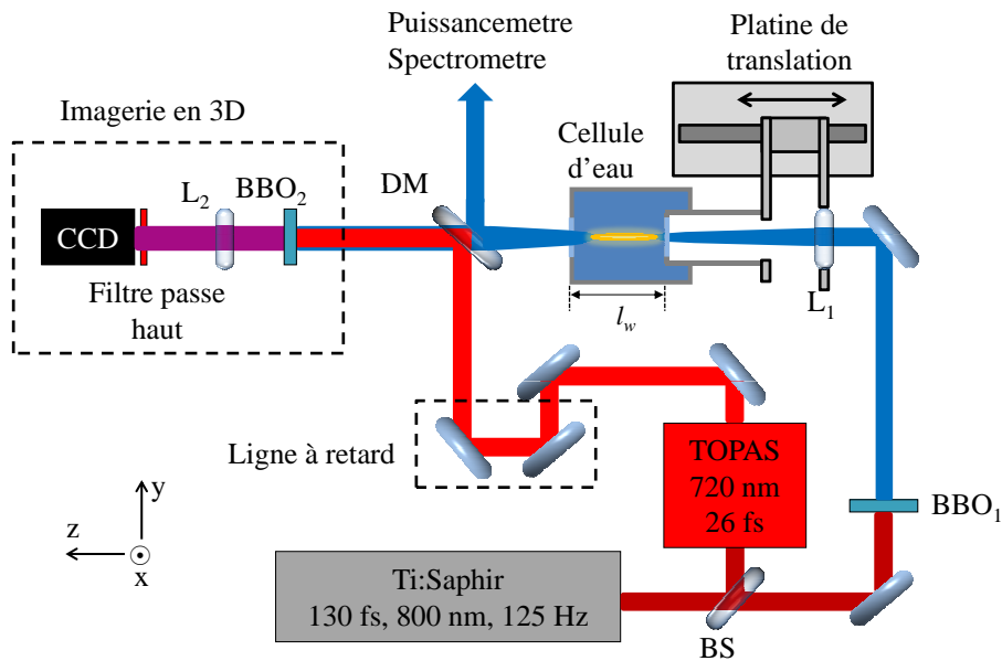
FIGURE 2.3: Montage expérimental. BS : séparatrice. L_1 : lentille convergente ( f = 50 mm, 200 mm ou 300 mm). L_2 : lentilles d'imagerie (deux focales de 125 mm). DM : miroir dichroïque. TOPAS : amplificateur paramétrique optique non-colinéaire (NOPA). La longueur de la cuvette d'eau l_w est variable de 4 mm à 40 mm.
