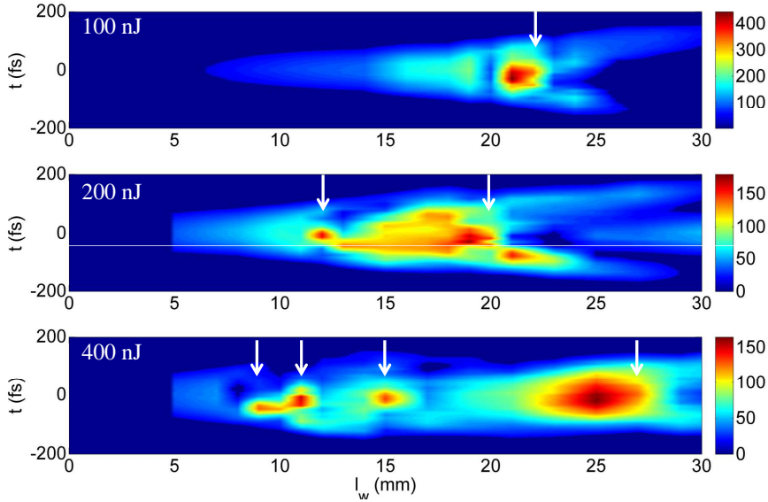
FIGURE 2.16: Profils temporels de la distribution axiale d'intensité I(x = 0, y = 0, z, t) en fonction de la longueur de propagation l_w obtenus expérimentalement à 100 nJ, 200 nJ et 400 nJ. L_1 = 300 mm. Les flèches indiquent la position des divisions de l'impulsion (voir tableau 2.1).
