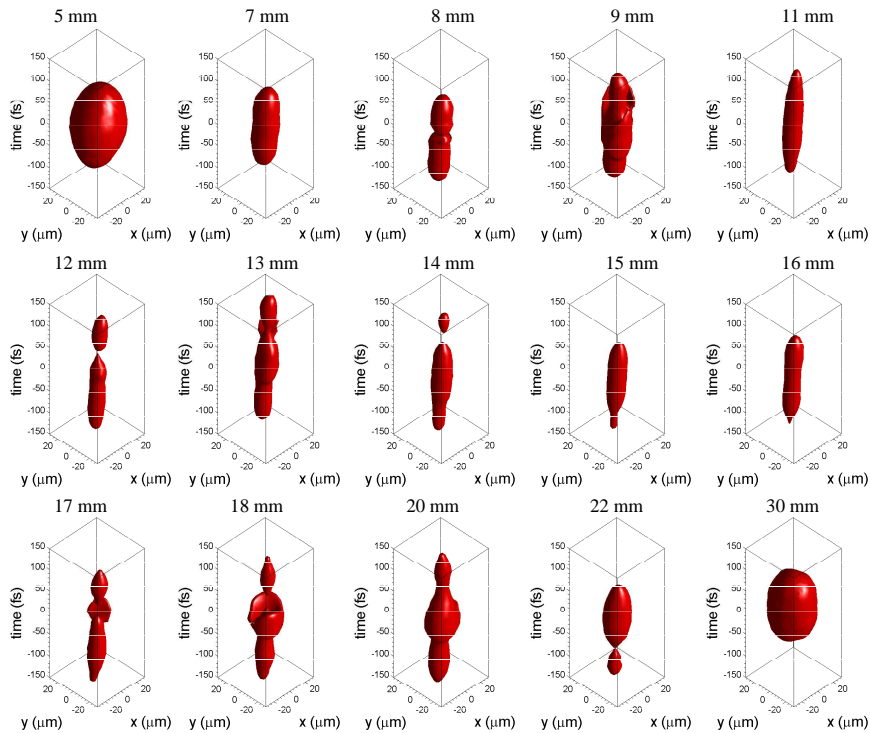
FIGURE 2.6: Suivi de la distribution d'intensité d'une impulsion de 400 nm, 100 fs au cours de sa propagation dans l'eau. l_w est augmentée progressivement de 5 mm à 30 mm. E_i = 450 nJ, L_1 : 200 mm. Les distributions ont été tracées pour un niveau d'intensité supérieur à 30 % du maximum. Taille de chaque fenêtre : 60 \mu\text{m} \times 60 \mu\text{m} \times 300 fs. La direction de propagation va de haut en bas (des temps positifs vers les temps négatifs).
