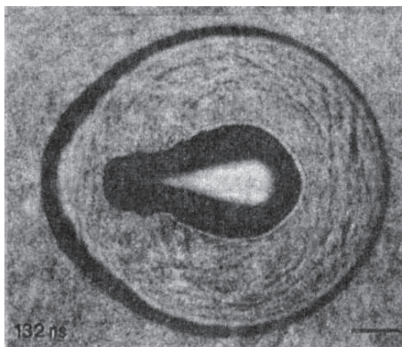
FIGURE 3.1: Front d'onde de choc (autour) et bulle de cavitation (au centre) générés par la propagation d'une impulsion de 10 mJ, 6 ns et \lambda = 1064 nm dans l'eau, 132 ns après l'interaction. Echelle : 100 \mu\text{m} [90].
