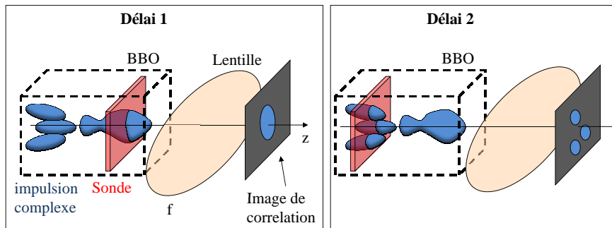
FIGURE 2.1: Représentation schématique de la technique de corrélation croisée.
