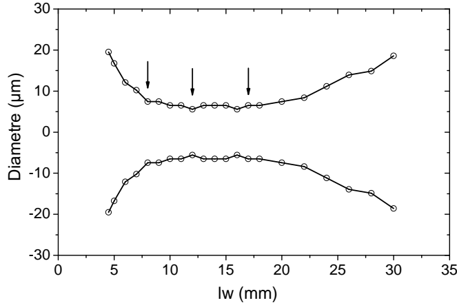
FIGURE 2.8: Evolution du diamètre du faisceau en fonction de la distance de propagation pour E_i = 450 nJ, L_1 : 200 mm. Les flèches indiquent la position des divisions de l'impulsion.
