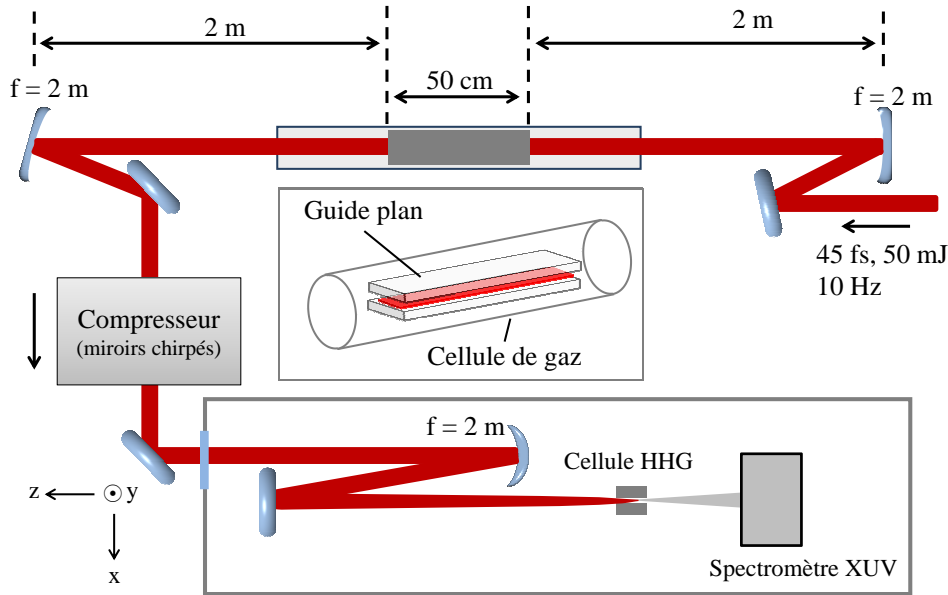
FIGURE 6.8: Schéma du montage de compression sur la ligne de génération d'harmonique du Lund Laser Center (LLC).
