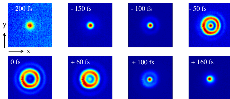
FIGURE 2.4: Images CCD de la corrélation entre l'impulsion et la sonde, générées au sein du \text{BBO}_2 pour f = 300 mm, E_i=100 nJ, l_w = 26 mm. Les temps indiqués représentent le retard entre l'impulsion et la sonde. La séquence est enregistrée pour un pas de 10,5 fs.
