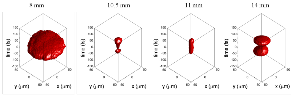
FIGURE 2.19: Suivi de la distribution d'intensité de l'impulsion au cours de sa propagation dans l'eau. l_w est augmentée progressivement de 6 mm à 16 mm. E_i = 70 nJ, L_1 : 50 mm. Les distributions ont été tracées pour un niveau d'intensité supérieur à 20 % du maximum.
