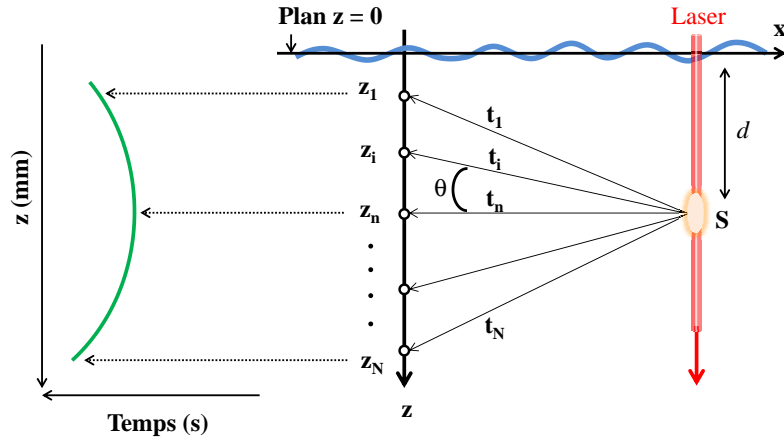
FIGURE 3.17: Schéma du principe des mesures de temps de vol.
