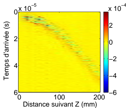
FIGURE 3.23: Temps de vol des signaux acoustiques lors d'un déplacement du capteur HF suivant l'axe z . \lambda = 800 mm, E_i = 290 mJ, f = 1000 mm et h = 730 mm. Unité : volts (V).
