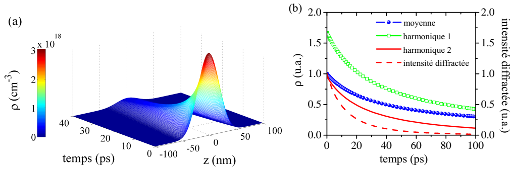
FIGURE 4.7: (a) Evolution temporelle d'une frange du réseau de plasma dans l'air pour \lambda = 800 nm, \varphi = 14^\circ , D = 1 cm 2 /s, \beta = 5 \times 10^{-8} cm 2 /s et \rho_0 = 10^{18} cm -3 . (b) Axe de gauche : densité électronique moyenne (cercle bleu), de la première (carré vert) et de la deuxième (ligne rouge) harmonique du réseau. Axe de droite : Intensité de la sonde diffractée par le réseau (pointillés rouges).
