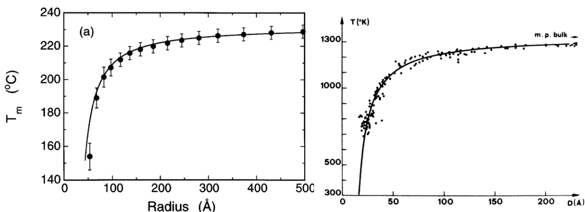
Figure 1-2 : Evolution du point de fusion de nanoparticules d'étain 8 (gauche) et d'or 7 (droite) en fonction de leur taille.
