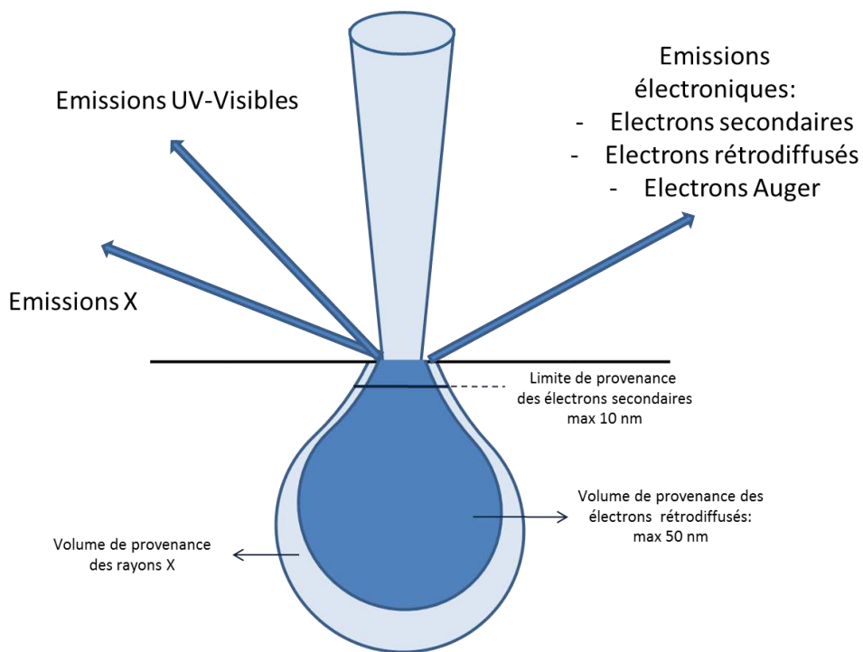
Figure 1-20 : Principales émissions électroniques et électromagnétiques dues aux interactions d'un faisceau d'électrons avec un échantillon. Les électrons se déplacent dans un volume appelé poire d'interaction.
