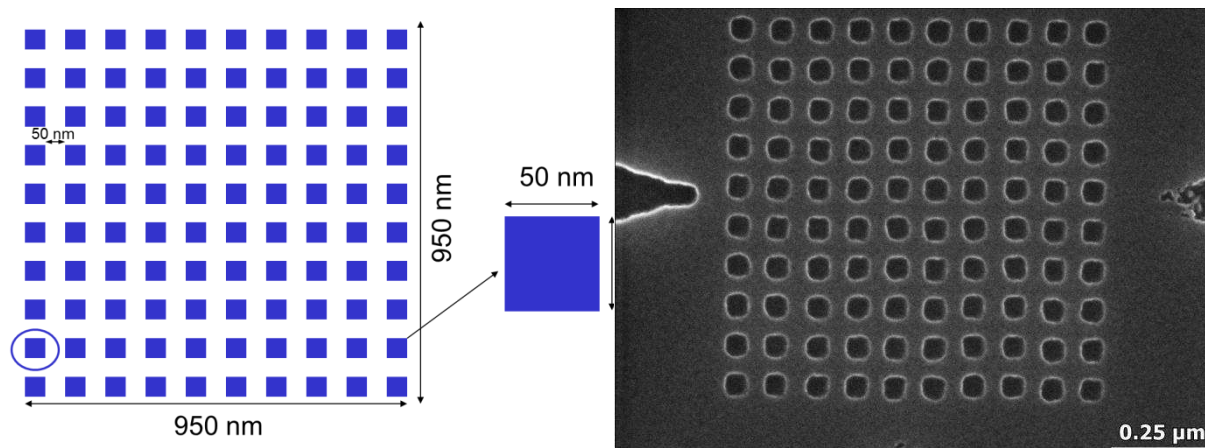
Figure 4-6 : Représentation schématique du réseau fabriqué au LPN, et image MEB du réseau obtenu.
