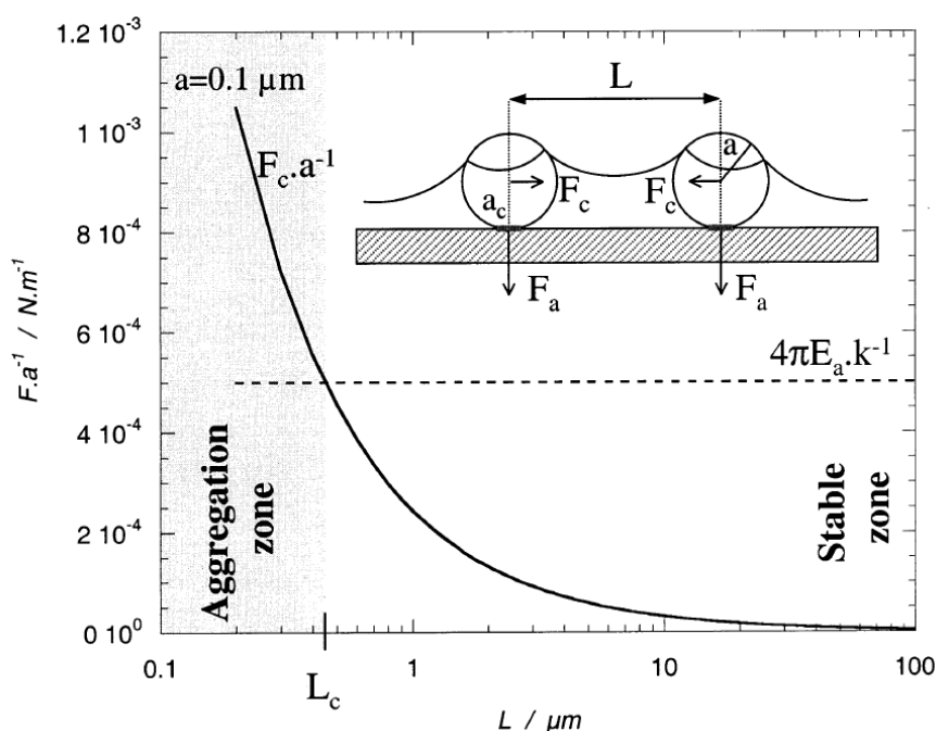
Figure 2-5 : Graphique représentant la prédominance des forces de capillarité ( F_c ) par rapport aux forces d'adhésion ( F_a ) en fonction de l'épaisseur de la couche de solvant ( a ). Lorsque les forces de capillarité sont prédominantes, les particules forment des agglomérats. Figure extraite de l'article de A. Thill et O. Spalla 74 .
