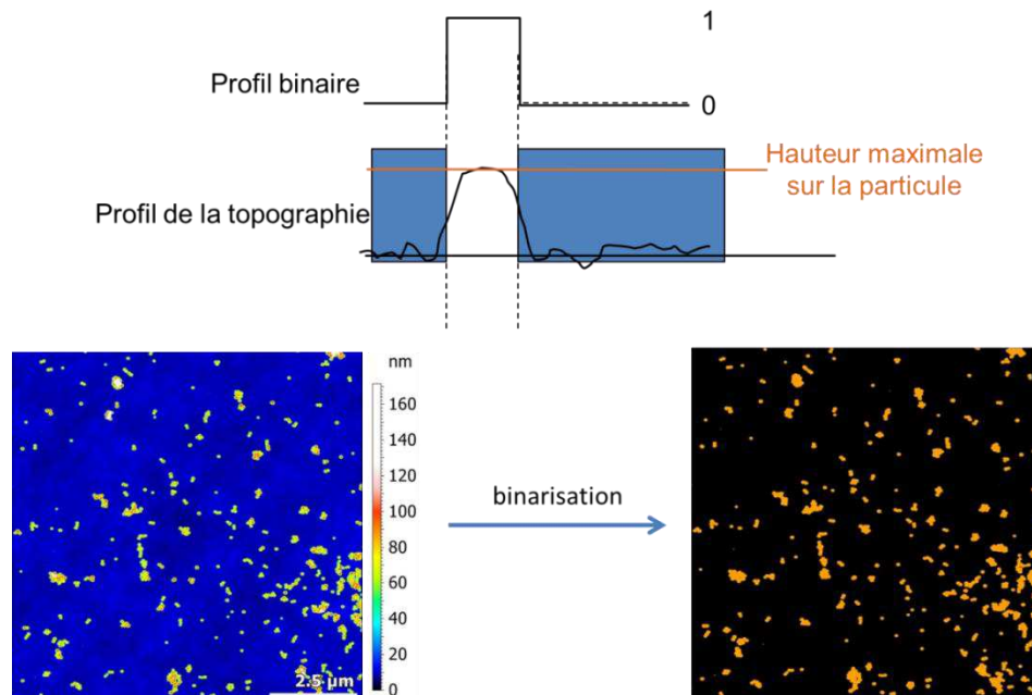
Figure 5-12 : Représentation schématique de la binarisation d'un profil d'une image topographique (haut). Binarisation d'une image topographique de nanoparticules imagée par AFM.
