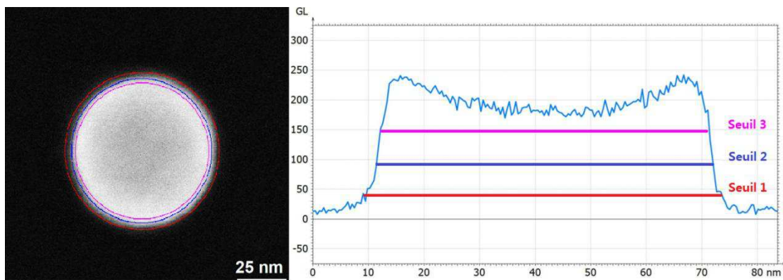
Figure 5-8 : Dépendance du diamètre équivalent en fonction du placement du seuil lors de la détection et de la détermination de la taille de la nanoparticule par seuillage : sur une image MEB (-contraste topographique, détecteur In-Lens, gauche), et sur un profil (droite).
