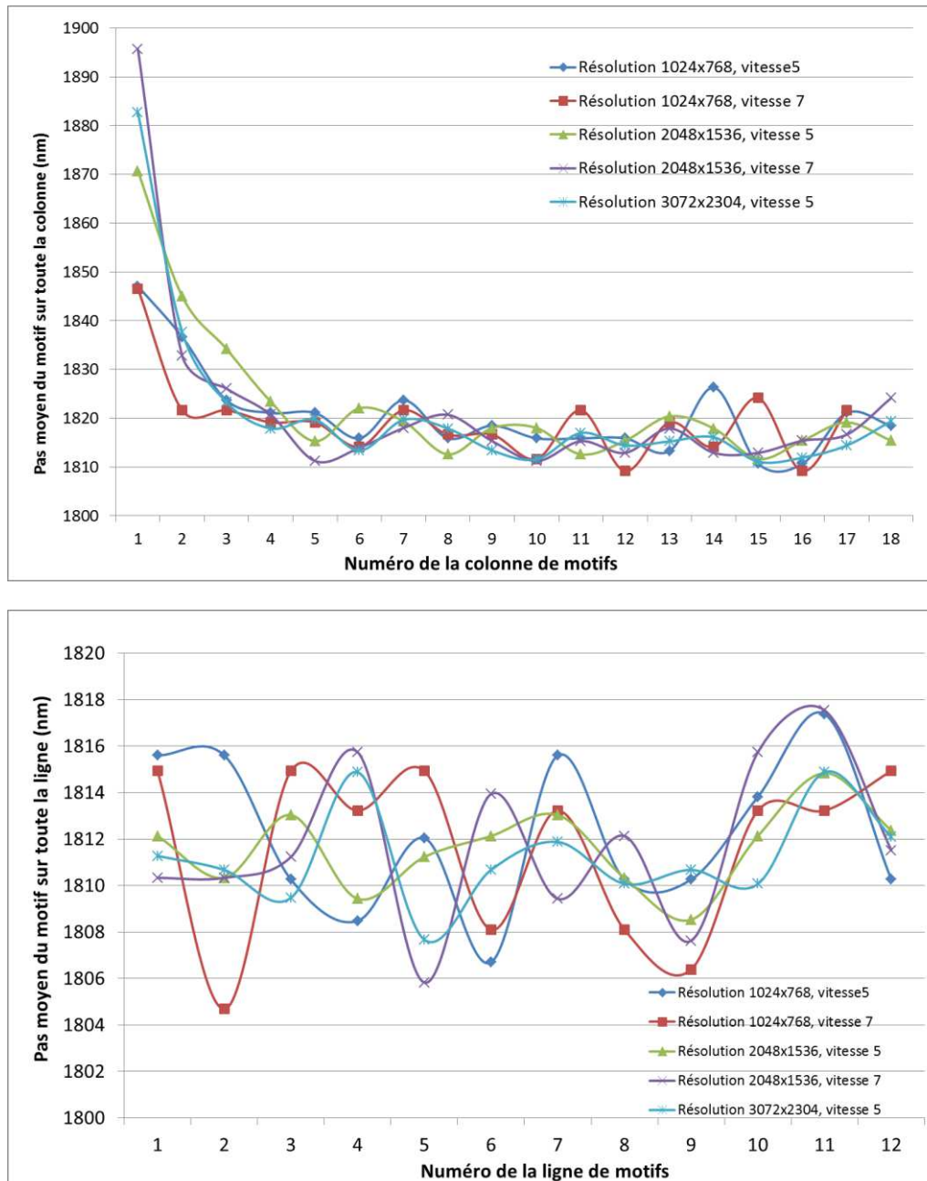
Figure 4-5 : Mesure du pas de réseau moyen suivant les axes X (haut) et Y (bas) et en fonction du numéro de la colonne (suivant X) ou de la ligne (suivant Y) de motifs dans l'image. Les motifs sont numérotés de gauche à droite sur l'image suivant l'axe X et de haut en bas sur l'image suivant l'axe Y.
