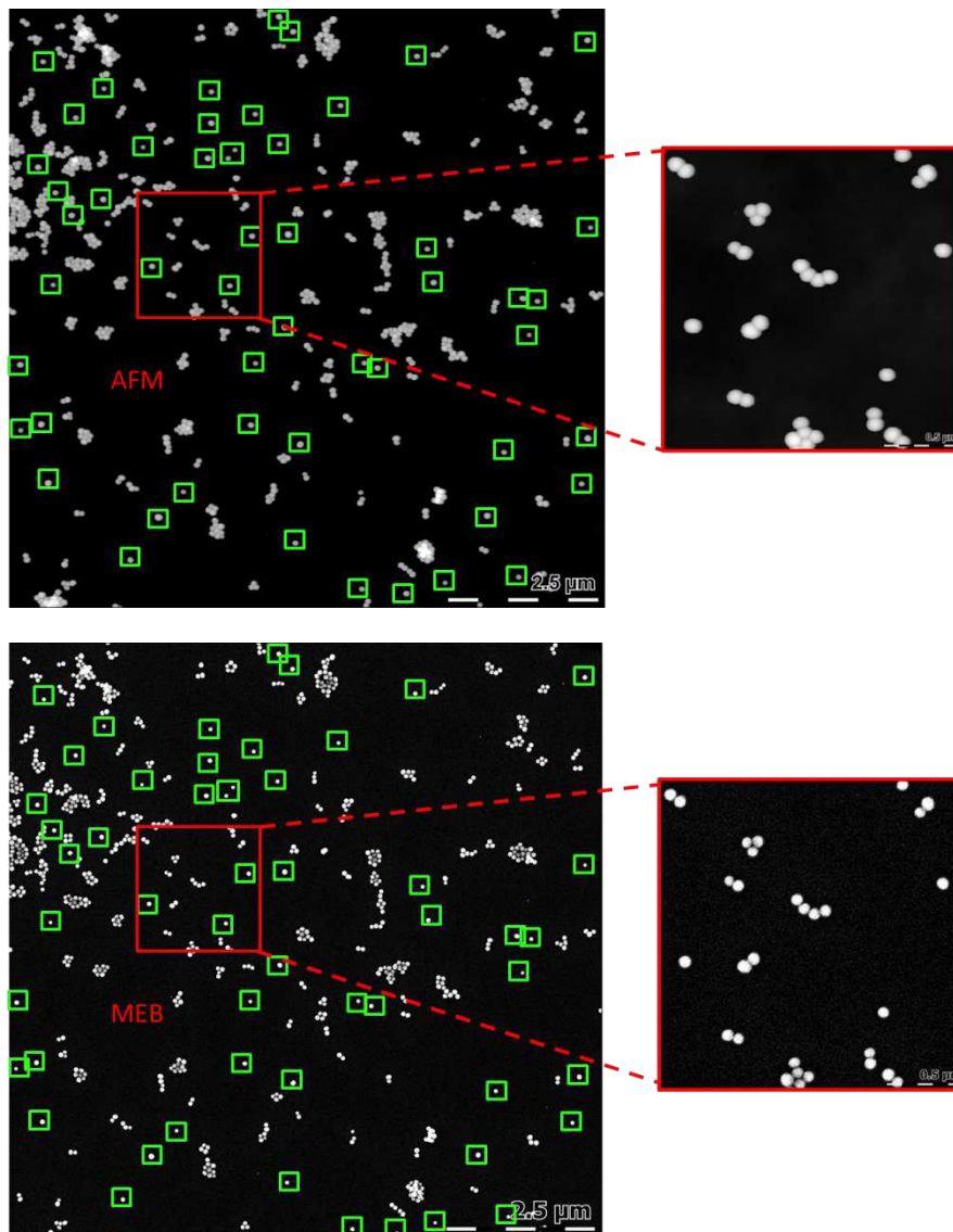
Figure 6-5 : Même groupe de 55 nanoparticules de \text{SiO}_2 déposées sur du silicium (échantillon B), images par AFM (haut) et par MEB (bas). Sur la droite, un zoom montrant 29 nanoparticules images par AFM (haut) et par MEB (bas).
