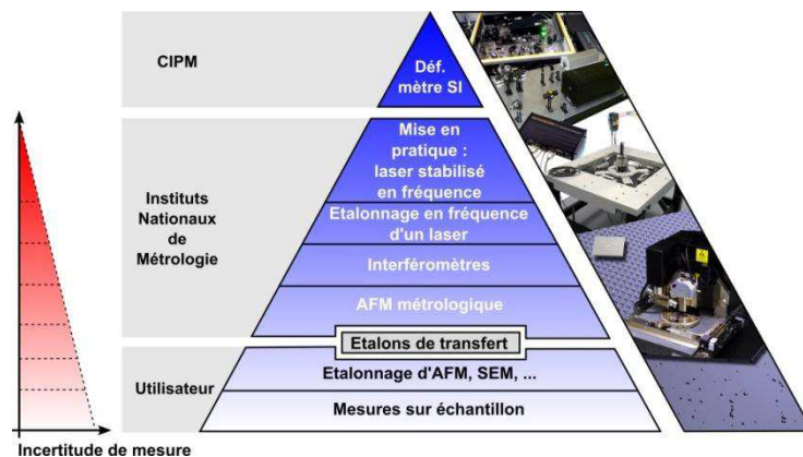
Figure 1-10 : Exemple de chaîne de traçabilité (microscopies) appliquée aux mesures dimensionnelles à l'échelle du nanomètre.
