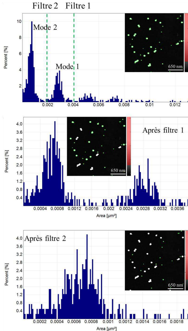
Figure 5-3 : Distribution en aire d'une population bi-modale de nanoparticules sphériques imagées par AFM (image correspondante en insert). Définition de filtre paramétré en fonction de l'aire des éléments afin de sélectionner les particules devant compter dans la distribution (pointillés verts). Sur l'histogramme du haut, aucun filtre n'est appliqué ; sur l'histogramme central, le filtre 1 est appliqué ; sur l'histogramme du bas, le filtre 2 est appliqué.
