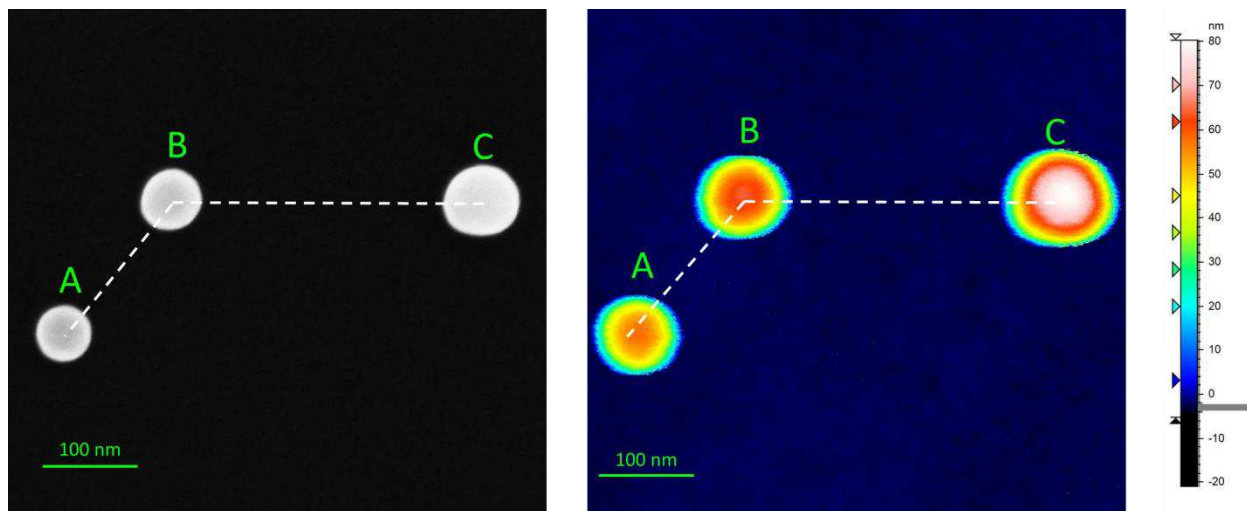
Figure 6-6 : Image MEB (gauche) et image AFM (droite) de trois mêmes nanoparticules de \text{SiO}_2 .
