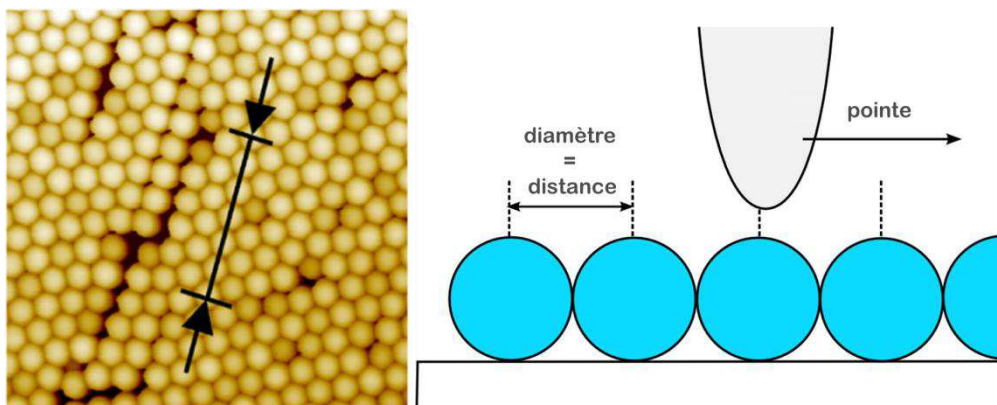
Figure 1-19 : Mesure de taille de nanoparticules déposée en une monocouche par mesure du pas du réseau constitué de nanoparticules. Cette méthode est mise en œuvre par l'équipe de J. Garnaes (DFM – Institut de métrologie danois) 48 et également par l'équipe de F. Méli (METAS – Institut de métrologie Suisse)
