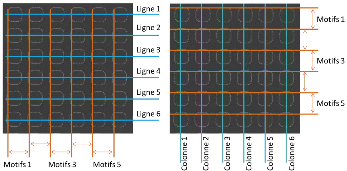
Figure 4-4 : Méthode de mesure du pas de réseau moyen suivant l'axe X (gauche) et suivant l'axe Y (droite) pour chaque colonne et ligne de motifs respectivement. Les colonnes de motifs sont numérotées de gauche à droite et les lignes de motifs sont numérotées de haut en bas. Les moyennes de pas de réseau sur chaque colonne sont calculées pour connaître les pas de réseau moyens en fonction du numéro de motifs.
