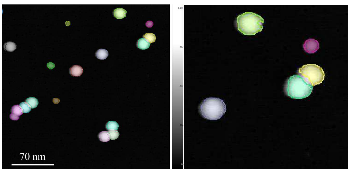
Figure 5-4 : Détection individuelle de particules agglomérées par la méthode de segmentation par partage des eaux (gauche, traitement effectué grâce à SPIP ©) et zoom (droite).
