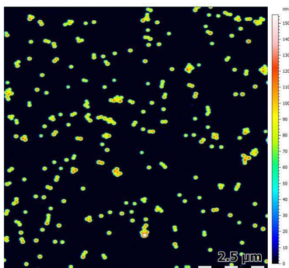
Figure 5-20 : Image AFM (topographie redressée) réelle utilisée pour montrer la performance de la méthode semi-automatique. La population de particules de SiO 2 déposée est monodisperse.
