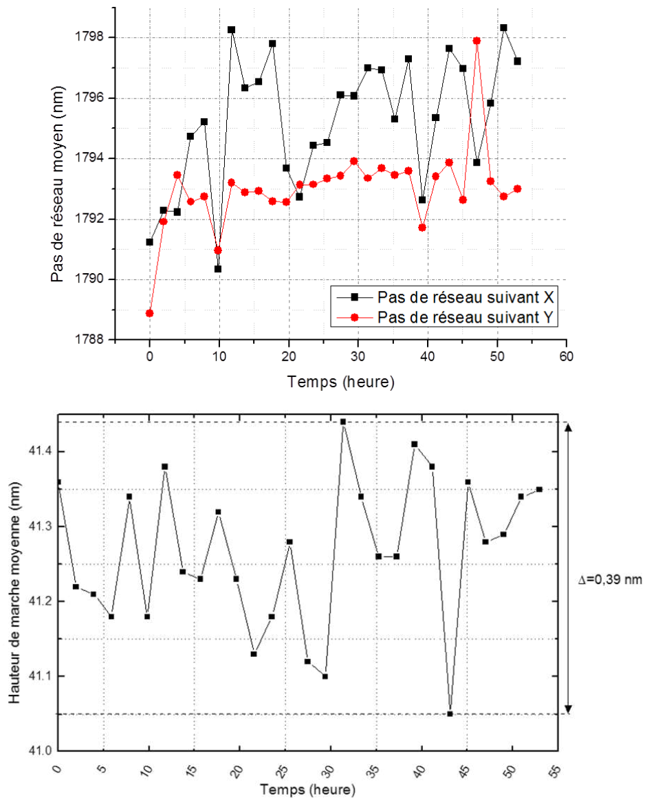
Figure 3-5 : Etude de reproductibilité : pas du réseau (haut) et hauteur de marche moyenne (bas) mesurés pour l'étalon STS2-440P à des positions différentes sur l'étalon.
