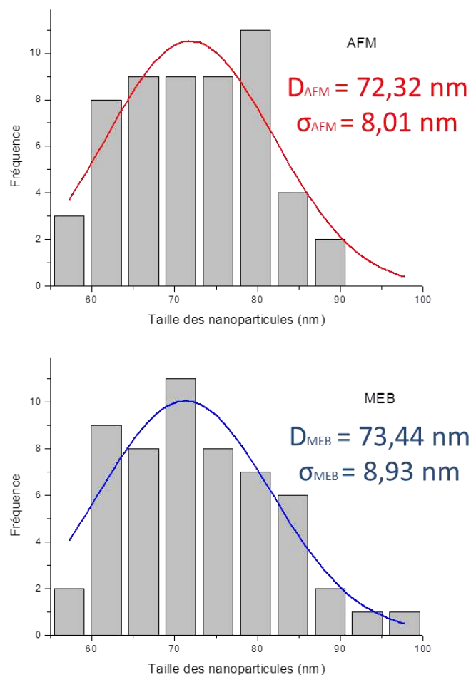
Figure 6-7 : Histogrammes de distribution en taille construits à partir des mesures obtenues par AFM et par MEB sur la population d'un même groupe de 55 nanoparticules de SiO 2 isolées (échantillon C).
