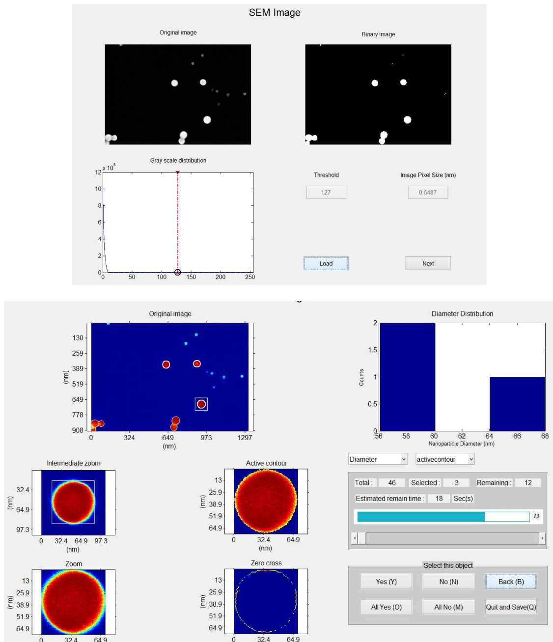
Figure 5-16 : Interfaces du programme Nanoselect : pour le chargement et la binarisation des images pour une image MEB (contraste topographique, détecteur In-Lens, haut), et pour la sélection des particules une à une.
