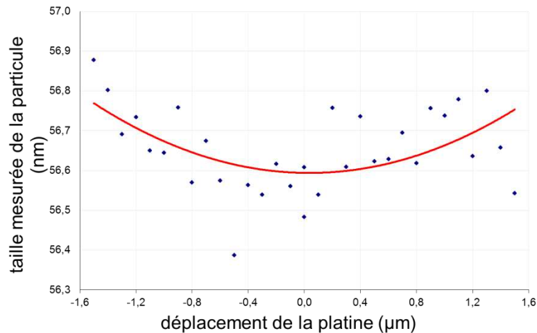
Figure 4-13 : Mesures de taille d'une nanoparticule en fonction de la défocalisation. Cette défocalisation est effectuée en faisant varier la position verticale de la platine porte-échantillon pas à pas (pas de 0,1 μm).
