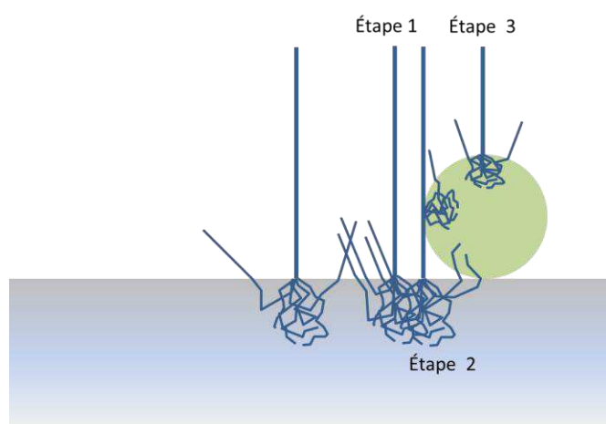
Figure 5-7 : Schéma représentant le balayage d'une particule déposée sur un substrat par un faisceau d'électrons en trois étapes.
