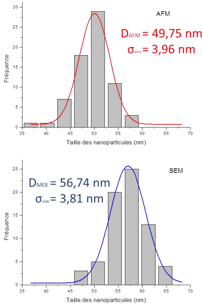
Figure 6-4 : Histogrammes de distribution en taille construits à partir des mesures obtenues par AFM et par MEB sur la population d'un même groupe de 70 nanoparticules d'or isolées (échantillon B).
