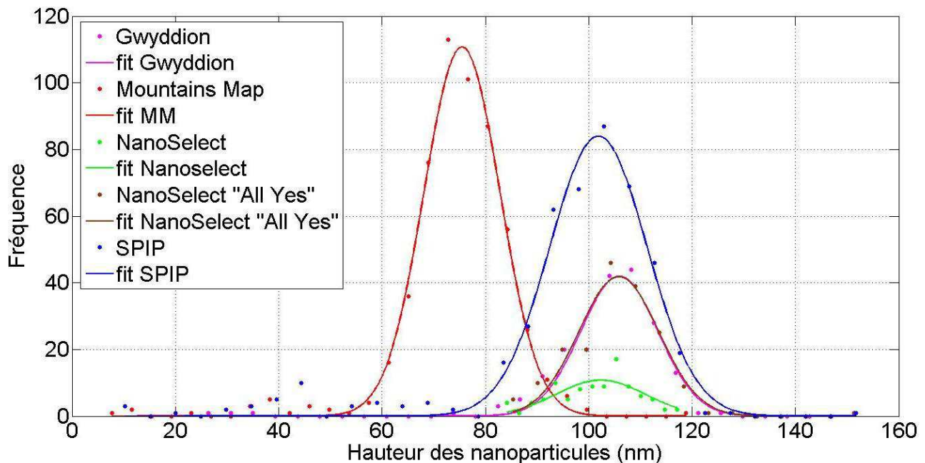
Figure 5-21 : Distributions en taille de la même image d'une population monodisperse de nanoparticules de \text{SiO}_2 obtenues par différents logiciels.
