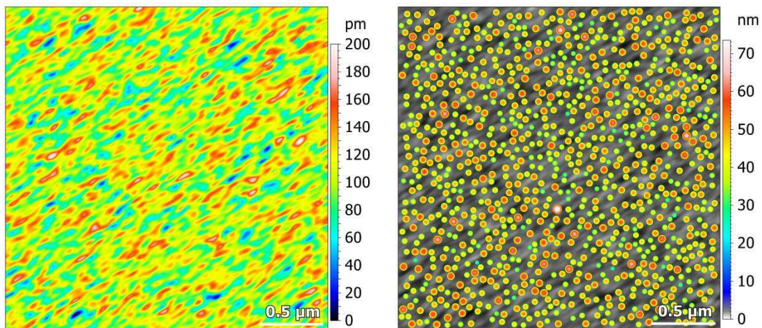
Figure 5-19 : Image simulée de la surface avec de la rugosité (2,5 \mu\text{m} x 2,5 \mu\text{m} – 2500 x 2500 pixel) (gauche) et image simulée du dépôt de particules sur cette surface simulée (droite).
