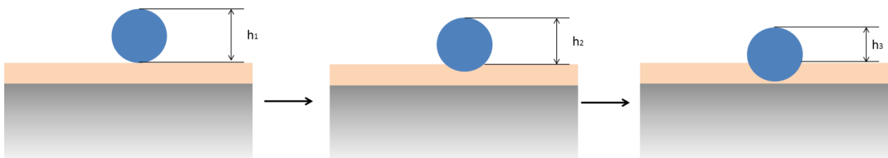
Figure 4-15 : Dégradation du « tapis » d'impuretés et impact sur la mesure de taille de nanoparticules par AFM.
