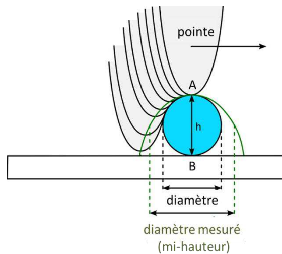
Figure 1-17 : Principe de mesure utilisé dans cette étude pour la mesure du diamètre d'une nanoparticule sphérique par AFM. Le trait vert correspond au trajet de la pointe sur l'échantillon, mettant en avant le phénomène de convolution pointe/surface.
