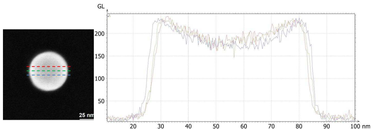
Figure 5-5 : Sélection d'un profil sur une image MEB pour l'obtention du diamètre de la particule de façon manuelle. L'erreur sur le choix du placement des profils a été amplifiée de façon à bien remarquer l'influence de ce dernier sur la mesure de diamètre.
