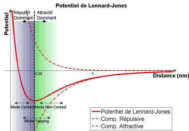
Figure 1-13 : Evolution de l'énergie potentielle entre la pointe AFM et la surface de l'échantillon en fonction de la distance qui les sépare 36 . Cette évolution suit le potentiel de Lennard-Jones.
