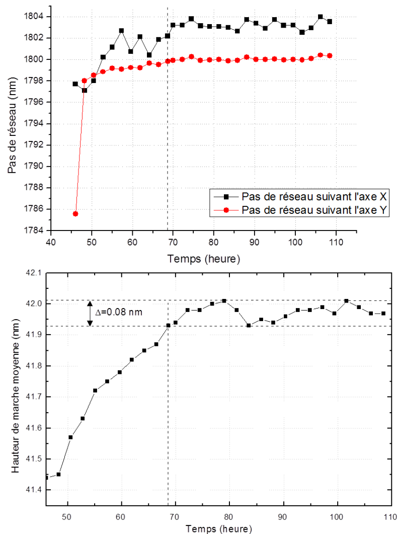
Figure 3-6 : Etude de répétabilité : suivi du pas moyen (haut) et de la hauteur de marche moyenne (bas) mesurés sur l'étalon STS2-440P sur une période de 65 heures, sur la même zone de l'étalon, et durant une période de stabilité thermique.
