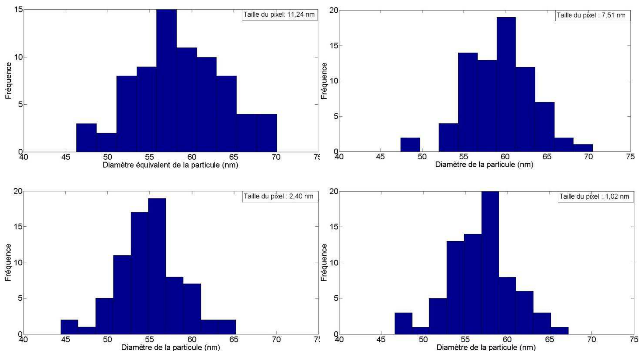
Figure 4-11 : Distribution en taille de 74 nanoparticules d'or imagées avec des tailles de pixel différentes. En haut à gauche, la taille du pixel est égale à 11,24 nm, en haut à droite, la taille du pixel est égale à 7,51 nm, en bas à gauche, elle est égale à 2,40 nm et en bas à droite, elle est égale à 1,02 nm.
