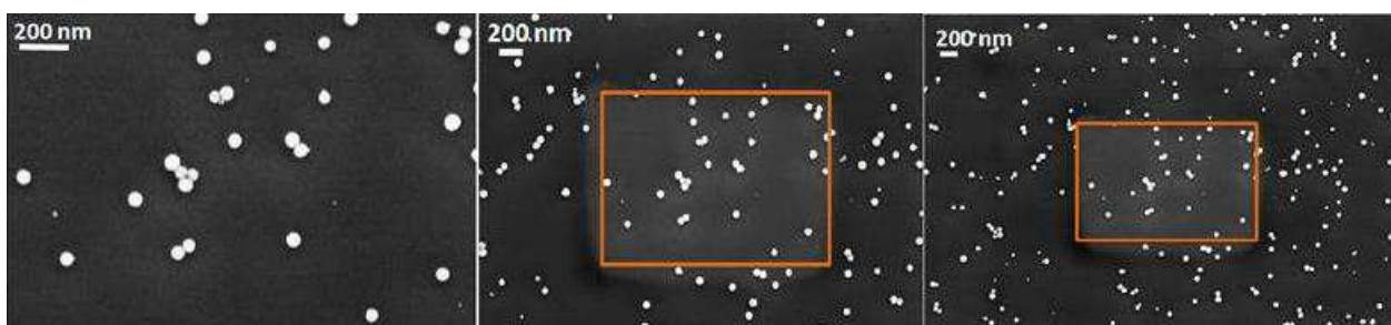
Figure 4-9 : Clichés MEB d'une même zone d'un échantillon de nanoparticules de SiO 2 déposé sur du silicium imagée avec trois résolutions différentes en conservant la même taille de pixel : (gauche) résolution de 1024 x 768 pixels, (centre) résolution de 2048 x 1536, et (droite) résolution de 3072 x 2304 pixels.
