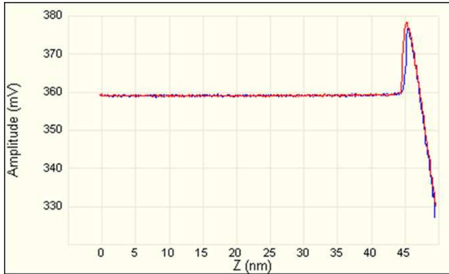
Figure 3-15 : courbe d'approche retrait d'une pointe de silicium OTESPA-R3 sur une particule de \text{SiO}_2 .
