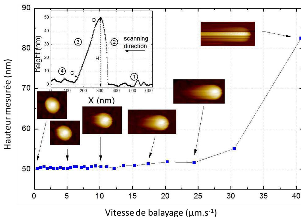
Figure 3-14 : Influence de la vitesse de balayage sur la mesure de hauteur de nanoparticules. En insert, un profil AFM de la particule étudiée pour une vitesse de balayage de 10 \mu\text{m}.\text{s}^{-1}
