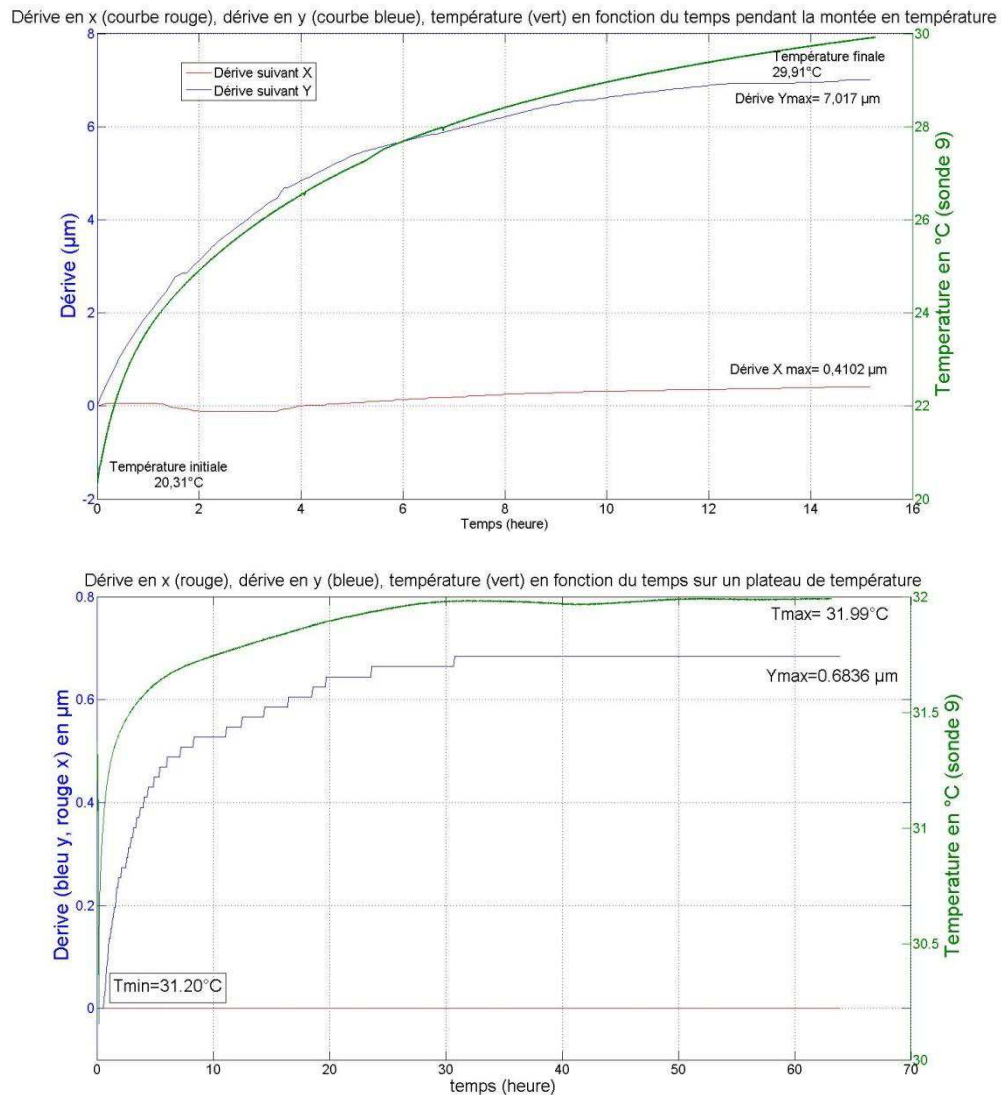
Figure 3-11 : Suivi des positions en X (rouge) et en Y (bleue) du motif représenté en Figure 3-10 ainsi que la température durant les deux phases de l'expérience : le graphique du haut correspond à la montée en température, et en bas sont reportées les données de fin de montée en température et du plateau. La température se stabilise donc au bout de 16+30 = 46 heures.
