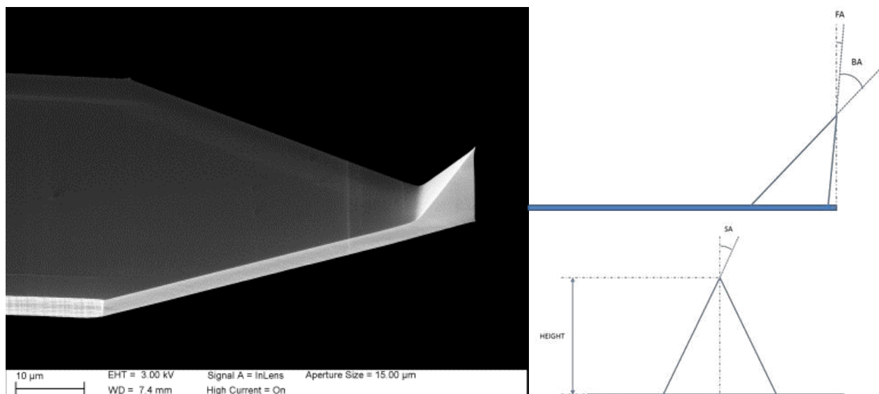
Figure 3-3 : Image MEB d'une pointe OTESPA (gauche) et schéma explicatif de ses spécificités (droite). Pour les pointes OTESPA-R3, les spécificités sont les suivantes : BA (Back Angle) = 35 \pm 1^{\circ} , FA (Front Angle) = 0 \pm 1^{\circ} , SA (Side Angle) = 18 \pm 1^{\circ} , Height (hauteur) comprise entre 9 \mu\text{m} et 19 \mu\text{m} .
