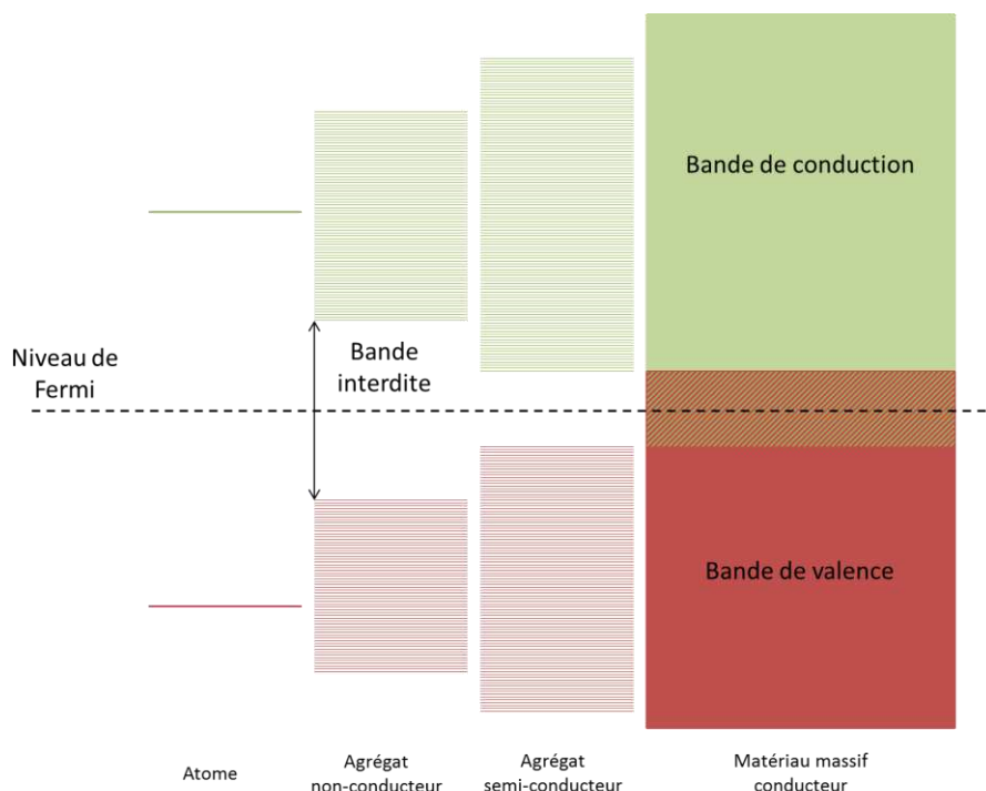
Figure 1-3 : Représentation schématisée des niveaux d'énergie de valence et de conduction d'un atome, d'agrégats de taille nanométrique et d'un matériau conducteur à l'état massif.
