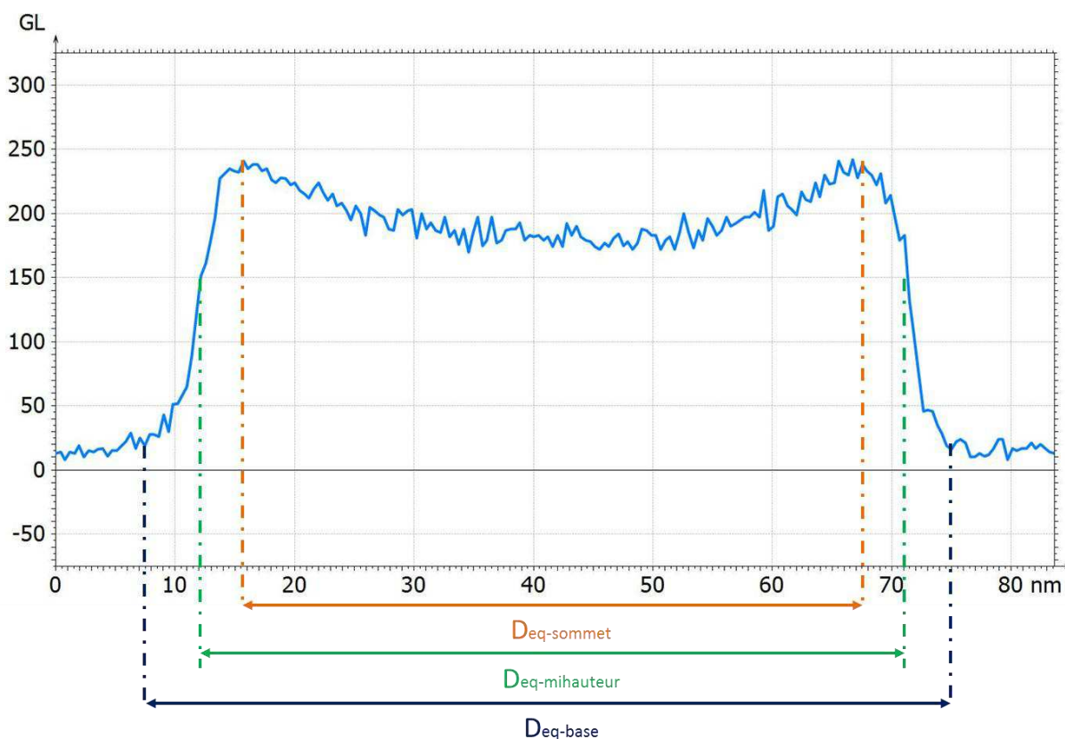
Figure 5-6 : Mesure du diamètre selon 3 critères différents : mesure prise à la base de la nanoparticule (bleu), mesure prise au sommet de la nanoparticule (rouge) et mesure prise à mi-hauteur de la nanoparticule (vert).
