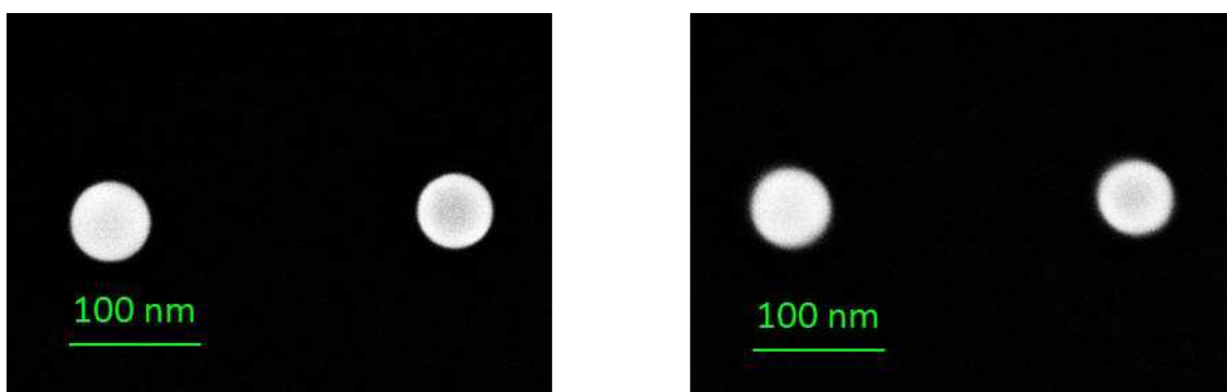
Figure 4-12 : Clichés MEB de nanoparticules de SiO 2 . A gauche, le faisceau d'électrons est focalisé sur l'échantillon, à droite, il est défocalisé (1,5 µm de déplacement vertical de la platine par rapport à son plan focal).
