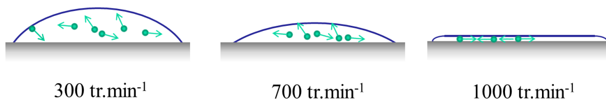
Figure 2-13 : Variation de l'épaisseur de la couche de solvant en fonction de la vitesse de rotation. A 300 tr.min -1 , le mouvement brownien est dominant. A 1000 tr.min -1 , les nanoparticules sont soumises aux forces de capillarités.
