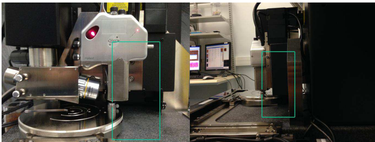
Figure 3-12 : Chaînes métrologiques suivant l'axe X (axe rapide/gauche) et suivant l'axe Y (axe lent/droite).
