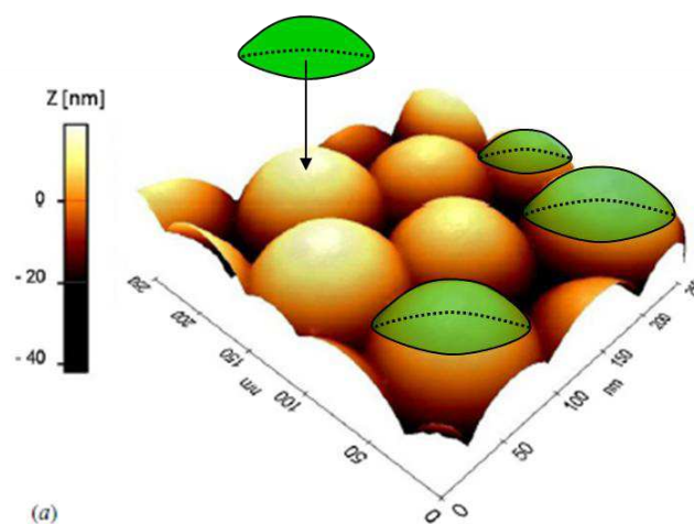
Figure 1-18 : Méthode de la « calotte sphérique » mise en œuvre par O. Couteau et G. Roebben (Commission Européenne, Joint Research Center, Institute for Materials and Measurements – IRMM, Belgique)
