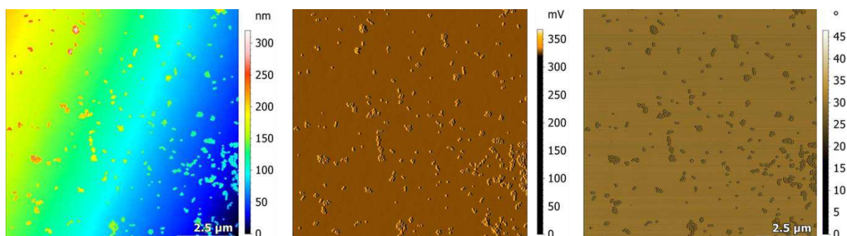
Figure 5-10 : Images AFM brutes. A gauche une image de topographie, la même image en amplitude et l'image de phase.
