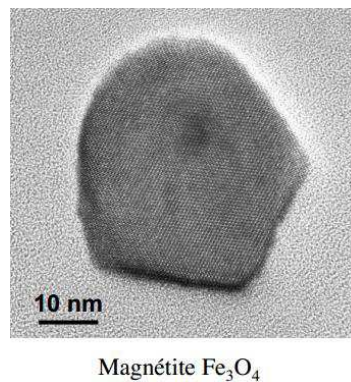
Figure 1-22 : Image d'une nanoparticule de magnétite \text{Fe}_3\text{O}_4 imagée par MET 56 .
