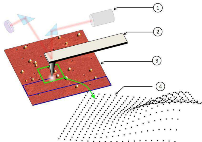
Figure 1-12 : Principe d'interaction pointe/échantillon avec ; (1) le système de détection des déflexions du levier, (2) ensemble levier/pointe, (3) échantillon à imager, (4) image de topographie mesurée.
