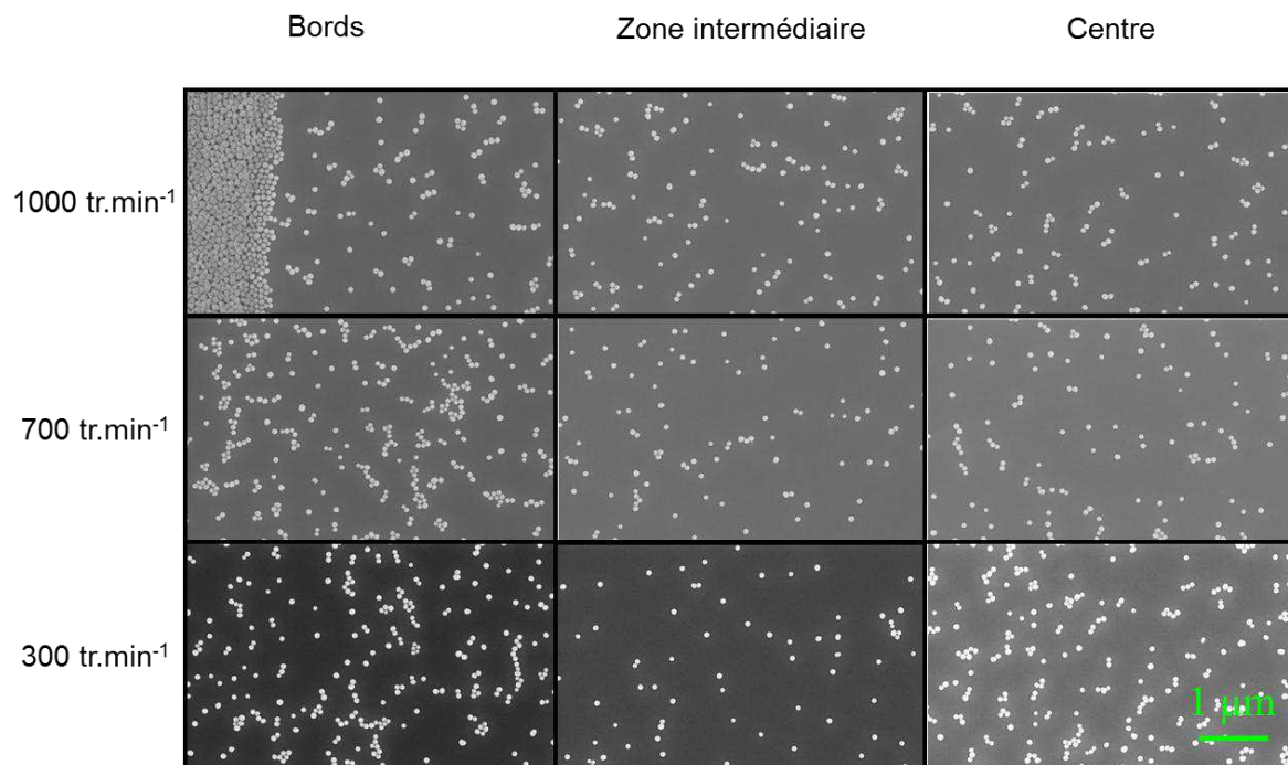
Figure 2-14 : Images MEB d'une population de SiO 2 déposée par spin-coating sur du silicium avec différentes vitesses de rotation lors de la première étape (étalement). Comme pour le mica, pour chaque échantillon, trois zones ont été mises en évidence : (i) les bords de l'échantillon (iii) le centre de l'échantillon, et (ii) une zone intermédiaire entre les zones (i) et (iii).
