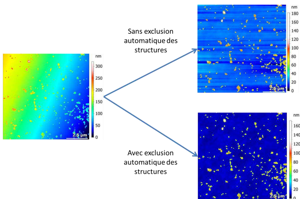
Figure 5-11 : Images topographiques issues de l'AFM. A gauche, l'image brute, à droite, les images redressées. En haut à droite, le redressement a été effectué ligne à ligne, sans exclusion automatique des structures. En bas à droite, le redressement a été effectué ligne à ligne avec exclusion automatique des structures (MountainsMap).
