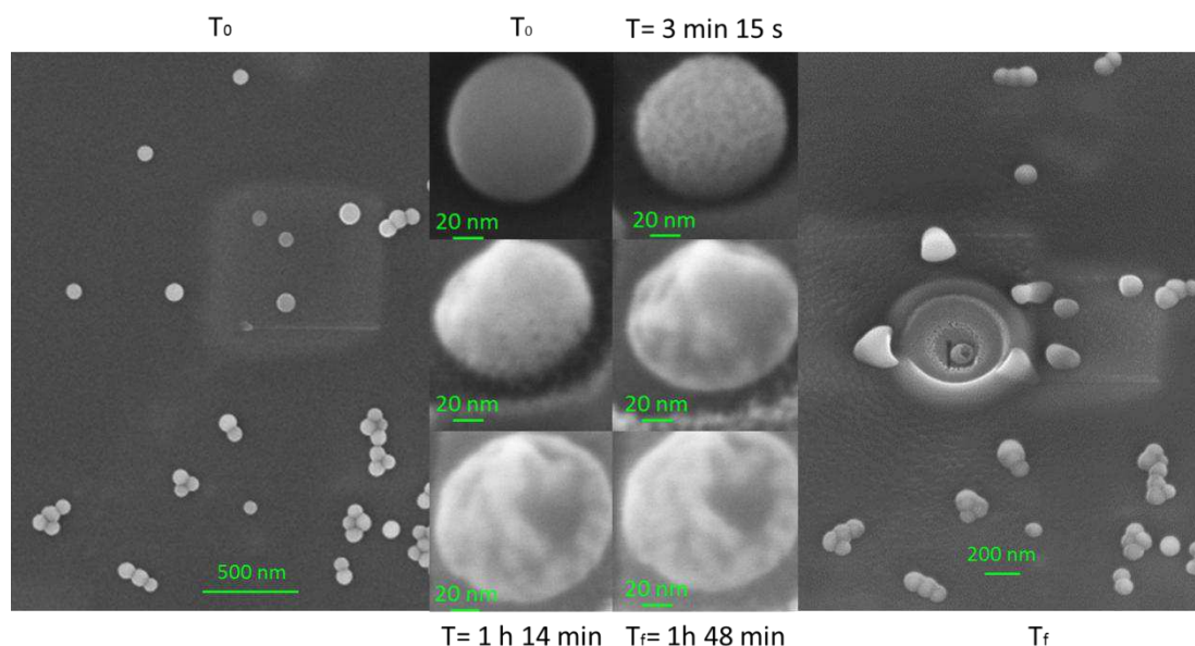
Figure 4-8 : Dégradation d'une nanoparticule de \text{SiO}_2 déposée sur du silicium et de son environnement proche. Nous pouvons observer que la zone où est posée la particule a également été dégradée.
