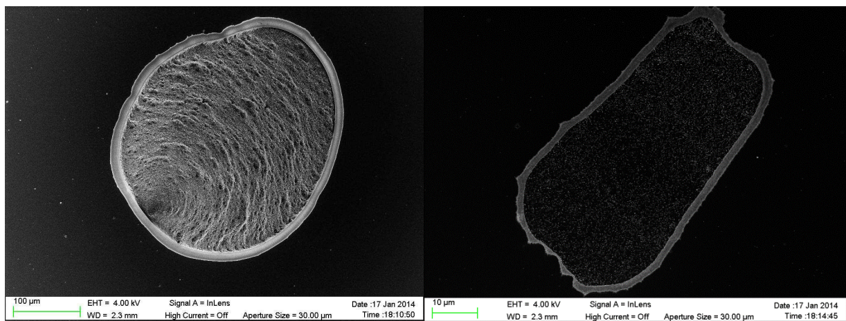
Figure 2-7 : Images MEB des « cercles » formés par le séchage de gouttelettes présentes sur les substrat de silicium.
