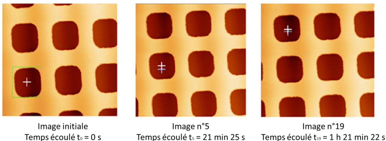
Figure 3-10 : Images AFM de l'étalon STS2-440P ( 5 \mu\text{m} \times 5 \mu\text{m} ) acquises en continu durant la phase de montée en température de l'électronique et traitées par WSxM (redressement et suivi des positions d'un motif grâce à la fonction « particlemovementanalysis »). Il n'a pas été demandé de mouvement en position sur l'échantillon, et seules les dérives expliquent les déplacements des motifs sur l'image. La croix blanche indique la position du centre du motif sur l'image en cours, la croix bleue indique la position du centre du motif sur l'image qui précède.
