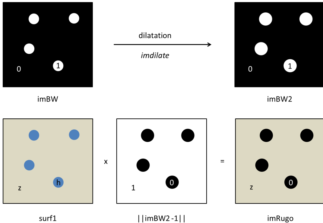
Figure 5-13 : Représentation schématique des calculs permettant d'obtenir une image de la rugosité en excluant les points correspondant aux nanoparticules représentés par des 0.
