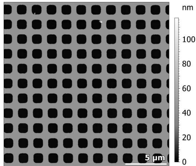
Figure 3-4 : Image AFM de l'étalon de transfert STS2-440P.
