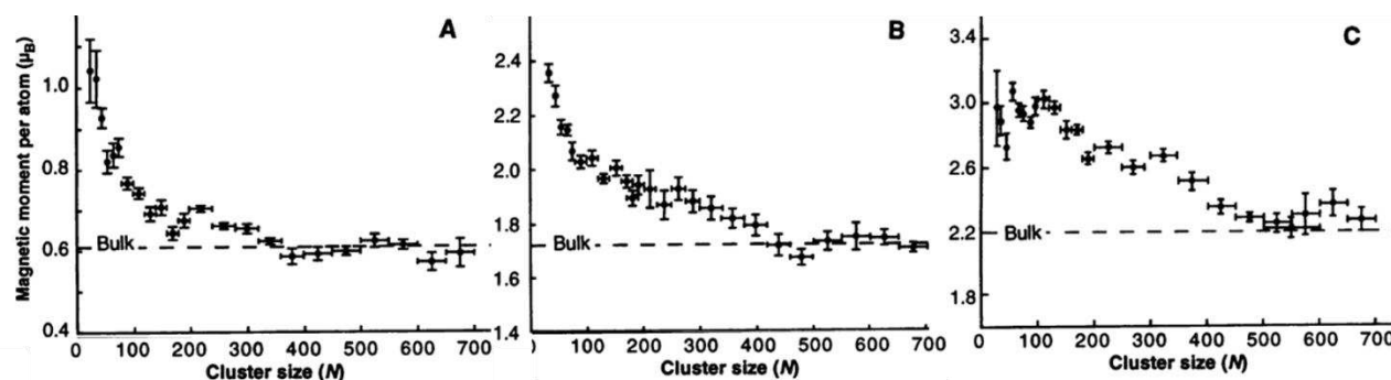
Figure 1-5 : Evolution du moment magnétique du Nickel (A), du Cobalt (B) et du Fer (C) en fonction de la taille des nanoparticules exprimée en nombre d'atomes.
