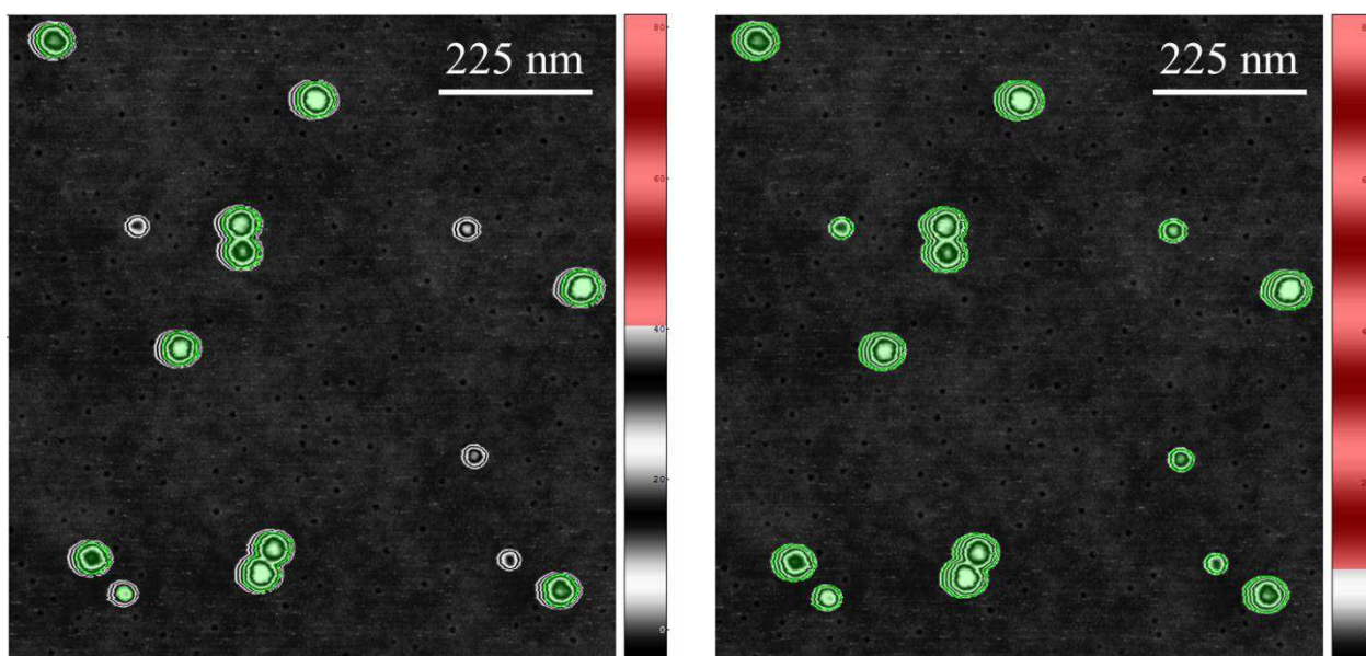
Figure 5-2 : Détection de particules par seuillage (logiciel SPIP©) avec deux valeurs de seuil différentes. Les éléments colorés en vert sont les éléments détectés. A gauche, le seuil a été placé à une valeur de 40 nm, toutes les particules ne sont pas détectées. A droite, le seuil a été placé à environ 10 nm, toutes les particules sont détectées. On notera que les particules agglomérées sont détectées en ne comptant que pour un seul élément.
