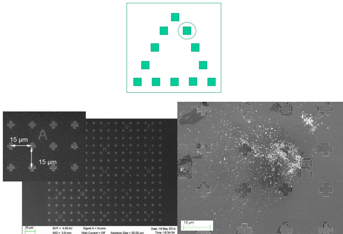
Figure 6-1 : Vue schématique de 12 motifs de localisation sur un substrat de 1 mm x 1 mm de silicium (haut). Image MEB (contraste topographie, détecteur In-Lens) d'une structure de localisation gravée sur un substrat de silicium (bas-gauche). Image MEB (contraste topographie, détecteur In-Lens) d'un dépôt de nanoparticules de SiO 2 sur un tel substrat (bas-droite).
