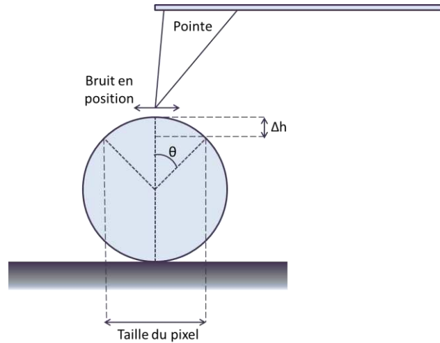
Figure 3-16 : Schéma représentant l'influence d'un mouvement de la pointe dans le plan sur la mesure de hauteur d'une nanoparticule sphérique.
