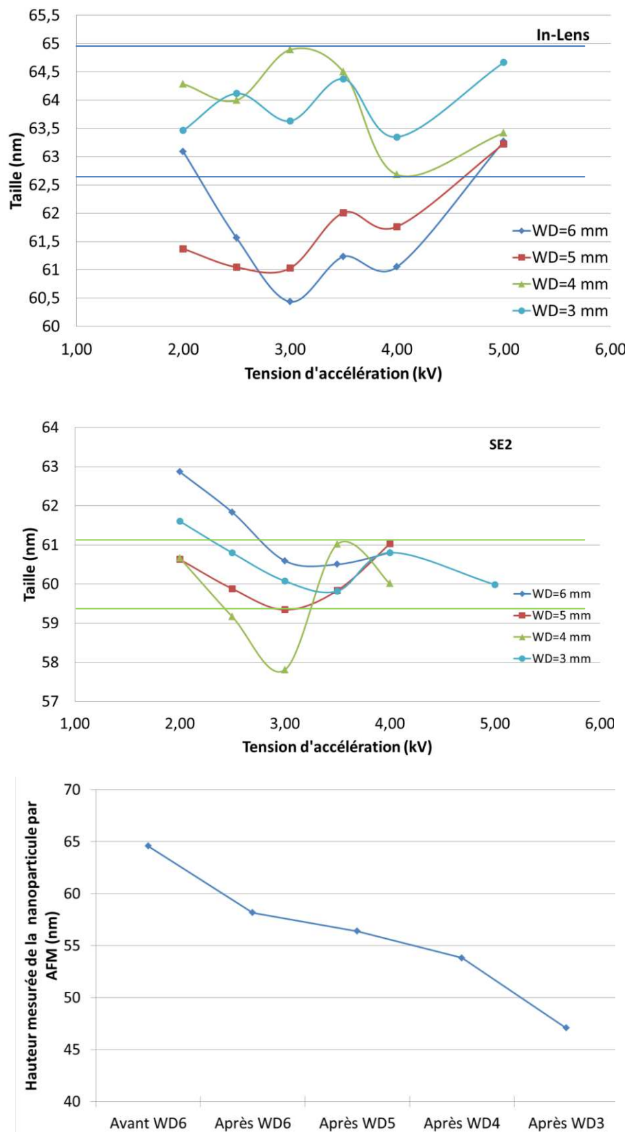
Figure 4-14 : Mesure de taille d'une même nanoparticule par MEB pour différentes distances de travail (WD, pour working distance) et différentes tensions d'accélération avec le détecteur In-Lens (haut) et avec le détecteur SE2 (centre). Contrôle de la dégradation de la nanoparticule ou de son environnement par AFM avant et après chaque série d'images à une distance de travail donnée.
