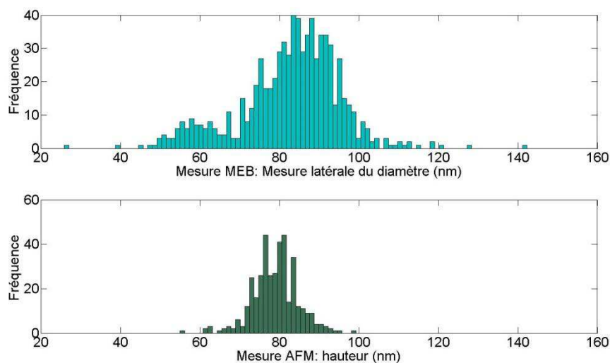
Figure 6-2 : Distribution en taille de nanoparticules de l'échantillon A obtenu par MEB (haut) et par AFM (bas).
