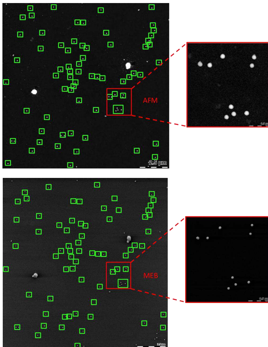
Figure 6-3 : Même groupe de 70 nanoparticules d'or déposées sur du mica (échantillon B), imagées par AFM (haut) et par MEB (bas). Sur la droite, un zoom montrant 9 nanoparticules imagées par AFM (haut) et par MEB (bas).
