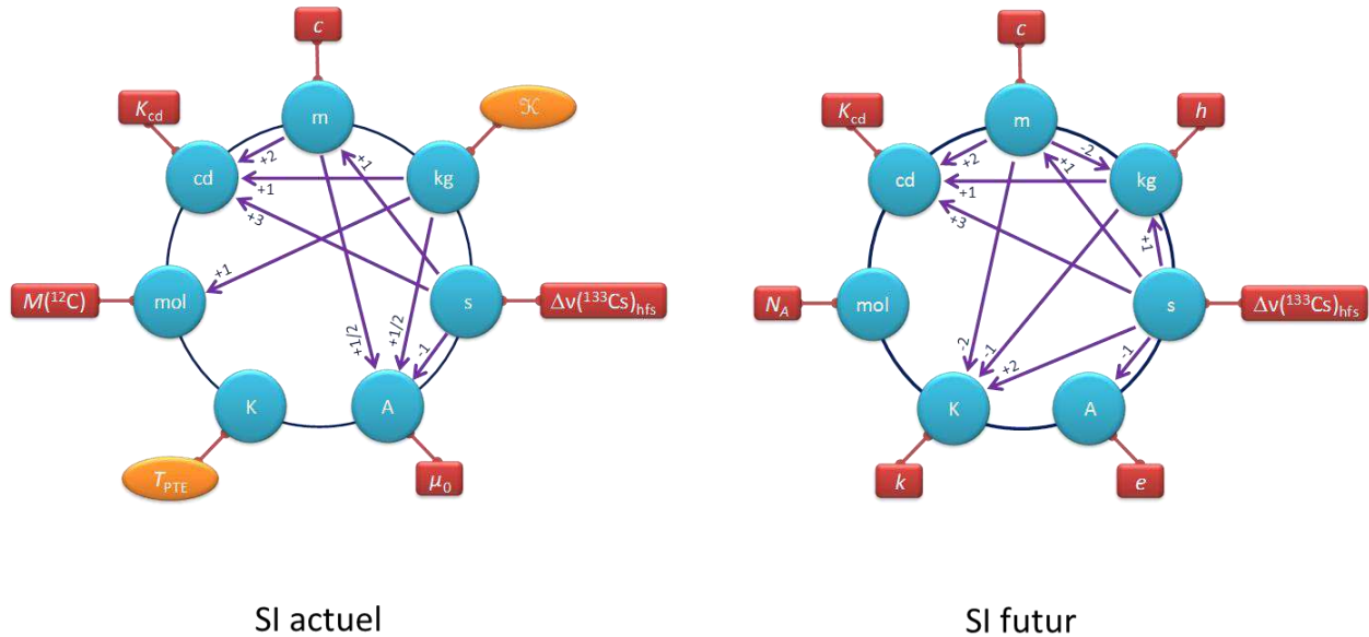
Figure 1-9 : Grandeurs du Système International d'unités actuel (gauche) et celui mis en œuvre uniquement à partir de constantes fondamentales dans les prochaines années(droite). Les sept unités de base sont : le mètre m (unité de longueur), le kilogramme kg (unité de masse), la seconde s (unité de temps), l'ampère A (unité d'intensité de courant électrique), le kelvin K (unité de température), la mole mol (unité mesurant la quantité de matière), et la candela cd (unité d'intensité lumineuse) 41 .
