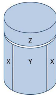
Figure 1-16 : Schéma d'un scanner d'AFM piézoélectrique générant des déplacements dans les trois directions de l'espace. Les céramiques notés X et Y permettent les déplacements latéraux et celle notée Z permet les déplacements verticaux.
