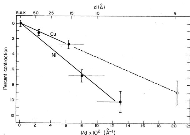
Figure 1-6 : Evolution de la distance entre les atomes (paramètre de maille) pour des particules de Nickel et de Cuivre en fonction de la taille des nanoparticules 13 .
