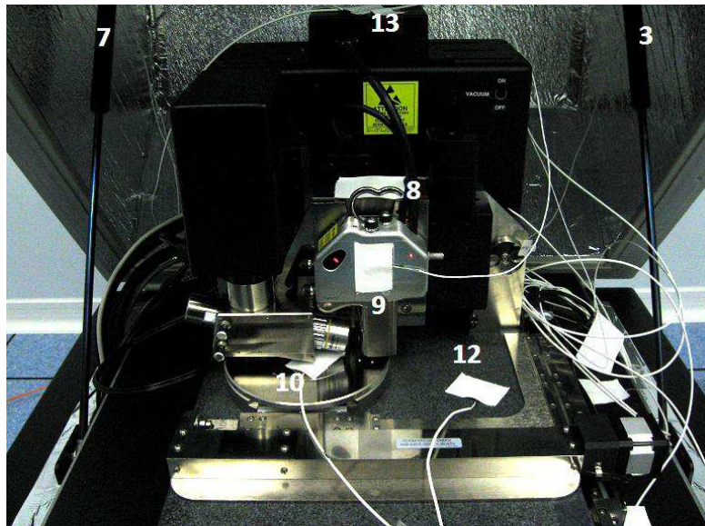
Figure 3-8 : photographie de l'AFM et du caisson le contenant montrant les sondes de températures mises en place pour la corrélation dérive de l'instrument- température.
