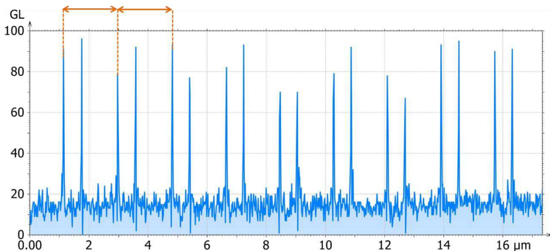
Figure 4-3 : Profil d'une image MEB d'un réseau étalon avec l'apparition de pics en niveau de gris sur les bords des motifs. La mesure d'un pas de réseau correspond à la distance entre deux pics non consécutifs.
