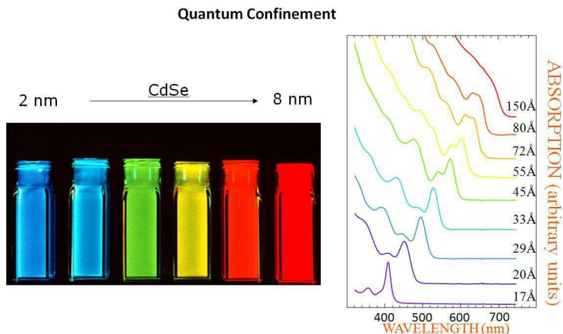
Figure 1-4 : Observation de la modification des propriétés optiques en fonction de la taille des particules : photographie de suspensions colloïdales de CdSe observées en fluorescence et spectre d'absorption de particules de CdSe en fonction de la taille de celles-ci 10 .
