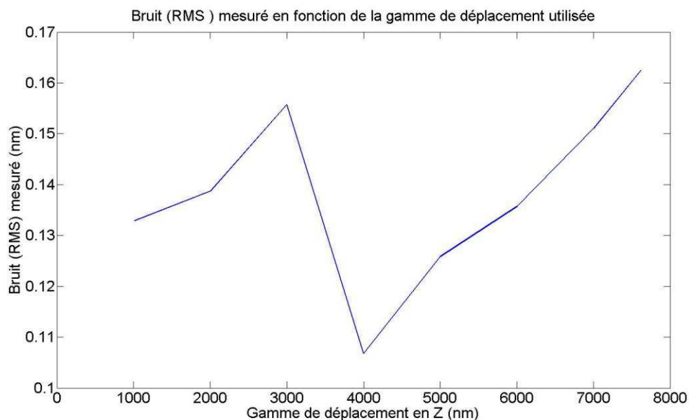
Figure 3-7 : Bruit RMS en fonction de la gamme de déplacement (Z-Range) utilisée.
