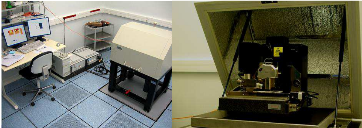
Figure 3-2 : Photographies des protections acoustiques et vibratoires mises en œuvre sur l'AFM du LNE (Dimension V, Veeco).
