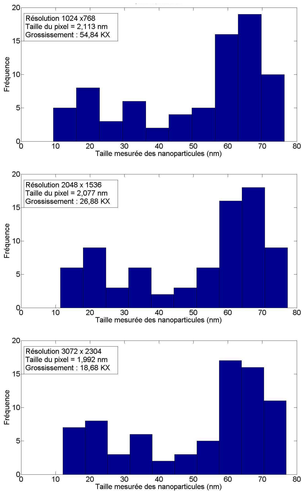
Figure 4-10 : Histogrammes en taille de nanoparticules de SiO 2 images par MEB avec trois grossissements différents en fixant la taille de pixel(haut). Pour une résolution de 1024 x 768 pixels, (centre) pour une résolution de 2048 x 1536 pixels, et (bas) pour une résolution de 3072 x 2304 pixels.
