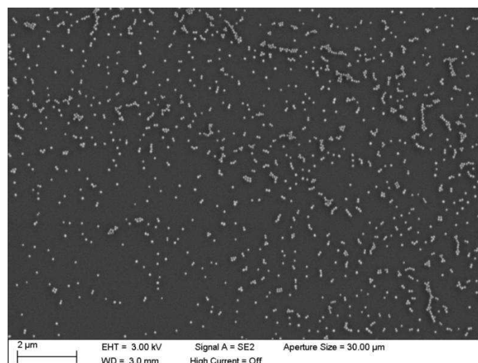
Figure 2-9 : image MEB d'un échantillon de particules de \text{SiO}_2 obtenu par évaporation d'une gouttelette forcée par air comprimé.
