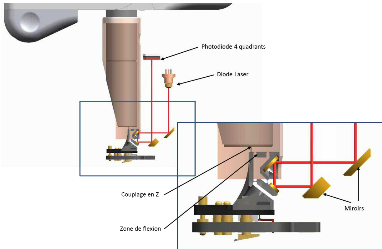
Figure 3-1 : Vue schématique simplifiée de la tête hybride du Dimension Nanoman V.
