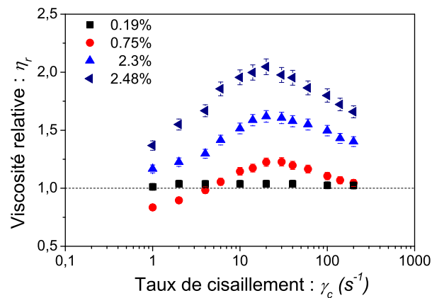
FIGURE 6.12 – Viscosité relative \eta_r de suspensions bactériennes en fonction du taux de cisaillements \dot{\gamma}_c et pour plusieurs fraction volumique \phi .
