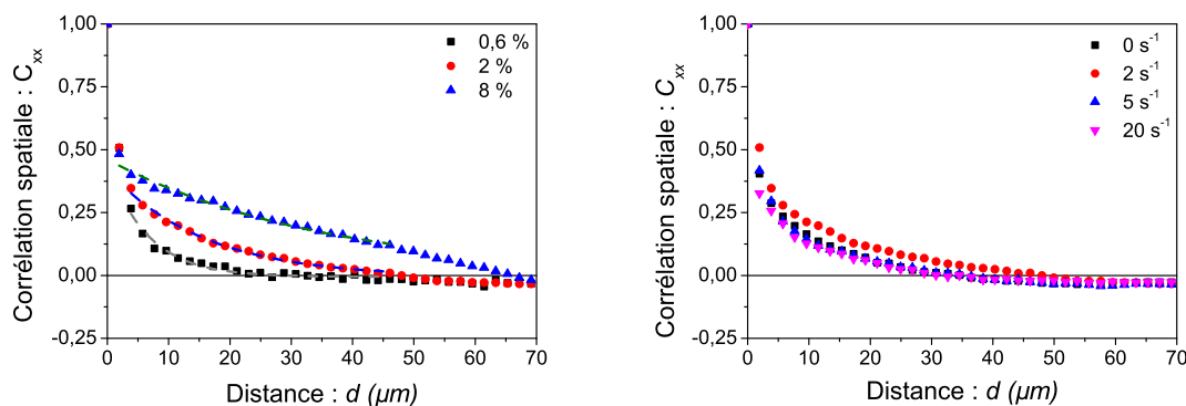
FIGURE 5.17 – Fonctions de corrélation spatiale. À gauche : cas pour un gradient de vitesse \dot{\gamma}_c = 2 \text{ s}^{-1} et pour différentes fractions volumiques \phi = 2\% au centre du canal. Pointillés : ajustement par une exponentielle décroissante. À droite : cas pour une fraction volumique \phi = 2\% et pour différents gradients de vitesse \dot{\gamma}_c au centre du canal.
