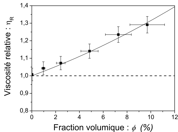
FIGURE 6.6 – Mesure de viscosité relative dans le cas de billes de 2 \mu\text{m} de diamètre à un taux de cisaillement caractéristique \dot{\gamma} = 5 \text{ Hz} . La courbe pleine correspond à une loi de Batchelor (6.7).
