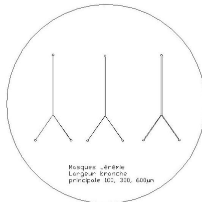
FIGURE 6.18 – Exemple de dessin CAO. Cas de canaux pour viscosimétrie de 100, 300 et 600 µm de large
