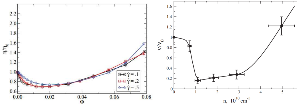
FIGURE 1.24 – Viscosité relative en fonction de la fraction volumique pour des taux de cisaillement faibles. À gauche : simulations numériques [37]. À droite : expérience utilisant des Bacillus subtilis [39].
