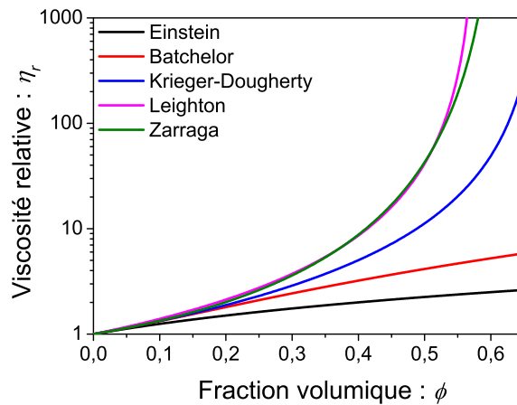
FIGURE 1 – Viscosité relative \eta_r donnée par les modèles d'Einstein [1], de Batchelor [2], ainsi que les fits empiriques de Krieger-Dougherty [3], de Leighton [4], et de Zarraga [5].
