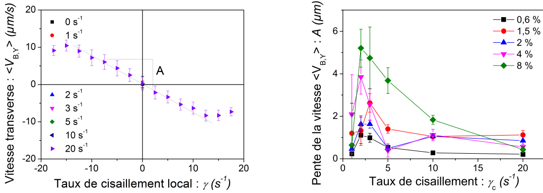
FIGURE 5.14 – Mesure de la pente A de la vitesse transverse et courbe en fonction du taux de cisaillement caractéristique imposé \dot{\gamma}_c .
