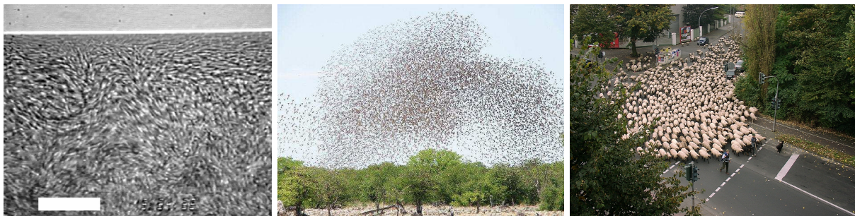
FIGURE 3.1 – À droite : image de Bacillus Subtilis près d'une ligne de contact, l'échelle mesure 35\ \mu\text{m} [58]. Au centre : vol en essaim de travailleurs à bec rouges CC : Alastair Rae . À gauche : troupeau de moutons à Cologne CC : Túrelío .
