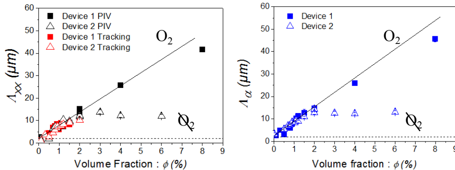
FIGURE 3.11 – À gauche : longueurs de corrélations de vitesses \Lambda_{xx} en fonction de la fraction volumique \phi pour deux méthodes de traitement et pour deux approvisionnement différents en oxygène. À droite : longueurs de corrélations des orientations \Lambda_{\alpha} pour les mêmes expériences.
