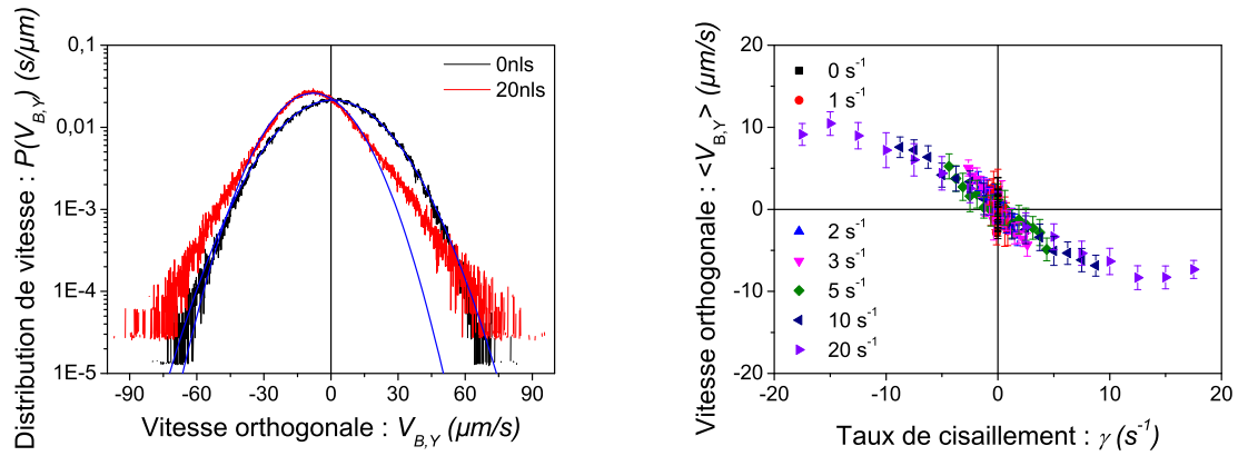
FIGURE 5.13 – À gauche : Distributions des vitesses transverses des bactéries pour \phi = 2\% à H/4 et à deux débits différents. À droite : vitesse transverse moyenne des bactéries en fonction du gradient de vitesse local \dot{\gamma} dans l'écoulement de Poiseuille et pour plusieurs taux de cisaillement caractéristiques imposés \dot{\gamma}_c .
