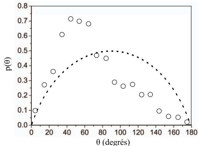
FIGURE 1.6 – Distribution de l'angle en sortie de tumble basé sur les résultats de Berg. Cercles : résultats expérimentaux [8]. Pointillés : courbe correspondant à une réorientation isotrope dans l'espace ( p(\theta) = \frac{1}{2} \sin \theta ).
