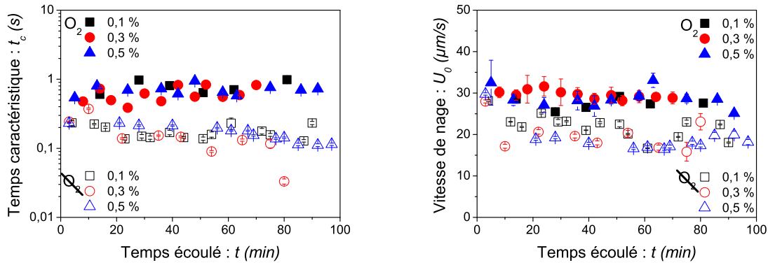
FIGURE 2.5 – Variation de l'activité de Escherichia Coli avec et sans apport en oxygène et en présence de L-Sérine à une concentration de 250mM. À gauche : temps caractéristique de nage t_c en fonction du temps écoulé t . À droite : vitesse de nage 3D U_0 en fonction du temps t dans la même situation.
