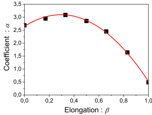
FIGURE 4.10 – Coefficient \alpha en fonction de l'élongation \beta des nageurs pour V_0/U_0 = 13 .
