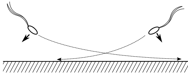
FIGURE 1.10 – Schéma de l'absorption des bactéries aux parois.
