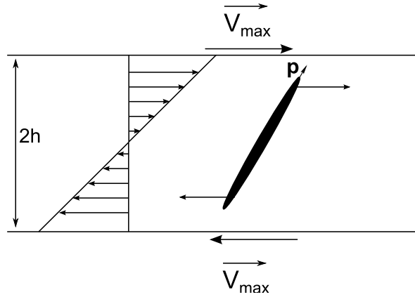
FIGURE 1.18 – Bâtonnet soumis à un cisaillement
