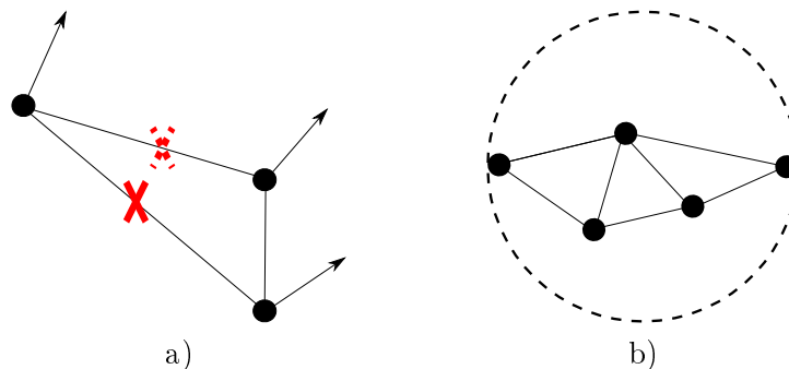
FIGURE 3.14 – a) : Schéma du test sur les couples d'un triangle dont l'un des liens ne respecte pas le critère imposé. Dans le cas des éléments-couples , les deux liens respectant le critère sont acceptés. Dans le cas des éléments-triangles , seul est conservé celui qui respecte le plus le critère. b) : Schéma d'un cluster comprenant N = 5 particules et dont l'extension \Delta est définie comme le diamètre du cercle en pointillés.
