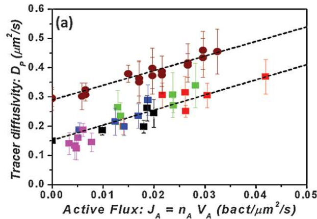
FIGURE 1.11 – Coefficient de diffusion en fonction du flux actif. Carrés : d = 2\mu\text{m} , cercles : d = 1\mu\text{m} [51]. Pointillés : courbes théoriques.
