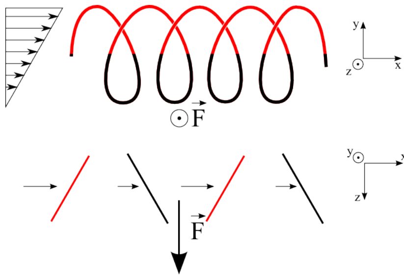
FIGURE 1.19 – Schéma de la rhéotaxie dans le cas de particules chirales simples. En haut : vue générale. En bas : schéma explicatif, vue de dessus simplifiée.
