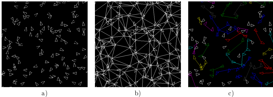
FIGURE 3.15 – Exemple du résultat de l'algorithme de tracking pour une fraction volumique \phi = 2\% et un angle \delta\theta = 25^\circ . a) Résultats de la détection. b) Triangulation de Delaunay. c) Clusters finaux, les triangles blancs représentant les bactéries solitaires. Les triangles indiquent la direction de nage.
