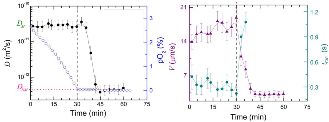
FIGURE 1.7 – Diffusivité D , vitesse de nage V , temps caractéristique t_{\text{run}} et taux d'oxygène en fonction du temps pour une même expérience. À gauche : diffusion de E. Coli RP437 et taux d'oxygène présent en solution en fonction du temps. À droite : vitesse de nage, et temps caractéristique t_{\text{run}} en fonction du temps [12].
