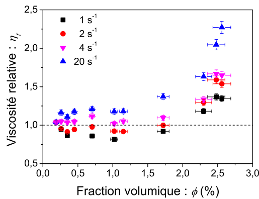
FIGURE 6.13 – Viscosité relative \eta_r de suspensions bactériennes en fonction de la fraction volumique \phi et pour plusieurs taux de cisaillements \dot{\gamma}_c .
