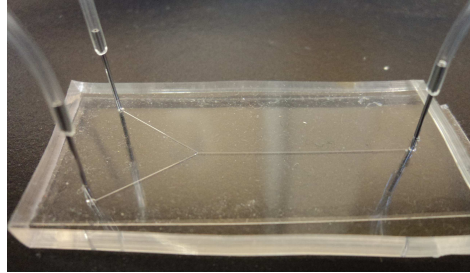
FIGURE 6.4 – Puce microfluidique utilisée pour nos expériences.
