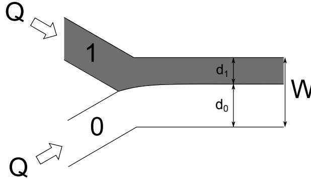
FIGURE 6.1 – Principe de fonctionnement du rhéomètre microfluidique. Ici la largeur du fluide 1 est inférieure à celle du fluide 0, il a donc une viscosité plus faible.
