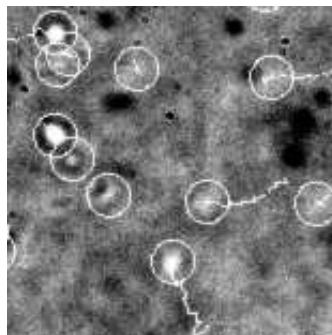
FIGURE 3.6 – Exemples de trajectoires obtenues par le tracking pour \phi = 0.1\% .
