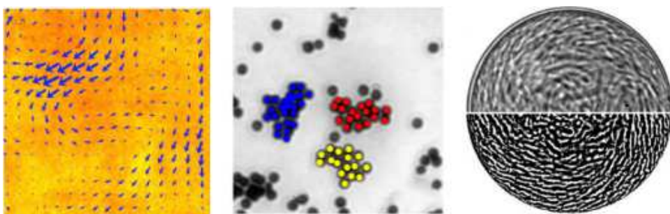
FIGURE 3 – À gauche : mouvements collectifs d'une suspension de Bacillus Subtilis (champ de 300 \mu\text{m} ) [31]. Au centre : Particules Janus sphériques sur un plan horizontal (champ de 35 \mu\text{m} ) [33]. À droite : Bacillus subtilis dans un réservoir de 70 \mu\text{m} [32].
