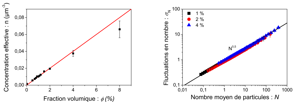
FIGURE 3.7 – À gauche : concentration volumique en bactérie mesurée par traitement d'image en fonction de la fraction volumique mesurée par absorption préalablement à l'expérience. La droite correspond à un accord pour un volume bactérien de 1\ \mu\text{m}^3 . À droite : fluctuations de densité en fonction de la densité moyenne pour différentes fractions volumiques. La droite correspond à une loi d'échelle en N^{0.5} .
