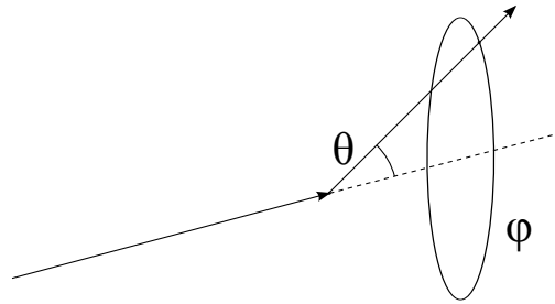
FIGURE 4.2 – Schéma d'un tumble actif.
