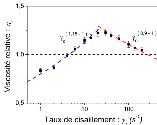
FIGURE 6.16 – Viscosité relative \eta_r de suspensions bactériennes en fonction du taux de cisaillements \dot{\gamma}_c et pour une fraction volumique \phi = 0.8\% ainsi que les ajustements à faibles et fort cisaillement selon la loi de Ostwald-de Waele.
