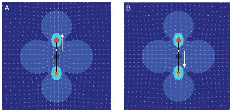
FIGURE 1.9 – Schémas de dipôles de force et des champs induits [20]. A) Cas d'un puller, B) Cas d'un pusher
