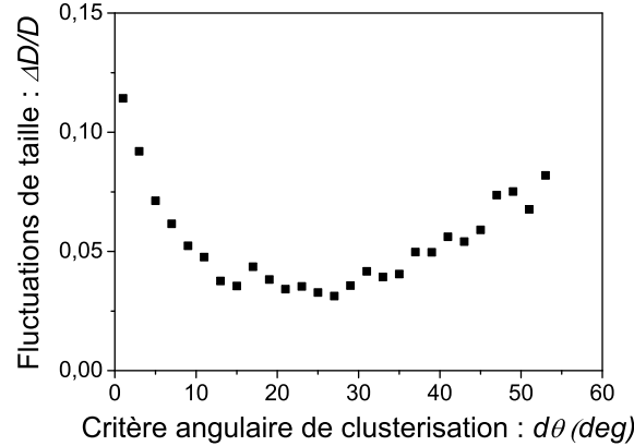
FIGURE 3.16 – Fluctuations de l'extension des clusters pour différents \delta\theta et \phi = 1\% .
