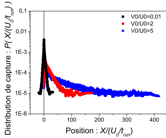
FIGURE 4.11 – Probabilité p(x) pour un nageur d'être entrée en contact avec la paroi à une distance x . Simulations pour \beta = 0.33 , R = 5 , t_{\text{run}} = 1 , U_0 = 1 , et pour V_0 = 0.01, 2 , et 5 .
