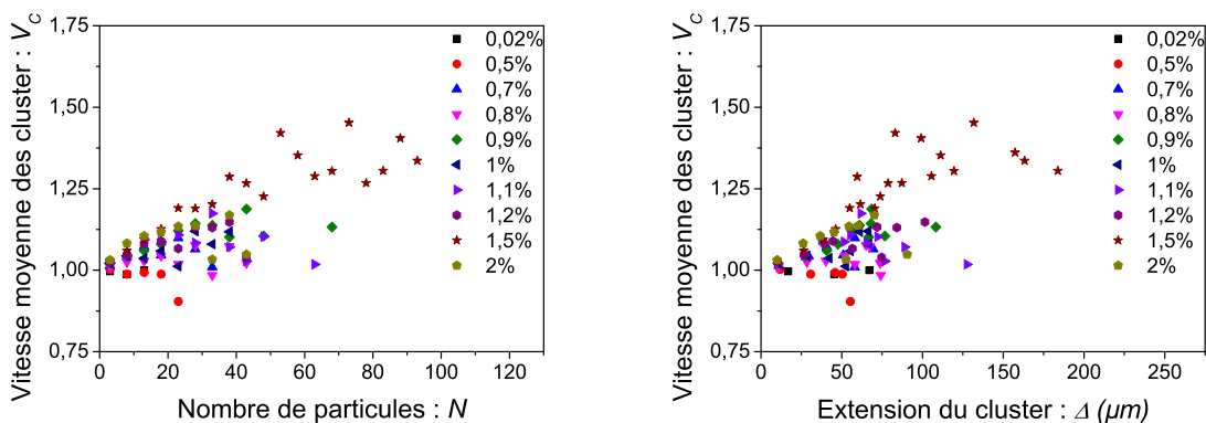
FIGURE 3.20 – Vitesse de déplacement du centre de masse des clusters en fonction de leurs tailles et pour différentes fraction volumiques dans le cas bactéries. À gauche : variation avec la taille en nombre de particules. À droite : variation en fonction de la taille en unité de longueur.
