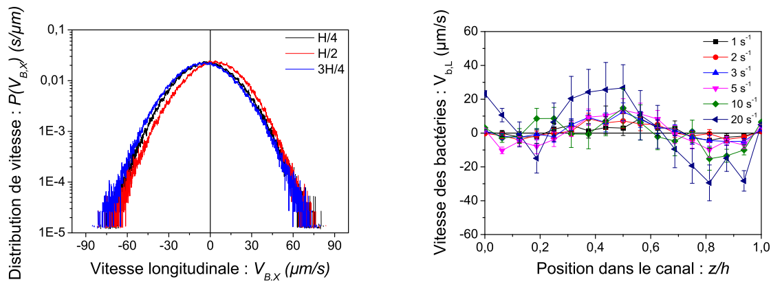
FIGURE 5.12 – À gauche : distributions de vitesse des bactéries dans le repère lagrangien pour d'une fraction volumique \phi = 2\% et pour un taux de cisaillement imposé \dot{\gamma}_c = 20\ \text{s}^{-1} à différentes hauteurs. À droite : profils de vitesse longitudinale des bactéries dans le repère lagrangien pour une fraction volumique de E. Coli \phi = 2\% et plusieurs taux de cisaillement \dot{\gamma}_c .
