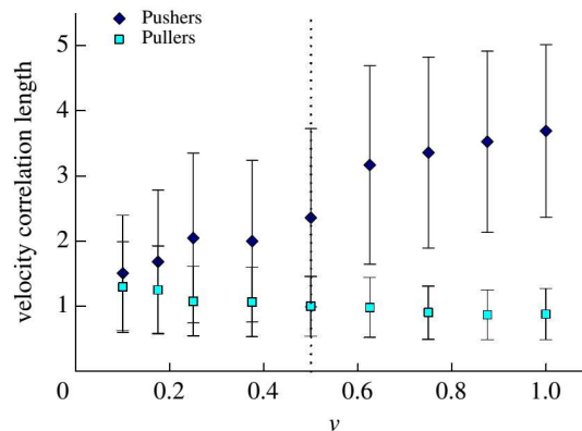
FIGURE 1.14 – Longueur de corrélation des vitesses en fonction de la fraction du volume exclu [26].
