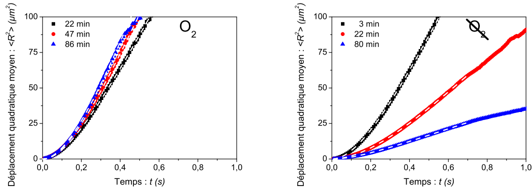
FIGURE 2.2 – Déplacement quadratique moyen des E. Coli pour une fraction volumique \phi = 0.3\% et sans L-Serine à trois temps t différents après le scellement complet de l'échantillon. À gauche : cas oxygéné (PDMS). À droite : cas non-oxygéné (parois en verre).
