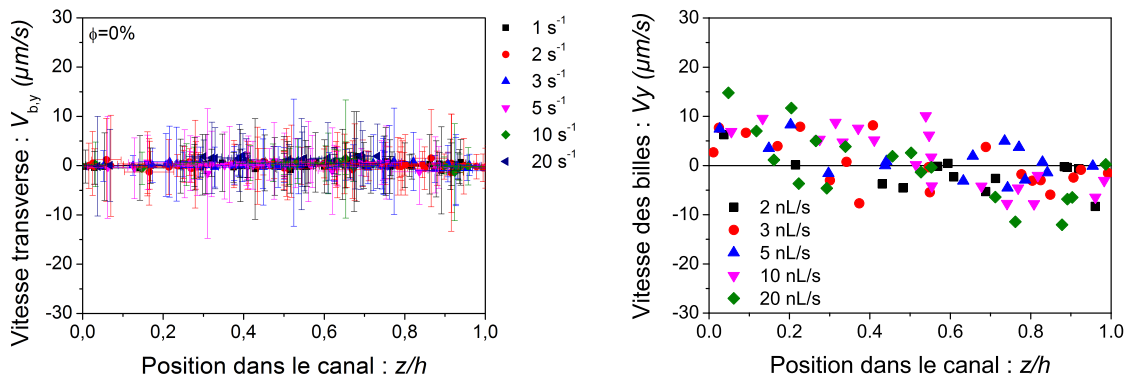
FIGURE 5.3 – Profils de vitesse transversale de traceurs passifs dans le cas d’une fraction volumique de E. Coli \phi = 0\% et \phi = 2\% et pour plusieurs débits imposés.
