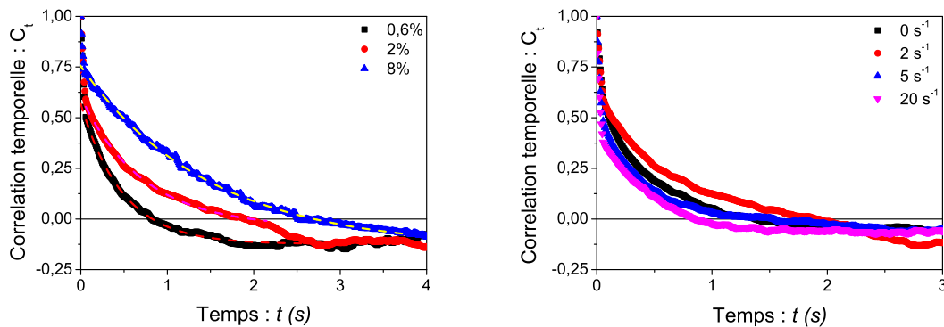
FIGURE 5.20 – Fonctions de corrélation temporelle. À gauche : cas pour un gradient de vitesse \dot{\gamma}_c = 2 \text{ s}^{-1} et pour différentes fractions volumiques \phi au centre du canal. Pointillés : ajustement par une exponentielle décroissante. À droite : cas pour une fraction volumique \phi = 2\% et pour différents gradients de vitesse \dot{\gamma}_c au centre du canal.
