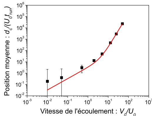
FIGURE 4.12 – Distance moyenne \langle x \rangle / (U_0 t_{\text{run}}) de contact avec la paroi en fonction de la vitesse de l'écoulement V_0/U_0 . Courbe pleine : ajustement des données avec le modèle.
