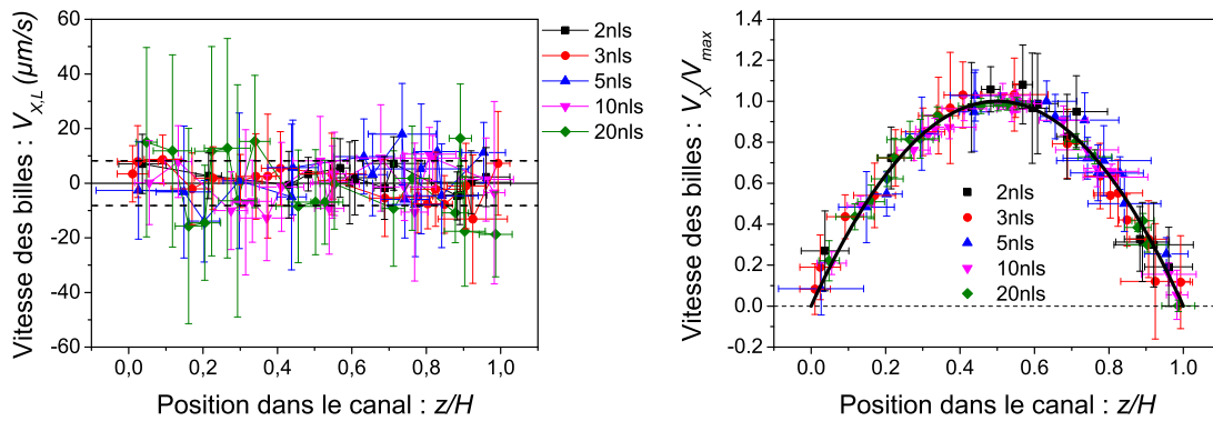
FIGURE 5.2 – Profils de vitesse longitudinale de traceurs passifs dans le cas d’une fraction volumique de E. Coli \phi = 2\% et pour plusieurs débits imposés. À gauche : repère lagrangien. À droite : repère eulérien.
