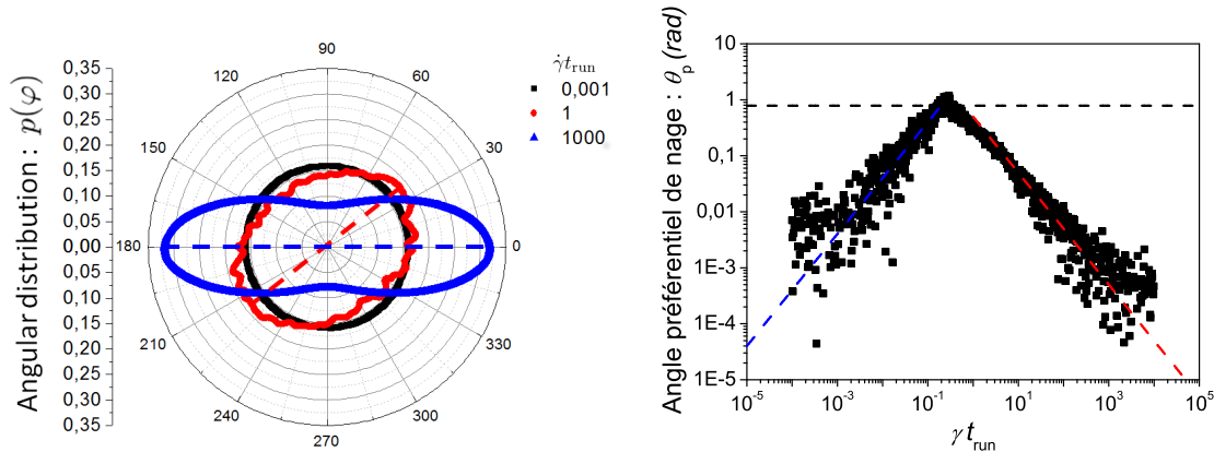
FIGURE 4.7 – Distributions et angle préférentiel d'ellipsoïdes d'élongation \beta = 0.6 en fonction du paramètre \dot{\gamma}t_{\text{run}} . Pointillés noirs : \pi/4 . Pointillés bleus et rouges : lois de puissance en (\dot{\gamma}t_{\text{run}})^{\pm 1} .
