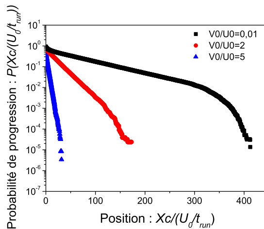
FIGURE 4.13 – Probabilité d'être en suspension après avoir parcouru une distance x/(U_0 t_{\text{run}}) . Simulations pour \beta = 0.33 , R = 5 , t_{\text{run}} = 1 , U_0 = 1 , et pour V_0 = 0.01, 2 , et 5 .
