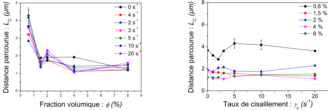
FIGURE 5.10 – Évolution de la distance parcourue par les bactéries projetée dans le plan focal L_c . À gauche : variation avec la concentration \phi en E. Coli. À droite : variation avec le taux de cisaillement \dot{\gamma}_c .
