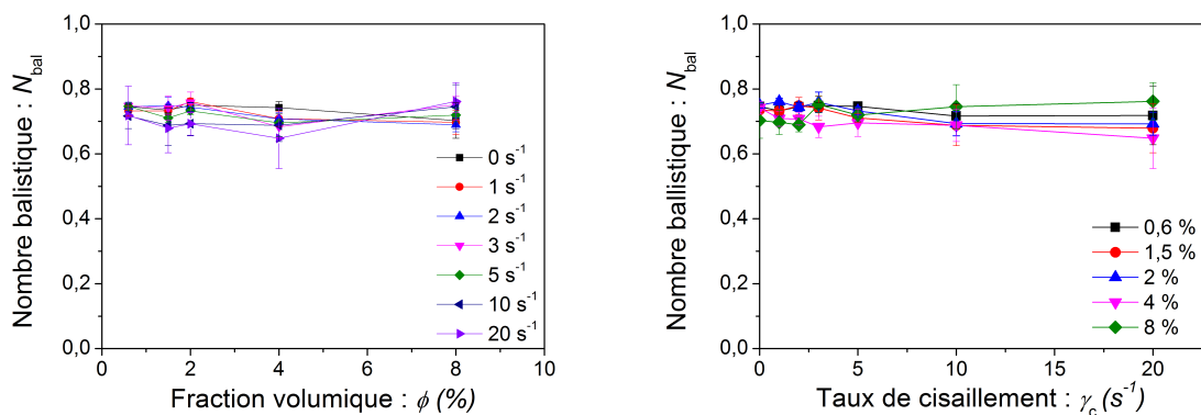
FIGURE 5.11 – N_{\text{bal}} en fonction du taux de cisaillement caractéristique \dot{\gamma}_c imposé et de la fraction volumique \phi en E. Coli.
