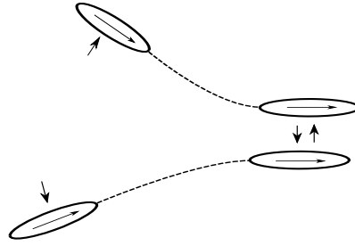
FIGURE 1.13 – Alignement entre deux pushers
