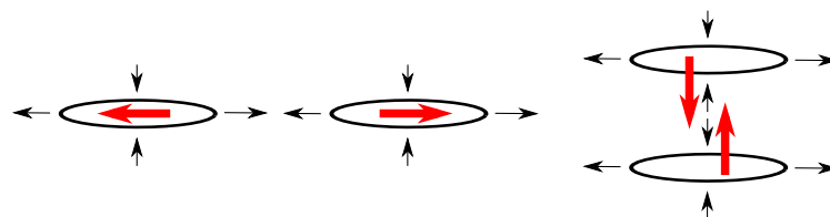
FIGURE 1.12 – Schéma d'interaction entre deux pushers . À gauche : cas d'une répulsion. À droite : cas d'une attraction. Les flèches noires représentent les champs hydrodynamiques produits par les nageurs, les flèches rouge les forces ressenties par les nageurs
