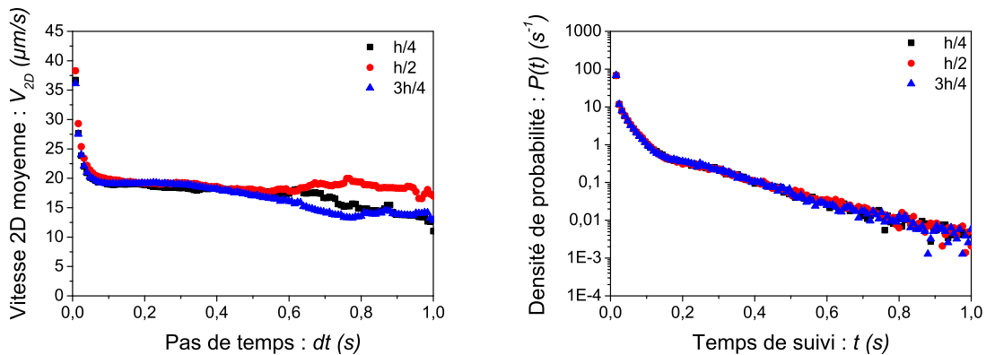
FIGURE 3.5 – À gauche : la vitesse de nage mesurée en fonction du pas de temps et pour différentes positions verticales dans le canal pour plusieurs hauteurs dans le canal. À droite : distribution du temps de suivi pour plusieurs hauteurs dans le canal. Cas d'une suspension de E. Coli concentrée à \phi = 0.5\% alimentée en oxygène et non soumise à un écoulement externe.
