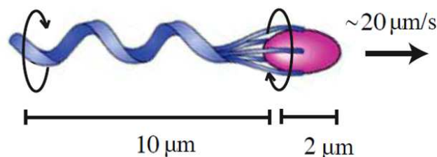
FIGURE 1.1 – Schéma d'une E. Coli
