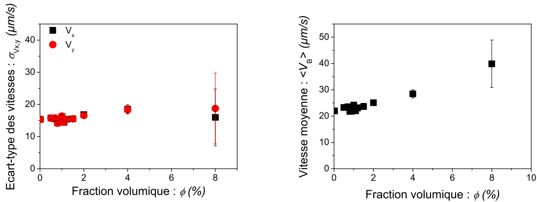
FIGURE 3.13 – À gauche : écart-type de la distribution de vitesse des bactéries selon les axes x et y en fonction de la fraction volumique de la suspension. À droite : vitesse moyenne de nage des bactéries en fonction de la fraction volumique de la suspension.
