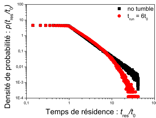
FIGURE 5.5 – Temps de résidence pour des nageurs simulés numériquement sans écoulement et dans le cas dilué. À gauche : Nageurs balistiques. À droite : Nageurs de type run-and-tumble .
