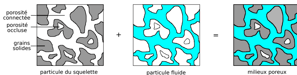
FIGURE 1.1 – Représentation du milieu poreux comme la superposition de deux milieux continus
