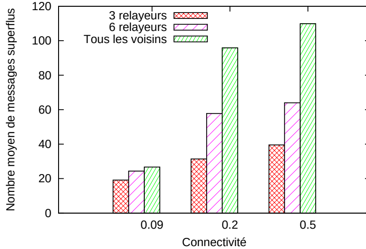
FIGURE 3.9 – Nombre de messages superflus générés lors du processus de dissémination.
