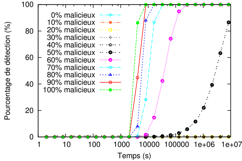
FIGURE 5.26 – Pourcentage de détection pour différents types de véhicules malicieux.
