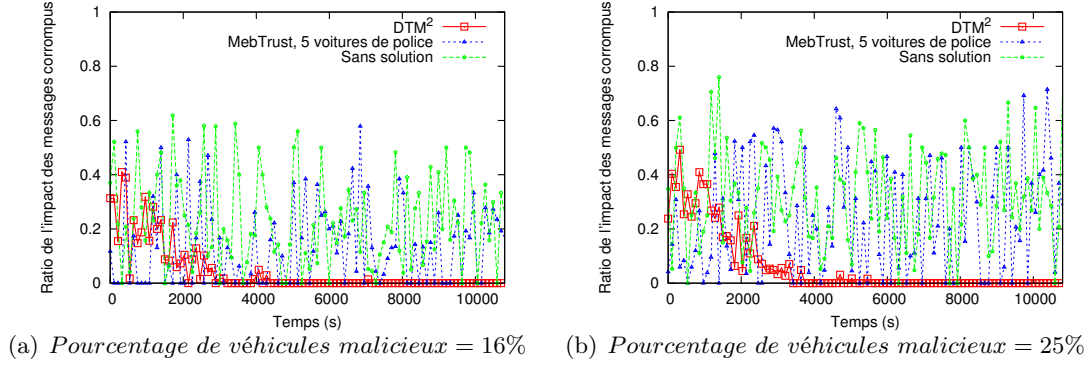
FIGURE 5.20 – Taux moyen de messages corrompus acceptés dans le scénario urbain, avec \lambda = 0.2 .
