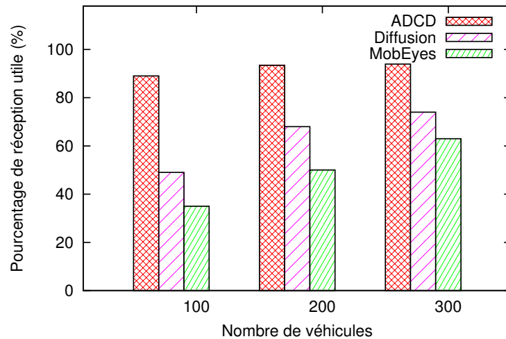
FIGURE 3.15 – Pourcentages de réception, avec 100, 200 et 300 véhicules.
