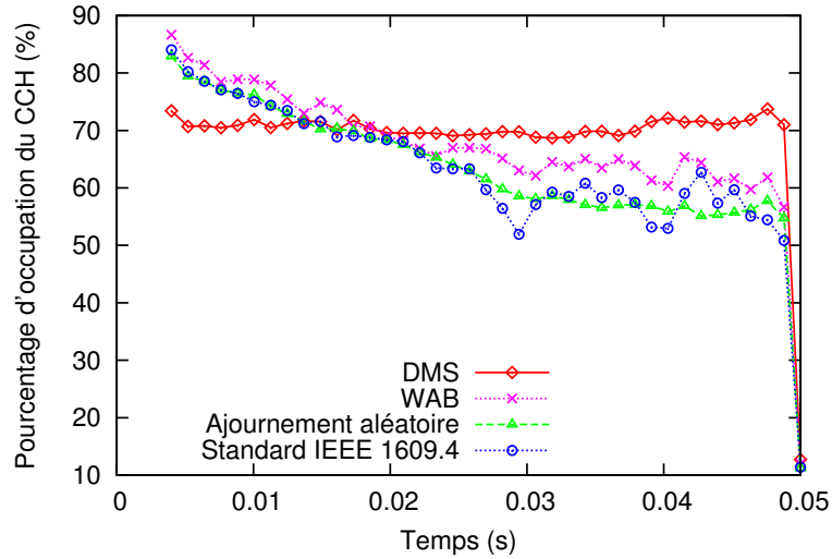
FIGURE 4.4 – Pourcentage moyen d’occupation du canal durant un intervalle CCH avec 100 véhicules mobiles.
