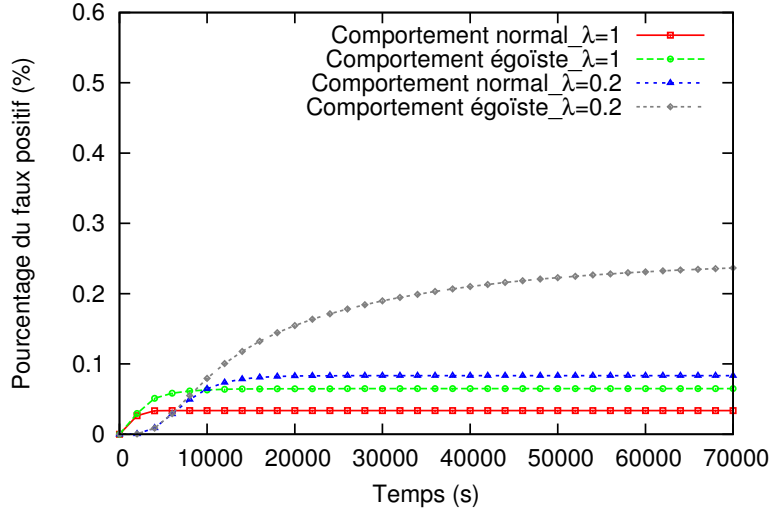
FIGURE 5.17 – Pourcentage analytique de faux positifs.
