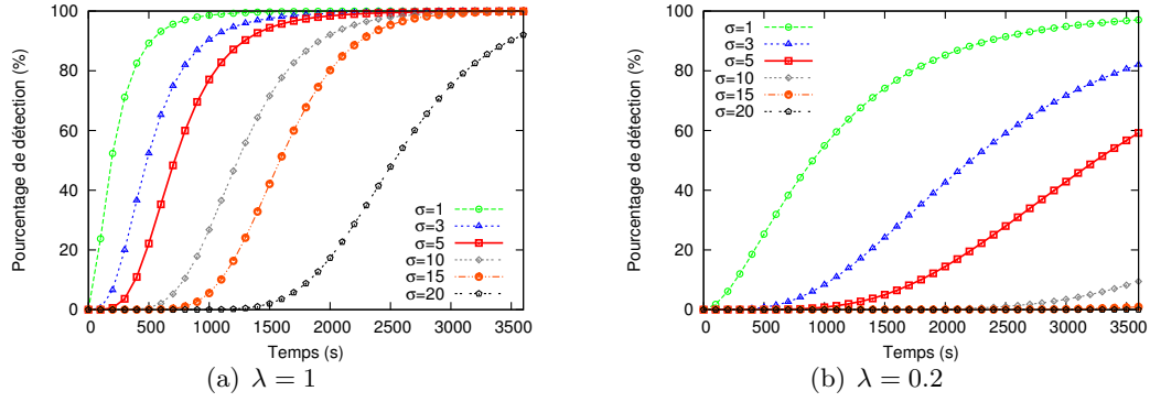
FIGURE 5.13 – Pourcentage de détection des véhicules malicieux par rapport à la variation de \sigma , qui impacte les récompenses données.
