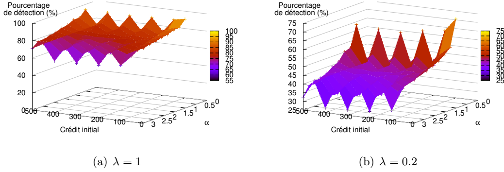
FIGURE 5.11 – Pourcentage de détection des véhicules malicieux par rapport à différentes valeurs de \theta_0 et de \alpha .
