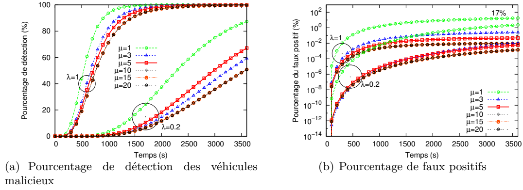
FIGURE 5.15 – Pourcentage de détection par rapport à différentes valeurs de \mu , influant sur le coût de réception d'un message.
