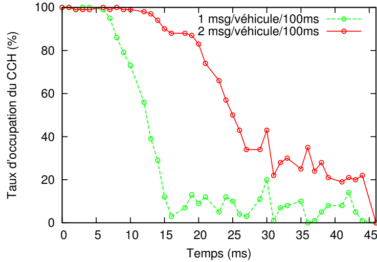
FIGURE 4.1 – Pourcentage d'occupation du canal lors des intervalles de CCH .
