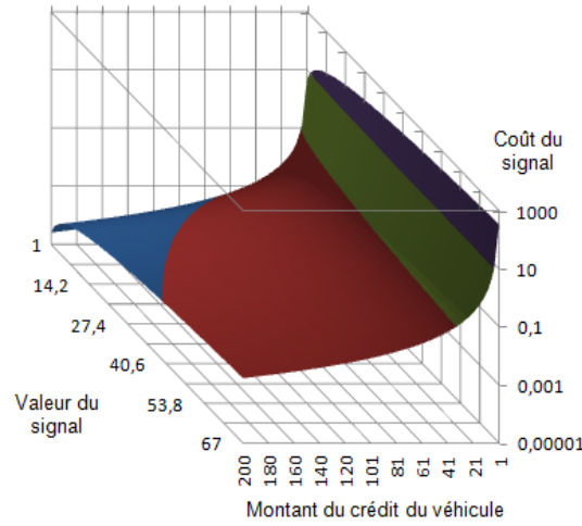
FIGURE 5.6 – Variation du coût d'un signal d'après sa valeur et le montant de crédit détenu par un véhicule.
