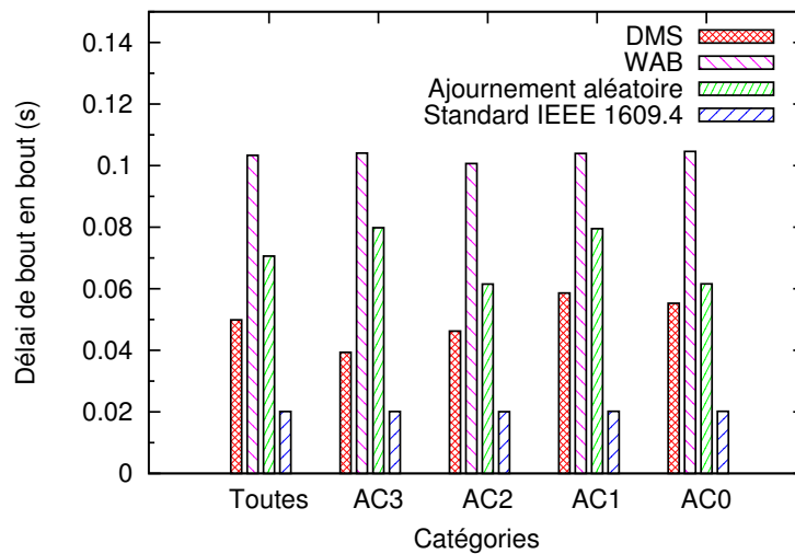
FIGURE 4.10 – Délai moyen de bout en bout pour les différentes catégories d'accès, avec 100 véhicules mobiles.
