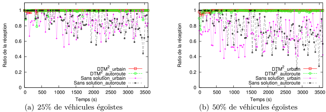
FIGURE 5.23 – Pourcentage moyen de réception dans un réseau comportant des véhicules égoïstes, avec \lambda = 0.2 .
