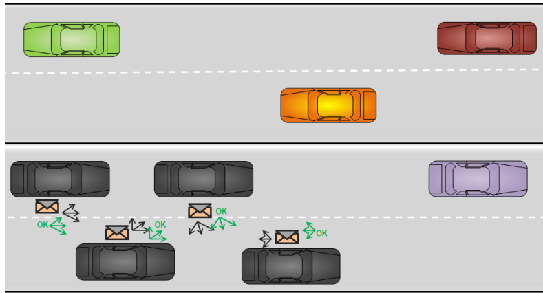
FIGURE 5.24 – Exemple d’une attaque coopérative entre véhicules malicieux. Ces véhicules s’entraident en s’envoyant des notifications positives.
