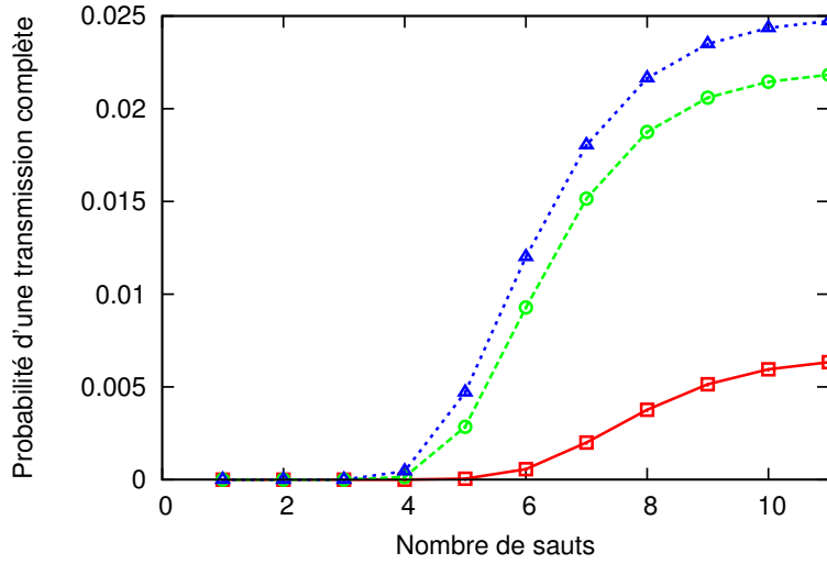
FIGURE 3.6 – Probabilité d'un acheminement complet avec \pi = 0.09 .
