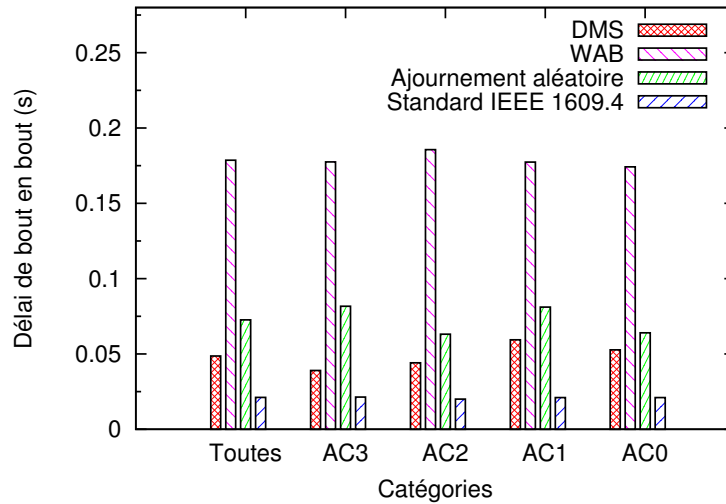
FIGURE 4.9 – Délai moyen de bout en bout pour les différentes catégories d'accès, avec 40 véhicules statiques.
