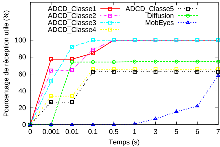
FIGURE 3.13 – Pourcentage de réception en fonction du temps.
