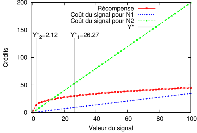
FIGURE 5.7 – Exemple des valeurs des coûts et des récompenses, lors de l'utilisation de différents signaux, pour chacune des sources N1 et N2.
