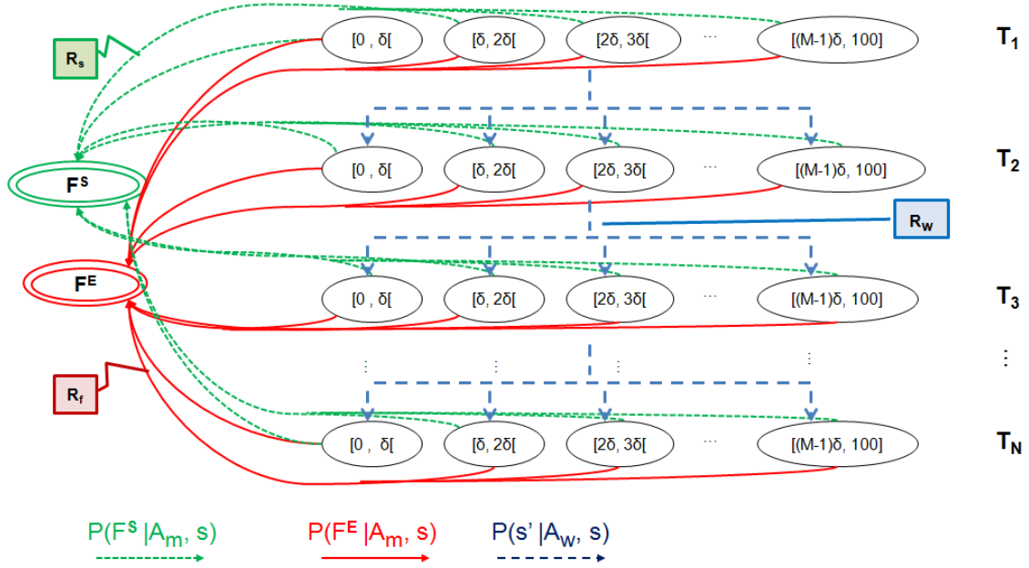
FIGURE 4.2 – Modélisation de la solution DMS en un processus de décision markovien.
