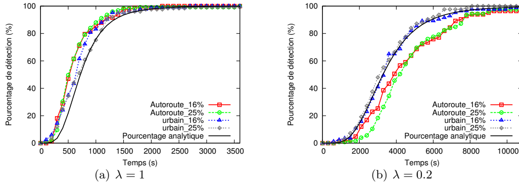
FIGURE 5.16 – Pourcentage de détection des véhicules malicieux.
