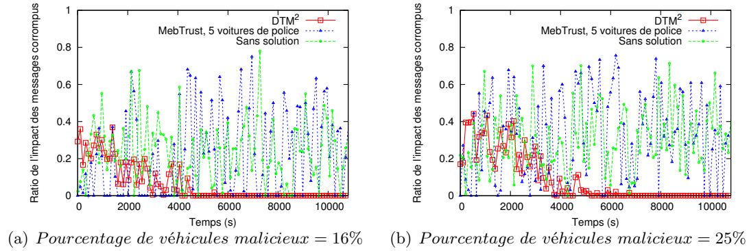
FIGURE 5.21 – Taux moyen de messages corrompus acceptés dans le scénario autoroute, avec \lambda = 0.2 .
