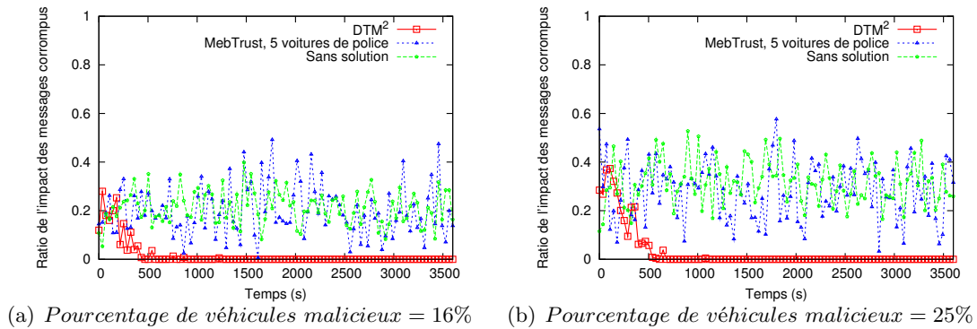
FIGURE 5.19 – Taux moyen de messages corrompus acceptés dans le scénario autoroute, avec \lambda = 1 .
