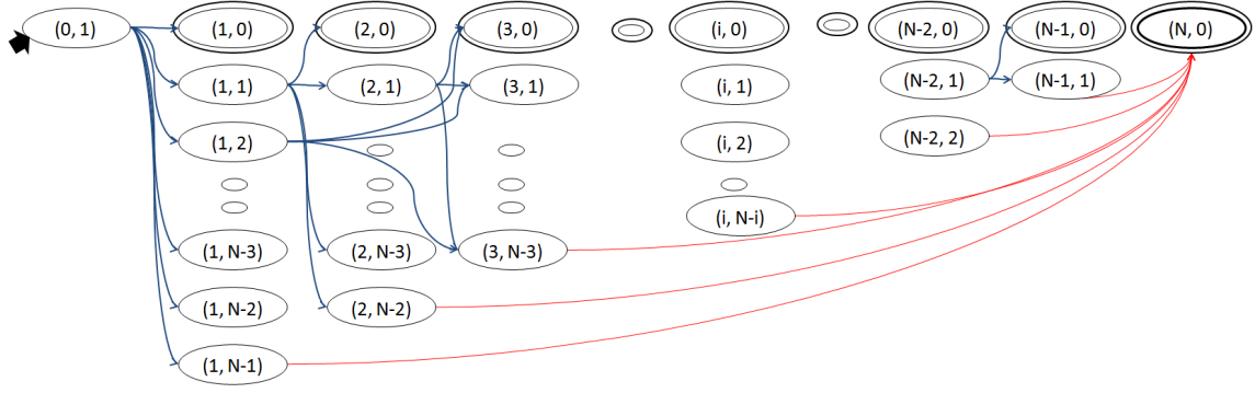
FIGURE 3.4 – Modélisation du processus de dissémination de données d'ADCD, par une chaîne de Markov à temps discret et à espace d'états discret.
