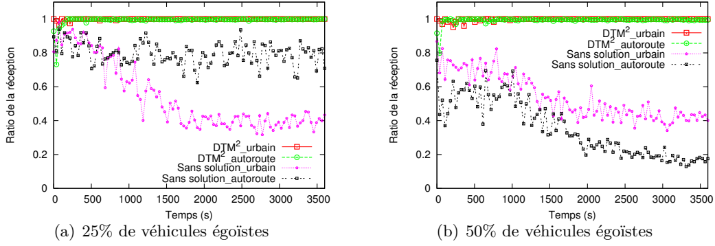
FIGURE 5.22 – Pourcentage moyen de réception dans un réseau comportant des véhicules égoïstes, avec \lambda = 1 .
