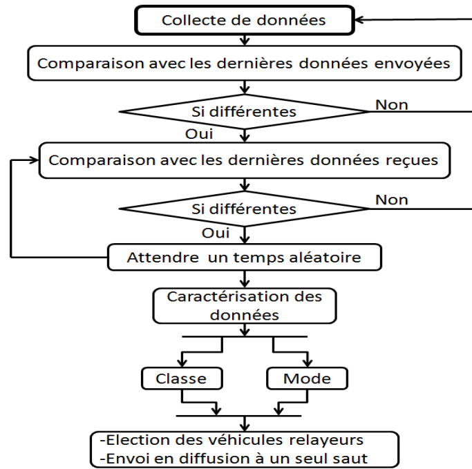
FIGURE 3.1 – Diagramme de flux pour le partage d'une information.
