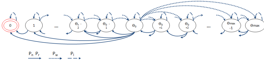
FIGURE 5.9 – Modélisation en chaîne de Markov pour l'optimisation des paramètres de DTM^2 .
