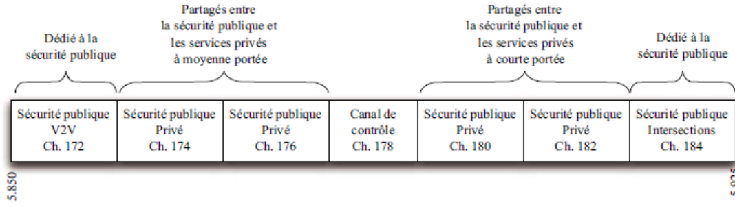
FIGURE 2.5 – Les sept canaux du standard IEEE 802.11p/WAVE [81].
