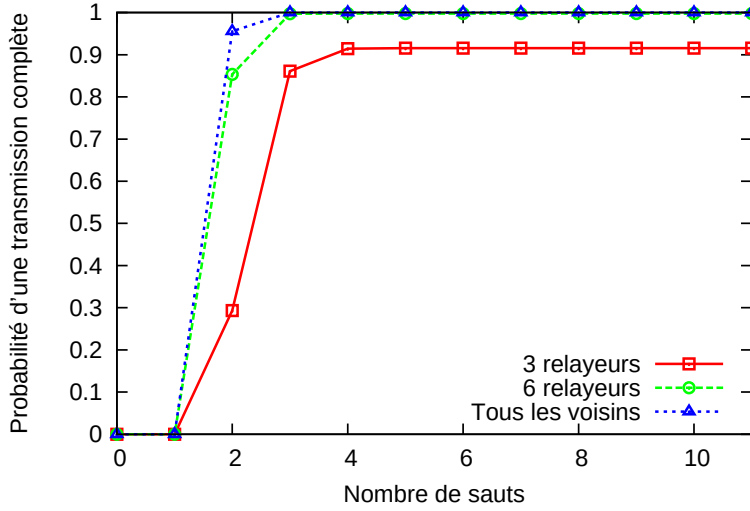
FIGURE 3.8 – Probabilité d'un acheminement complet avec \pi = 0.5 .
