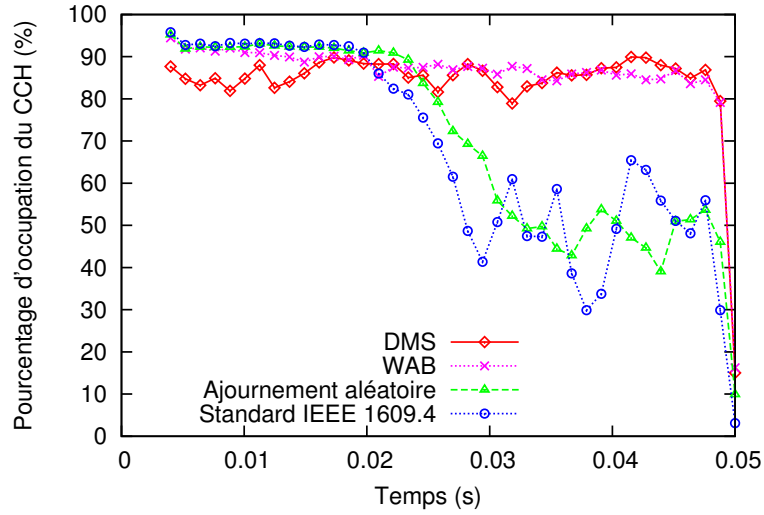
FIGURE 4.3 – Pourcentage moyen d’occupation du canal durant un intervalle CCH avec 40 véhicules statiques.
