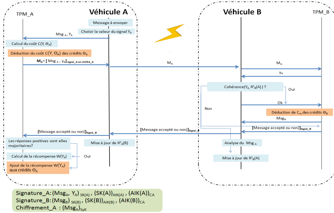
FIGURE 5.5 – Processus d'envoi et de réception d'un message dans DTM^2 .
