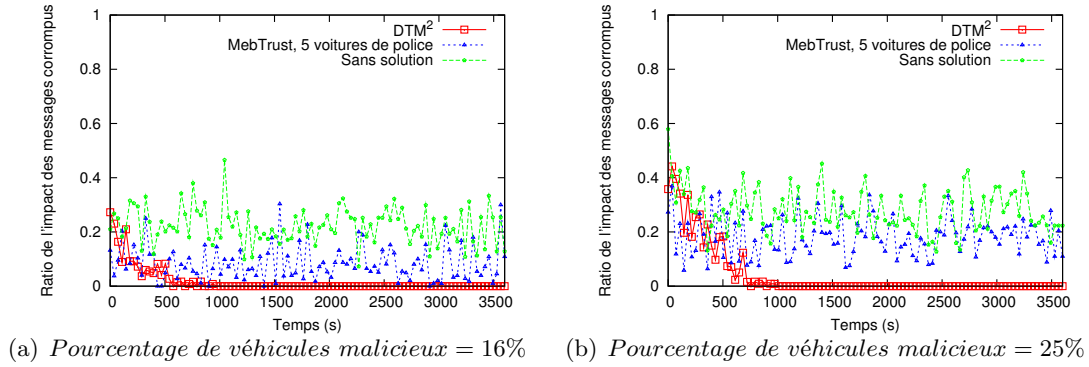
FIGURE 5.18 – Taux moyen de messages corrompus acceptés dans le scénario urbain, avec \lambda = 1 .
