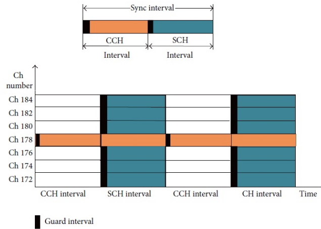
FIGURE 2.6 – Mécanisme du multi-canal [55].
