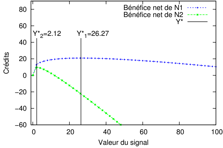
FIGURE 5.8 – Exemple du bénéfice net d'après la valeur de signal utilisée pour chacune des sources N1 et N2.
