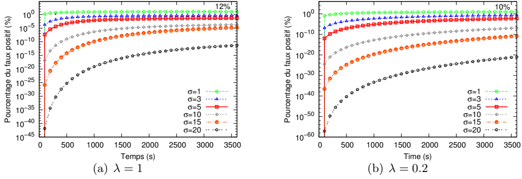
FIGURE 5.14 – Pourcentage de faux positifs par rapport à la variation de \sigma , qui impacte les récompenses données.
