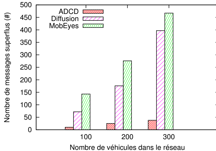
FIGURE 3.16 – Nombre de messages superflus reçus, avec 100, 200 et 300 véhicules.
