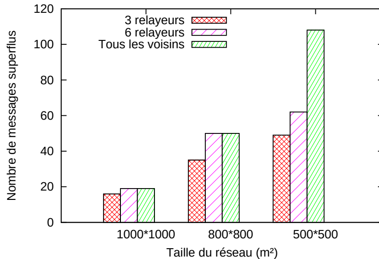
FIGURE 3.11 – Nombre de messages superflus.
