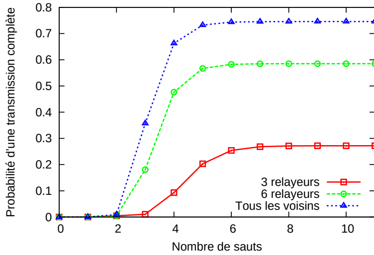
FIGURE 3.7 – Probabilité d'un acheminement complet avec \pi = 0.2 .
