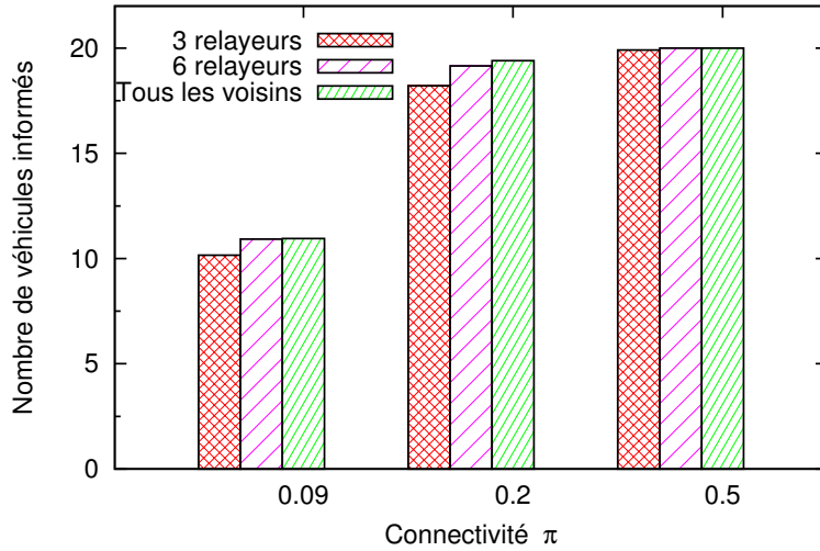
FIGURE 3.5 – Nombre de véhicules concernés par une information et l’ayant reçue, par rapport à différent nombre de relayeurs et à différente connectivité dans le réseau.
