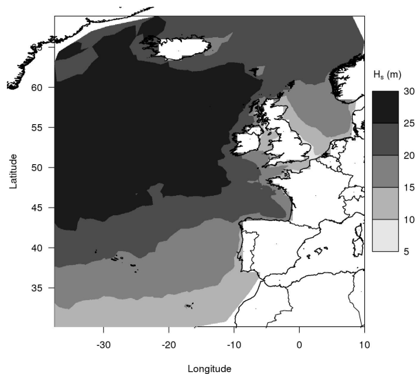
Figure 6.13: Estimation des hauteurs significatives de vagues centennales (m).
