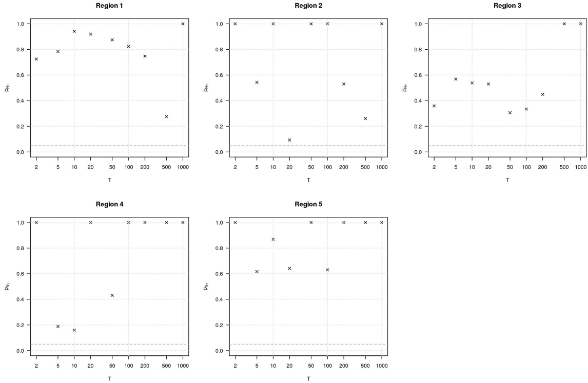
Figure 6.12: Critère N_{r,T} : p -values des 5 lois régionales, pour les périodes de retour T = 2, 5, 10, 20, 50, 100, 200, 500 et 1000 ans (surcotes de pleine mer). La ligne pointillée représente le seuil de décision p_{N_{r,T}} = 0.05 .
