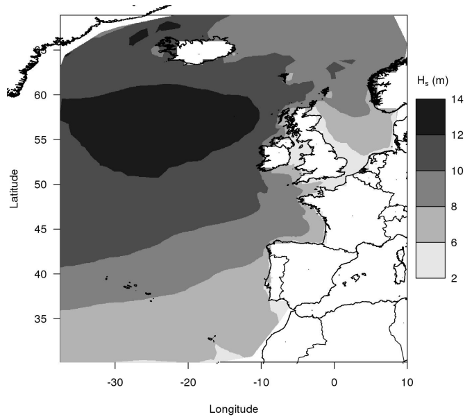
Figure 3.1: Quantiles d'ordre 0.995 des séries temporelles horaires de H_s (m).
