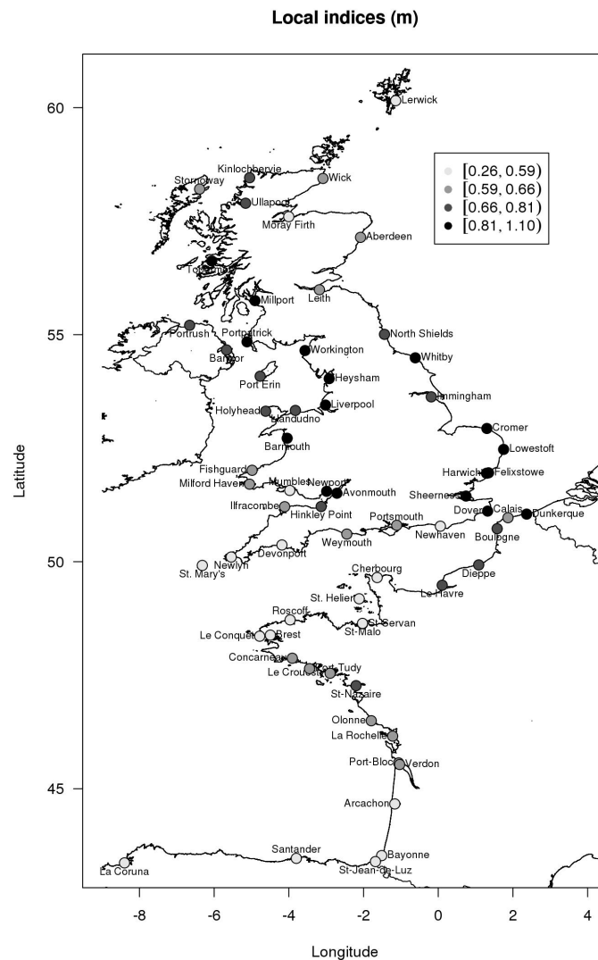
Figure 3.16: Surcotes de pleine mer - indices locaux (seuils dépassés en moyenne \lambda = 1 fois par an) en mètres.
