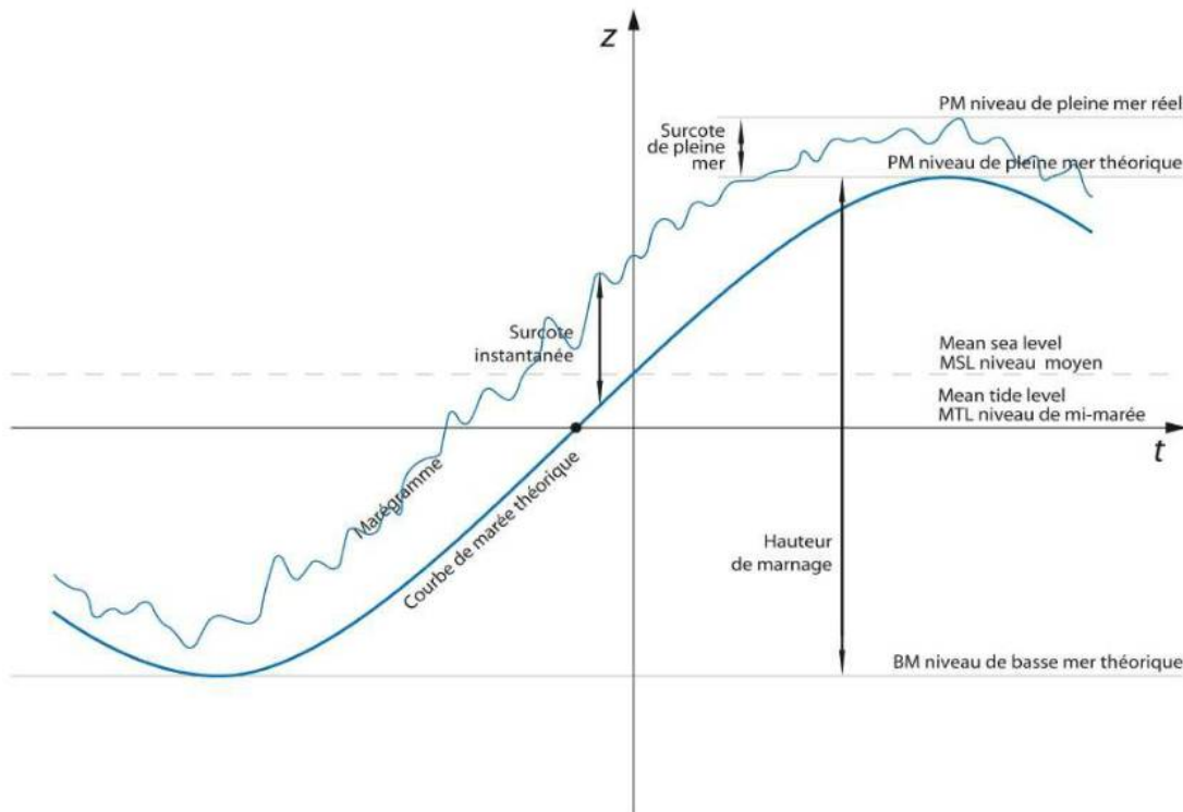
Figure 2.6: Définition de la surcote météorologique (instantanée et de pleine mer). Image issue de [72].
