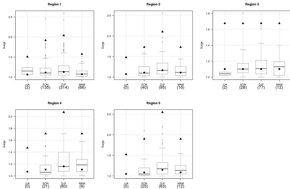
Figure 6.8: Médianes (points) et quantiles d'ordre 0.99 (triangles) estimés pour les 5 lois régionales, selon les 4 saisons d'occurrence des tempêtes (surcotes de pleine mer). Les boxplots des échantillons régionaux sont représentés en gris, et les chiffres entre parenthèses indiquent le nombre de tempêtes observées pour chaque saison.
