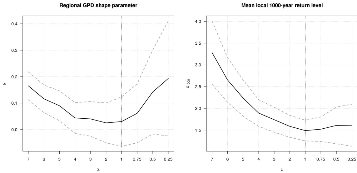
Figure 3.13: Estimation du paramètre de forme de la loi GPD régionale en fonction de \lambda (gauche) et estimation de la surcote de pleine mer millénaire locale moyenne en fonction de \lambda (droite). Les intervalles de confiance à 95% correspondants sont obtenus par la delta-méthode.
