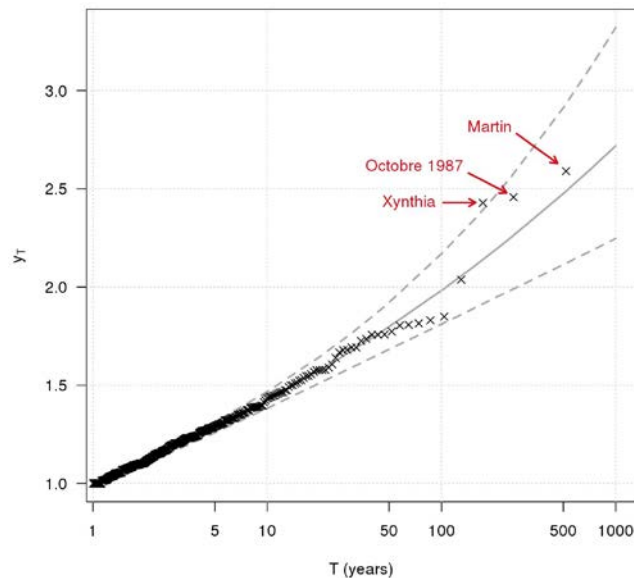
Figure 2. Evolution des niveaux de retour régionaux (normalisés) en fonction de la période de retour pour la région 1, avec intervalles de confiance bootstrap à 95%. Les croix correspondent aux observations de l'échantillon régional.
