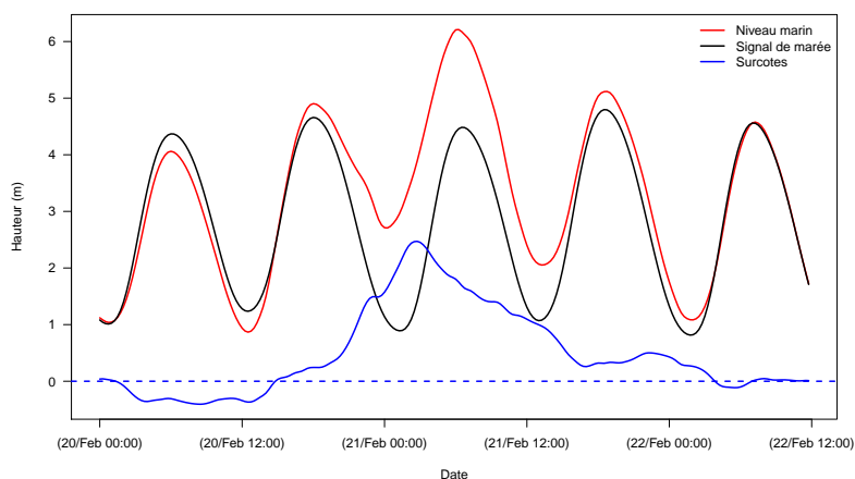
Figure 2.5: Décomposition du niveau marin à Cromer (Angleterre) autour du 21/02/1993.
