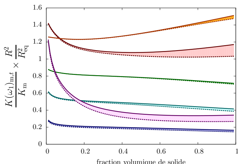
FIG. 3.5: Encadrement de la perméabilité équivalente de la cellule sphéroïdale normalisée par la perméabilité de la cellule sphérique pour les conditions aux limites mixtes. Rapport d'aspect \omega_1 du sphéroïde intérieur : bleu marine 20, bleu clair = 5, vert = 2, orange = 1/2, rouge = 1/5, violet = 1/20).
