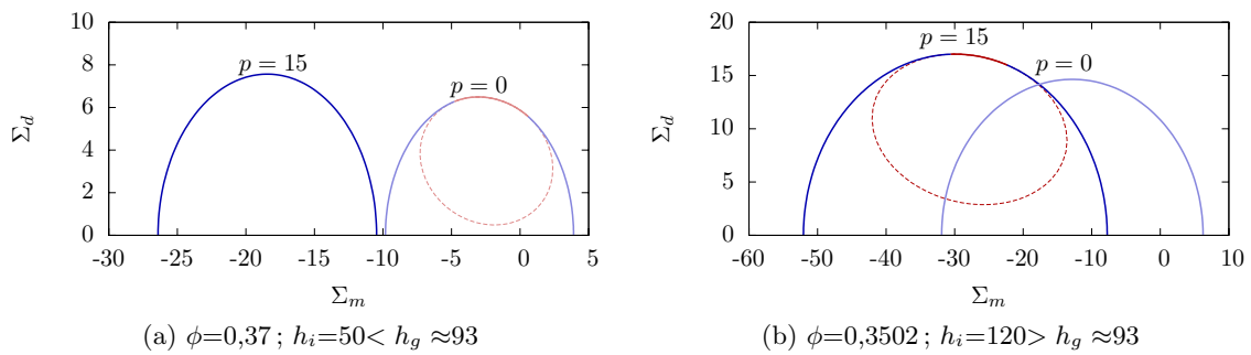
FIG. 6.14: Modification du critère de résistance macroscopique avec interfaces de Mohr-Coulomb en présence d'un fluide sous pression.
