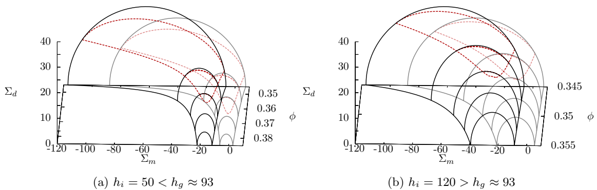
FIG. 6.15: Critère de résistance macroscopique avec interfaces de Mohr-Coulomb, sec (clair) ou avec fluide sous pression (foncé).
