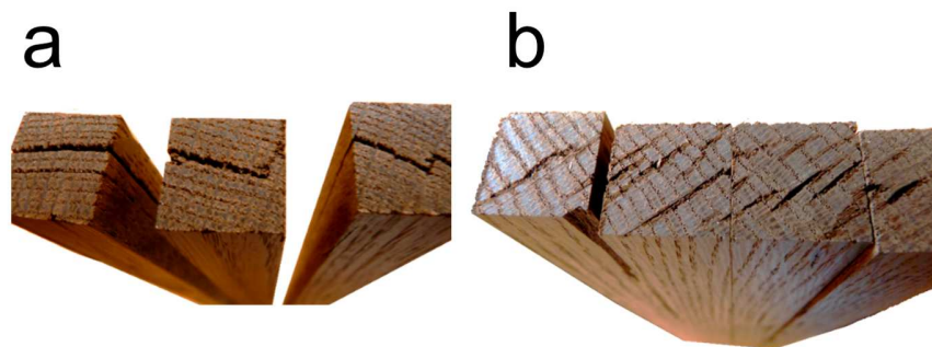
Figure 35 : Observation de gerces sur du chêne traité thermiquement, suivant les cernes annuels (a) et les rayons ligneux (b)
