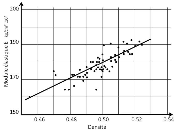
Figure 7 : Évolution du module élastique en fonction de la masse volumique pour l'épicéa [Kollmann and Côté, 1968]
