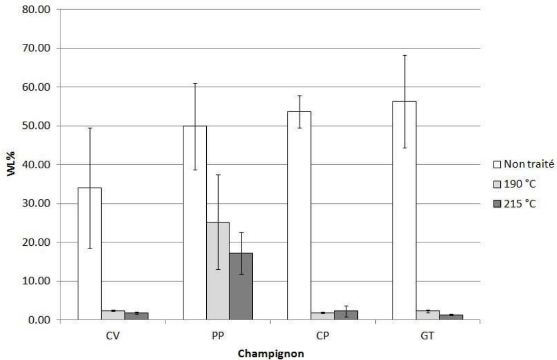
Figure 43 : Dégradation des éprouvettes de hêtre au bout de 12 semaines d'exposition au Coriolus versicolor (CV), Poria placenta (PP), Coniophora puteana (CP) et Gloeophyllum trabeum (GT)
