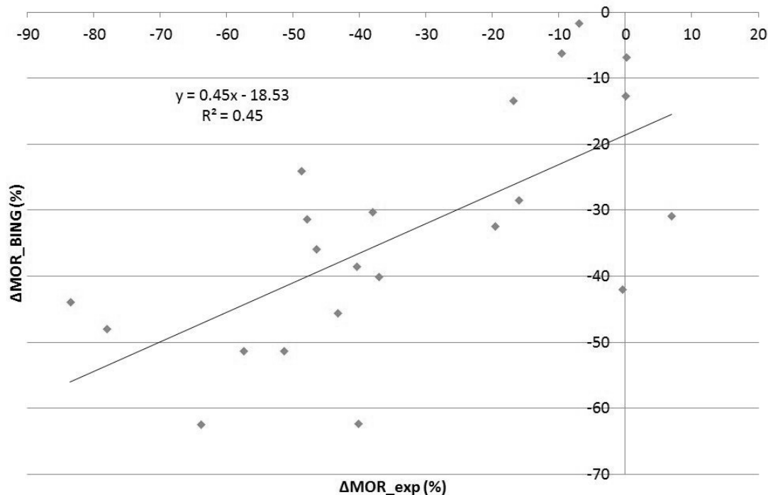
Figure 59 : Corrélation entre la variation de module de rupture estimée par l'analyse vibratoire avec la prise en compte de l'amortissement du signal et la variation de module de rupture obtenu en flexion d'éprouvettes de grandes dimensions de frêne chauffé
