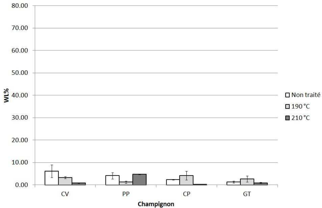
Figure 44 : Dégradation des éprouvettes de chêne sans aubier au bout de 12 semaines d'exposition au Coriolus versicolor (CV), Poria placenta (PP), Coniophora puteana (CP) et Gloeophyllum trabeum (GT)
