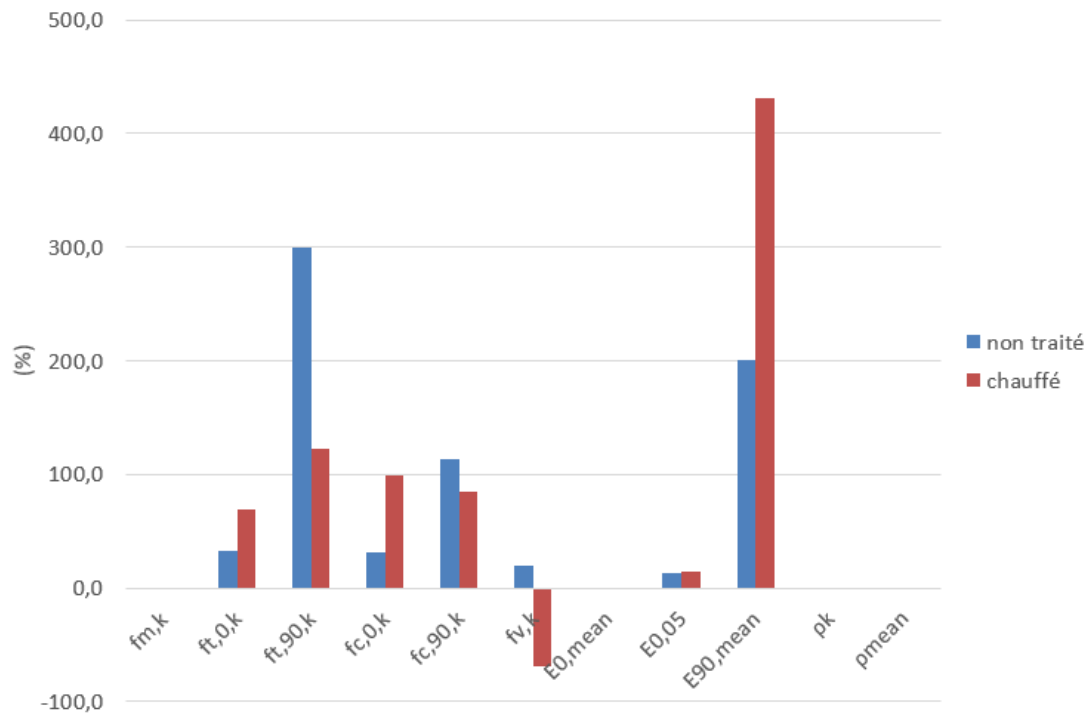
Figure 36 : Écarts entre les valeurs d'essais et les valeurs sécuritaires calculées par les relations données par la norme EN 338
