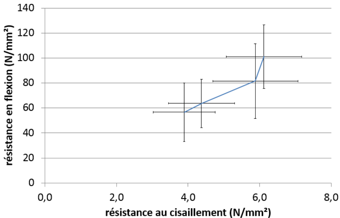
Figure 42 : Évolution de la résistance en flexion en fonction de la résistance au cisaillement pour le frêne chauffé à 170, 200, 215 et 228 °C
