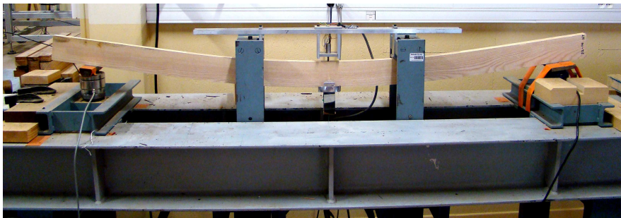
Figure 21 : Planche de frêne non traitée soumise à un essai de flexion sur chant
