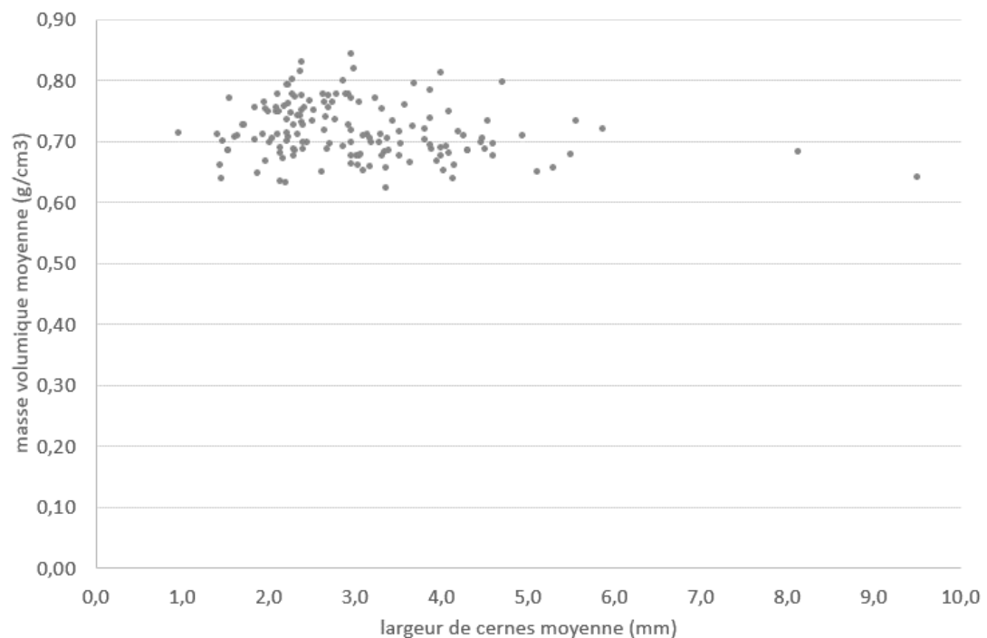
Figure 75 : masse volumique moyenne en fonction de la largeur de cernes moyenne pour des planches de frêne non traité
