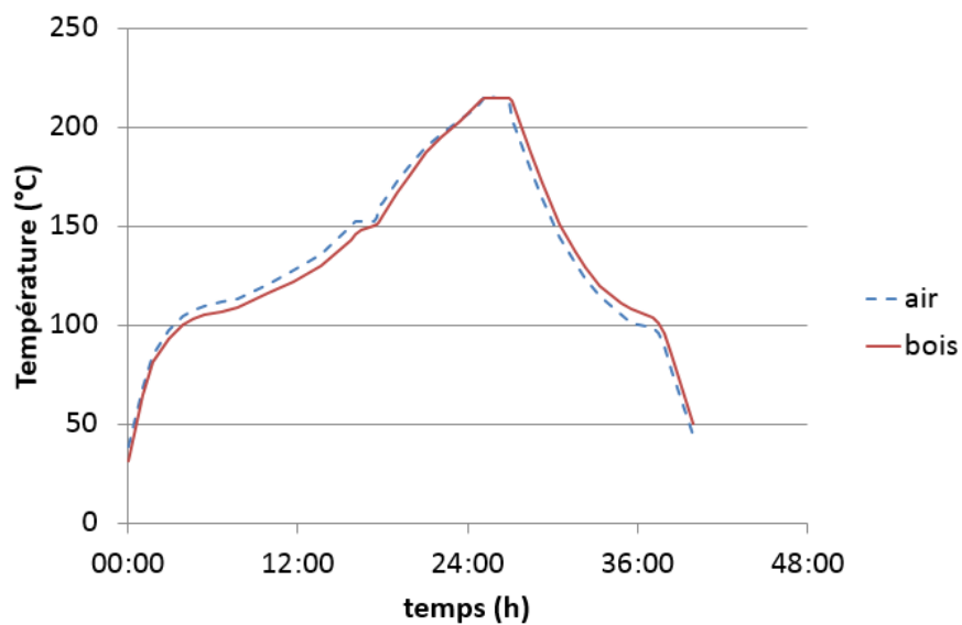
Figure 16 : Évolution de la température dans le bois de frêne au cours d'un cycle de traitement thermique à 215 °C
