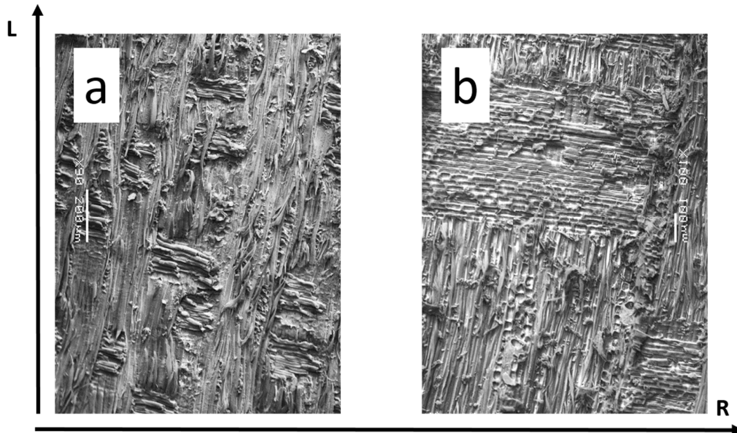
Figure 34 : Grossissement d'un plan de cisaillement au microscope électronique à balayage avec du frêne non traité (a) et du frêne chauffé à 215 °C
