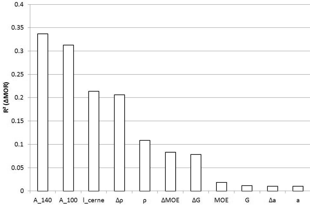
Figure 68 : Coefficients de détermination entre les indicateurs non destructifs et la variation de module de rupture en flexion
