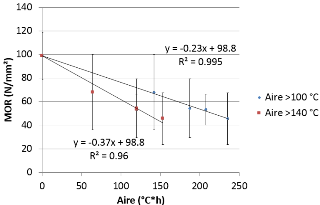
Figure 64 : Corrélation entre la résistance en flexion MOR et l'aire sous la courbe du traitement thermique de planches de frêne
