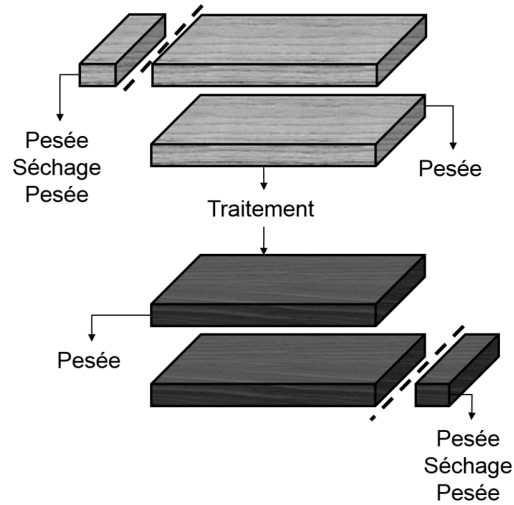
Figure 28 : Protocole pour la mesure de la perte de masse due au traitement thermique de planches de grandes dimensions
