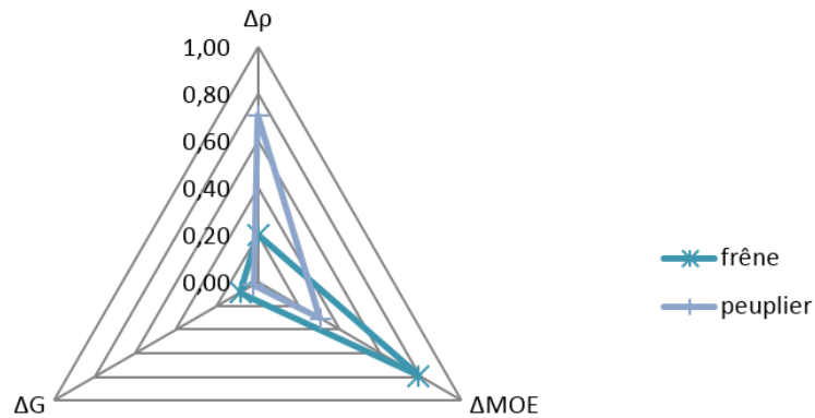
Figure 54 : Coefficients de détermination entre les variations de masses volumiques, de modules élastiques, de modules de cisaillement et les variations de résistances en flexion d'éprouvettes sans défaut de frêne et de peuplier
