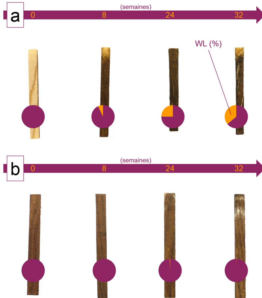
Figure 45 : Dégradation des éprouvettes de frêne en contact avec le sol après 8, 24, et 32 semaines d'exposition pour le frêne non traité (a) et le frêne chauffé à 215 °C (b)
