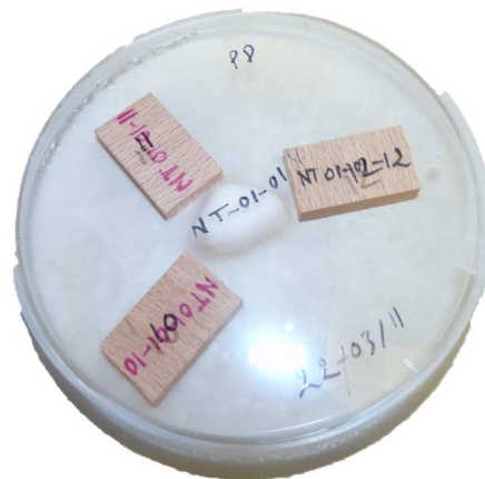
Figure 26 : Éprouvettes de hêtre mises en contact avec une souche de Poria placenta pour un essai en classe d'emploi 3 au LERMAB
