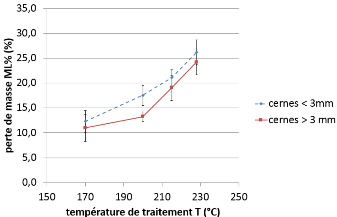
Figure 74 : Pertes de masses en fonction de la température de traitement du frêne mesurées pour des largeurs de cernes moyennes inférieures ou supérieures à
