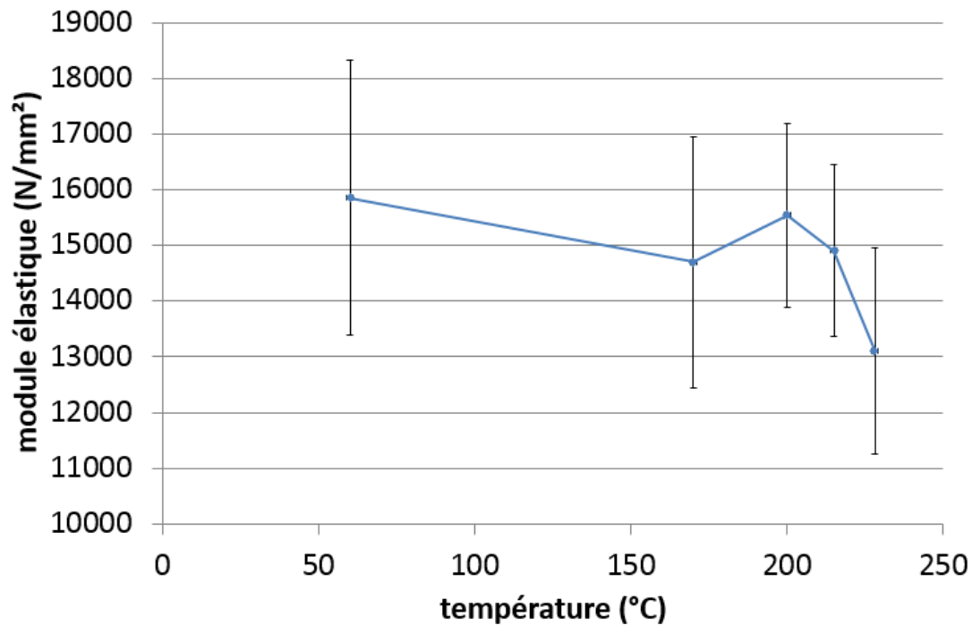
Figure 38 : Évolution du module élastique axial en fonction de la température de traitement sur des éprouvettes de frêne de grandes dimensions
