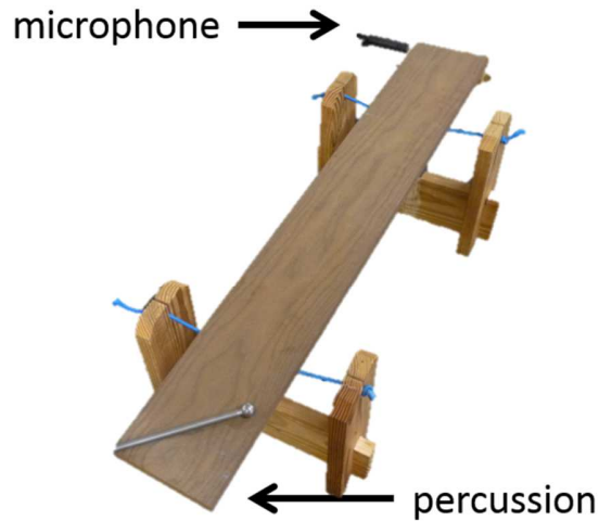
Figure 30 : Principe du dispositif BING : enregistrement des vibrations de l'éprouvette suite à une percussion. Le signal est capté par une carte d'acquisition, filtré et numérisé, puis traité par un ordinateur
