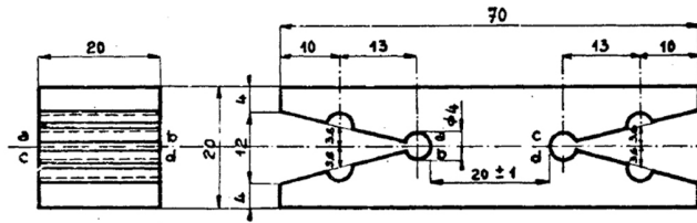
Figure 23 : Éprouvette d'un essai de traction transversale
