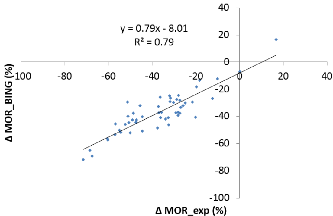
Figure 51 : Corrélation entre la variation de module de rupture estimée par l'analyse vibratoire et la variation de module de rupture obtenu en flexion destructive de petites éprouvettes sans défaut de bois chauffés (chêne, douglas, frêne, hêtre et peuplier)
