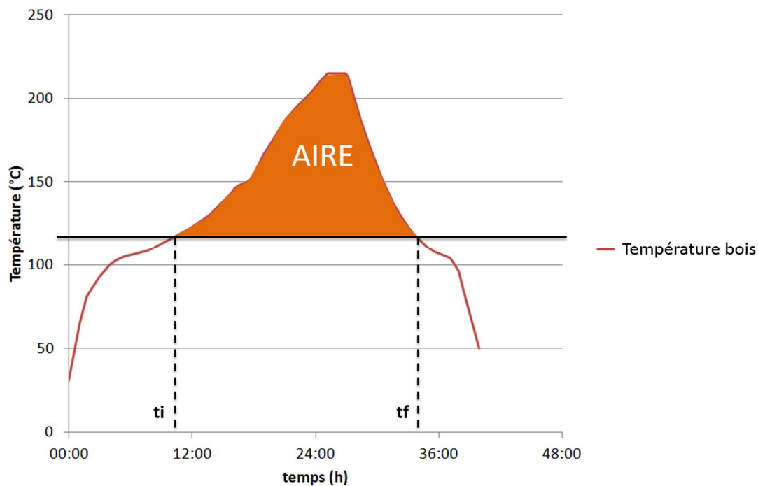
Figure 63 : Illustration de la surface utilisée comme indicateur
