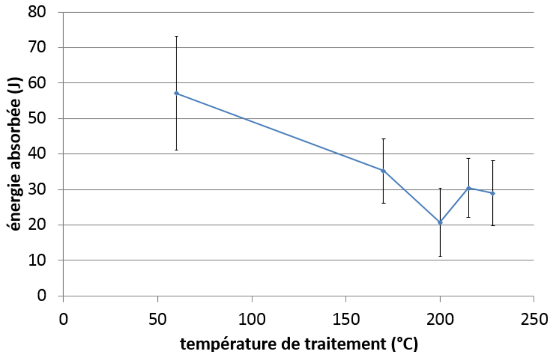
Figure 37 : Évolution de l'énergie absorbée en flexion dynamique en fonction de la température de traitement
