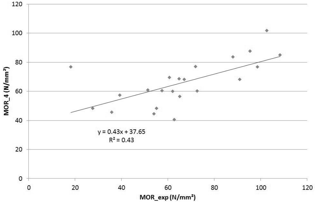
Figure 72 : Relation entre la contrainte à la rupture mesurer de manière destructive MOR_{exp} et la contrainte à la rupture estimée de manière non destructive avec 4 indicateurs MOR_4
