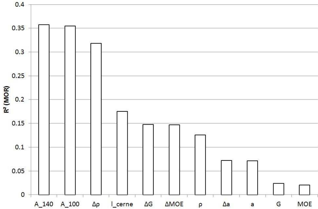
Figure 71 : Coefficients de détermination entre les indicateurs non destructifs et le module de rupture en flexion
