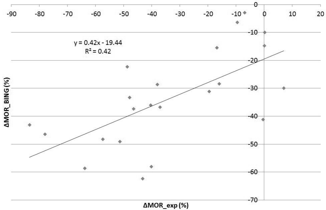
Figure 58 : Corrélation entre la variation de module de rupture estimée par l'analyse vibratoire et la variation de module de rupture obtenu en flexion d'éprouvettes de grandes dimensions de frêne chauffé
