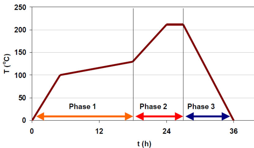
Figure 13 : Cycle type tel qu'il est proposé dans le manuel Thermowood [Finnish Thermowood Association]
