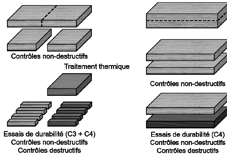
Figure 14 : Protocole utilisé pour comparer des lots de bois traités et non traités ; à gauche : campagnes sur de petites éprouvettes sans défaut ; à droite : campagnes sur des planches de grandes dimensions
