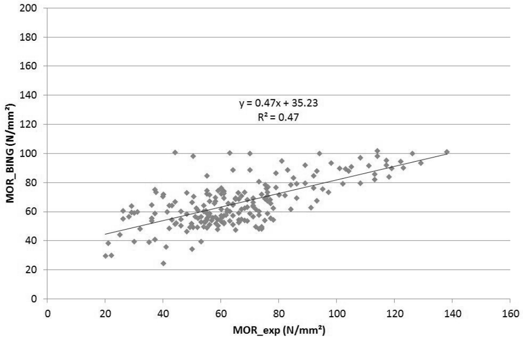
Figure 50 : Corrélation entre le module de rupture estimé par l'analyse vibratoire et le module de rupture réel obtenu en flexion de petites éprouvettes sans défaut de bois chauffés à 190 et 215 °C (chêne, douglas, frêne, hêtre et peuplier)
