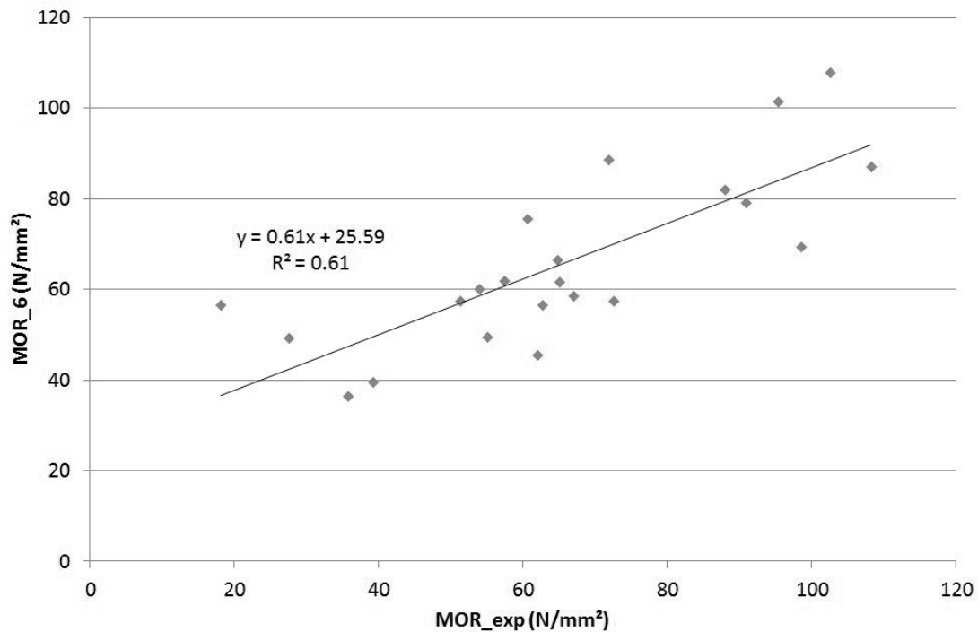
Figure 73 : Relation entre la contrainte à la rupture mesurer de manière destructive MOR_{exp} et la contrainte à la rupture estimée de manière non destructive avec 6 indicateurs MOR_6
