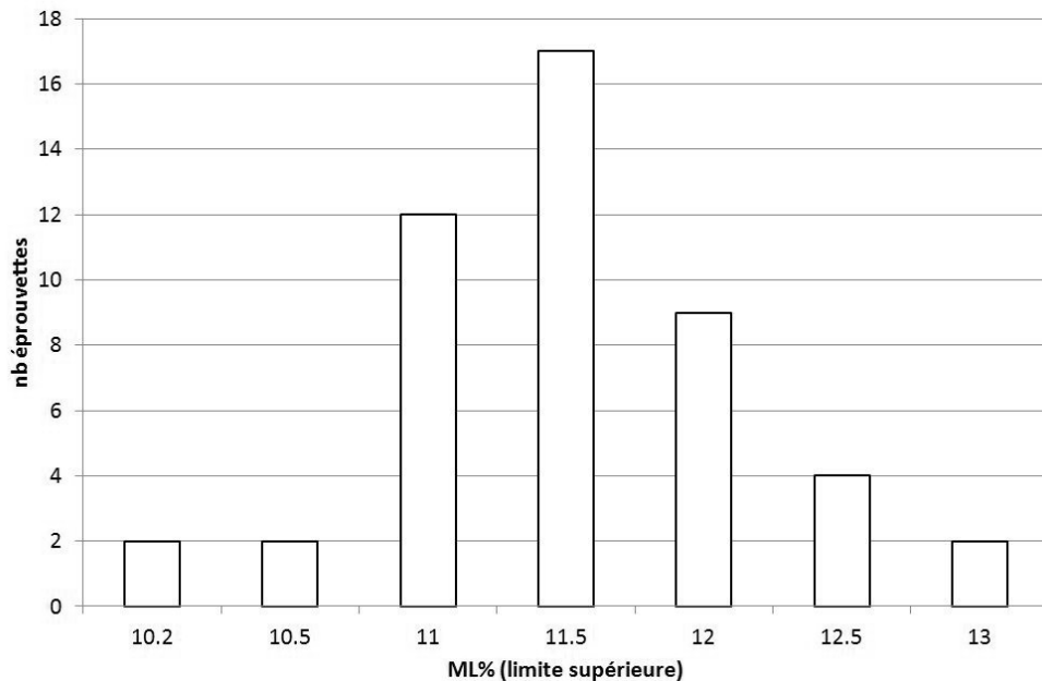
Figure 66 : Distribution des pertes de masse de 48 éprouvettes réparties aléatoirement dans un four de traitement thermique
