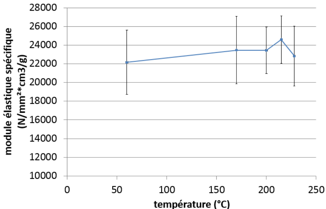
Figure 40 : Évolution du module élastique spécifique axial du frêne en fonction de sa température de traitement
