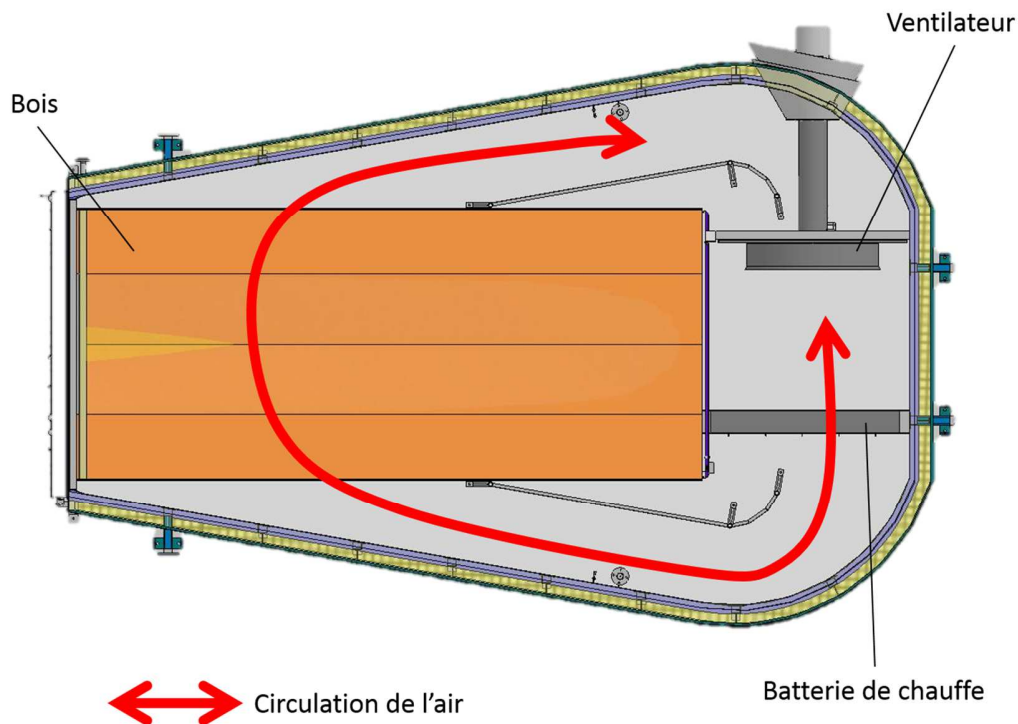
Figure 12 : Schéma d'un four Thermowood tel qu'il a été construit chez Bois Durables de Bourgogne
