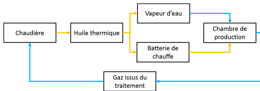
Figure 11 : Schéma illustrant les flux de chaleur (en orange) et de matières (en bleu) dus au traitement du bois avec le procédé Thermowood
