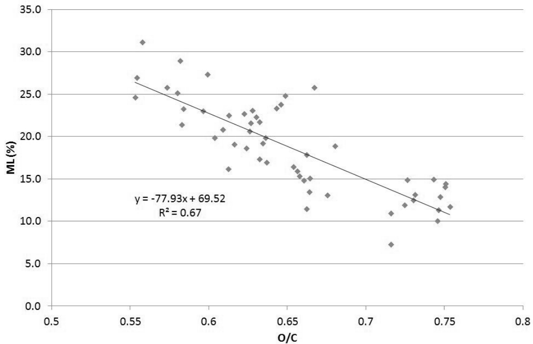
Figure 62 : Corrélation entre la perte de masse et le rapport O/C de planches de frêne chauffées
