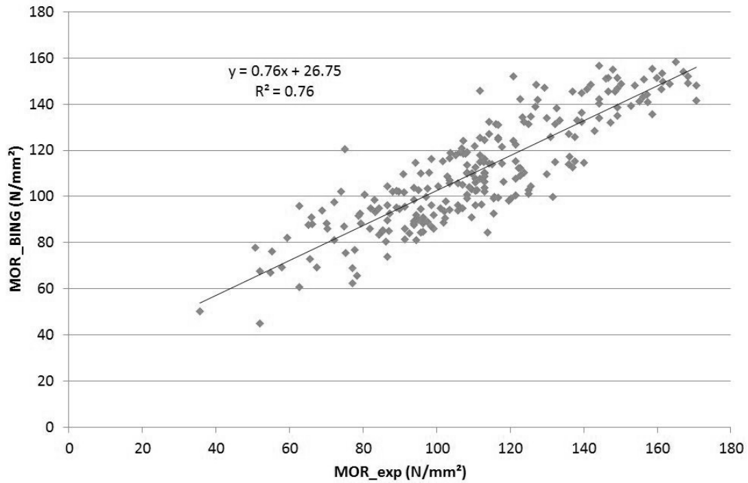
Figure 49 : Corrélation entre le module de rupture estimé par l'analyse vibratoire et le module de rupture réel obtenu en flexion destructive de petites éprouvettes sans défaut de bois non traités (chêne, douglas, frêne, hêtre et peuplier)
