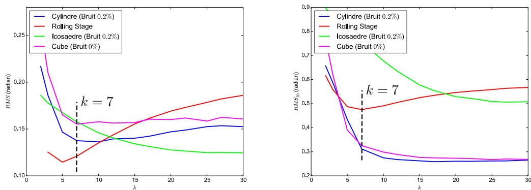
FIGURE 5.19 – Précision pour différents modèles en fonction de k , à autres paramètres fixés.
