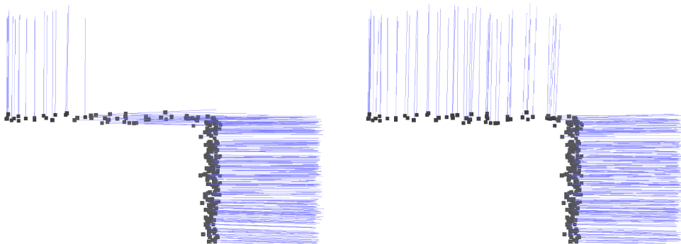
FIGURE 5.11 – Effet de l'anisotropie sur l'estimation de normales. À gauche, Li et al. [2010] et à droite, notre méthode avec tirage quasi uniforme.
