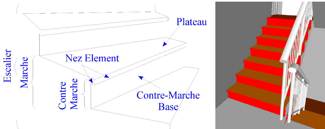
FIGURE 9.6 – Les éléments de la grammaire d'escalier (à gauche) et un exemple de reconnaissance automatique sur un modèle CAO (à droite).
