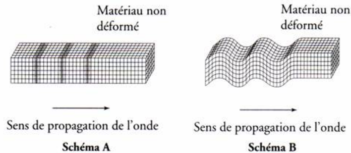
FIGURE I.10. Onde de compression (schéma A) et onde de cisaillement (schéma B). www.wikipedia.com
