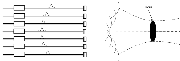
(b) Focalisation du front d'ondes.
