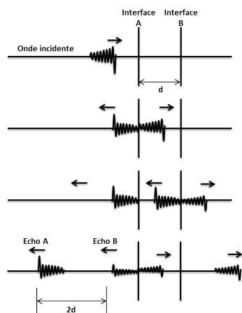
(a) Émission et réception d'un train d'ondes, à l'interface entre deux milieux une partie de l'onde traverse et l'autre est réfléchiée.
