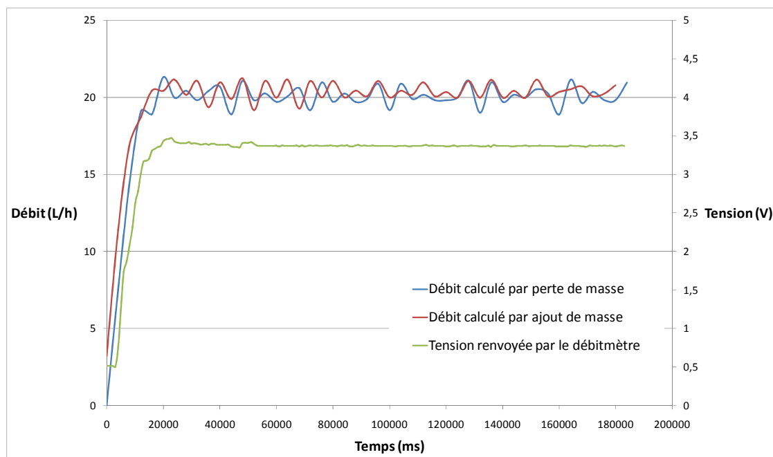
Figure 2-12 : Tension renvoyée par le débitmètre en Ryton pour des débits calculés par perte et ajout de masse de 20L/h.
