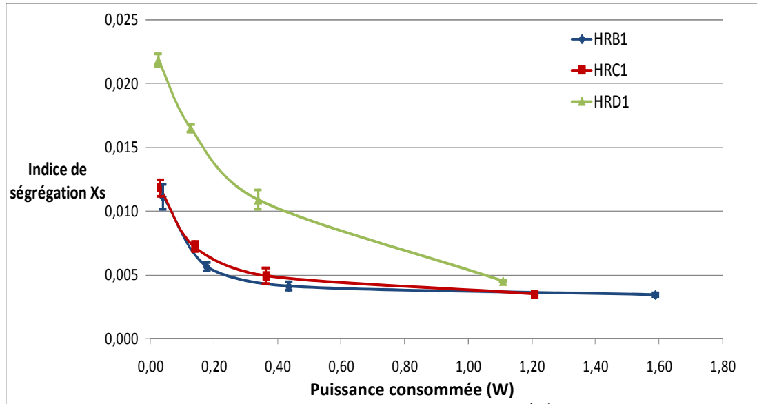
Figure 3-5: Evolution de X_s en fonction de la puissance consommée dans l'installation pour les trois géométries de mélangeur étudiées (jeu de concentrations n°2).
