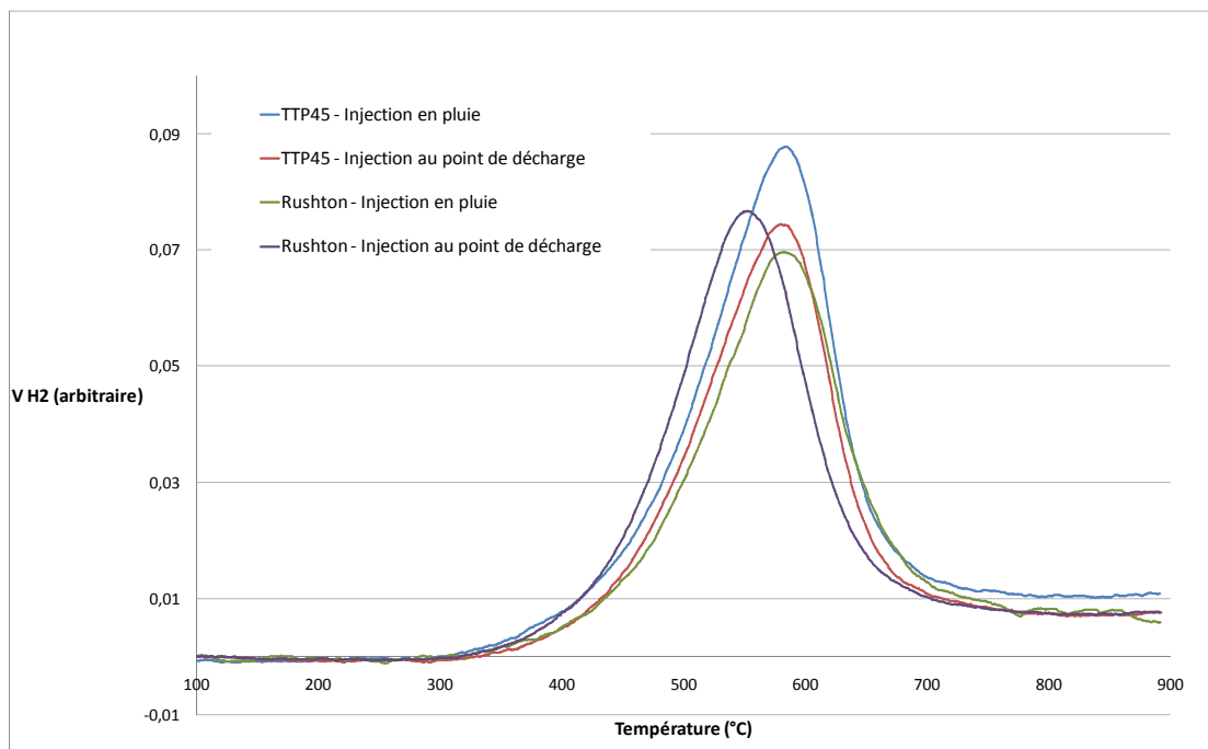
Figure 4-2 : Evolution de la consommation de H 2 en fonction de la température pour des particules d'oxydes mixtes Ce 0,25 Zr 0,70 La 0,02 Y 0,03 synthétisées en réacteur semi-fermé agité pour différentes conditions de mélange et calcinées à 1100°C.
