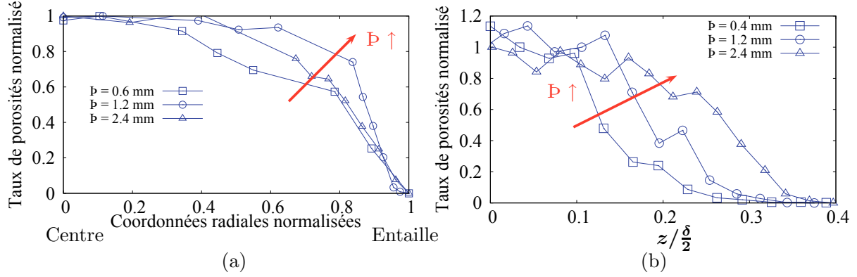
FIG. 5.4: (a) Taux de porosité normalisés des différentes éprouvettes NT4 en fonction des coordonnées radiales normalisées. (b) Taux de porosité normalisés dans la direction axiale z pour les éprouvettes NT4. On se réfère aux différentes éprouvettes NT4 par leurs déplacement résiduel \bar{P} .
