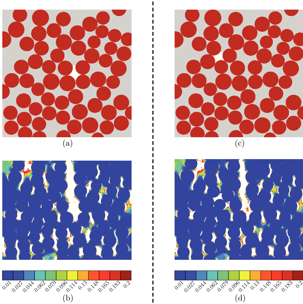
FIG. 6.23: (a) et (c) VER 1 avec un taux de macro-pores de 0.4%. Le pore est disposé à des enplacements différents. (b) et (d) Cartes d'isovaleurs du calcul du taux de porosité dans la matrice pour chacun des VER déformés avec propagation de fissures pour les cas (a) et (c) respectivement ( \epsilon_{macr} = 0.07 ).
