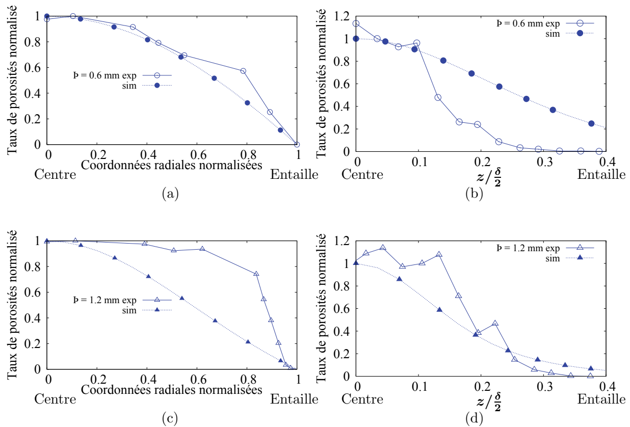
FIG. 5.14: (a) et (c) Taux de porosité normalisé en fonction des coordonnées radiales normalisées pour P 0.6 mm et 1.2 mm respectivement. (b) et (d) Taux de porosité normalisé en fonction des coordonnées axiales normalisées pour P 0.6 mm et 1.2 mm respectivement. Les marqueurs vides représentent les données expérimentales, les marqueurs pleins sont les données numériques.
