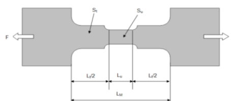
Figure 2.14. Forme de l'éprouvette
