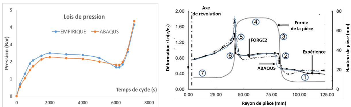
Figure 5.6. Comparaison des résultats numériques et expérimentaux
