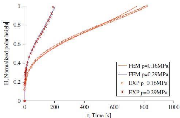
Figure 2.9. Prédications du modèle de Norton-Hoff pour un alliage de Magnésium AZ31 [85]
