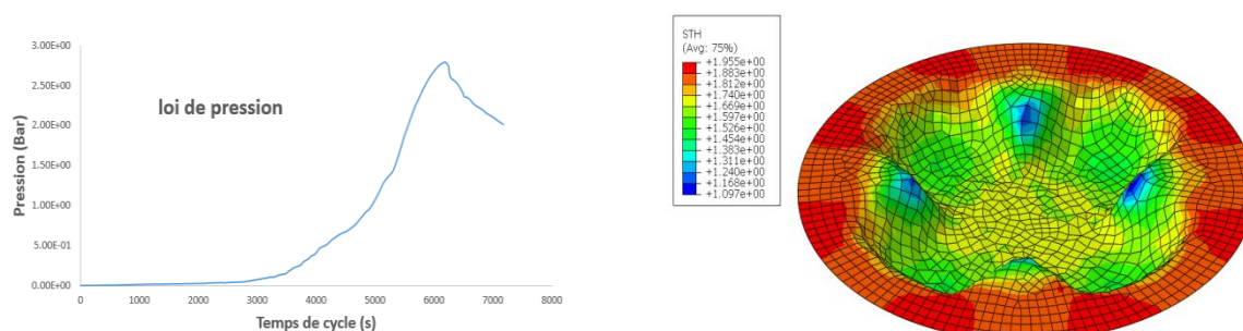
(a) Loi de pression (b) Évolution de l'épaisseur en fin de remplissage Figure 5.14. Gonflage d'une pièce complexe sous ABAQUS/Explicit
