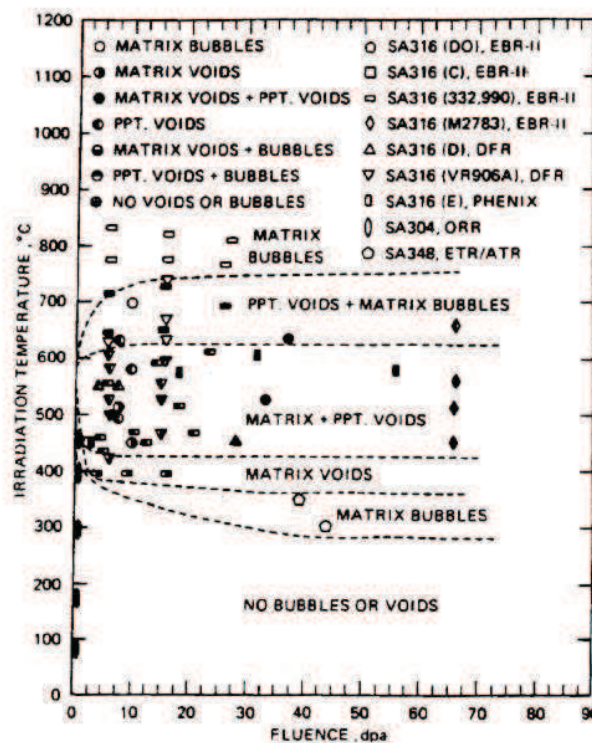
Figure I.10: Formation des cavités en fonction de la dose et de la température [Maziasz 1993, Zinkle 1993]- la distinction bulles/cavités a été effectuée selon un critère de taille et de forme, à la vue des récents résultats de Zouari [Zouari 2012], le terme bulle serait à remplacer par cavité.
