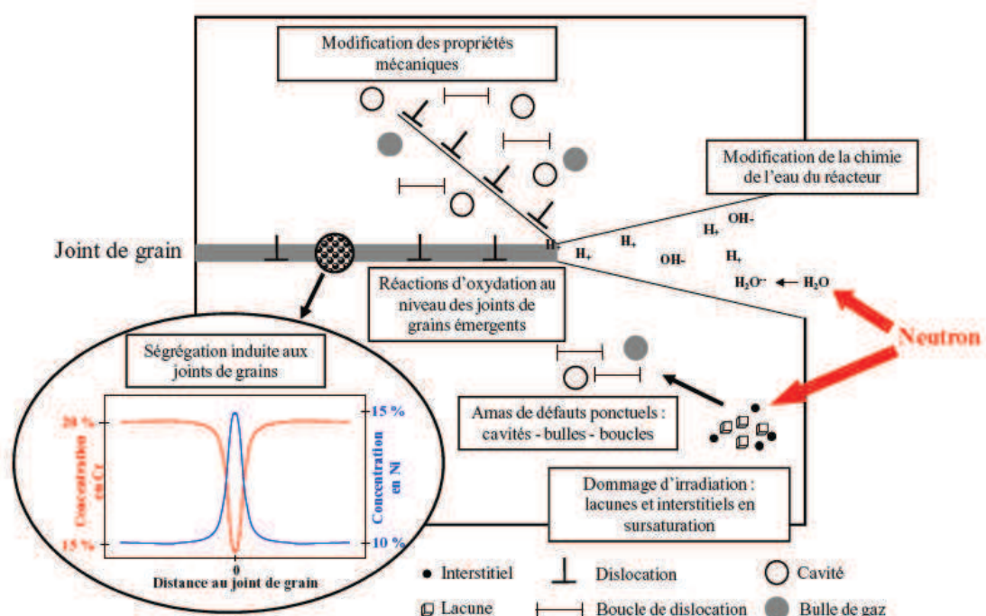
Figure I.30 : Processus susceptibles d'agir dans le cadre de la fissuration par IASCC d'après [Bruemmer 1999 et Etienne 2009]
