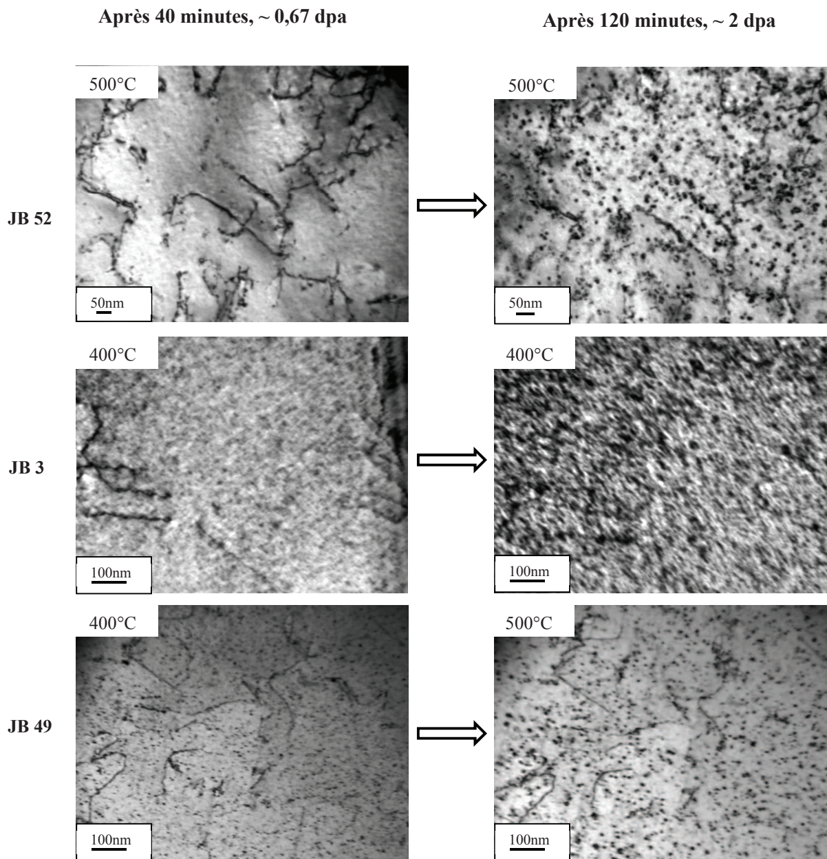
Figure II.31 : Evolution de la microstructure en fonction de la température après 0,67 dpa et 2 dpa
