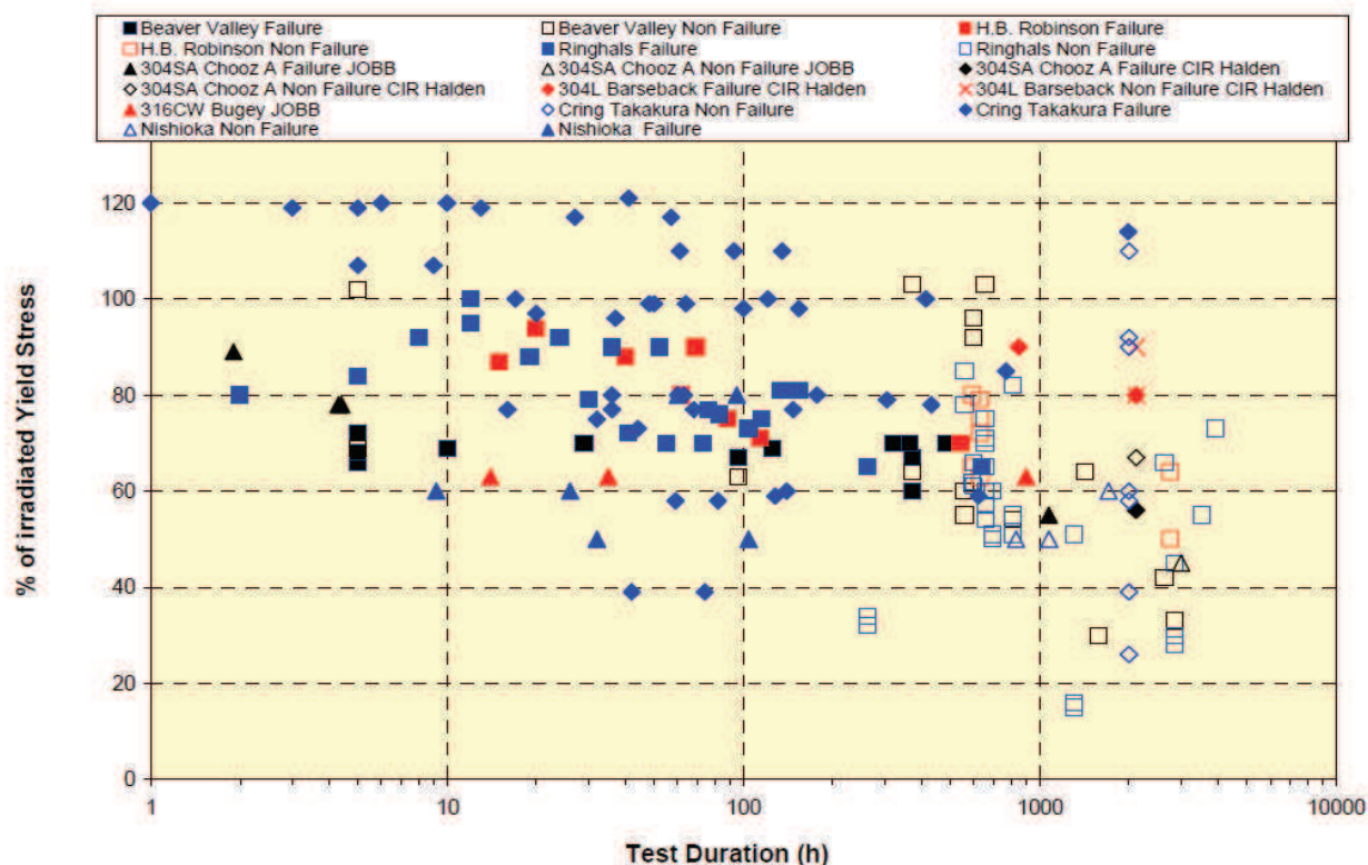
Figure I.36 : Contrainte macroscopique d'amorçage de l'IASCC en fonction de la durée d'essai sous charge constante [Fyftch 2009]
