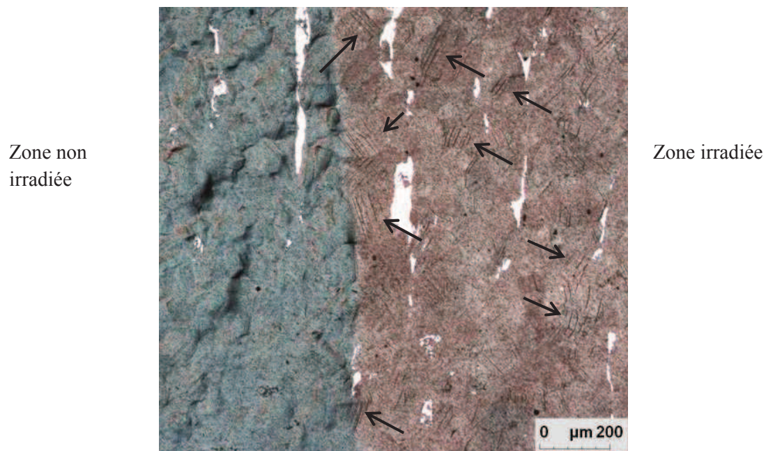
Figure III.48 : Image par microscopie optique de l'interface irradiée / non irradiée en surface de l'éprouvette E après 1% de déformation macroscopique –à droite la zone irradiée et à gauche la zone non irradiée. Les bandes blanches sont des bandes de ferrite. Les flèches noires désignent les bandes de déformation visibles sur la zone irradiée.
