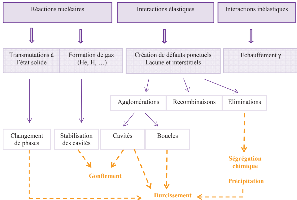
Figure I.5: Conséquences de l'irradiation sur les matériaux métalliques d'après [Barbu 2008] et [Was 2007a]
