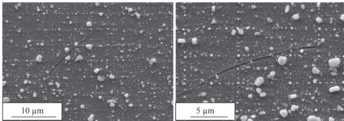
Figure III.30: Fissures apparues en surface de la zone non irradiée de l'éprouvette E après 1% de déformation
