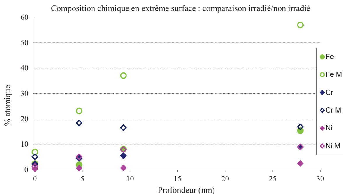
Figure II.13 : Analyses XPS de 0 à 28 nm des éléments majoritaires du 304L avec M =matériau non irradié
