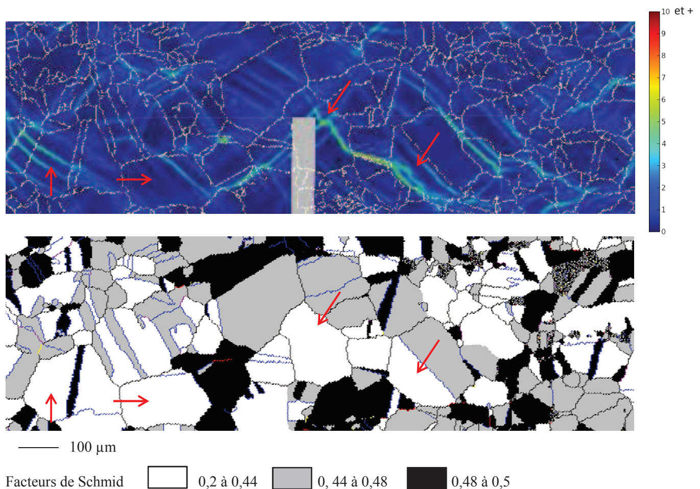
Figure III.46 : Comparaison entre le champ de déformation et les cartographies EBSD des facteurs de Schmid. Les flèches rouges indiquent des grains avec un faible FS mais qui sont parmi les plus déformés après 1% de déformation totale sur la zone irradiée.
