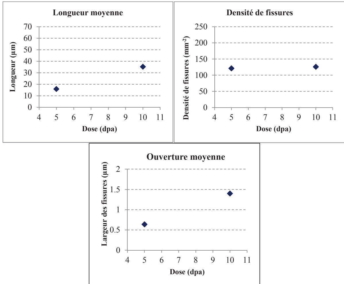
Figure III.27: Evolution du réseau de fissures d'un acier 304L déformé sous chargement monotone jusqu'à 10% en fonction de la dose d'irradiation
