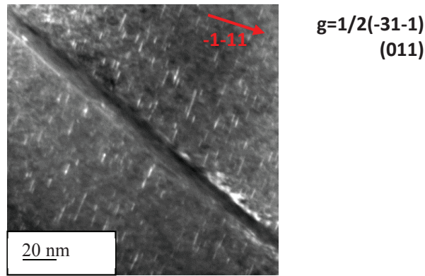
Figure IV.13 : Micrographie en fond noir, visualisation des boucles de Frank dans la matrice en conditions deux ondes g = 1/2(-31-1)
