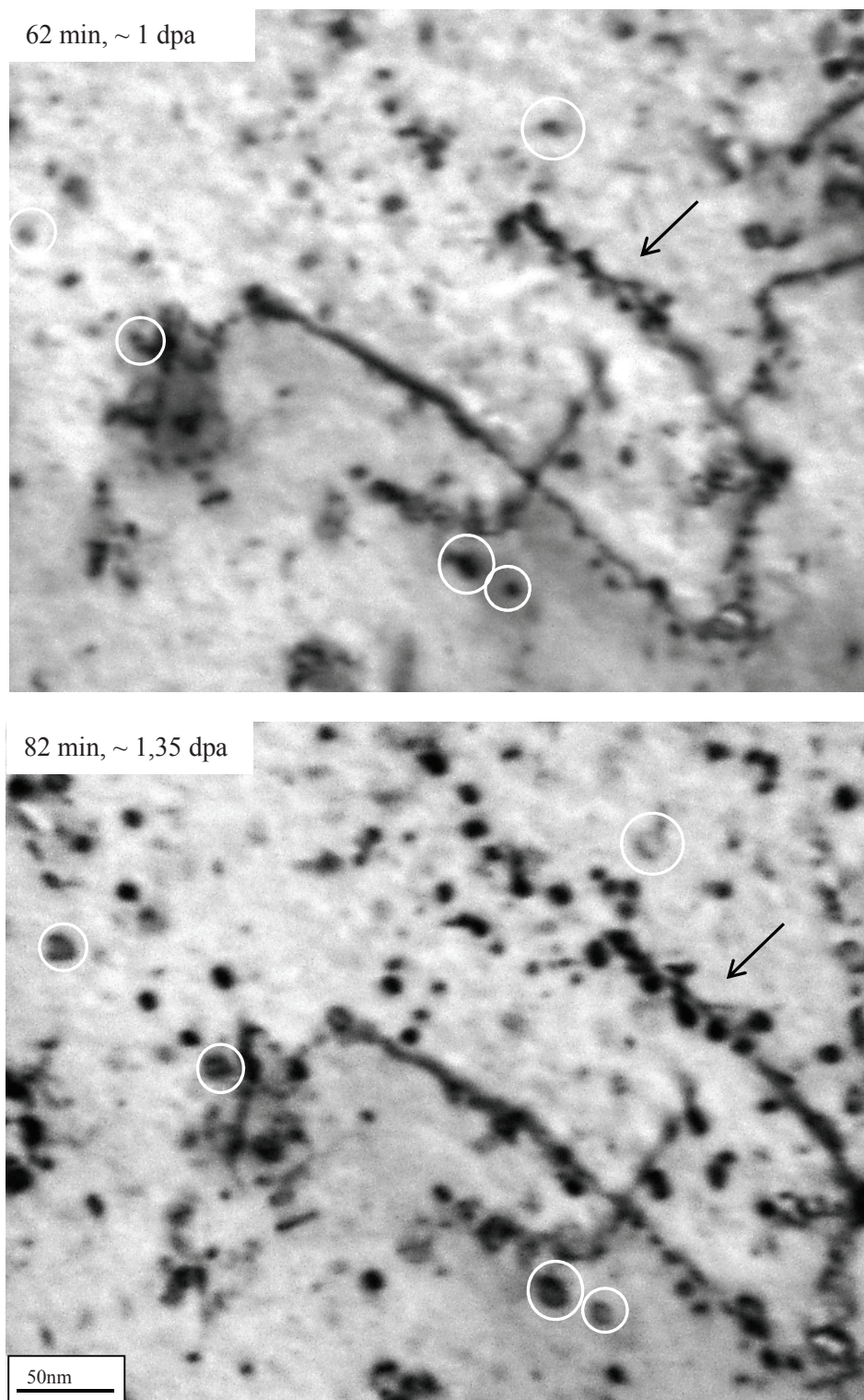
Figure II.30 : Boucles de dislocations après 1 et 1,35 dpa à 500°C – la flèche indique une grappe de défaut sur une ligne de dislocation et les cercles entourent les black dots (1 dpa) évoluant en boucles bien résolues (1,35 dpa)
