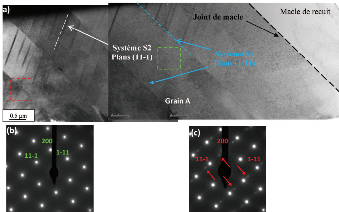
Figure IV.14 : Fissure A – (a) micrographie MET en fond clair du grain A en condition d'axe de zone [011] (b) cliché de diffraction correspondant au carré vert – un cliché de diffraction similaire est trouvé pour toute zone située entre les bandes de déformation des systèmes S1 et S2, (c) cliché de diffraction correspondant à la zone entourée en rouge – des taches de diffraction caractéristique d'une macle sont indiquées par des flèches rouges (plans de macle (1-11) )
