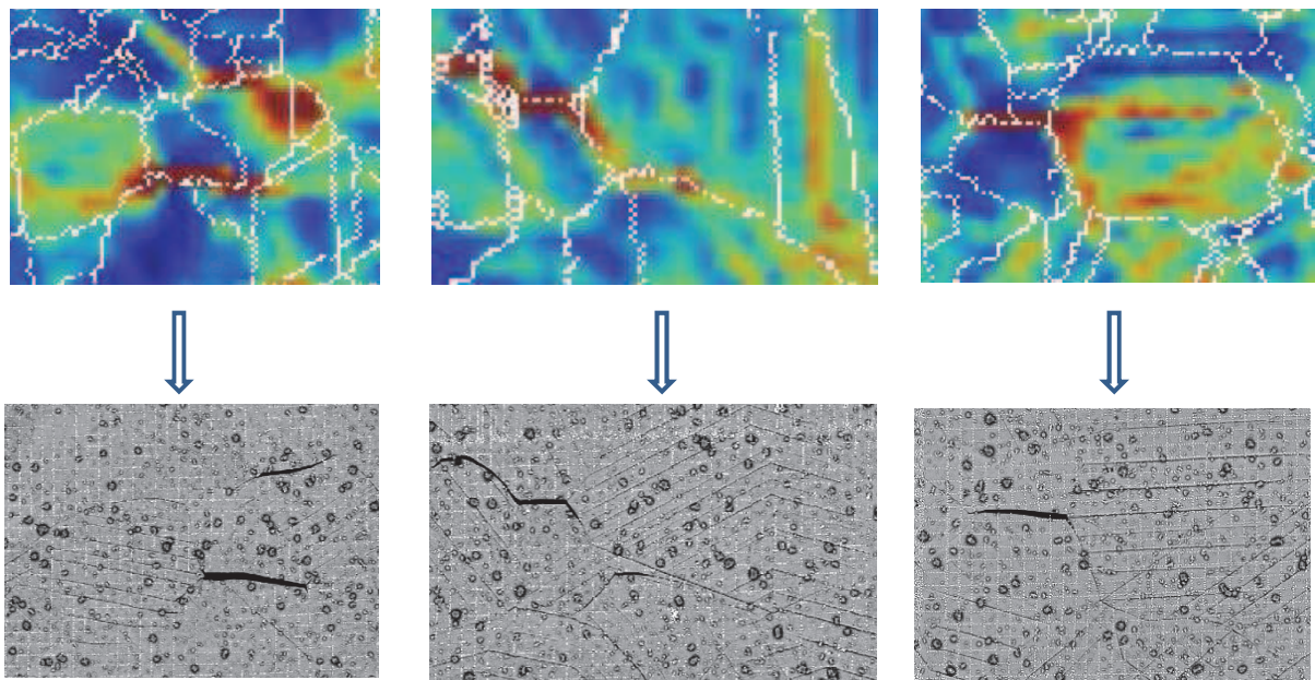
Figure III.41 : Exemples de joints fissurés et champs de déformation associés. Des bandes de déformation émergentes sont reconnaissables en surface des grains qui apparaissent fortement déformés sur les champs.
