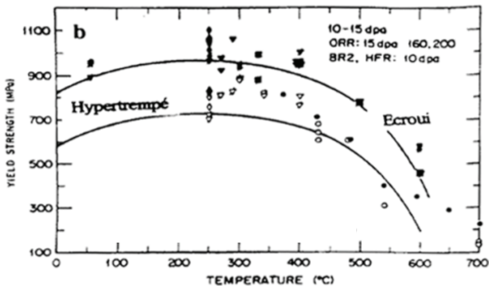
Figure I.24: Evolution de la limite d'élasticité d'aciers austénitiques en fonction de leur état métallurgique et de la température d'irradiation [Odette 1991]
