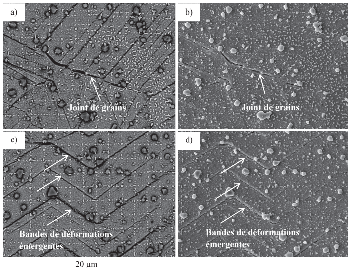
Figure III.11 : Exemple d'images (a) et (c) en électrons rétrodiffusés, (b) et (d) en électrons secondaires de deux zones de la surface de l'éprouvette E (5 dpa) après 10% de déformation
