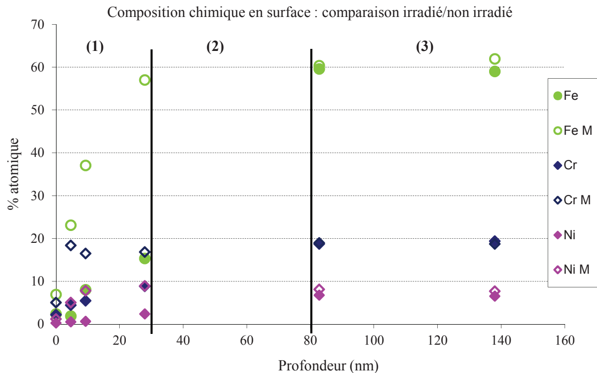
Figure II.11 : Analyses XPS de 0 à 140 nm des éléments majoritaires du 304L avec M=matériau non irradié
