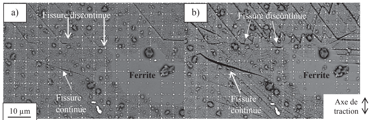
Figure III.17 : (a) Eprouvette E après 1% de déformation, (b) même zone après 5% de déformation
