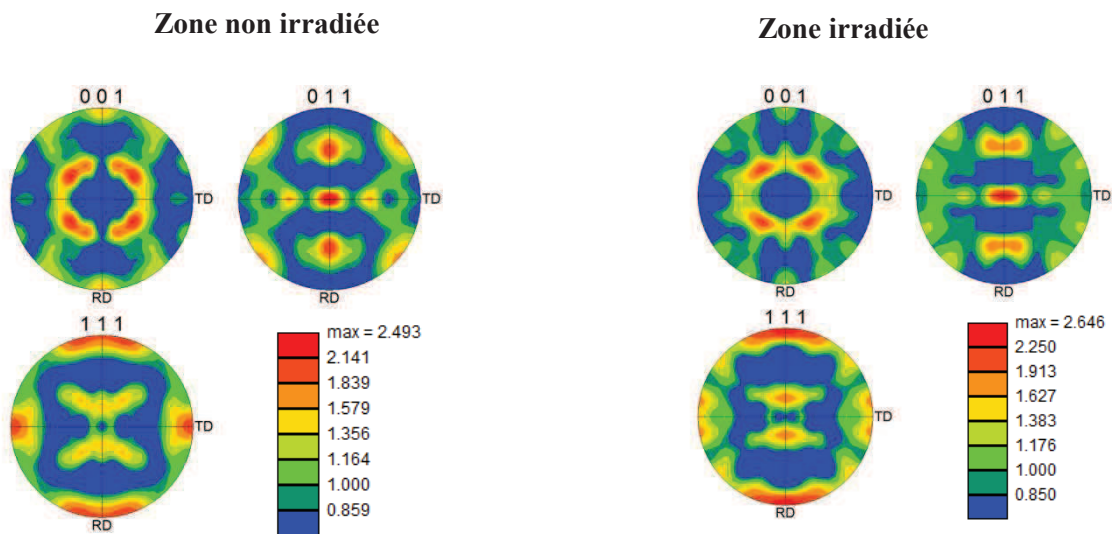
Figure II.15: Figures de pôles de la matrice austénitique – comparaison entre zones irradiée et non irradiée
