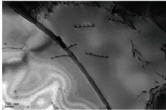
Figure D.2 : Micrographie en fond clair après recuit de 2h30 à 490°C puis polissage électrolytique d'1s – absence de précipités
