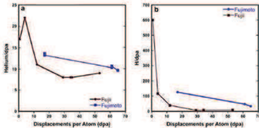
Figure I.17: Concentrations moyennes en hélium (a) et hydrogène (b) mesurées par Fujimoto et Fujii [Fujimoto 2005, Fujii 2002]
