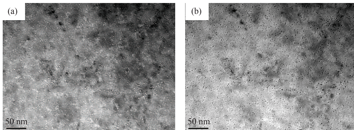
Figure C.4 : 304L irradié aux ions nickel à 2 dpa et 500°C en (a) sous-focalisation et (b) sur-focalisation (b) – présence de cavités
