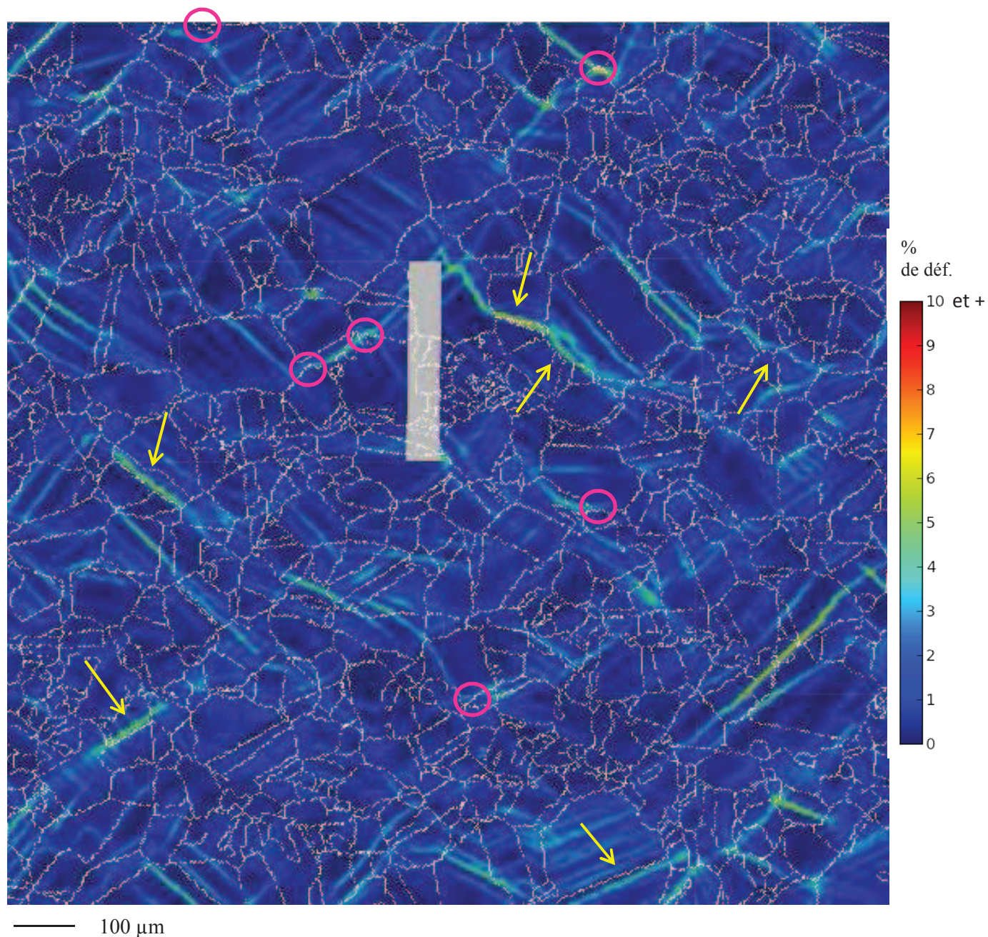
Figure III.45 : Champ de déformation équivalente de Von Mises après 1% de déformation macroscopique à 2.10^{-7} \text{ s}^{-1} sur l'acier 304L irradié à 5 dpa. Les cercles roses désignent les principaux joints fissurés. Les flèches jaunes indiquent les joints déformés non fissurés (CSLs ou généraux).
