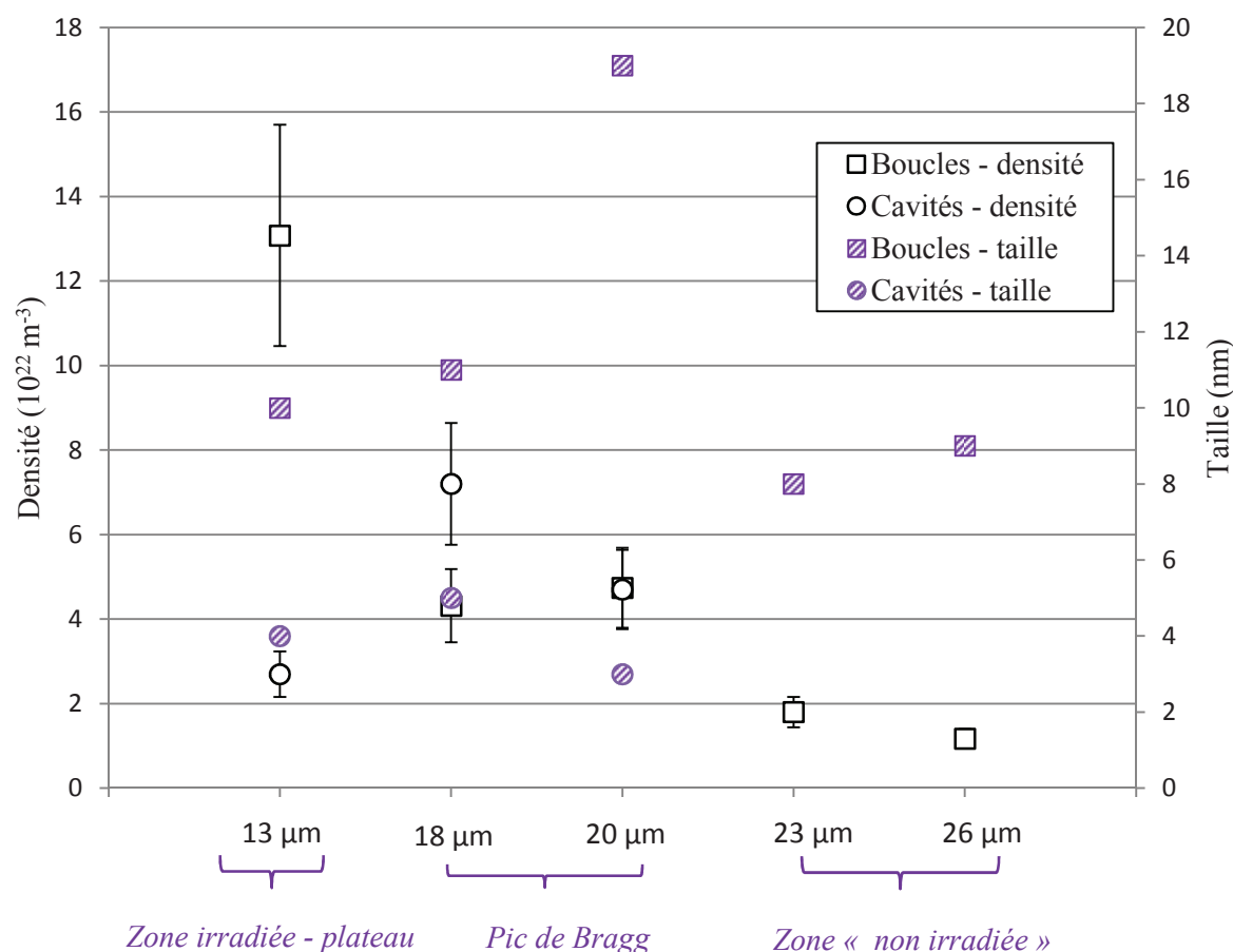
Figure II.20 : Evolution des densités et tailles de défauts en fonction de la profondeur d'irradiation sur un 304L – irradiation aux protons 2 MeV à 5 dpa et 360°C
