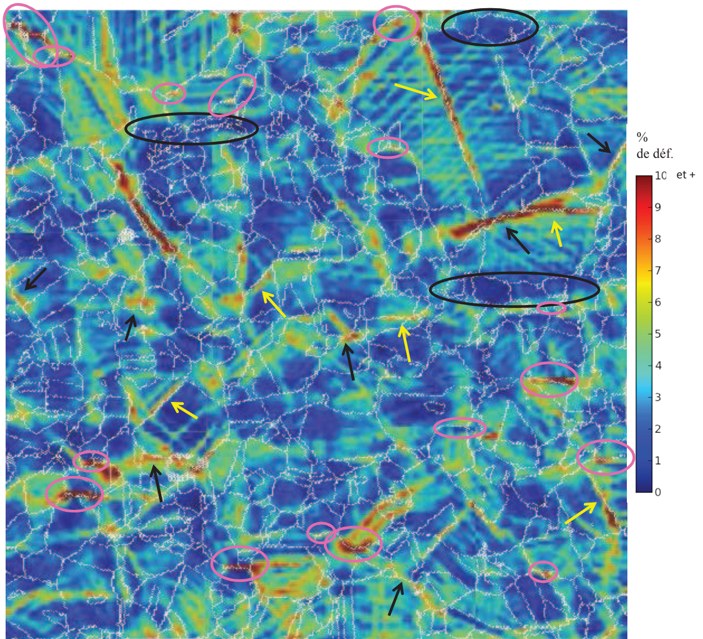
Figure III.40 : Champ de déformation équivalente de Von Mises sur l'acier 304L irradié à 5 dpa et déformé jusqu'à 2% de déformation macroscopique à 2.10^{-7} \text{ s}^{-1} . Les zones en bleu sont les moins déformées et celles en rouge les plus déformées. Les cercles roses désignent les principaux joints fissurés. Les flèches noires et jaunes signalent respectivement les joints généraux et spéciaux fortement déformés mais non fissurés et les cercles noirs les bandes de ferrite.
