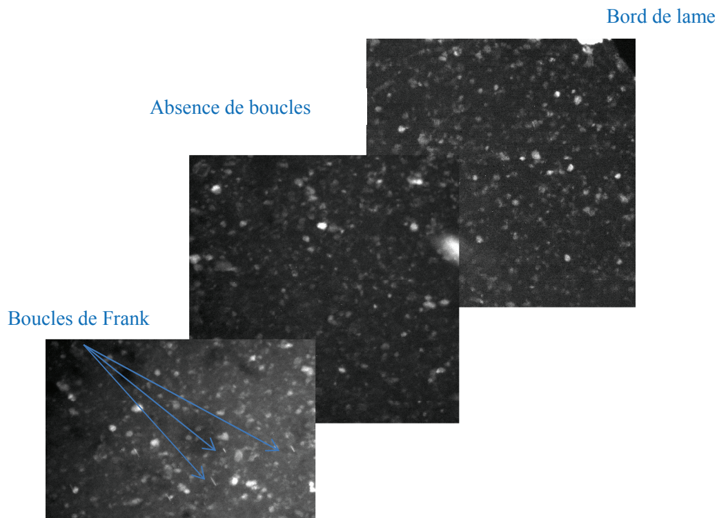
Figure II.32 : Zone dénudée en boucles de Frank en bord de lame. Apparition des premières boucles pour une épaisseur supérieure à 50 nm.
