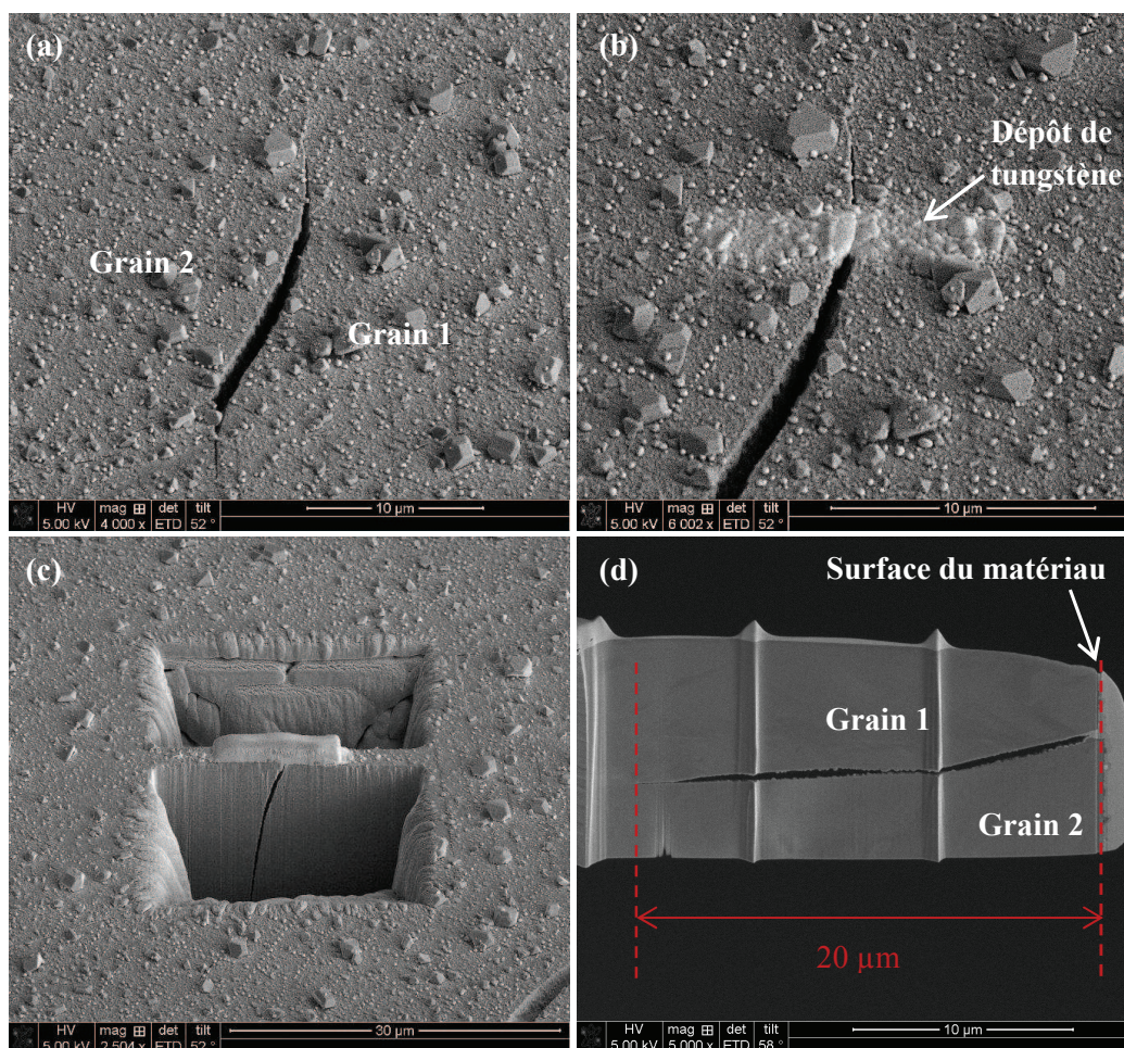
Figure IV.4 : Prélèvement par FIB de la fissure D, (a) vue générale en surface, (b) zone de prélèvement ; la trace de contraste plus clair indique le dépôt de tungstène fait en surface avant le prélèvement, (c) vue en cours d'amincissement, (d) vue générale de la lame mince
