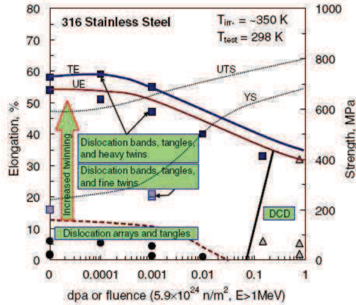
Figure 1.27: Carte de déformation pour un acier 316 irradié aux neutrons entre 65°C et 100°C et testé en traction à température ambiante [Farrell 2004]- DCD : Dislocation Channeling Deformation, UE : Uniform Elongation, TE : Total Elongation
