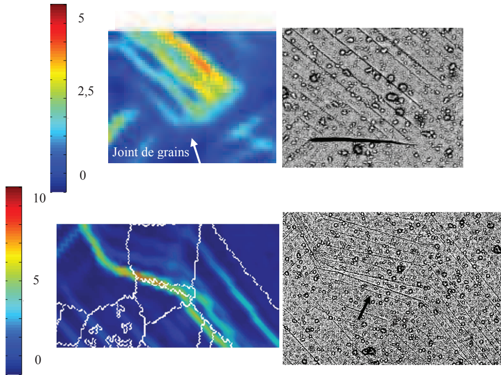
Figure IV.24 : (a) Localisation de la déformation intragranulaire après 1% de déformation macroscopique, pas de localisation sur le joint, (b) image MEB de la même zone après 5% de déformation, le joint a fissuré – (c) Localisation de la déformation sur un joint de grains après 1% de déformation et (d) image MEB de la même zone après 5% de déformation, joint non fissuré
