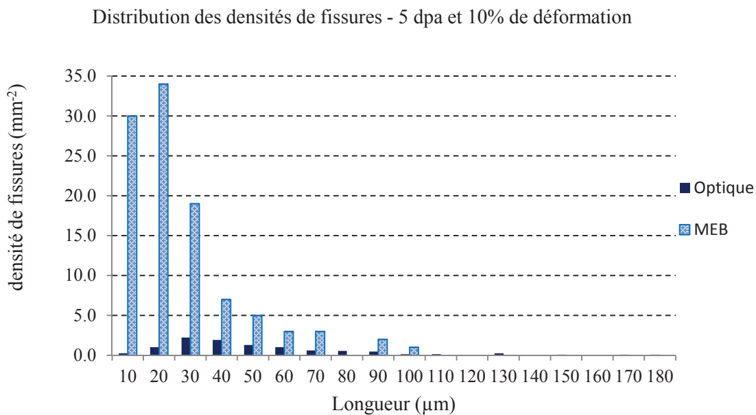
Figure III.12 : Distribution des densités de fissures détectées par longueur sur l'éprouvette A en fonction de l'outil de détection
