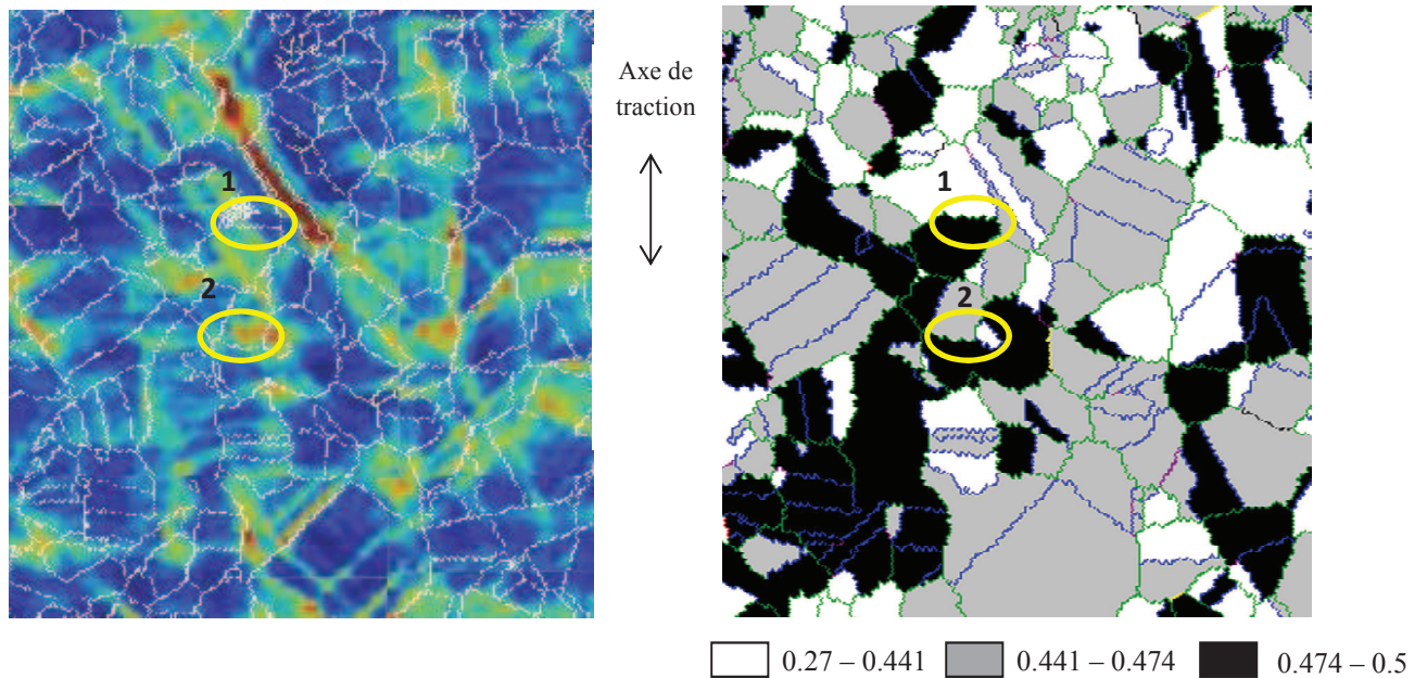
Figure III.43 : Champs de déformation et cartographie de FS associée ; en jaune deux joints généraux perpendiculaires à l'axe de traction et non fissurés.
