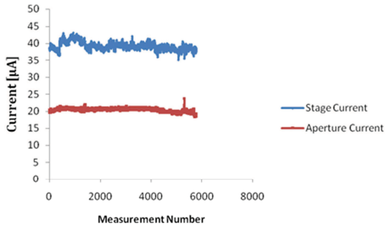
Figure II.8 : Suivi du courant de faisceau au niveau du montage (en bleu) et du courant correspondant à l'ouverture en tantale fixée au-dessus de la zone à irradier (en rouge) durant l'irradiation
