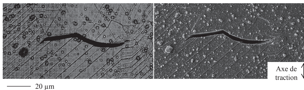
Figure III.10 : Fissure intergranulaire présente en surface de l'éprouvette D (5 dpa, 2% de déformation) imagée (a) en électrons rétrodiffusés et (b) en électrons secondaires.
