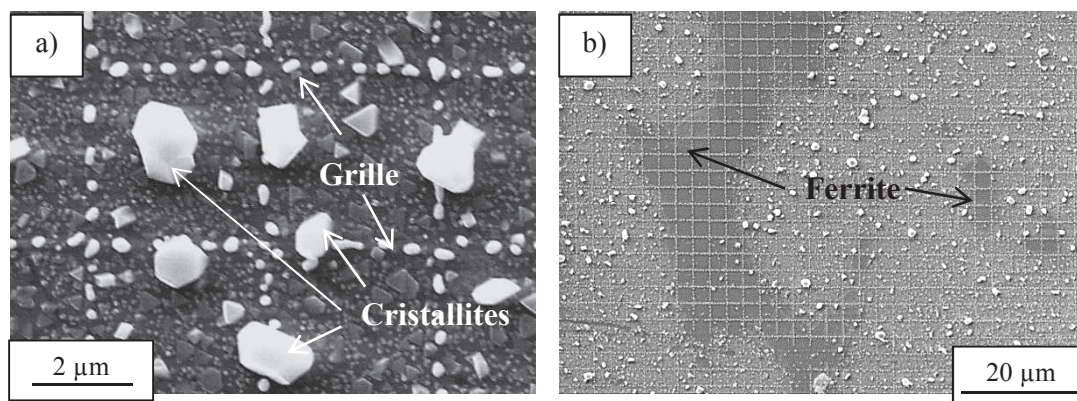
Figure III.6 : Dégradation des grilles d'or après exposition en milieu primaire REP à 350°C pendant environ 210h – les micrographies sont volontairement très contrastées pour faire apparaître (a) la globulisation de l'or et (b) la différence d'oxydation de la ferrite
