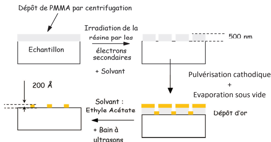
Figure III.4 : Schéma de principe de la microlithographie électronique [Doumalin 2000]
