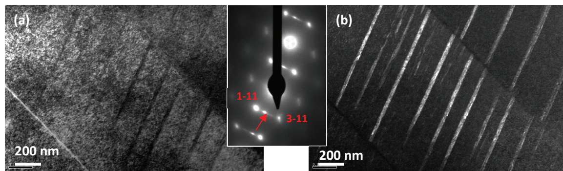
Figure IV.16 : Bande de déformation du système S2 - micrographie MET et cliché de diffraction associé (a) fond clair (b) fond noir réalisé sur la traînée de diffusion indiquée par une flèche rouge.
