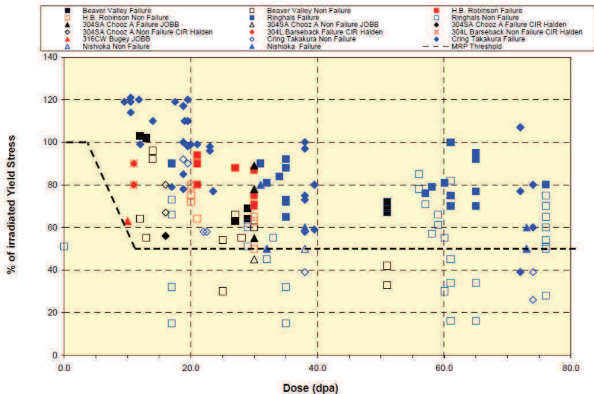
Figure I.35 : Contrainte macroscopique d'amorçage de l'IASCC en fonction de la dose pour des essais sous charge constante[Fyfe 2009]
