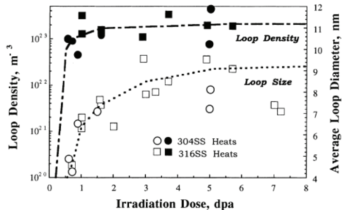
Figure I.7 : Densité et taille des boucles en fonction de la dose pour des irradiations à 280°C en milieu REP ou REB [Bruemmer 1999]
