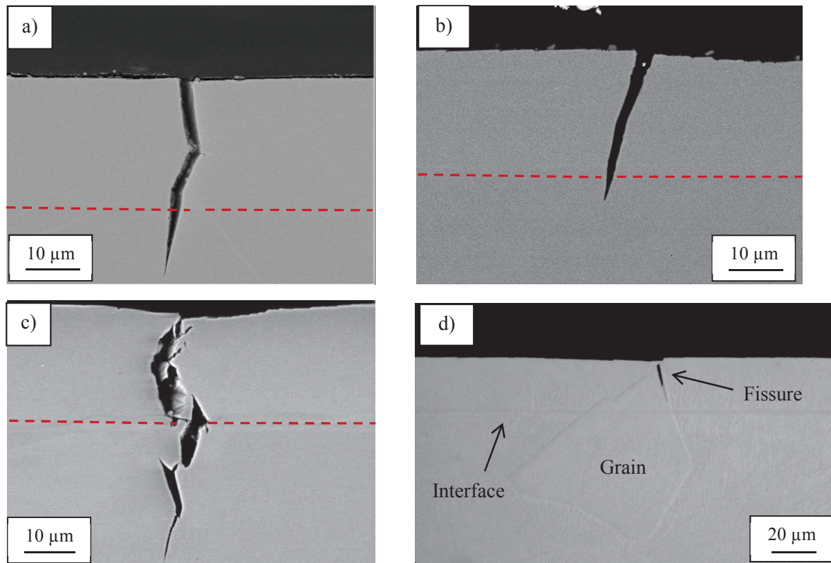
Figure III.23 : Coupes transverses (a) éprouvette A, 5 dpa, 10% de déformation (monotone), (b) éprouvette E 5 dpa, 10% de déformation (pseudo-cyclique), (c) éprouvette B, 10 dpa, 10% de déformation (monotone), (d) éprouvette A, microscopie optique. L'interface irradié / non irradié est en pointillés rouges sur les images a, b et c.
