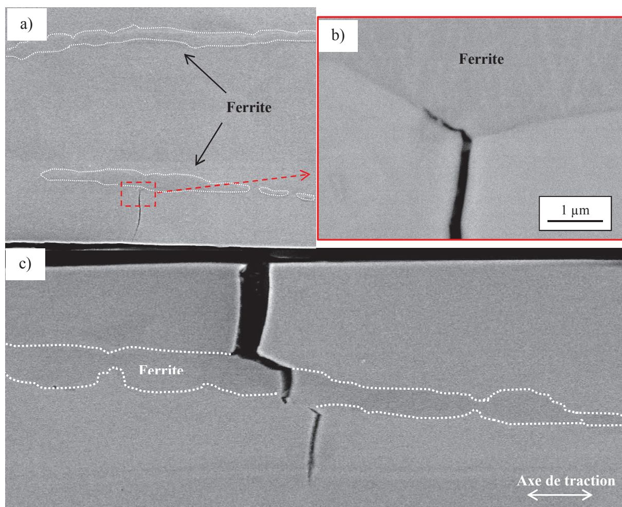
Figure III.22: Coupes transverses MEB : (a) et (b) éprouvette A, 10% de déformation et 5 dpa, (c) éprouvette B, 10% de déformation et 10 dpa
