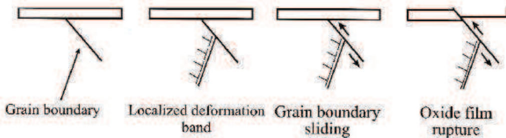
Figure I.39 : Mécanisme schématisé de la rupture du film d'oxyde suite au glissement du joint de grains [Was 2007a]
