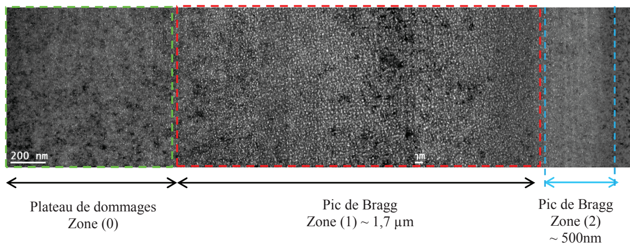
Figure II.18 : Cavités imagées en sous-focalisation le long de la lame FIB suite à l'irradiation aux protons à 360°C et 5 dpa de l'acier 304L
