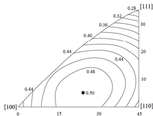
Figure III.33 : Cartographie des facteurs de Schmid en fonction de l'orientation cristalline dans un C.F.C.
