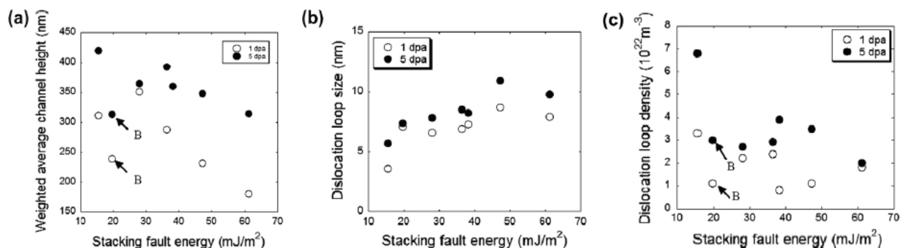
Figure I.38 : Effets de l'E.D.E. sur (a) les hauteurs des marches en surface, (b) la taille et (c) la densité des boucles de dislocation [Jiao 2010]
