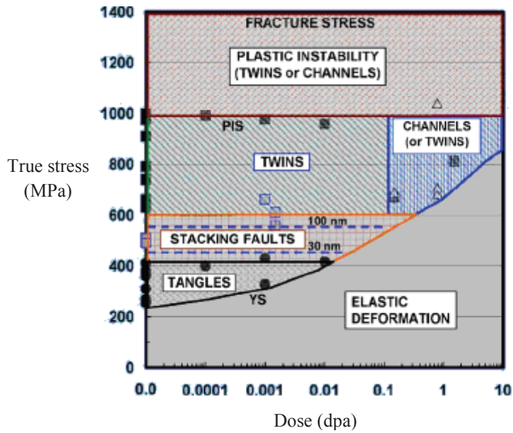
Figure I.28 : Carte de déformation d'un acier 316 en fonction de la dose et de la contrainte vraie [Byun 2006]
