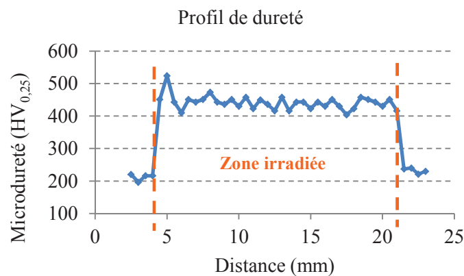
Figure II.9: Profil de dureté le long de la longueur (L=18mm) de la zone irradiée ; la charge appliquée est de 25g
