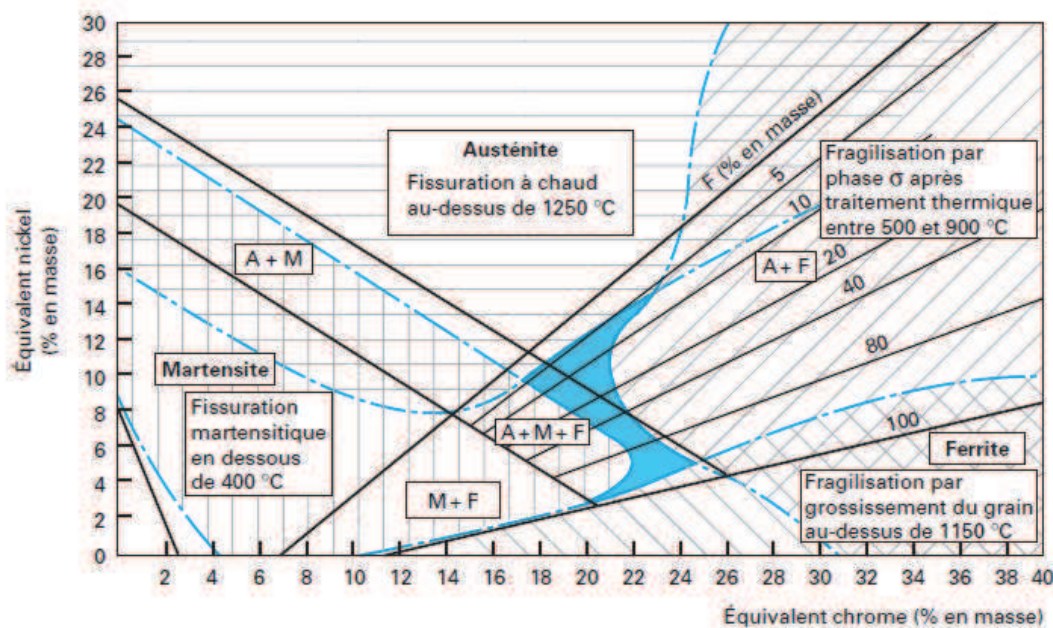
Figure I.2 : Diagramme de Schaeffler d'après [Cunat 2000]
