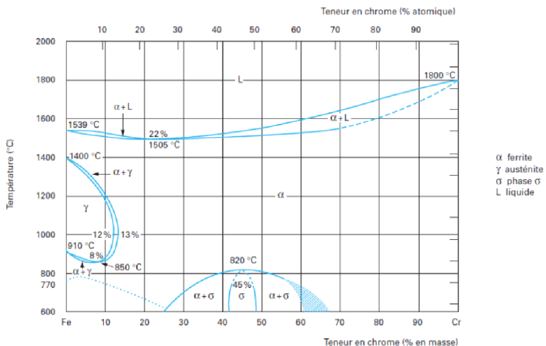
Figure I.1 : Diagramme de phase Fe-Cr d'après [Cunat 2000]
