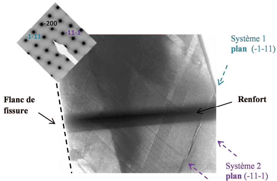
Figure IV.10 : Fissure D - fond clair dans le grain 1 en axe de zone [011] – bandes de déformation orientées parallèlement aux plans (-1-11) et (-11-1)
