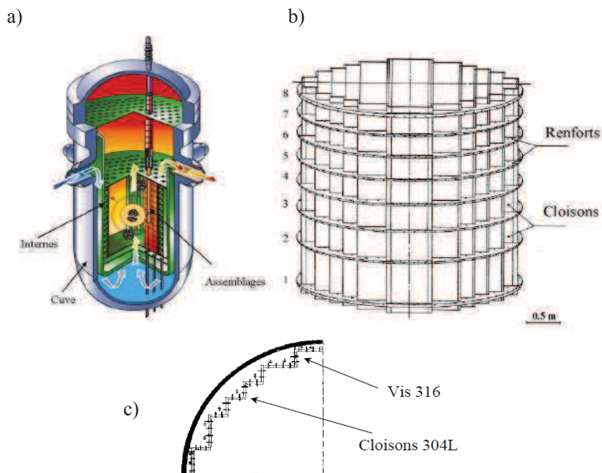
Figure 3 : (a) Vue intérieure d'une cuve de réacteur à eau sous pression français, (b) renforts et structures internes, (c) coupe des structures internes [Pokor 2002]
