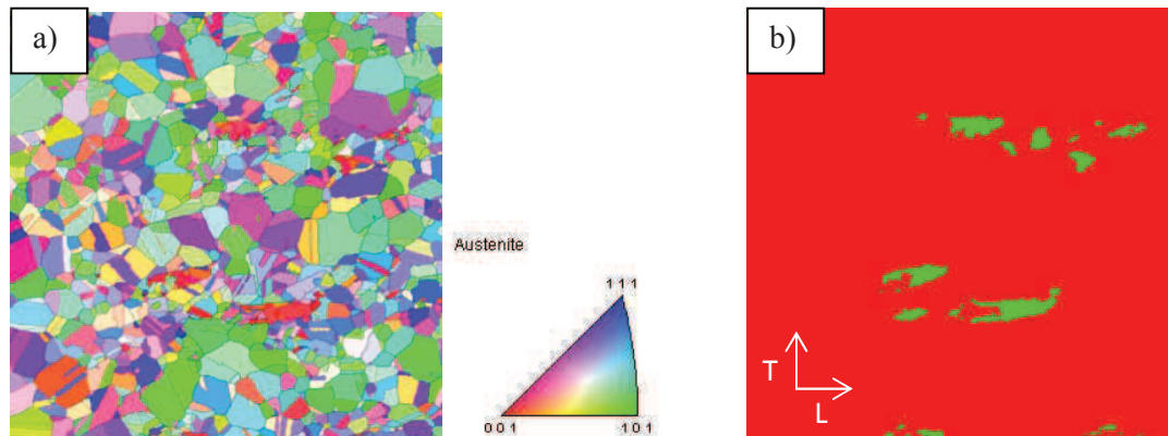
Figure II.2 : (a) Figure de pôles inverse selon [001] et (b) cartographie des phases de l'acier 304L étudié – en rouge l'austénite et en vert la ferrite
