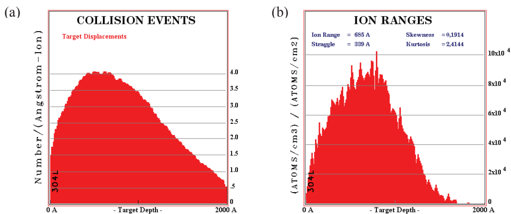
Figure II.24 : Simulations SRIM (a) du profil d'endommagement pour une irradiation aux ions \text{Ni}^{++} à 500 keV et un angle d'incidence de 45° et (b) du profil d'implantation des ions He à 20 keV et un angle d'incidence de 45°
