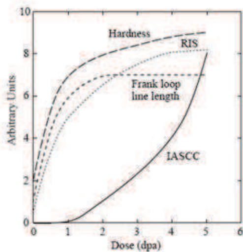
Figure I.33 : Représentation schématique des modifications liées à l'irradiation et sensibilité à l'IASCC en fonction de la dose [Was 2007a]
