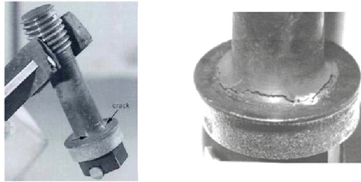
Figure 4 : Vis de cloisonnement en acier 316 présentant une fissure au niveau du congé. Cette vis provient du REP Tihange (Belgique) [Thomas 2002]
