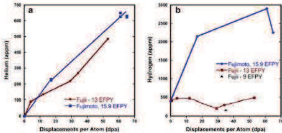
Figure I.17: Concentrations moyennes en hélium (a) et hydrogène (b) mesurées par Fujimoto et Fujii [Fujimoto 2005, Fujii 2002]
