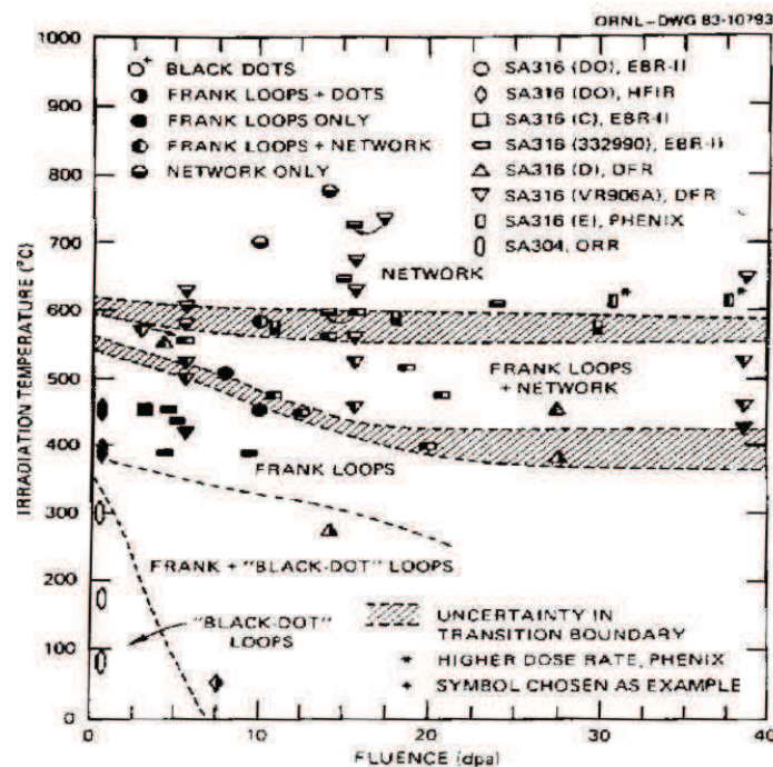
Figure I.8 : Domaine d'existence des boucles, black dots et réseau de dislocations d'[Maziasz 1993]
