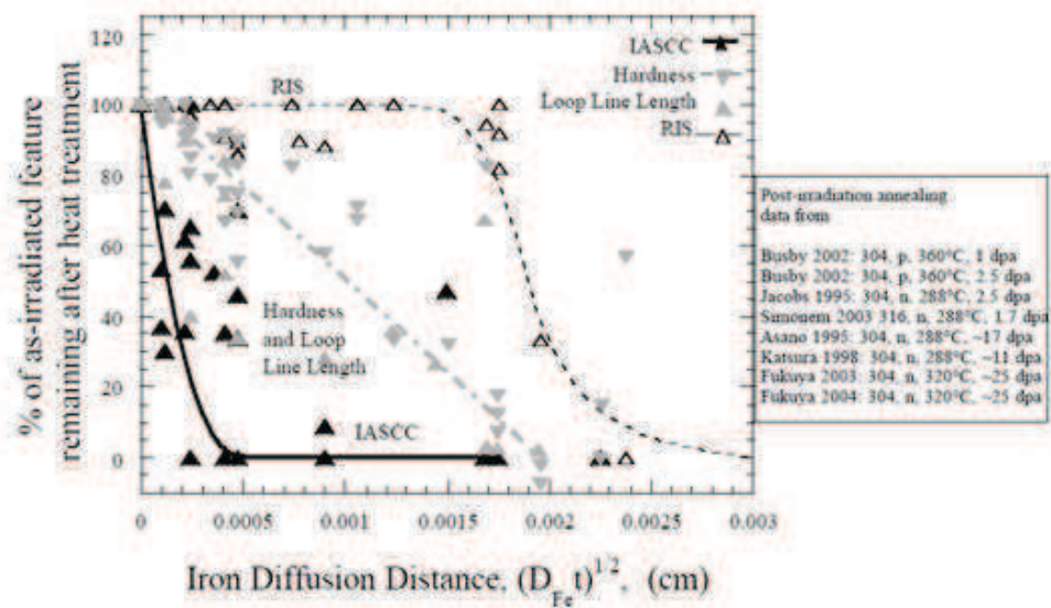
Figure I.32 : Restauration de la microstructure et de la microchimie par traitements thermiques et influence sur la sensibilité à l'IASCC [Was 2009]
