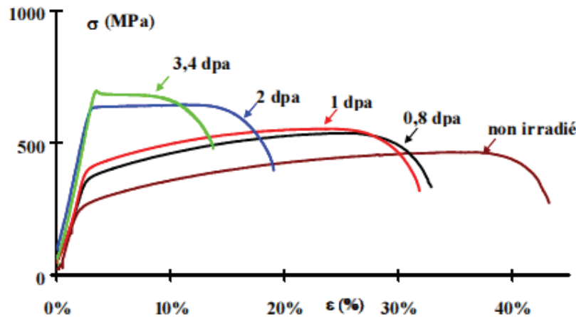
Figure 1.25 : Courbes de traction d'un acier 304 hypere trempé irradié et testé à 330°C [Pokor 2002]
