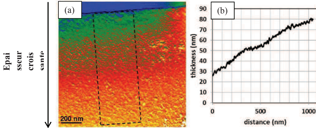
Figure C.2 : (a) Cartographie de l'épaisseur relative en bord de lame et (b) évolution de l'épaisseur avec la distance au bord correspondant au rectangle de l'image (a). Les couleurs de la cartographie donnent une information qualitative de l'épaisseur. Plus l'image est rouge, plus la lame est épaisse.
