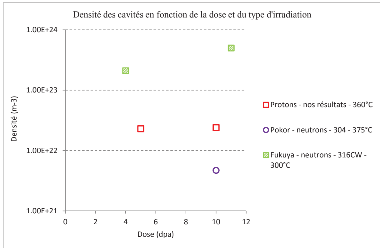
Figure II.22 : Comparaison des densités de cavités mesurées sur des aciers commerciaux de type 304 et 316 après irradiations aux protons et neutrons pour 5 et 10 dpa - les résultats comparatifs sont issus de [Pokor 2004] et [Fukuya 2006]
