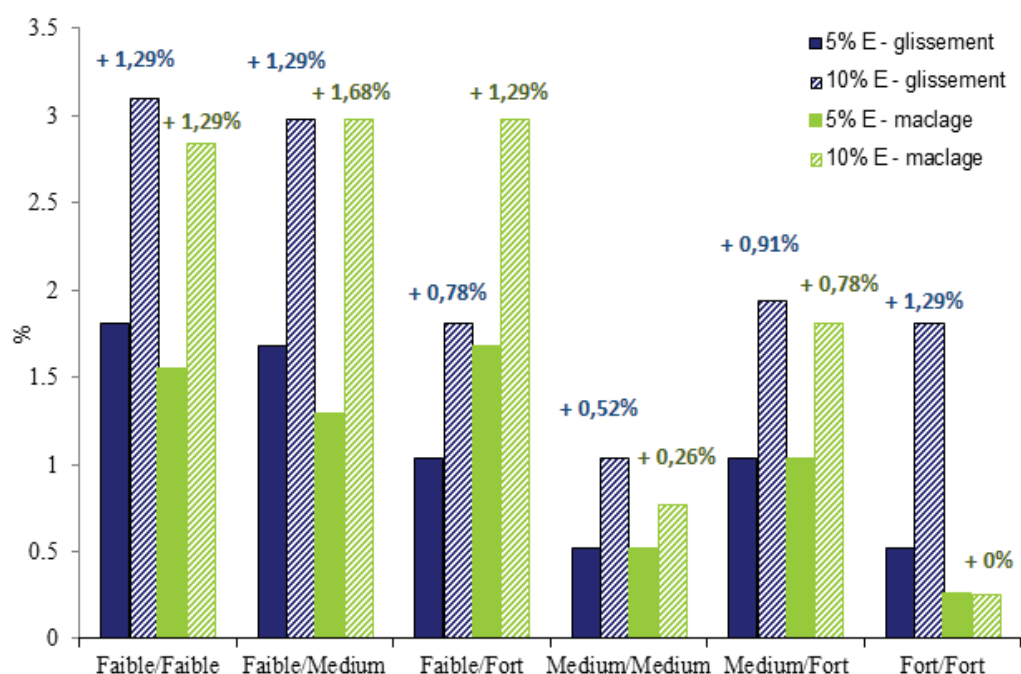
Figure IV.22 : Comparaison glissement / maillage sur le pourcentage de joints fissurés pour chacune des catégories en fonction du taux de déformation macroscopique – les pourcentages indiqués sont indépendants les uns des autres et les augmentations entre 5 et 10% de déformation sont signalés au-dessus des barres correspondantes
