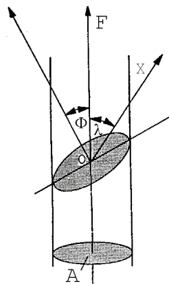
Figure I.34 : Représentation schématique de la loi de Schmid
