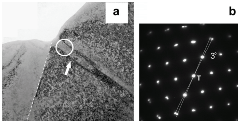
Figure IV.20 : Micrographie en fond clair sur un acier austénitique modèle irradié à 5,5 dpa et déformé à 7% – (a) intersection entre un joint de grains (en pointillé) et une bande de déformation, (b) cliché de diffraction en axe de zone \langle 110 \rangle - rotation du réseau cristallin de l'ordre de 3^\circ au niveau de l'élargissement de la bande de déformation à l'intersection avec la fissure [Jiao 2007]
