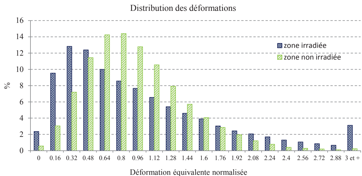
Figure III.49 : Distributions normalisées des déformations locales sur les zones irradiée et non irradiée de l'éprouvette E après 1% de déformation macroscopique
