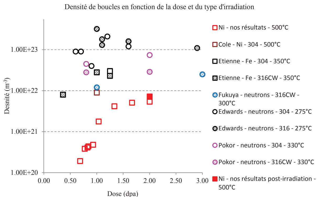
Figure II.37 : Comparaison des densités de boucles de Frank mesurées après des irradiations aux neutrons et aux ions lourds en fonction de la dose – les résultats présentés sont issus des références [Etienne 2010], [Cole 1995], [Fukuya 2006], [Edwards 2003] et [Pokor 2004]
