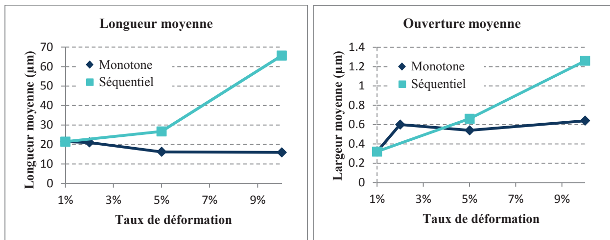
Figure III.25: Evolution de la longueur et de l'ouverture moyennes des fissures avec le taux de déformation en fonction du trajet de chargement (acier 304 L irradié à 5 dpa)
