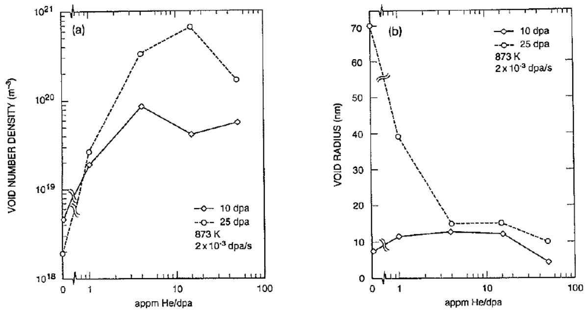
Figure II.40 : Dépendance au rapport He/dpa de la densité et de la taille moyenne des cavités dans un acier 316 irradié aux ions Ni à 600°C et 2.10^{-3} dpa.s -1 – les doses de 10 et 25 dpa ont été calculées via SRIM avec une énergie de déplacement du Fe fixée à 25 eV [Katoh 1994]
