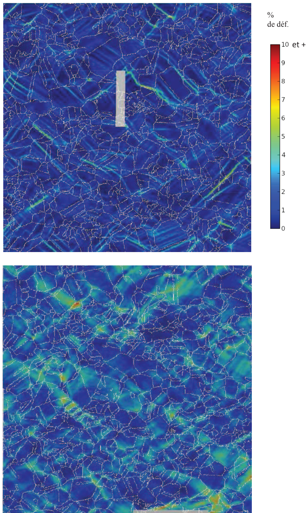
Figure III.47 : Champs de déformation équivalente de Von Mises après 1% de déformation à 2.10^{-7} \text{ s}^{-1} pour (a) une zone irradiée (5 dpa) et (b) une zone non irradiée de l'éprouvette E
