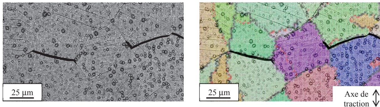
Figure III.15: Fissures intergranulaires en surface de l'éprouvette D (5 dpa) après 2% de déformation - à droite la superposition MEB/EBSD confirme leur caractère intergranulaire
