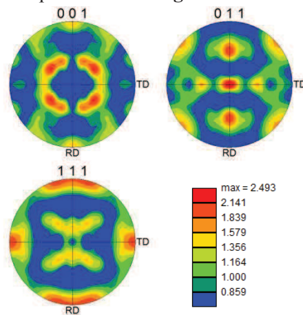
Figure II.3 : Figures de pôles avec symétrie orthotrope de la phase austénitique
