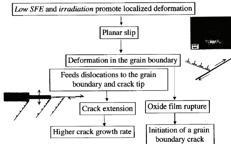
Figure I.40: Processus d'amorçage et de propagation des fissures favorisé par la localisation de la déformation [Was 2004]
