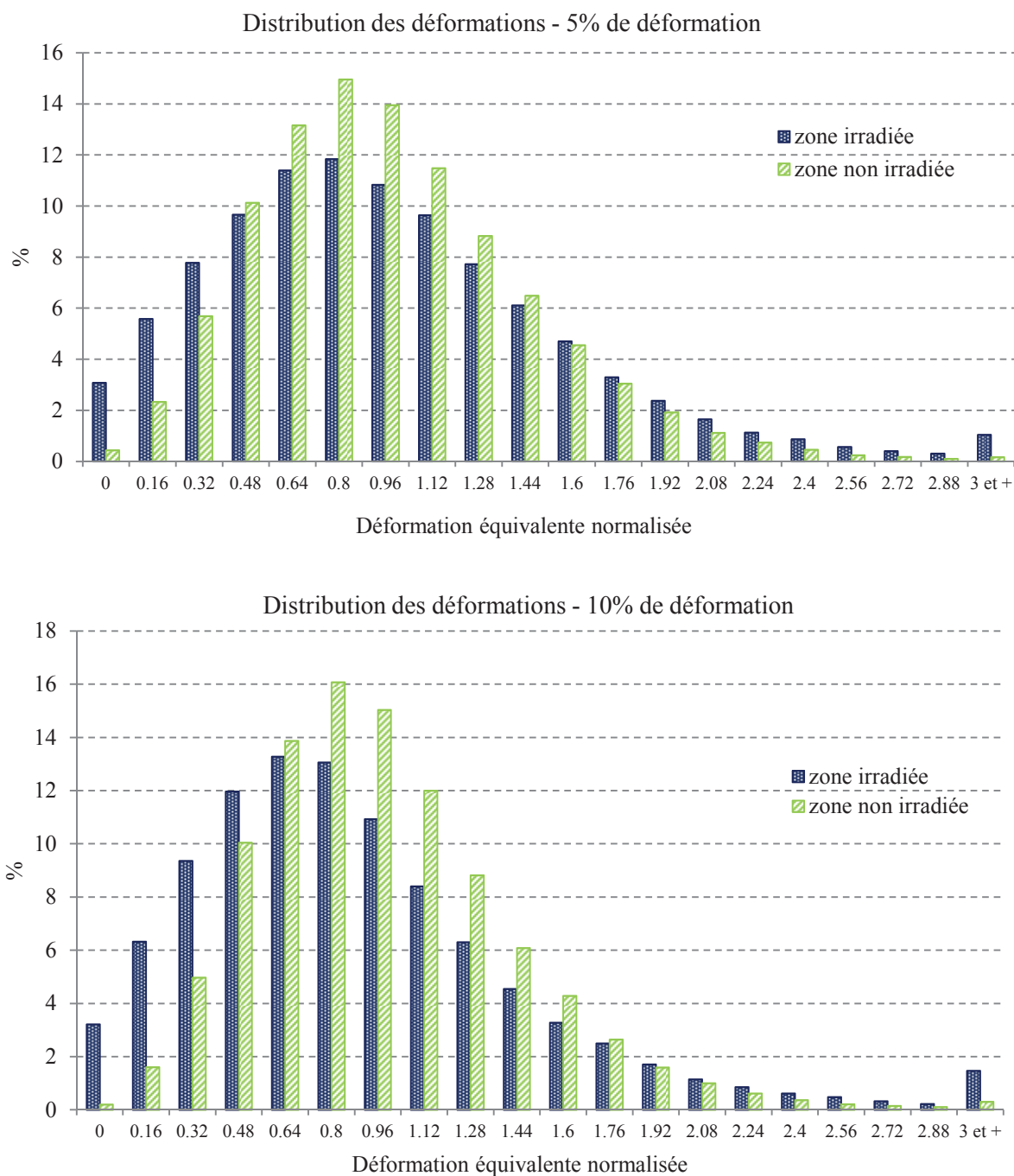
Figure III.54: Distributions normalisées des déformations après 5% (2 ème étape) et 10% (3 ème étape) de déformation macroscopique pour les zones irradiée et non irradiée de l'éprouvette E
