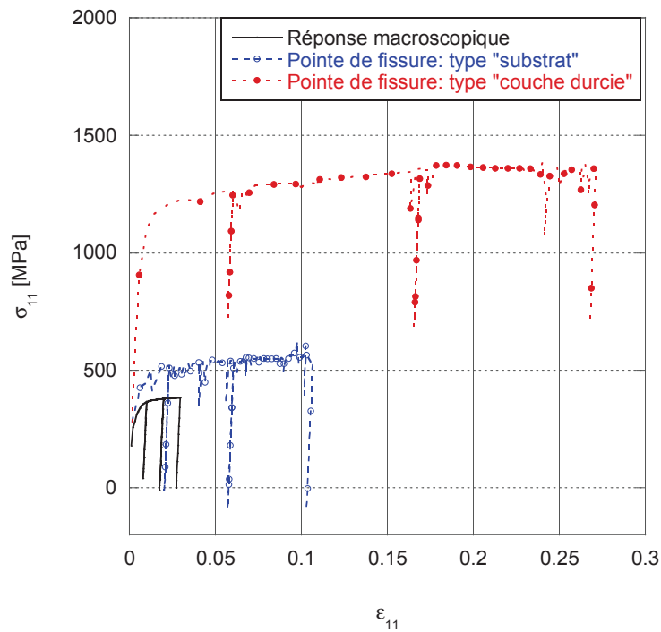
Figure IV.30 : Courbes contrainte – déformation en pointe de fissure à mi-épaisseur (M) de la couche irradiée pour un chargement séquentiel à 1, 2 puis 3% de déformation en fonction des propriétés mécaniques de la couche. En bleu, propriétés identiques au substrat, en rouge couche durcie. En noir, réponse globale de la structure
