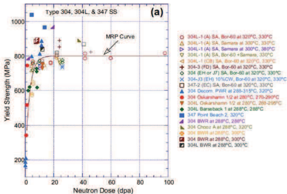
Figure I.23 : Effet de la dose sur la limite d'élasticité pour des aciers inoxydables austénitiques irradiés et testés entre 270°C et 380°C [Chopra 2011]
