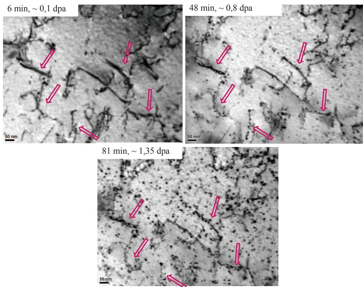
Figure II.27 : Apparition et croissance des défauts à 500°C - les flèches roses pointent des lignes de dislocations sur lesquelles se forment des amas de défauts. Les premiers défauts visibles apparaissent après 0,6 dpa environ
