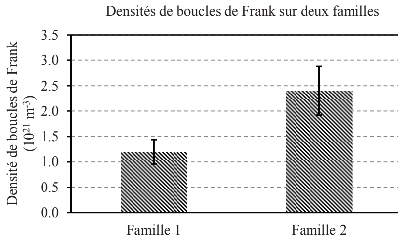
Figure II.33 : Densité des boucles de Frank pour 2 familles, après 2 dpa à 500°C et 0 appm He/dpa
