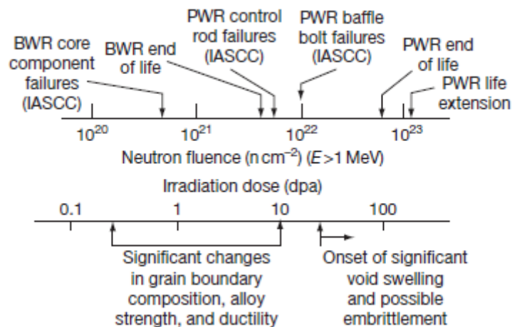
Figure I.31 : Effet de la dose sur la sensibilité à l'IASCC des aciers de type 304 en milieu REP et REB [Bruemmer 1999]
