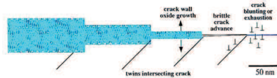
Figure I.29 : Schéma d'une pointe de fissure observée dans une vis en acier inoxydable 316, irradiée dans un réacteur à eau sous pression à une dose de 8,5 dpa et 299°C [Thomas 2002].
