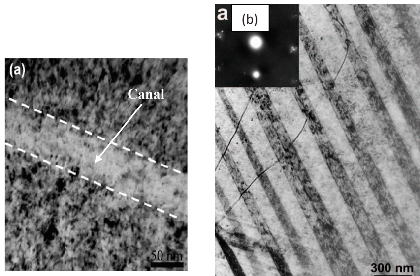
Figure I.26: Micrographies MET (a) d'un acier inoxydable irradié aux protons à 5 dpa et 360°C puis sollicité jusqu'à 7% de déformation à 288°C sous argon [Jiao 2010] et (b) macles observées après déformation de 10% à température ambiante sur un acier 316LN irradié à 200°C et 10 dpa aux ions Fe [Lee 2001a]
