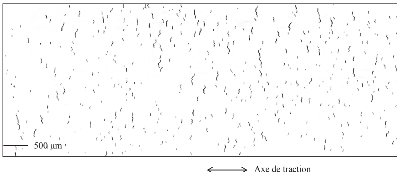
Figure III.9 : Reconstitutions seuillées des zones utiles à partir des images de microscopie optique : (a) éprouvette A, 5 dpa 10% de déformation imposée et (b) éprouvette B, 10 dpa, 10% de déformation imposée. Chaque ligne représente une fissure.
