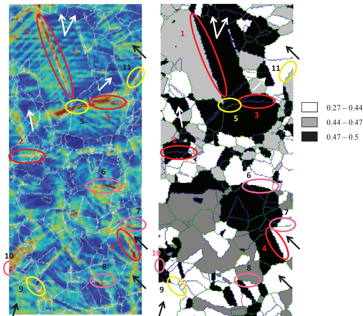
Figure III.44 : Comparaison entre champs de déformation et cartographie de FS. En rouge les joints \Sigma 3 et en jaune les joints généraux qui sont fortement déformés mais non fissurés. Les joints fissurés sont signalés en rose. Les flèches noires indiquent des grains ayant un faible FS mais pourtant déformés ; les flèches blanches indiquent des grains ayant un FS élevé mais pourtant peu déformés.
