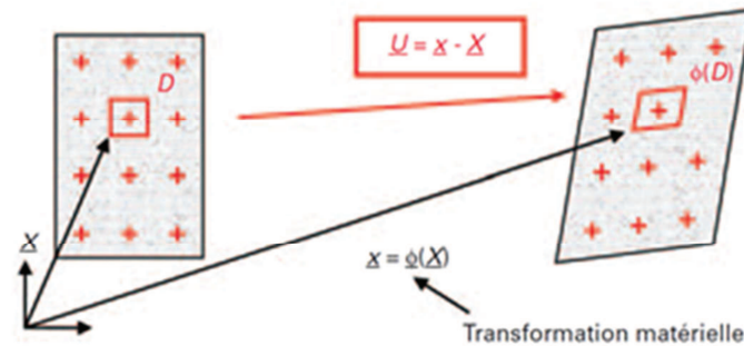
Figure III.37 : Principe de la mesure de champ par corrélation d'images, \underline{U} est le champ de déplacement [Brémand 2011]
