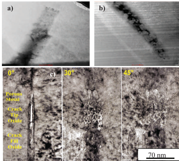
Figure IV.9 : Fissure A – (a) et (b) Images en STEM-HAADF des deux pointes de fissure, (c) Micrographies MET d'une pointe de fissure d'un acier 304L irradié à 0,7 dpa et déformé en milieu BWR [Bruemmer 2006]
