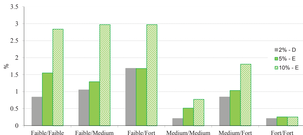
Figure IV.21 : Pourcentage de joints fissurés pour chacune des catégories en fonction du taux de déformation macroscopique
