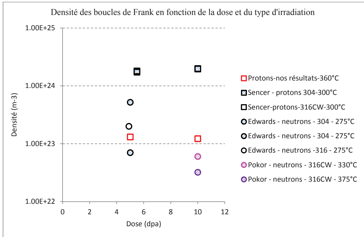
Figure II.21 : Comparaison des densités de boucles de Frank mesurées sur des aciers de type 304 et 316 après irradiations aux protons et neutrons pour 5 et 10 dpa – les résultats comparatifs sont issus de [Sencer 2003], [Edwards 2003] et [Pokor 2004]
