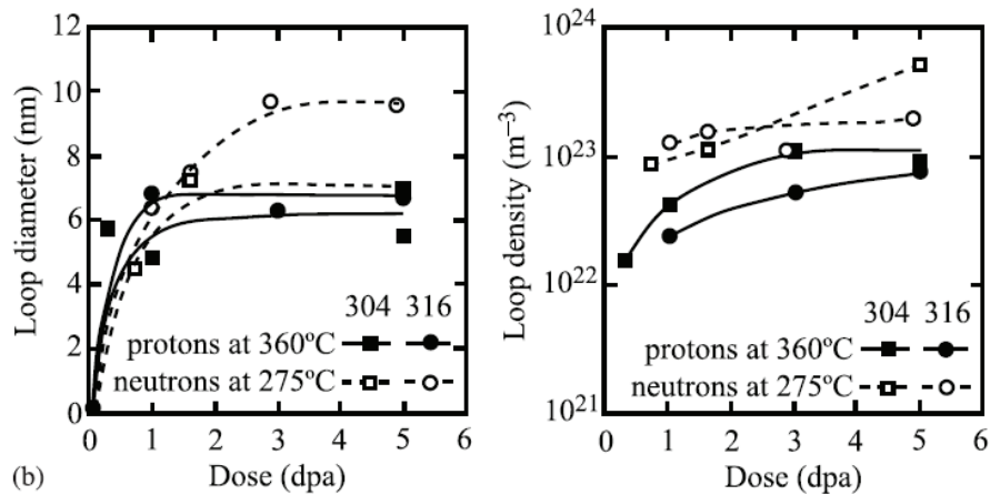
Figure I.22 : Comparaison de la taille et densité des boucles de dislocation après irradiations aux neutrons à 275°C et aux protons à 360°C d'un même acier austénitique commercial [Was 2002]
