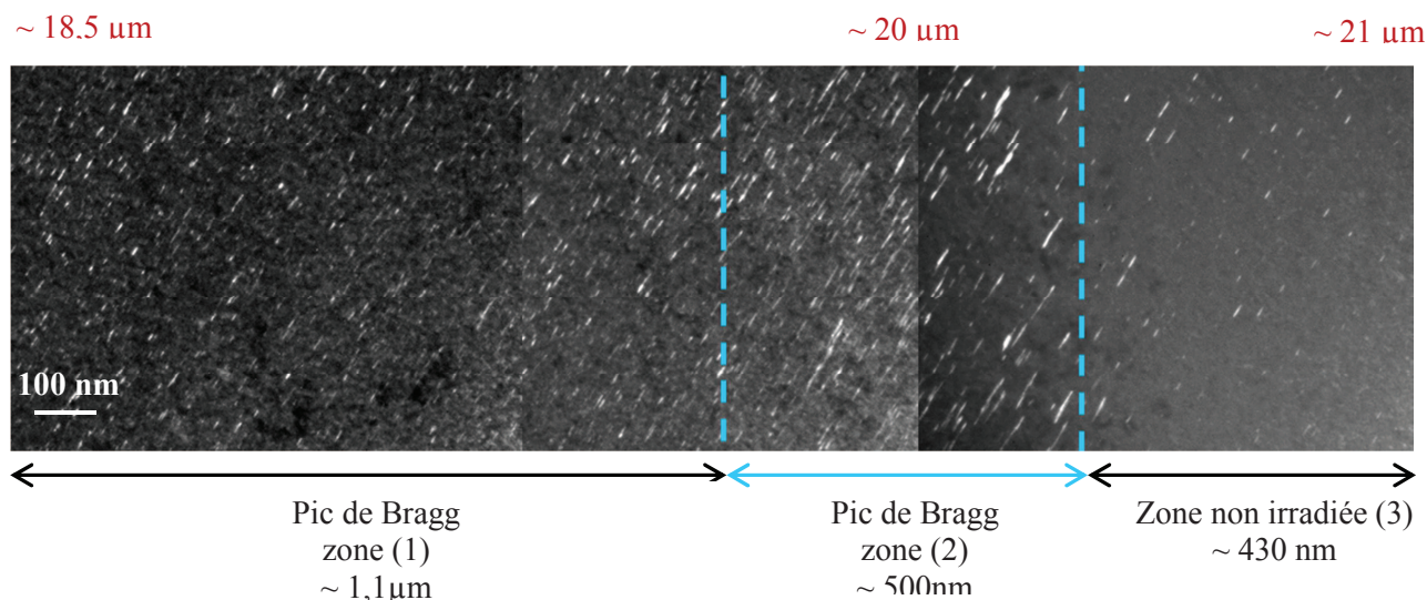
Figure II.17 : Boucles de dislocation imagées grâce à la technique de la traînée diffuse le long de la lame FIB suite à l'irradiation aux protons à 360°C et 5 dpa du 304L – les profondeurs depuis la surface du matériau sont indiquées en rouge
