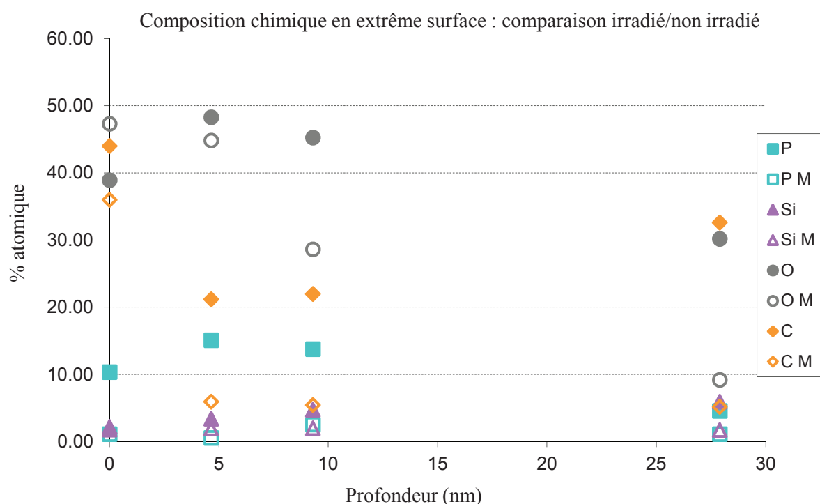
Figure II.14 : Analyses XPS de 0 à 28 nm des éléments minoritaires et impuretés du 304L avec M =matériau non irradié
