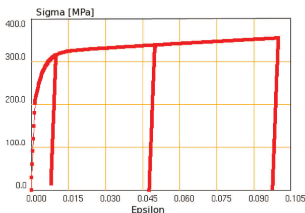
Figure IV.32: Courbe contrainte-déformation schématisant dans le cas d'un chargement séquentiel
