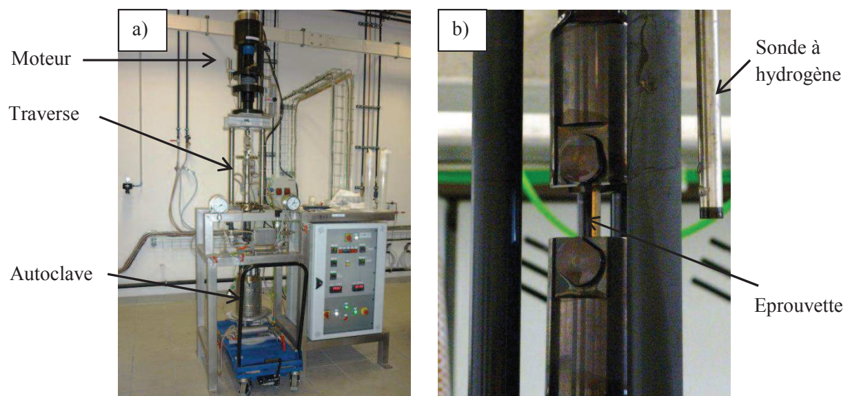
Figure III.7 : a) Machine de traction et autoclave, b) Système de maintien de l'éprouvette
