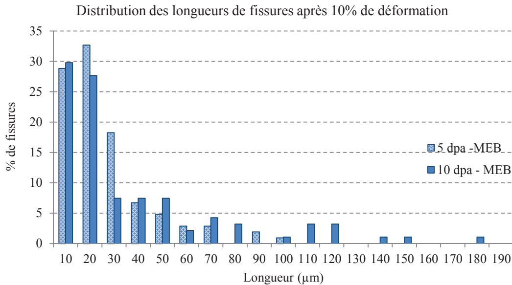
Figure III.14 : Distribution des longueurs de fissures pour 5 et 10 dpa après 10% de déformation Analyse MEB
