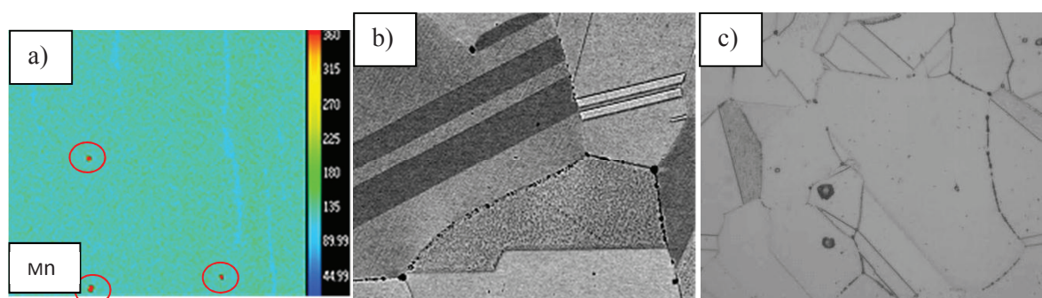
Figure II.1: (a) microsonde de Castaing : sulfures de manganèse, (b) et (c) MEB en électrons rétrodiffusés et microscopie optique : précipités aux joints de grains (carbures de chrome supposés)
