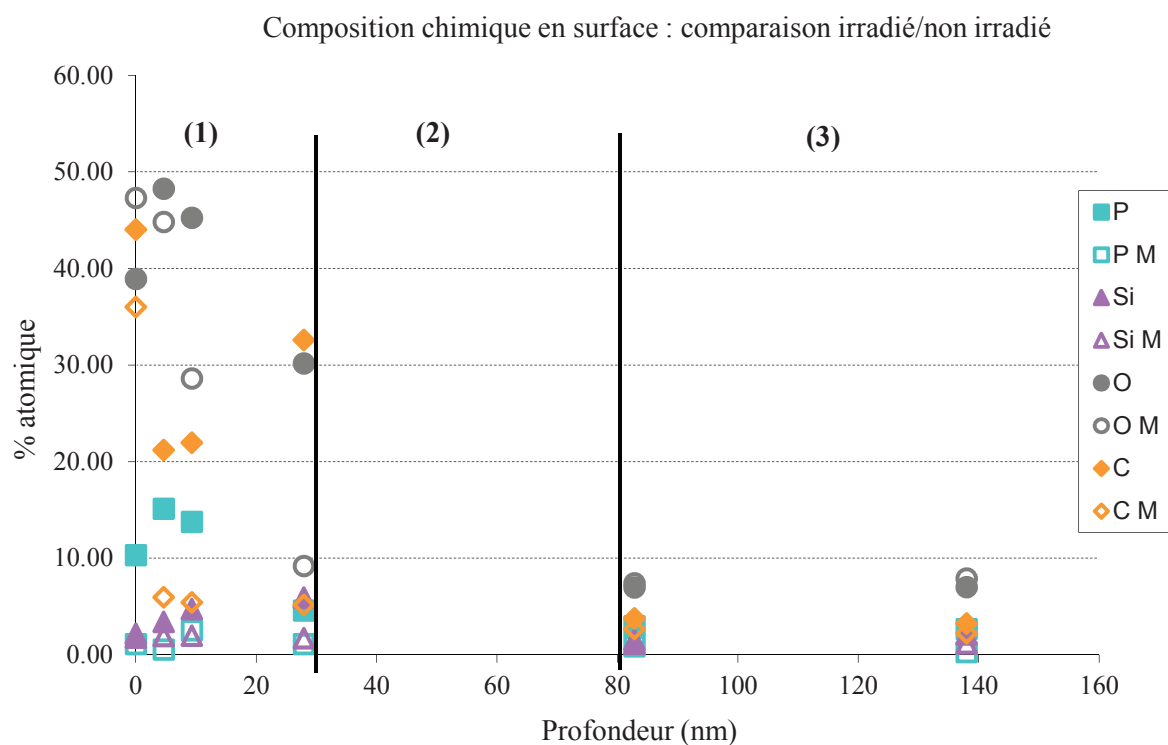
Figure II.12 : Analyses XPS de 0 à 140 nm des éléments minoritaires et impuretés du 304L avec M =matériau non irradié
