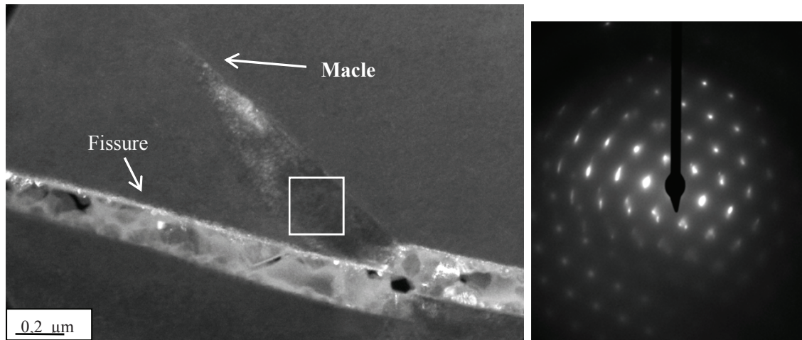
Figure IV.19 : (a) Micrographie en fond noir au niveau de l'intersection entre une macle et la fissure, élargissement de la bande de déformation, (b) cliché de diffraction en axe de zone \langle 110 \rangle au niveau de l'élargissement – rotation du réseau cristallin de l'ordre de 12^\circ
