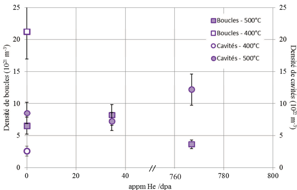
Figure II.35 : Densité de boucles et de cavités en fonction du taux d'hélium implanté et de la température d'irradiation à 2 dpa
