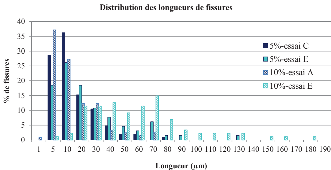
Figure III.26: Distributions des longueurs de fissures à 5 dpa pour 5 et 10% de déformation sous chargement interrompu (éprouvette E) et monotone (éprouvettes A et C)
