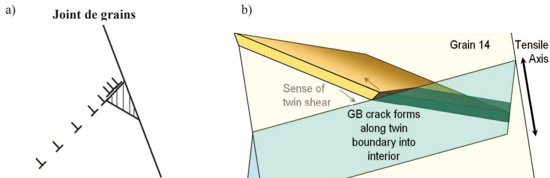
Figure IV.28: (a) Formation d'une microfissure à l'intersection canal / joint de grains du fait de la contrainte générée par l'empilement des dislocations selon le mécanisme dit de Zener-Stroh ; (b) Formation d'une microcavité à l'intersection macle / joint de grain [Bieler 2006]
