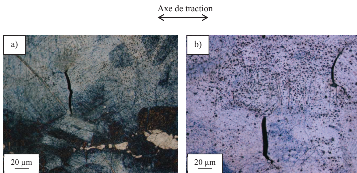
Figure III.8 : Exemples d'images de microscopie optique utilisées pour déterminer la SER du matériau: (a) éprouvette A, 5 dpa, 10% de déformation, (b) éprouvette B, 10 dpa, 10% de déformation
