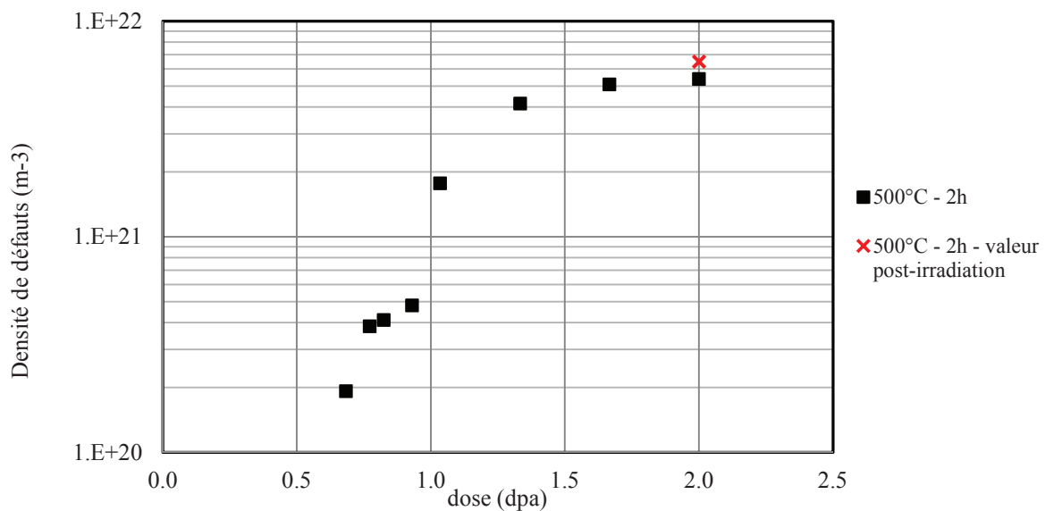
Figure II.29 : Evolution de la densité de boucles visibles en fonction de la dose, au cours d'une irradiation aux ions Ni+ jusqu'à 2 dpa à 500°C
