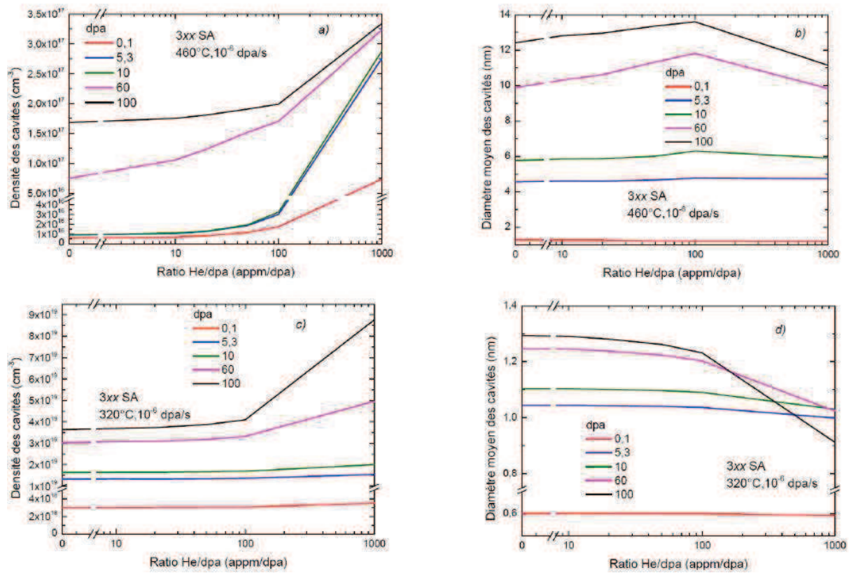
Figure II.39 : Prédiction du modèle en termes d'évolution avec le rapport He/dpa, entre 0 et 1000 appm/dpa, de la densité (a, c) et de la taille moyenne des cavités (b,d) pour un acier de type 3xx SA irradié avec un débit de dose de 10^{-6} \text{ dpa.s}^{-1} , à 460^{\circ}\text{C} (a,b) et 320^{\circ}\text{C} (c,d) [Zouari 2012]
