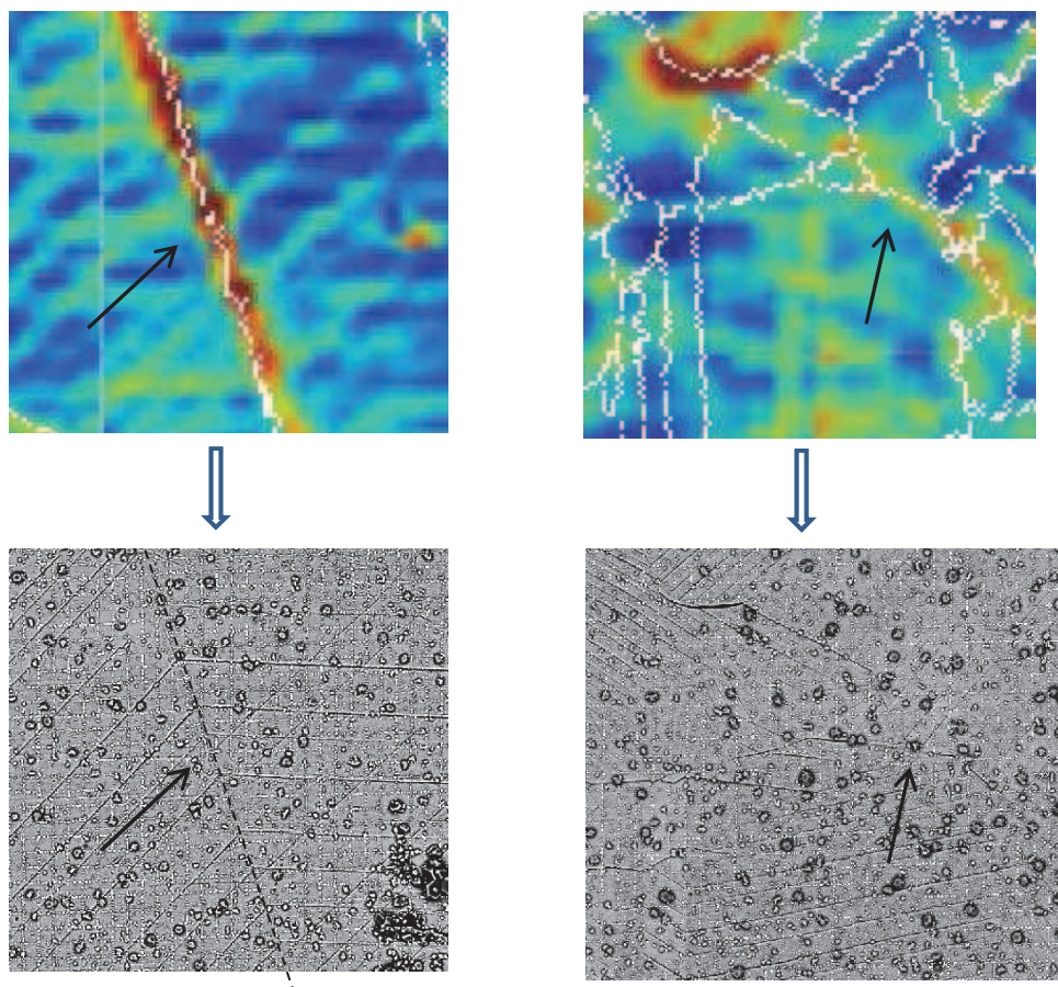
Figure III.41 : Exemples de joints fortement déformés mais non fissurés et champs de déformation associés.
