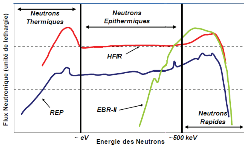
Figure I.4 : Spectre de fission en fonction du type de réacteur : en vert les réacteurs à neutrons rapides (RNR), en rouge le réacteur à spectre mixte HFIR et en bleu les REP [Zouari 2012]
