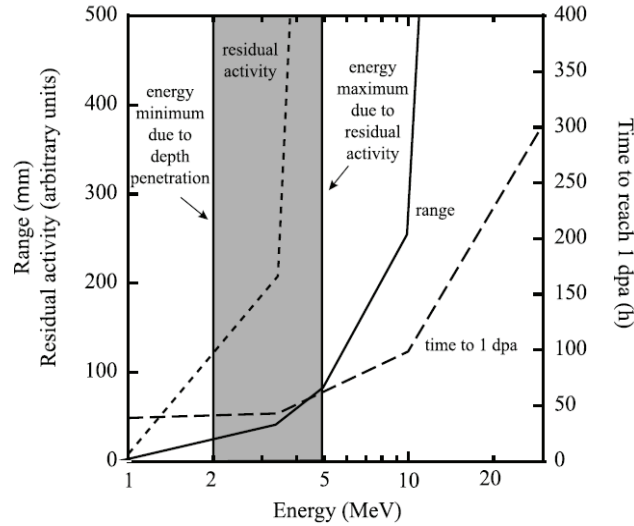
Figure I.21: Evolution de la profondeur, de l'activité résiduelle et du temps nécessaire pour atteindre 1dpa en fonction de l'énergie des protons [Was 2007a]
