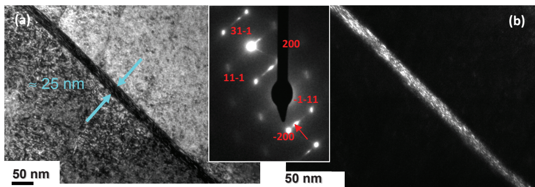
Figure IV.15 : Bande de déformation du système S1 - micrographie MET et cliché de diffraction associé (a) fond clair (b) fond noir réalisé sur la traînée de diffusion indiquée par une flèche rouge.
