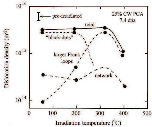
Figure I.6: Effet de la température d'irradiation sur la densité de dislocations d'un acier austénitique inoxydable irradié aux neutrons [Zinkle 1993].
