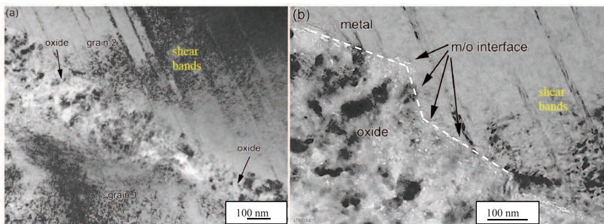
Figure IV.18: Micrographies MET (fond clair) d'une fissure sur un acier 316CW (vis) irradié à 8,5 dpa en milieu REP – (a) vue générale avec présence de nombreuses bandes de cisaillement interagissant avec les flancs de la fissure, (b) interface bandes de cisaillement et flancs de fissure, création d'une marche [Bruemmer 2006]
