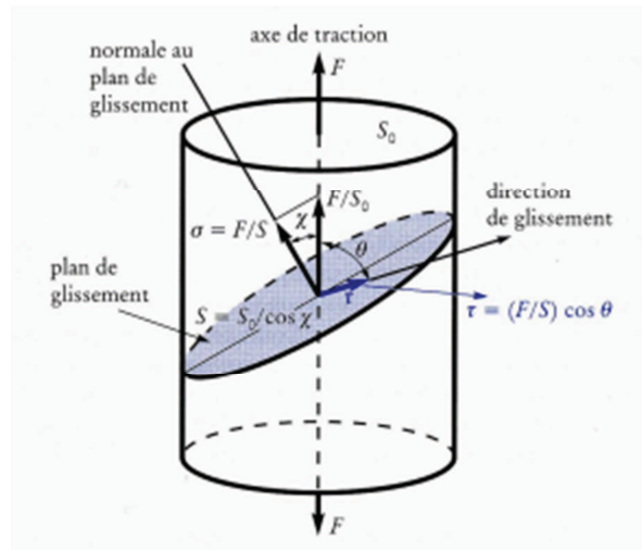
Figure III.32: Représentation schématisée de la loi de Schmid [Schmid 1950]
