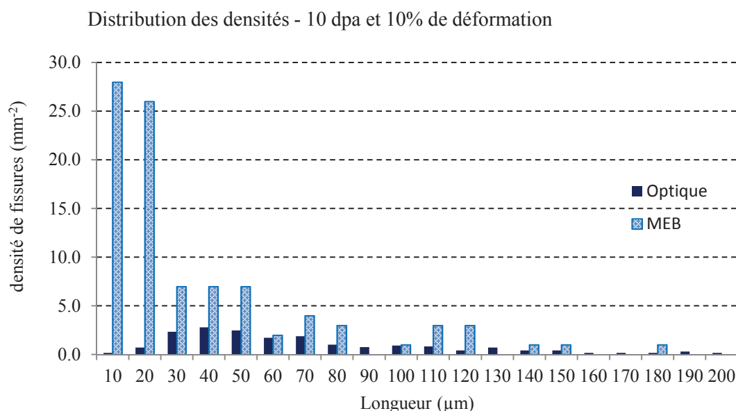
Figure III.13 : Distribution des densités de fissures détectées par longueur sur l'éprouvette B en fonction de l'outil de détection
