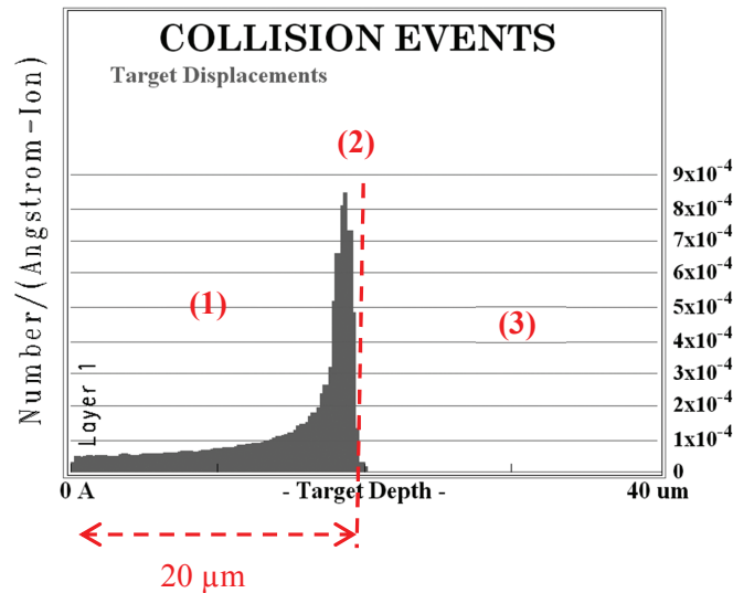
Figure II.5 : Profil d'endommagement d'un acier 304L calculé avec le logiciel SRIM pour des protons de 2 MeV
