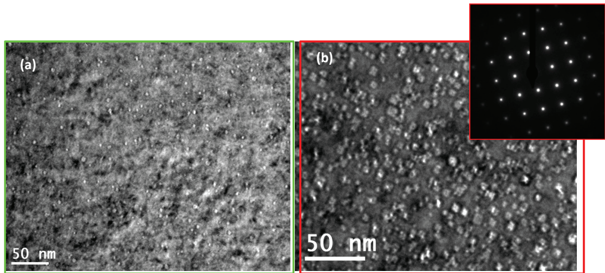
Figure II.19 : Cavités imagées (a) sous-focalisation, zone irradiée (0) sur le plateau de dommages et (b) sur-focalisation, pic de Bragg, zone irradiée (1) – cliché de diffraction, axe de zone \langle 001 \rangle
