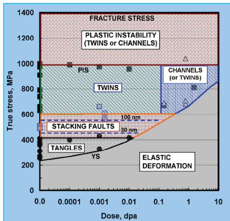
Figure IV.2: Carte des modes de déformation en fonction de la contrainte vraie et de la dose des aciers inoxydables austénitiques [Byun 2006]
