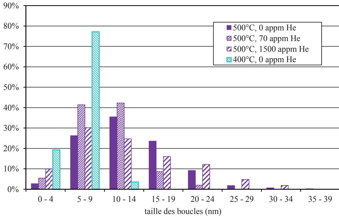
Figure II.36 : Distribution de la taille des boucles en fonction de la température et de la quantité d'hélium implanté à 2 dpa
