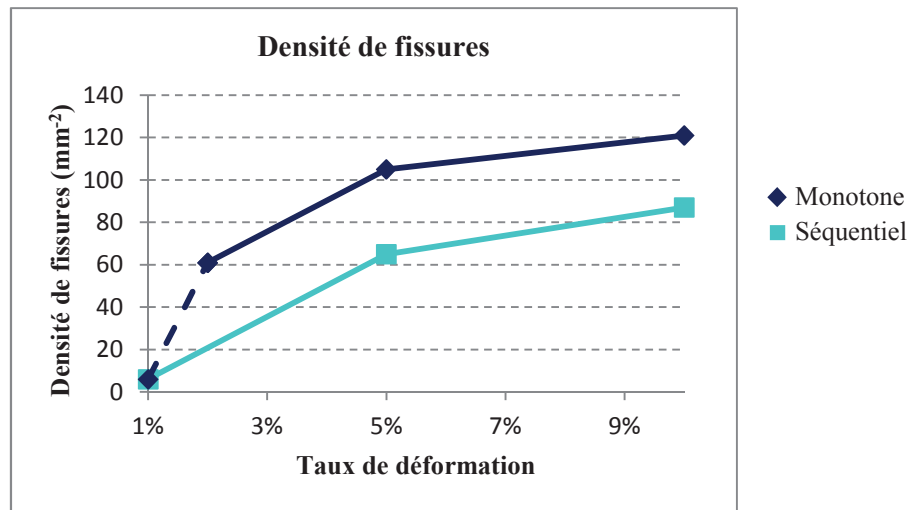
Figure III.24: Evolution de la densité de fissures avec le taux de déformation en fonction du trajet de chargement (acier 304L irradié à 5 dpa)
