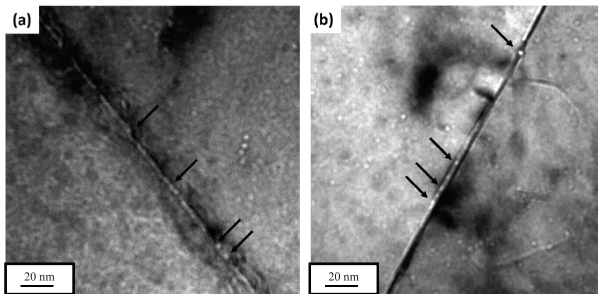
Figure II.34: Micrographies MET en fond clair sous-focalisées révélant la présence de cavités aux joints de grains (flèches noires) avec (a) joint général et 0 appm He et (b) joint \Sigma 3 et 70 appm He
