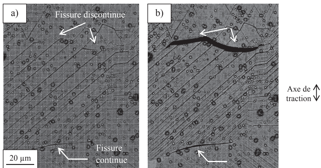
Figure III.18 : (a) Eprouvette E après 5% de déformation, (b) même zone après 10% de déformation
