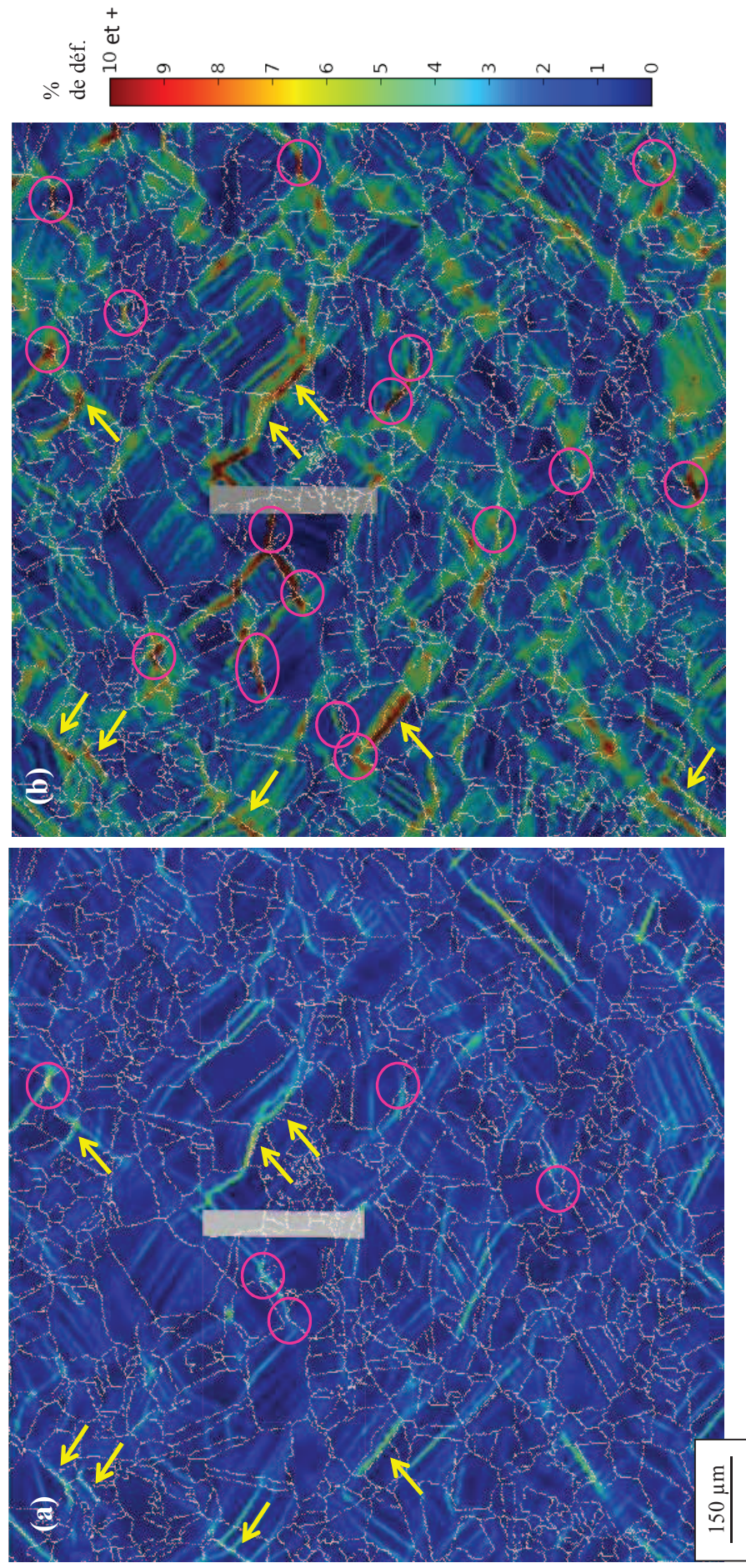
Figure III.52: Déformation équivalente de Von Mises sur la zone irradiée (a) après 1% et (b) après 5% - les cercles roses signalent les principales fissures et les flèches jaunes les joints déformés mais non fissurés
