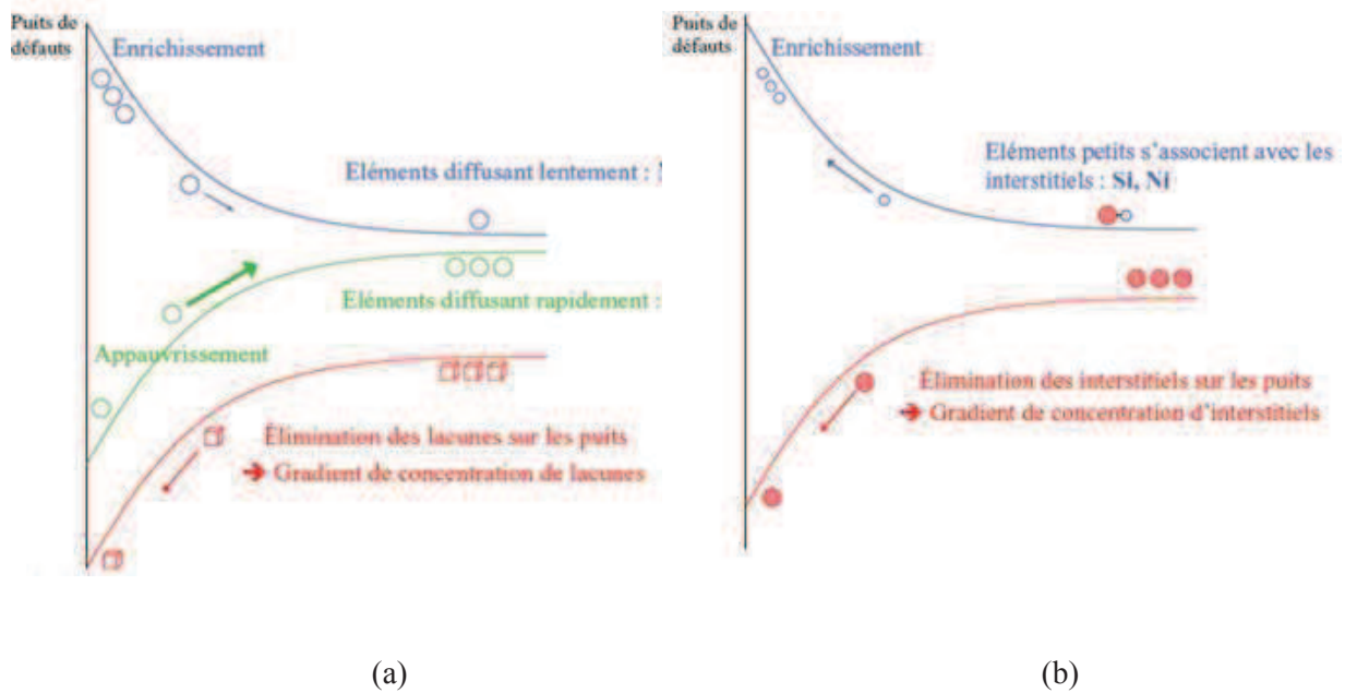
Figure I.12: Mécanismes envisagés dans le cas de la ségrégation induite par l'irradiation (RIS) d'après [Bruemmer 1999] et [Etienne 2009], (a) Kirkendall inverse et (b) association d'interstitiels
