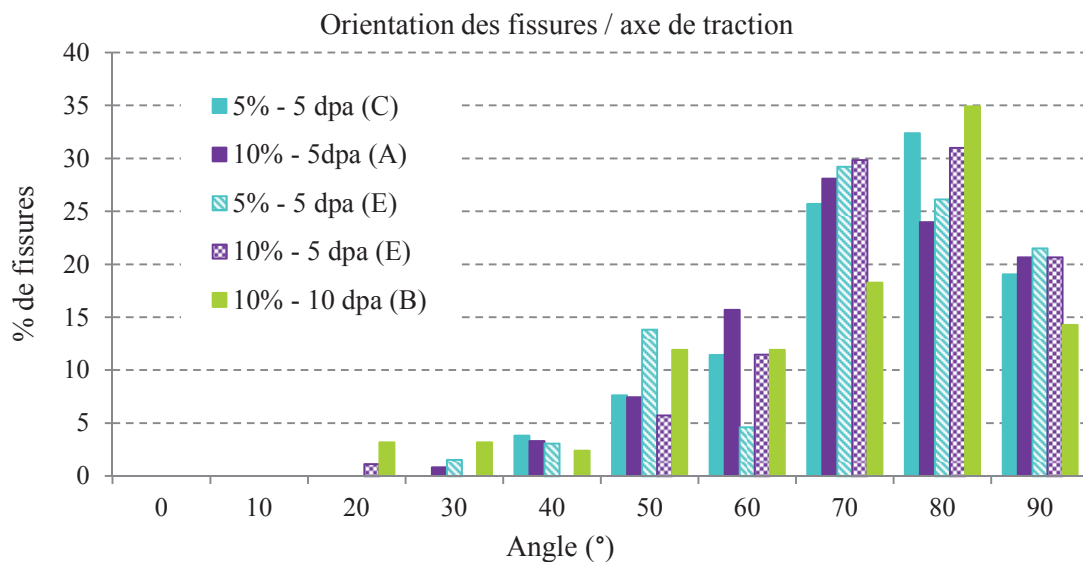
Figure III.19: Distribution des inclinaisons des fissures par rapport à l'axe de traction pour les essais A et C (monotone, 5 dpa), B (monotone, 10 dpa) et E (séquentiel, 5 dpa)
