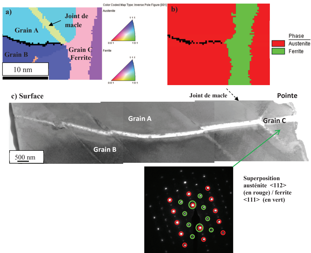
Figure IV.8 : Présentation générale de la fissure A, (a) figure de pôles inverses et (b) identification de phase par EBSD réalisée en coupe transverse, (c) micrographies MET en fond clair et cliché de diffraction obtenu dans la zone indiquée par la flèche verte
