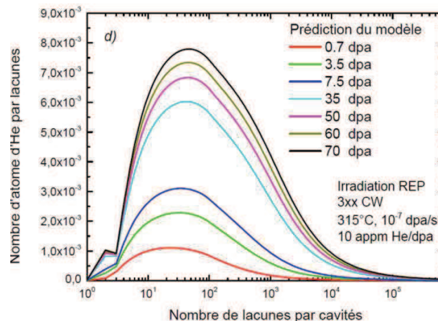
Figure II.41 : Evolution avec la dose du nombre d'atomes d'He par lacune dans un acier inoxydable austénitique écroui irradié en conditions REP [Zouari 2012]
