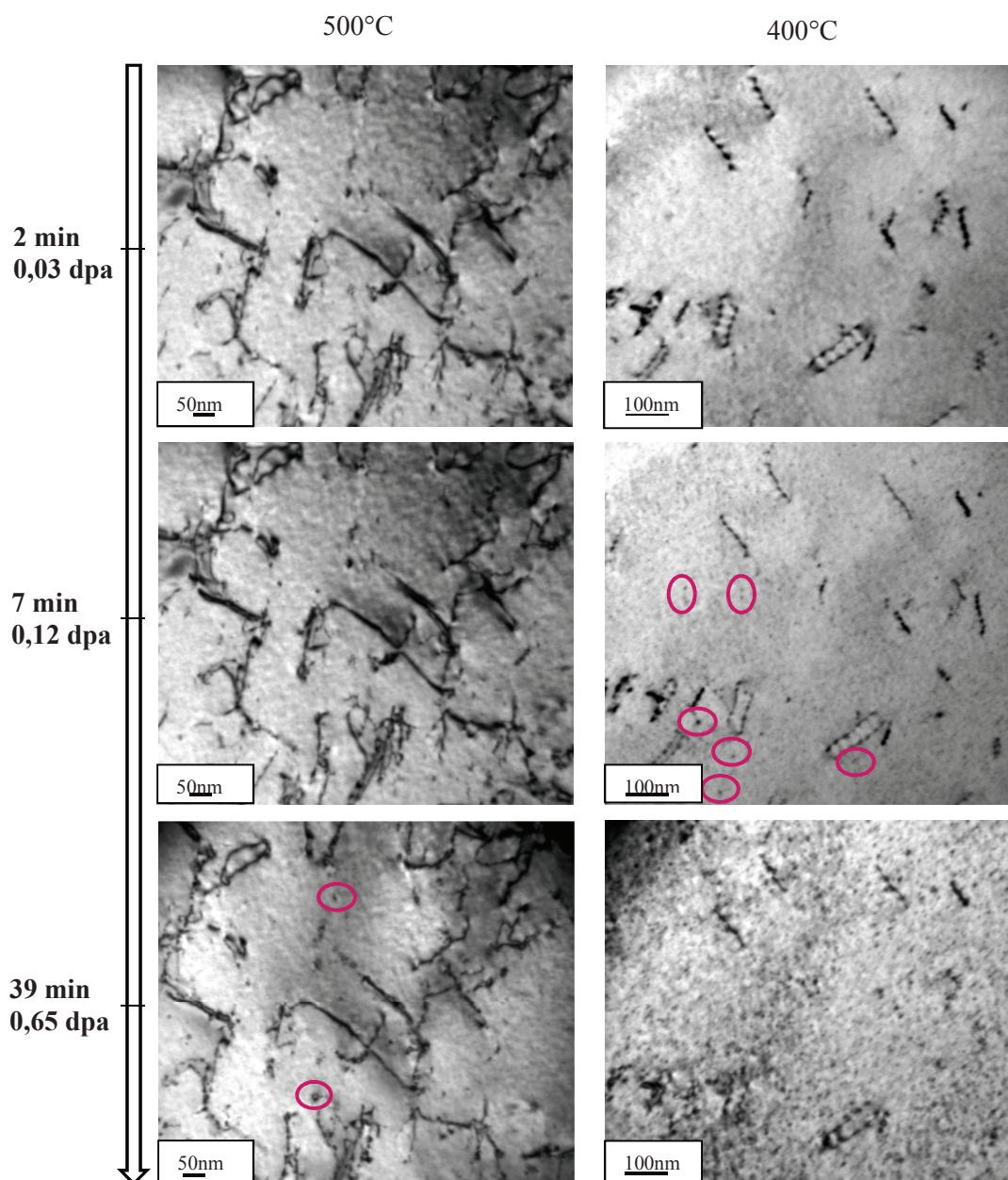
Figure II.28 : Evolution de la microstructure de 0 à 0,65 dpa à 500°C et 400°C en cours d'irradiation Ni++ 500 keV - en rose, les premiers défauts (non exhaustif).
