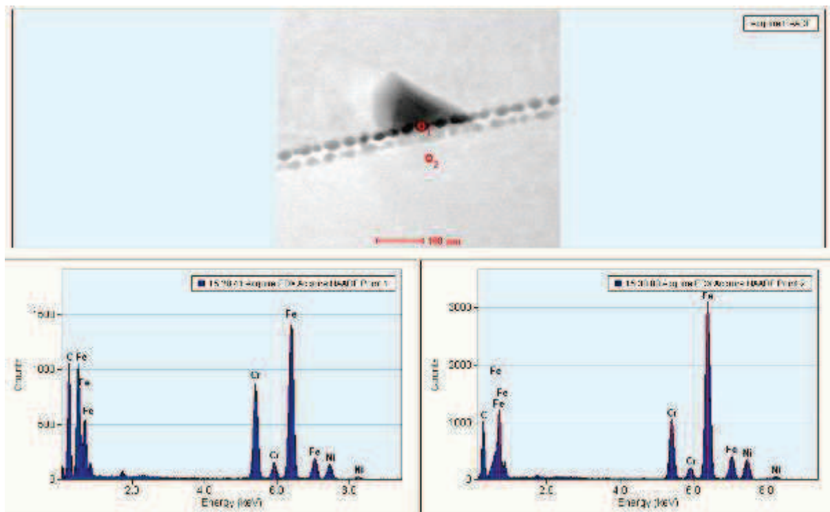
Figure D.3 : Micrographie en STEM-HAADF d'un joint de grains après traitement thermique in situ à 500°C pendant 2h d'une lame après recuit à 1050°C et analyses EDX : comparaison entre la matrice (point 2) et le précipité (point 1). Il s'agit d'un carbure de chrome.
