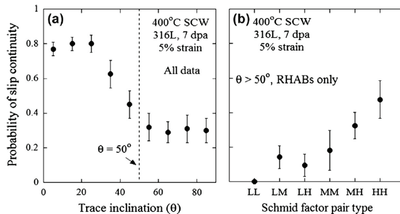
Figure IV.26 : Probabilité de continuité de la déformation en fonction (a) de l'inclinaison du joint de grains et (b) du facteur de Schmid des grains adjacents [West 2013]
