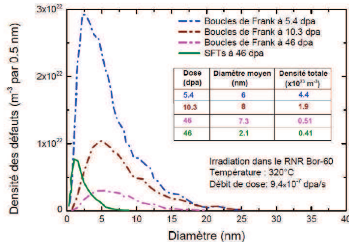
Figure I.11: Distributions des boucles de Frank (traits pointillés) et des SFTs (traits pleins) dans un 304L irradié dans le RNR Bor-60 à 320°C et 9,4 \cdot 10^{-7} \text{ dpa.s}^{-1} à 5, 10 et 46 dpa [Fournier 2012, d'après Zouari 2012]
