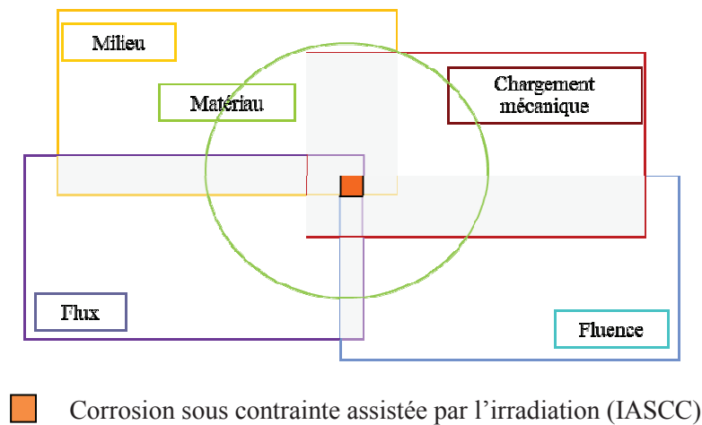
Figure 2 : Diagramme de Venn des mécanismes d'endommagement faisant intervenir simultanément l'action de plusieurs facteurs [CEA 2010]
