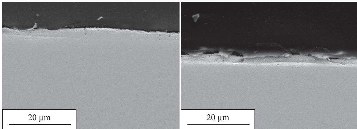
Figure III.29 : Observations MEB en coupe transverse de la zone non irradiée de l'éprouvette C, après 5% de déformation macroscopique. Aucune fissure n'est visible en volume sur la zone non irradiée.
