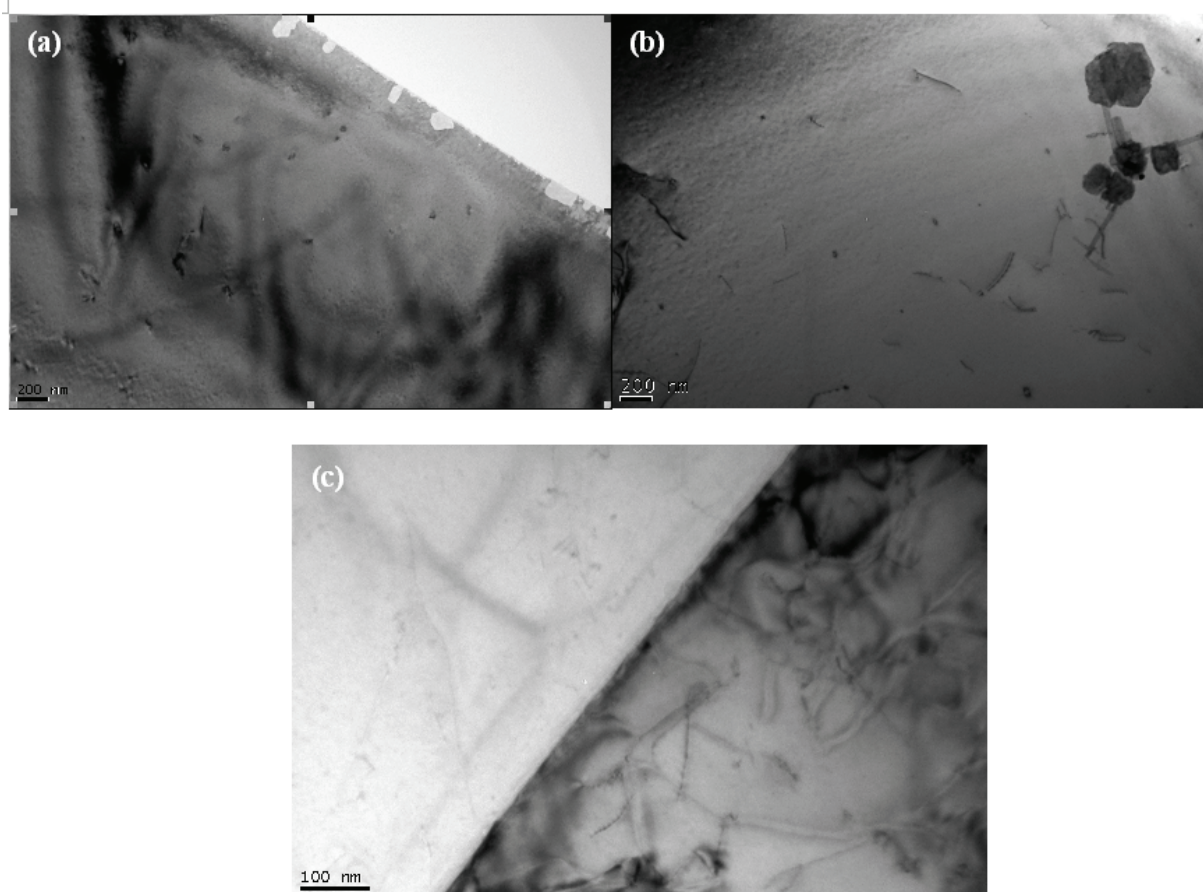
Figure D.4 : Micrographies en fond clair après traitement thermique à 500°C pendant 2h30 d'une lame « en l'état de réception », (a) et (b) présence de précipités en bord de lame et (c) joint de grain, pas de carbures de chrome
