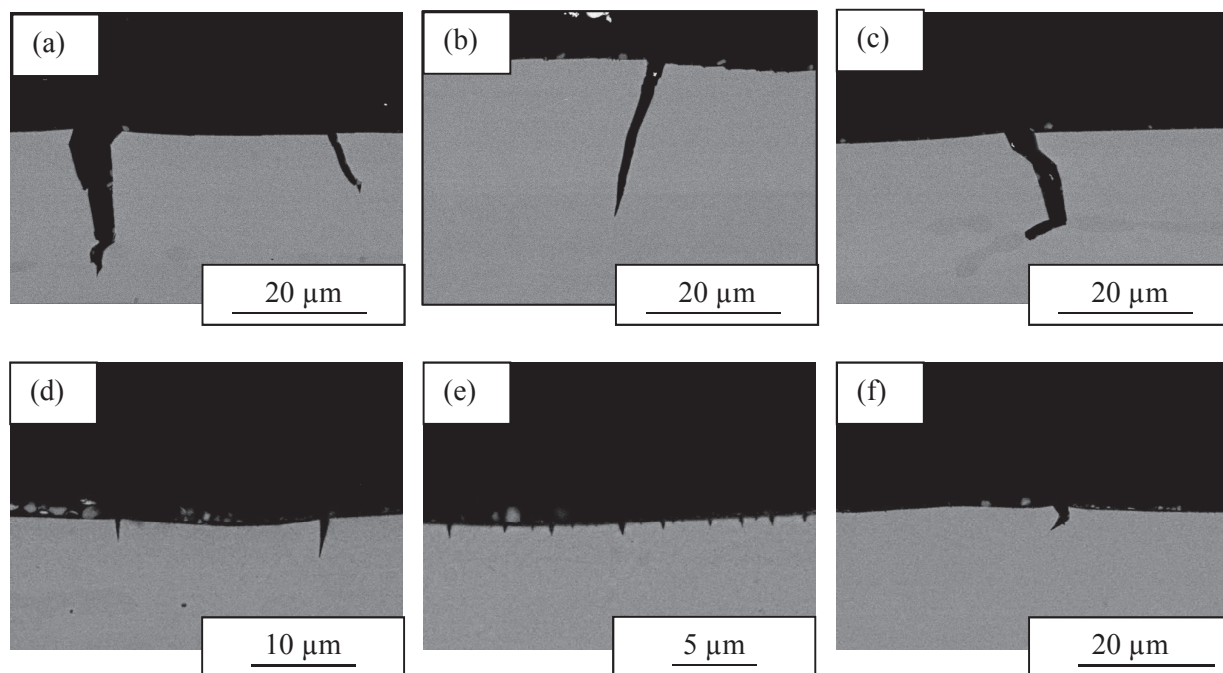
Figure III.31 : Images MEB en coupe de l'éprouvette E après 10% de déformation (a, b et c) pour la zone irradiée, (d, e et f) pour la partie non irradiée
