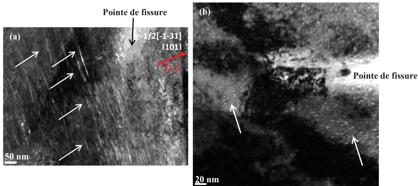
Figure IV.7 : Pointe de la fissure D (a) Micrographie en fond noir d'une famille de boucles de Frank (b) micrographie en fond clair sous-focalisée des cavités
