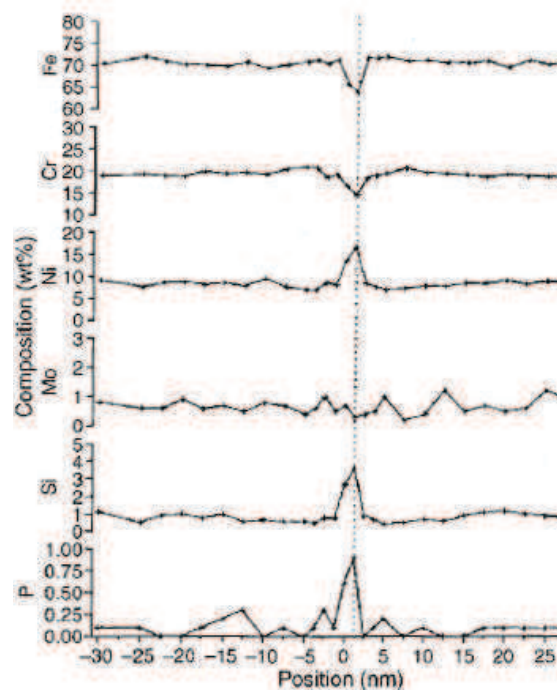
Figure I.13 : Profil de composition obtenu sur un acier de type 304 après irradiation aux neutrons à 275°C [Was 2007b]
