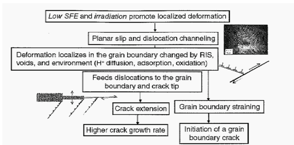
Figure IV.23 : Schéma du mécanisme proposé par Hojna [Hojna 2013] pour expliquer la fissuration par IASCC, modifié d'après le mécanisme proposé par Was [Was 2003]
