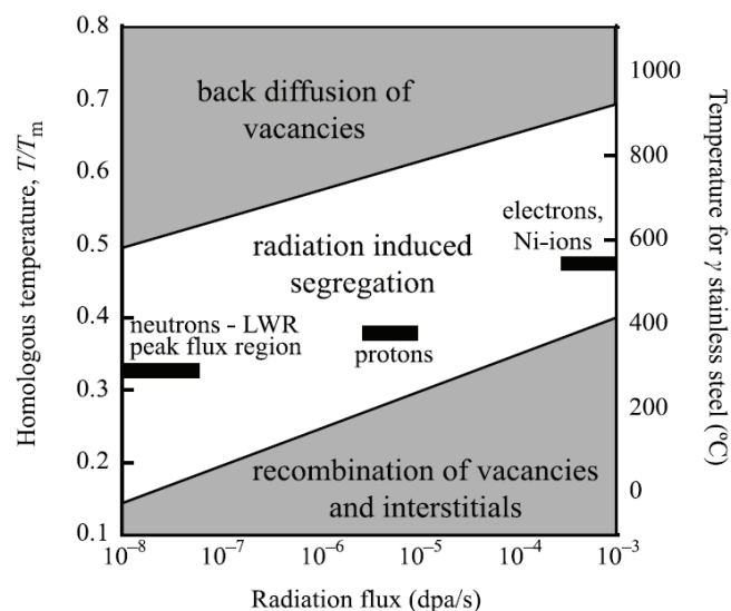
Figure I.20 : Prédiction des effets de la température d'irradiation et du débit de dose sur la ségrégation induite par l'irradiation [Brummer 1999, Was 2007a]
