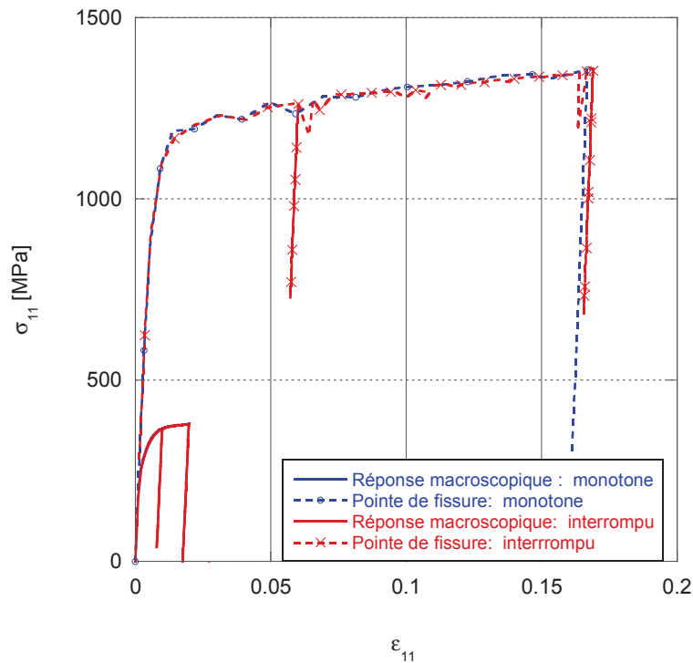
Figure IV.33 : Courbes contrainte –déformation en pointe de fissure pour 2% de déformation macroscopique imposée par traction monotone (pointillés bleus) ou en séquentiel 1% puis 2% (pointillés rouges) pour la profondeur d’entaille « mi-épaisseur » (M), en trait plein la réponse macroscopique de la structure pour les deux types de chargement
