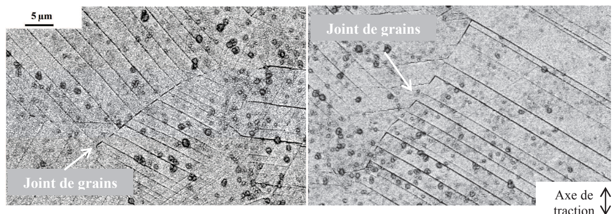
Figure III.16 : Exemples d'ouvertures discontinues présentes en surface de l'éprouvette A (5 dpa) après 10% de déformation en milieu primaire REP
