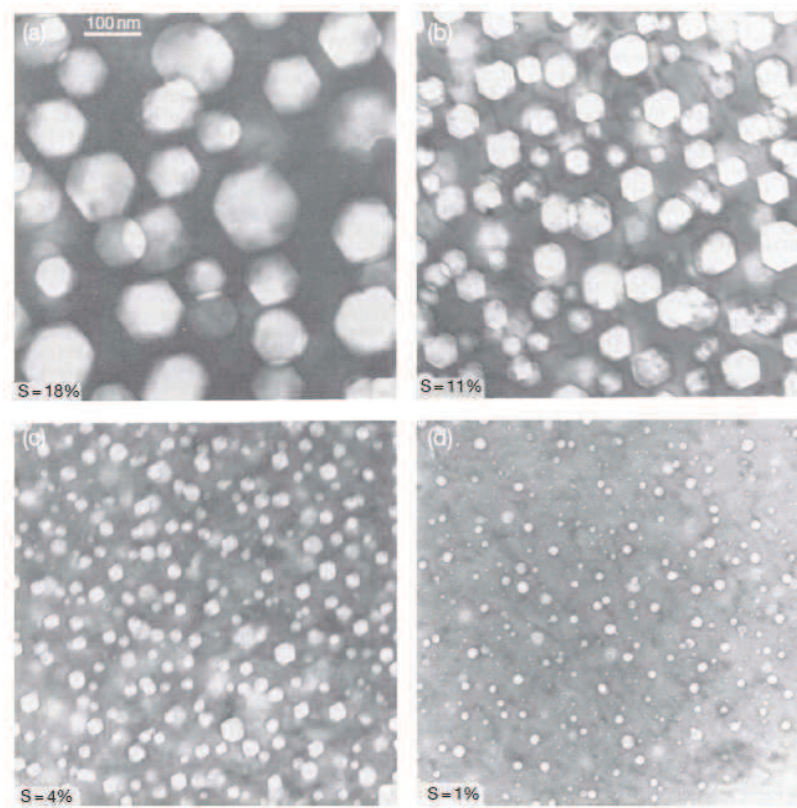
Figure II.38 : Morphologies des cavités observées sur un alliage Fe-Ni-Cr irradié à 70 dpa et 625°C avec (a) 0 appm d'He, (b) 1400 appm d'He co-implanté, (c) 1400 appm d'He pré-injecté à chaud et (d) 1400 d'He pré-implanté à froid [Packan 1979, d'après Dai 2012]
