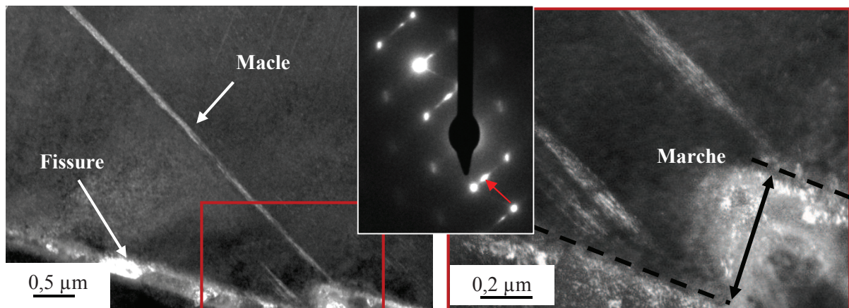
Figure IV.17 : Fond noir sur la traînée de diffusion – Intersection entre les macles du système primaire et la fissure A, formation d'une marche
