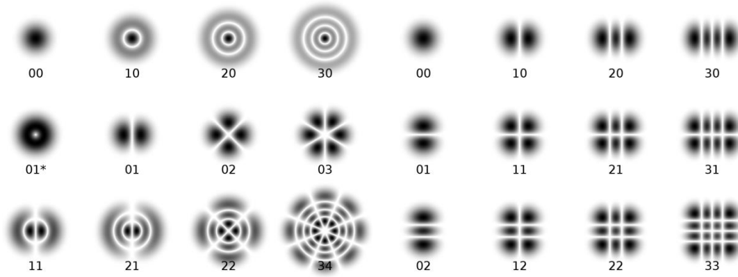
Figure 2.12 – Empreinte laser pour différents modes transverses.
