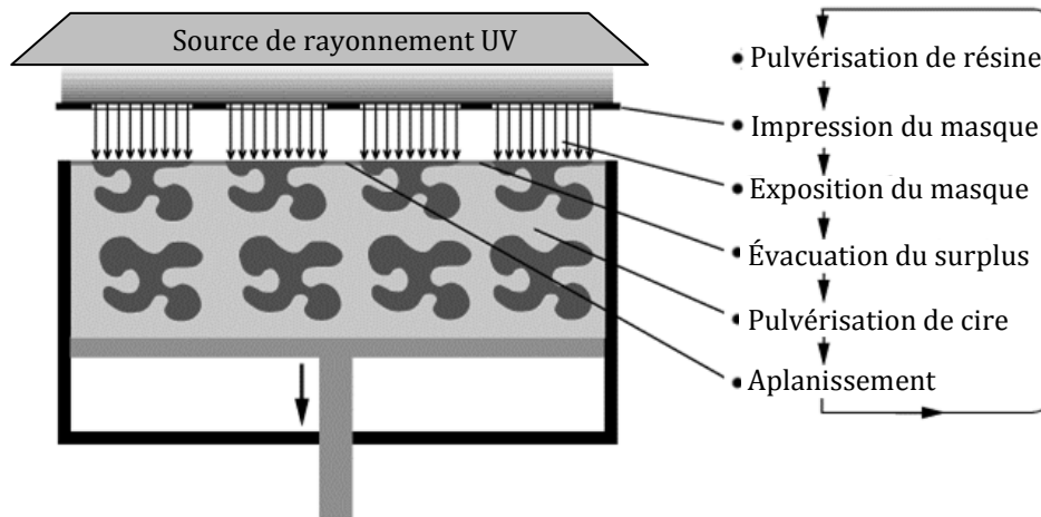
Figure 1.3 – Schéma descriptif du procédé de flashage. Traduction de l'auteur.
