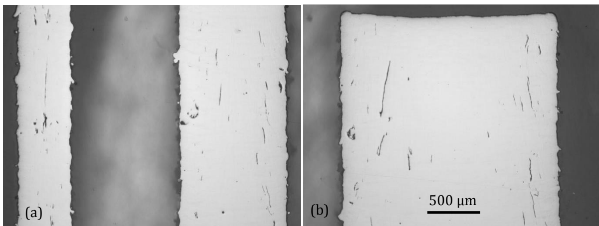
Figure 5.34 – Micrographies de l'échantillon brut de fabrication SLM fabriqué avec une épaisseur de couche de 30 µm représentant (a) les murs de 500 µm et de 1 mm d'épaisseur, (b) le mur de 2 mm d'épaisseur. L'échelle s'applique aux deux micrographies.
