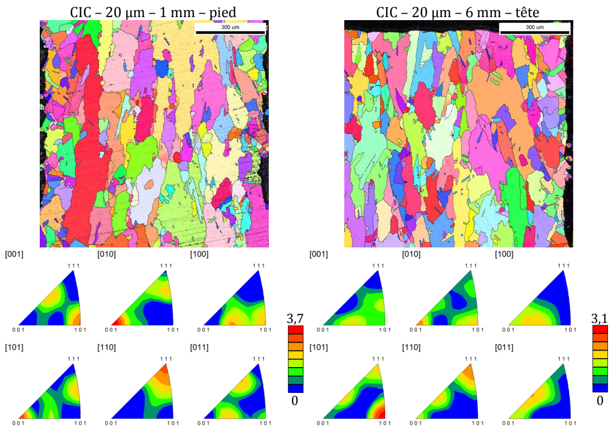
Figure 5.47 – Cartographies EBSD des murs de 1 mm de large produits par SLM en Inconel 738 avec une épaisseur de couche de 20 μm après traitement de compaction isostatique à chaud à 1200 °C. L’indexation des couleurs est identique à celle de la Figure 5.43, toujours selon [100]. Toutes les figures sont à la même échelle, et la barre représente 300 μm. Les figures de pôle inverse associées aux microstructures sont placées en dessous.
