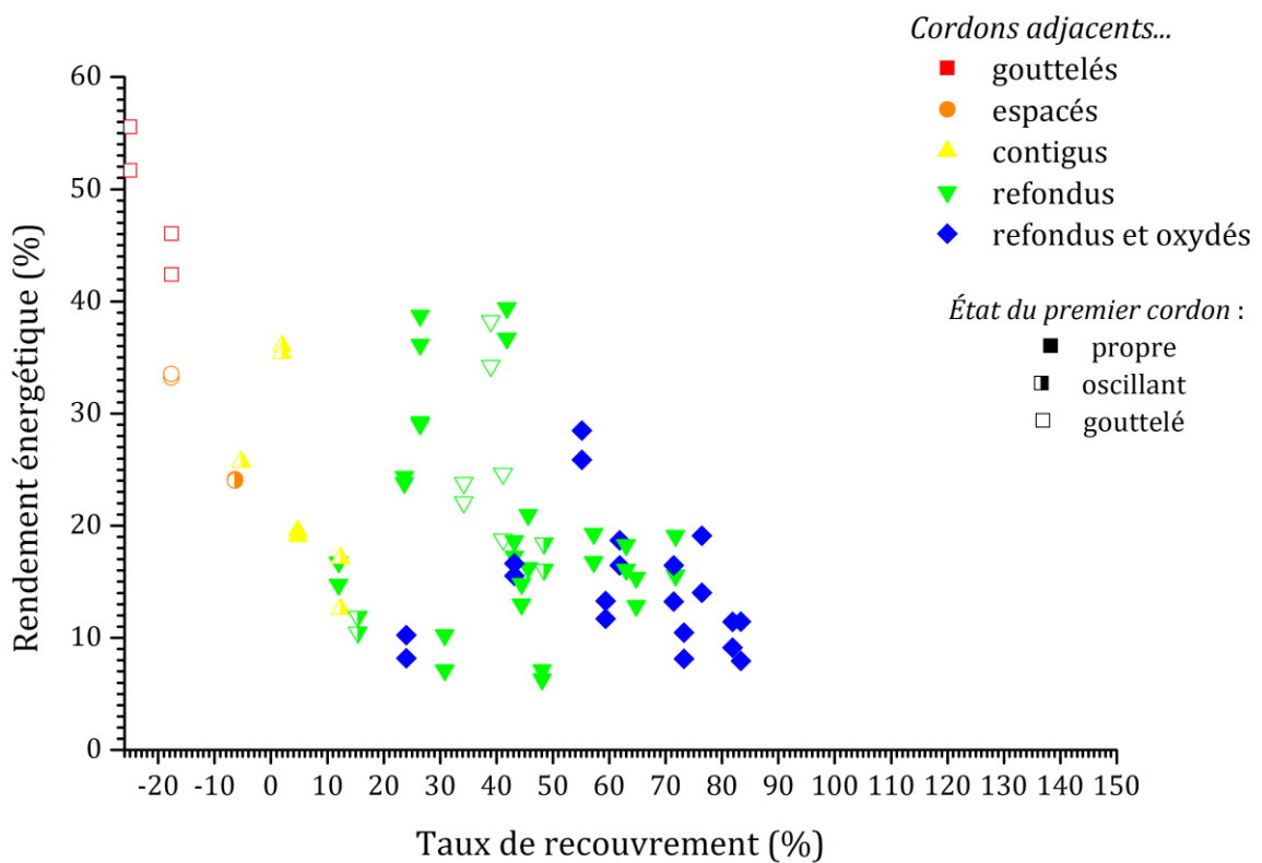
Figure 3.43 – Évolution du rendement énergétique pour les surfaces fabriquées en fonction du taux de recouvrement.
