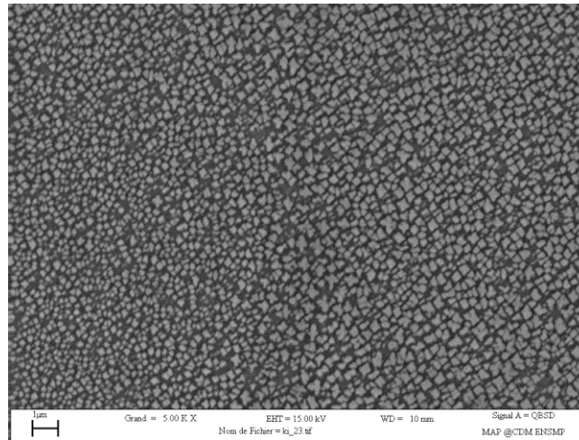
Figure 5.4 – Microstructure de l'Inconel 738 révélée par une attaque électrolytique dans \{0,5 \text{ g CuSO}_4 + 50 \text{ ml H}_2\text{O}\} à 5 V pendant 10 secondes. L'image MEB en mode BSE montre les différentes morphologies que peuvent présenter les précipités \gamma dans l'alliage brut de fonderie. La barre d'échelle indique 1 \mu\text{m} .
