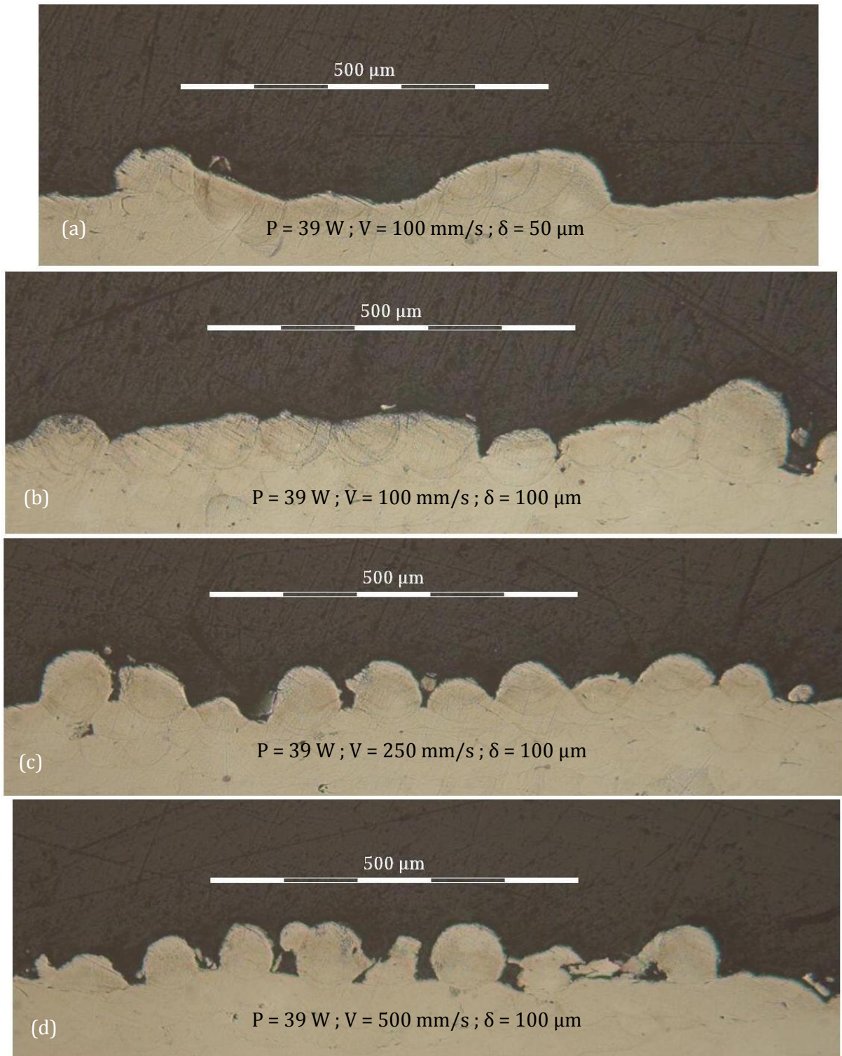
Figure 3.32 – Micrographie de certaines surfaces vues en coupe illustrant des cordons (a) refondus, (b) contigus, (c) espacés et (d) goutté. Tous les exemples proviennent des essais avec une puissance de 39 W.
