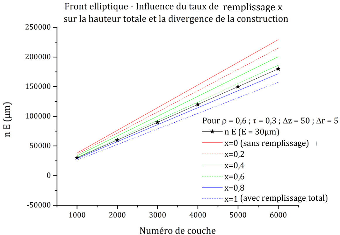
Figure 2.29 – Influence du taux de remplissage x sur la hauteur totale de la construction dans le modèle elliptique
