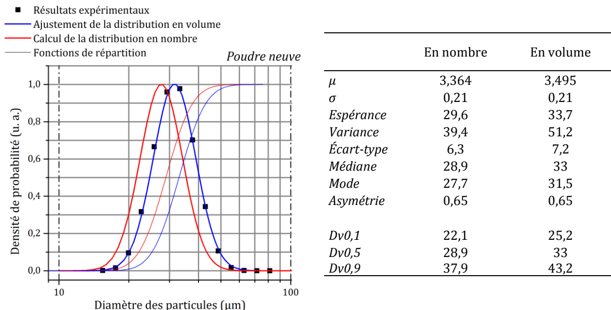
Figure 5.27 – Distribution granulométrique de la poudre d'Inconel 738 mesurée par granulométrie laser et tableau regroupant les différentes caractéristiques statistiques de la distribution granulométrique de l'Inconel 738.
