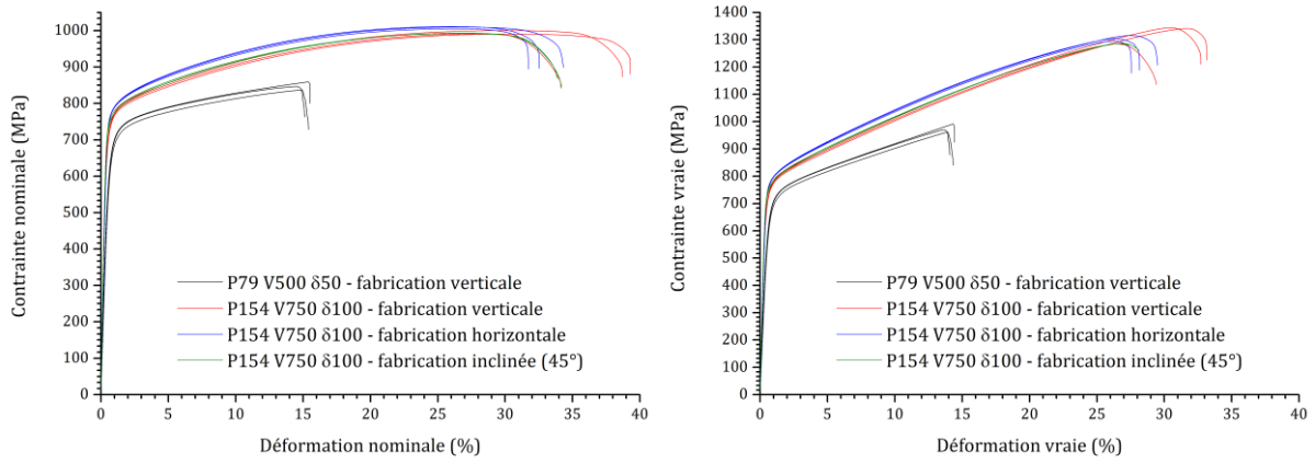
Figure 4.30 - Courbes de traction nominale et de traction vraie pour les éprouvettes fabriquées avec les paramètres de M1 (P154_V750_δ100) et de M2 (P79_V500_δ50) et pour les différents sens de fabrication.
