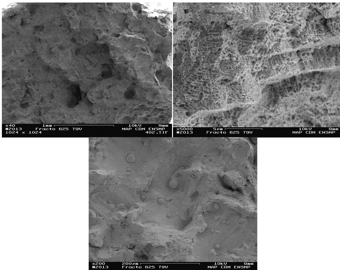
Figure 4.31 - Micrographie électronique du faciès de rupture d'une éprouvette verticale produite avec les paramètres M2 (P79_V500_δ50).
