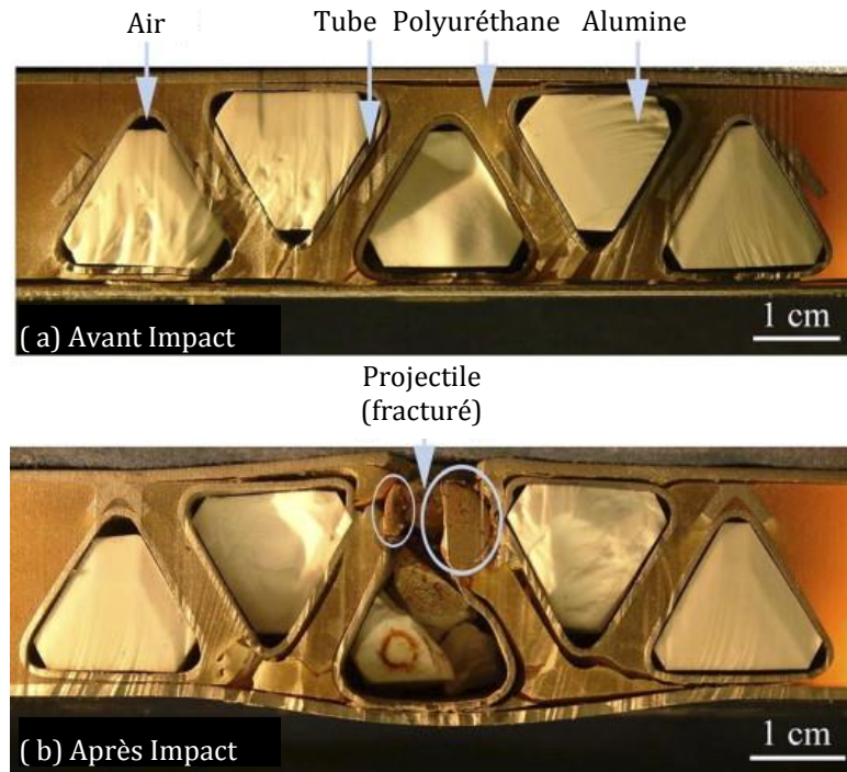
Figure 4.4 – (a) Vue en coupe de la structure pyramidale à un étage possédant des tubes à section triangulaire entourés de polyuréthane et contenant un insert en alumine, (b) vue en coupe de la structure après essai d’impact à 613 m/s. [YUN08]
