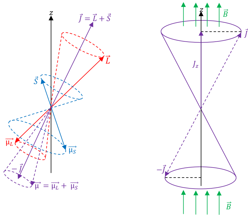
Figure A.6 – Représentation géométrique de l'effet Zeeman pour un spin -1/2 . (a) le moment magnétique total \vec{\mu} précesse autour du moment cinétique total \vec{J} , (b) \vec{J} précesse plus lentement autour du champ magnétique. Reproduit d'après [TEL13]
