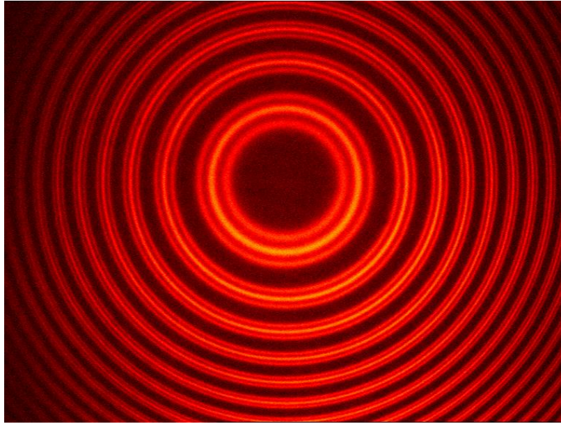
Figure A.8 – Effet Zeeman sur les anneaux d'égal inclinaison de la raie rouge du Cadmium à 6438 Å sous un champ de 280 mT, après passage dans un interféromètre de Fabry-Pérot. [MOU11]
