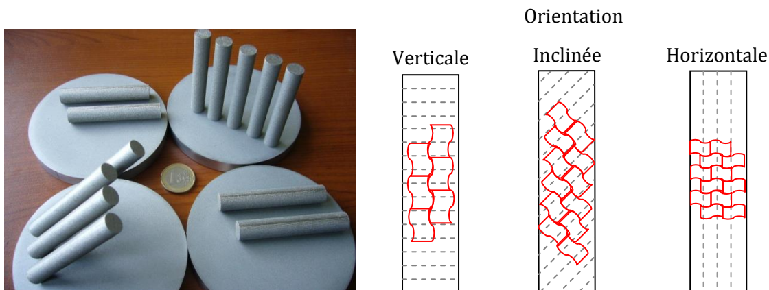
Figure 4.29 - Photographie des éprouvettes de traction après construction et représentation de l'arrangement des couches (en pointillé) et des grains (en traits continus) au sein des éprouvettes pendant l'essai de traction.
