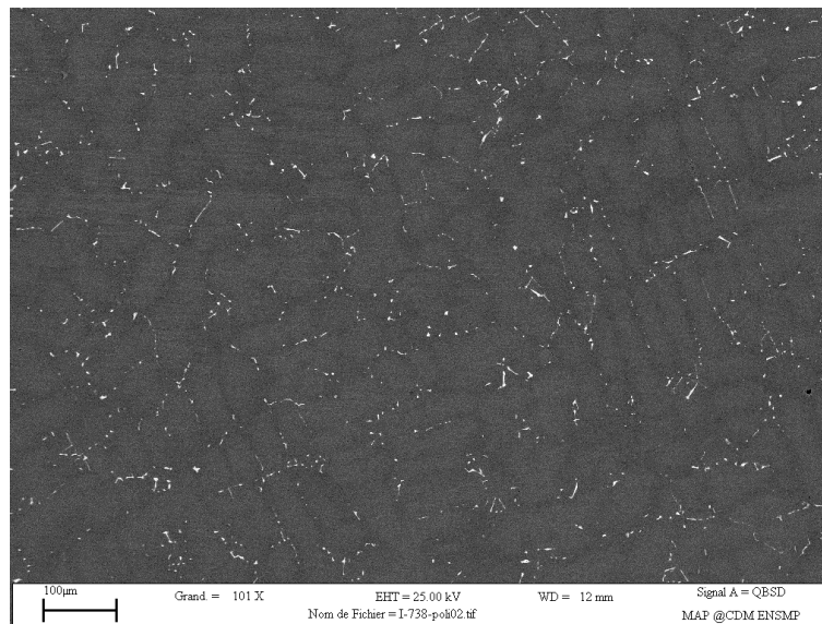
Figure 5.7 – Microstructure de l'Inconel 738 brut de fonderie. La photographie MEB, prise en électrons rétrodiffusés, présente une population de carbures, en blanc. Ces carbures, de type MC, se situent dans une large majorité au niveau du liseré gris foncé qui caractérise les zones inter-dendritiques. Les bras de dendrites, qui apparaissent en gris clair, semblent en être dépourvus. Au passage, de petits points noirs sont visibles, trahissant la présence de pores. L'échantillon a été observé suite à un polissage sans attaque.
