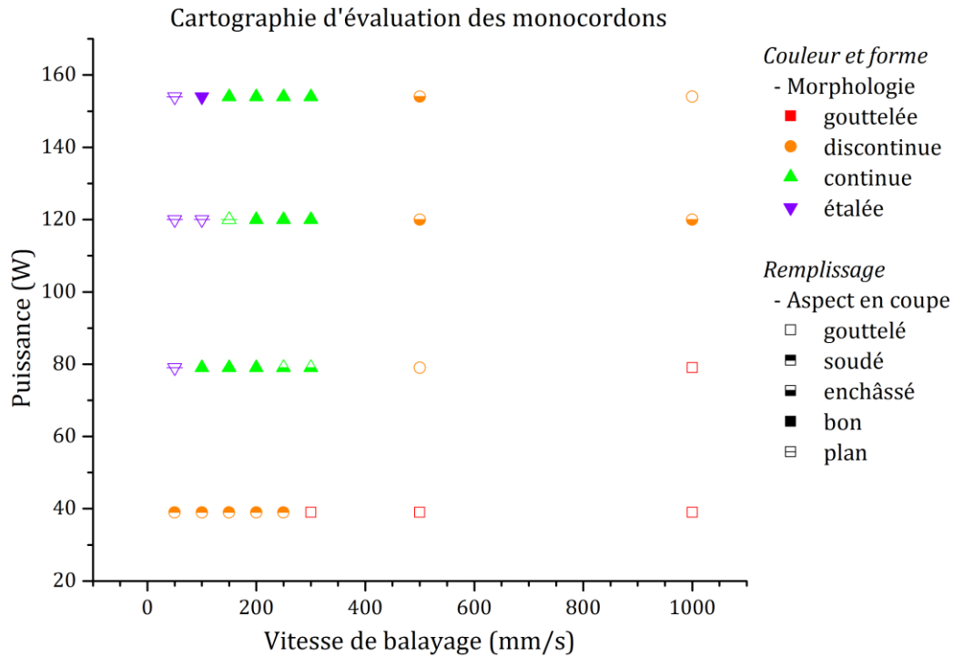
Figure 3.17 – Cartographie d'évaluation des cordons en fonction de la puissance et de la vitesse de balayage du faisceau laser sur le lit de poudre. L'évaluation est faite à la fois à partir de la morphologie extérieure des cordons et de leur aspect en section droite.
