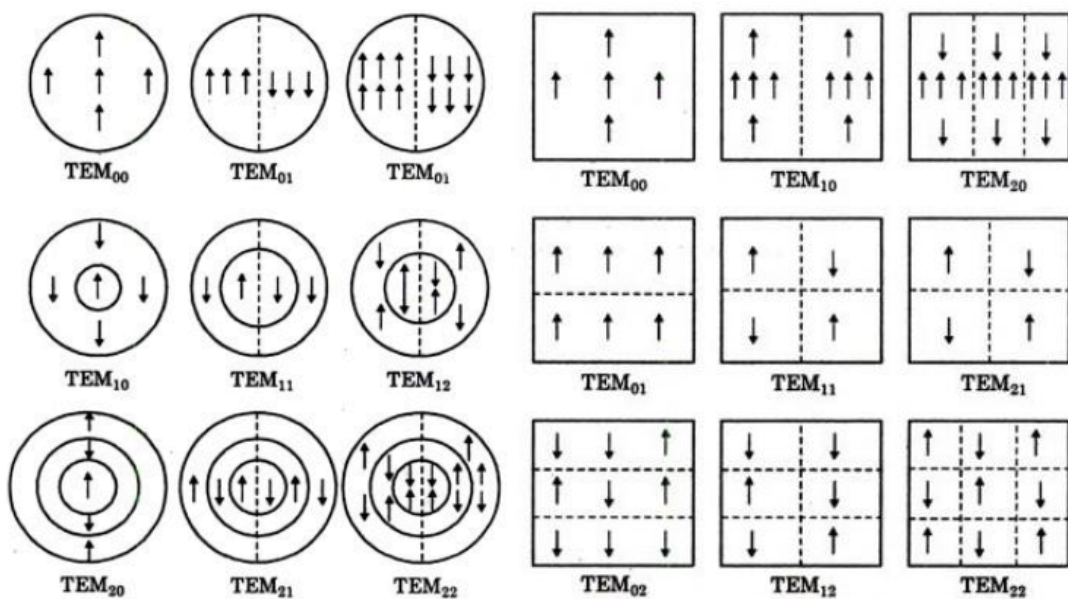
Figure 2.14 – Configuration de la polarisation linéaire pour différents modes. [GUP04]
