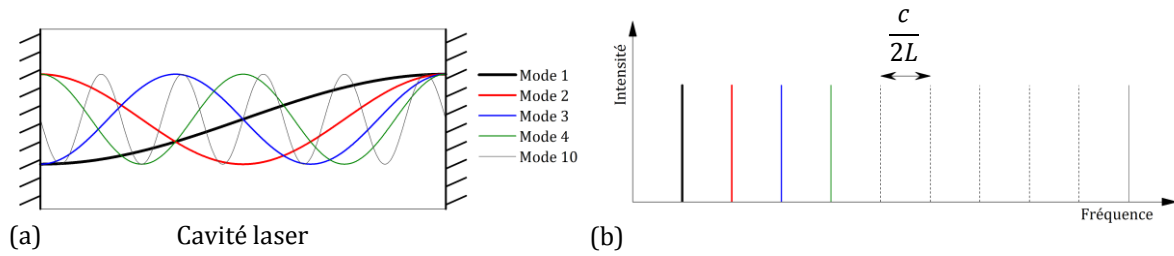
Figure 2.1 – (a) Représentation temporelle des premiers modes longitudinaux pouvant perdurer dans la cavité laser. Pour simplifier la représentation, la cavité est fermée par deux miroirs plans. En fait, une telle configuration ne permet pas de garantir la stabilité de l'oscillation laser. (b) Spectre fréquentiel de la cavité.
