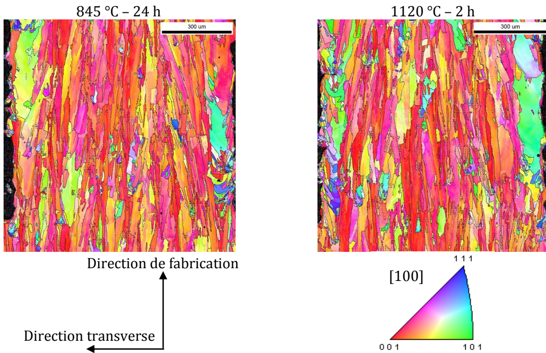
Figure 5.46 – Cartographies EBSD des murs de 1 mm d’épaisseur produits par SLM en Inconel 738 pour le mur de 1 mm de large produit avec une épaisseur de couche de 20 μm, après traitements thermiques à 845 °C et 1120 °C. L’indexation des couleurs est identique à celle de la Figure 5.43, toujours selon [100]. Toutes les figures sont à la même échelle, et la barre représente 300 μm.
