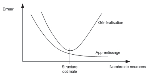
Figure 30 : Détermination de la structure optimale
