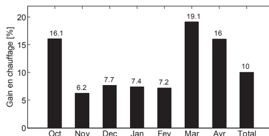
Figure 96 : Gains en chauffage selon le mois avec le régulateur ANN.
