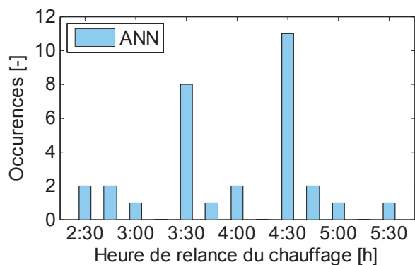
Figure 67 : Différentes heures de relance optimale déterminées par le régulateur ANN sur le mois.
