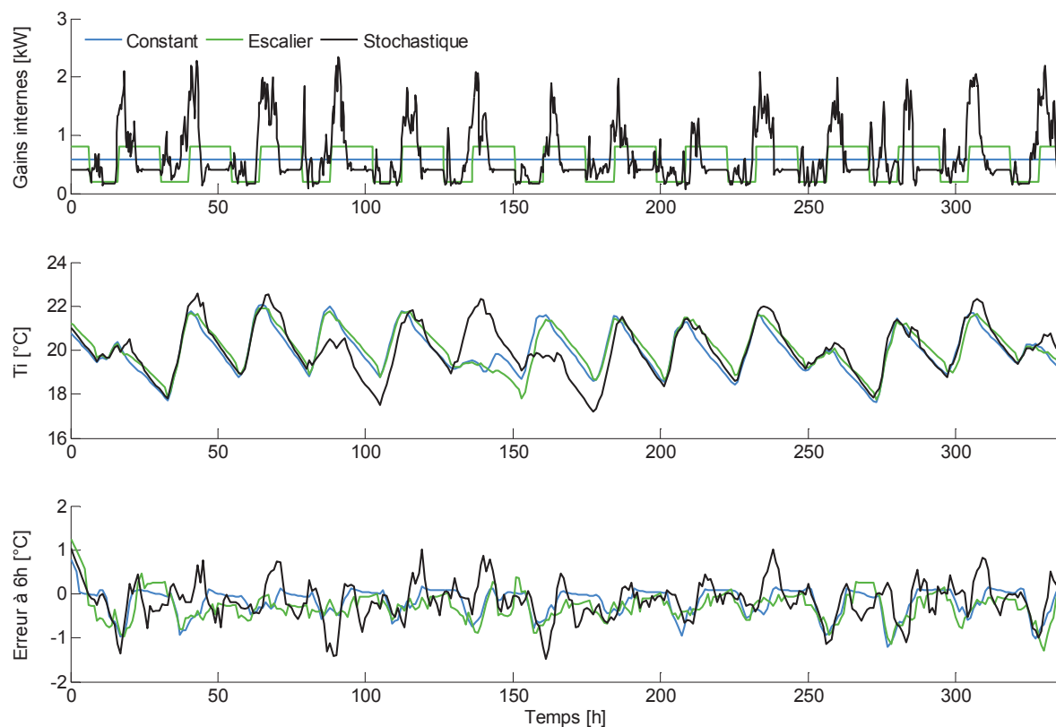
Figure 54: Résultats de prévision à 6 h de la température ambiante sur une journée en fonction du type de gains internes.
