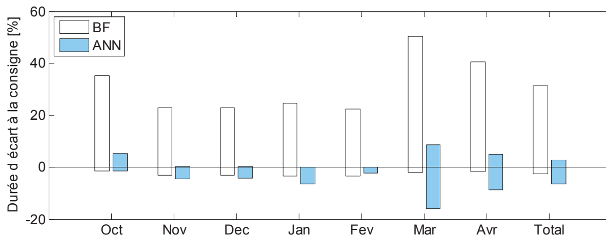
Figure 94: Ecart à la consigne en pourcentage de temps par mois et sur la saison de chauffage. Les valeurs positives correspondent aux périodes où T_i > 22.5\text{ °C} , les valeurs négatives à T_i < 21.5\text{ °C} .
