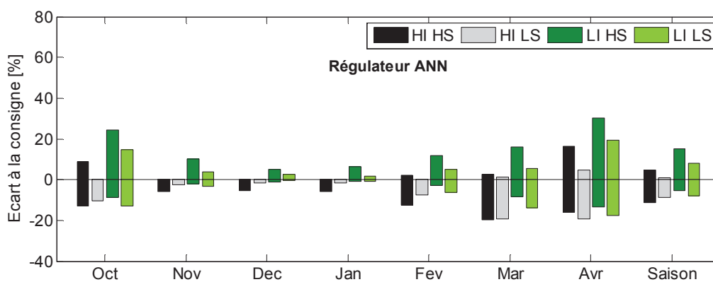
Figure 80 : Pourcentage d'heures d'écarts à la consigne selon le type de bâtiment. Régulateur ANN.
