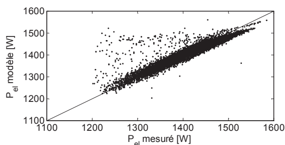
Figure 90 : Comparaison entre puissance compresseur P_{\text{el}} modèle et mesuré
