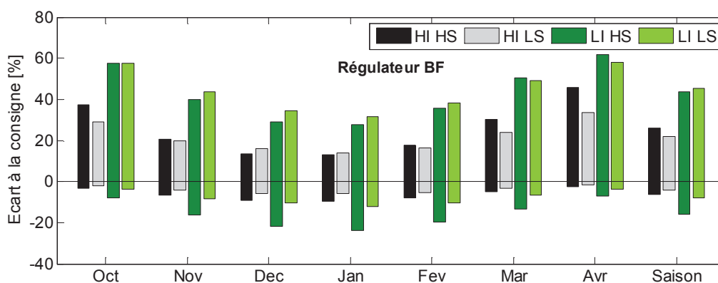
Figure 79 : Pourcentage d'heures d'écart à la consigne selon le type de bâtiment. Régulateur BF.
