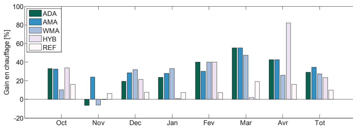
Figure 99: Gains en énergie de chauffage offerts par le régulateur prédictif.
