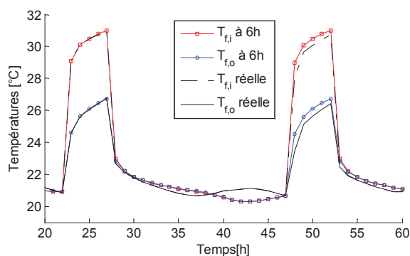
Figure 41 : Prévisions à 6 h du modèle ANN1 des températures entrée et sortie du plancher chauffant.
