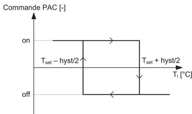
Figure 17: Régulation en boucle fermée sur la température ambiante.
