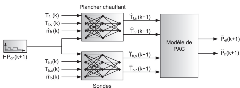
Figure 46 : Couplage des modèles du système de PAC géothermique pour la prévision de la puissance thermique fournie au plancher ( P_n ) et de la puissance électrique consommée ( P_e ).
