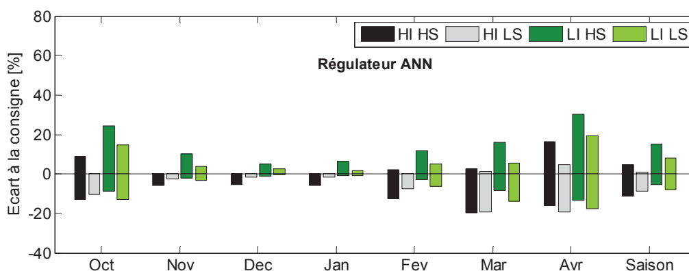
Figure 80 : Pourcentage d'heures d'écart à la consigne selon le type de bâtiment. Régulateur ANN.
