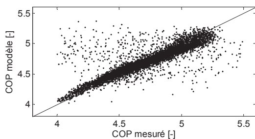
Figure 89 : Comparaison entre COP modèle et COP mesuré
