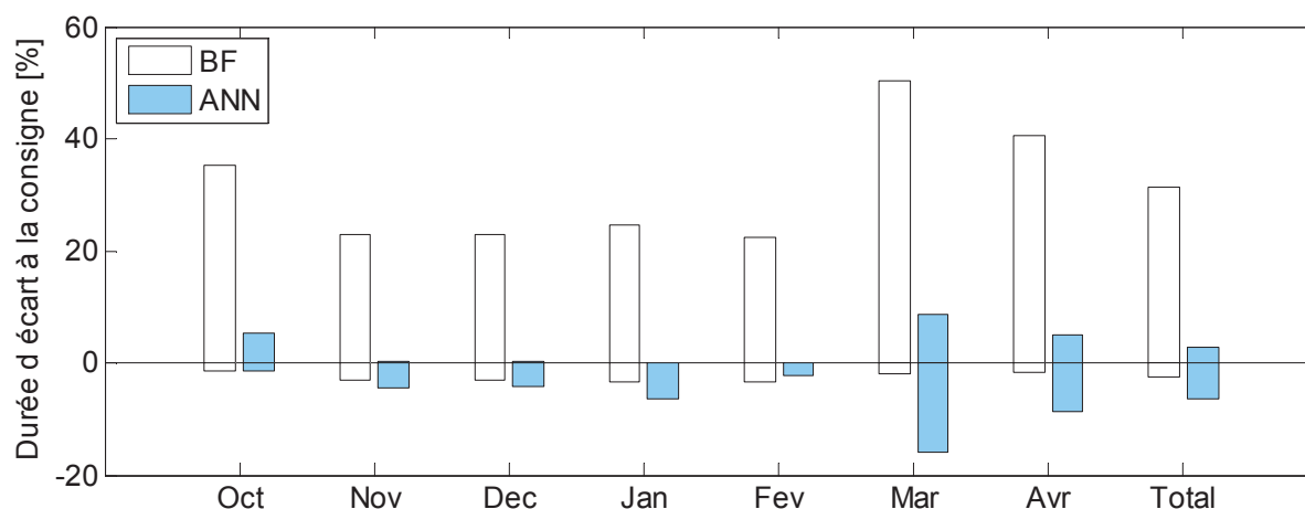
Figure 94: Ecart à la consigne en pourcentage de temps par mois et sur la saison de chauffage. Les valeurs positives correspondent aux périodes où T_i > 22.5\text{ }^\circ\text{C} , les valeurs négatives à T_i < 21.5\text{ }^\circ\text{C} .
