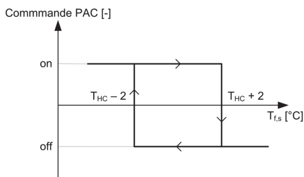
Figure 62 : Régulateur conventionnel BOC de référence.
