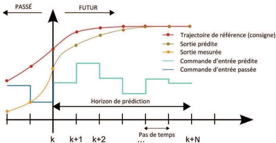
Figure 19: Schéma de principe de la commande prédictive.
