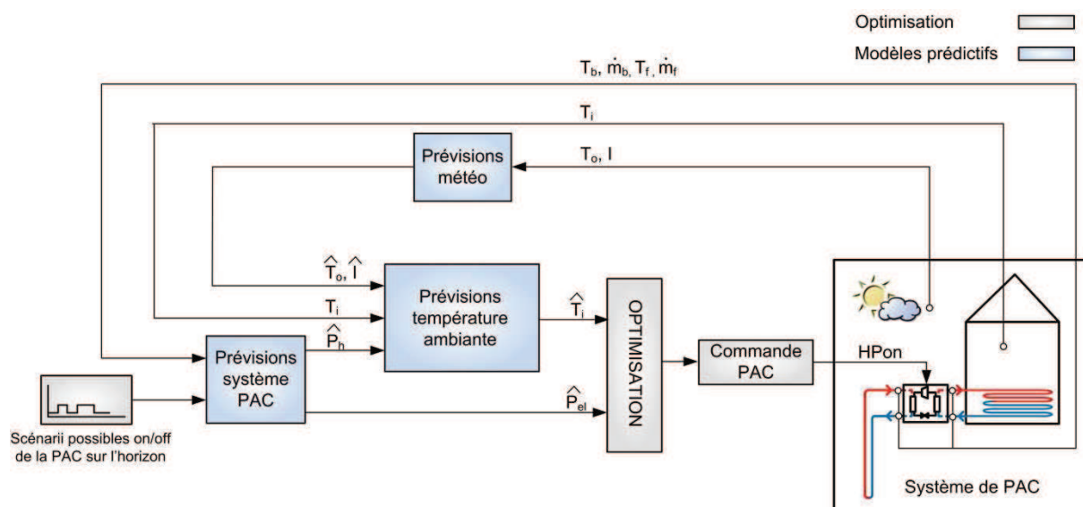
Figure 25: Structure modulaire du régulateur prédictif. Les valeurs prédites sont assignées d'un symbole « \hat{\quad} ».
