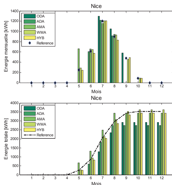
Figure 14 : Energies de refroidissement mensuelles et cumulée - Nice. [5]
