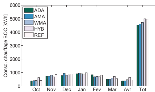
Figure 107 : Consommations en chauffage mensuelles et totale – Régulateur BOC.
