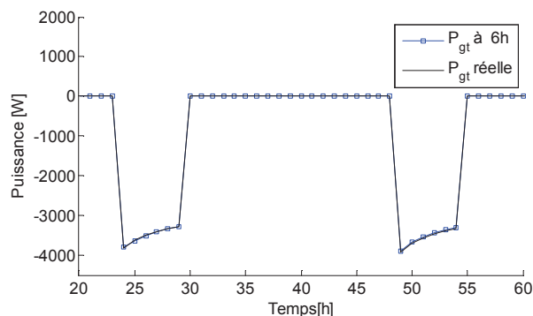
Figure 44 : Prévisions à 6 h du modèle ANN1 des températures entrée et sortie des sondes géothermiques sur un cycle de fonctionnement de la PAC.
