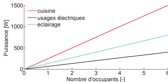
Figure 53: Puissance thermique des activités en fonction du nombre d'occupants actifs.
