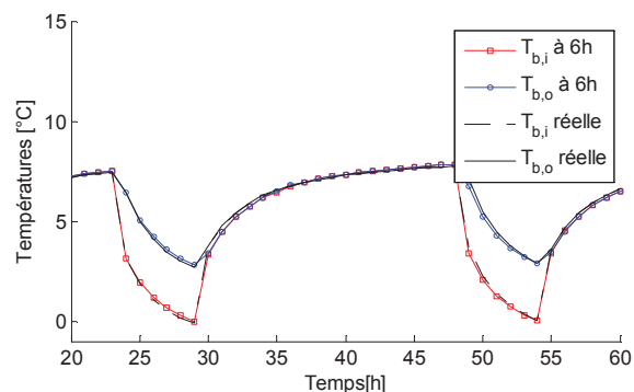
Figure 43 : Prévisions à 6 h du modèle ANN1 des températures entrée et sortie des sondes géothermiques sur un cycle de fonctionnement de la PAC.
