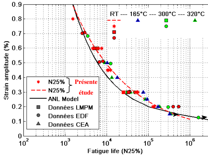
Figure III.9 : Courbes de fatigue de l'acier 304L - points expérimentaux obtenus comparés aux résultats de la littérature et à la courbe moyenne ( \epsilon - N_f )
