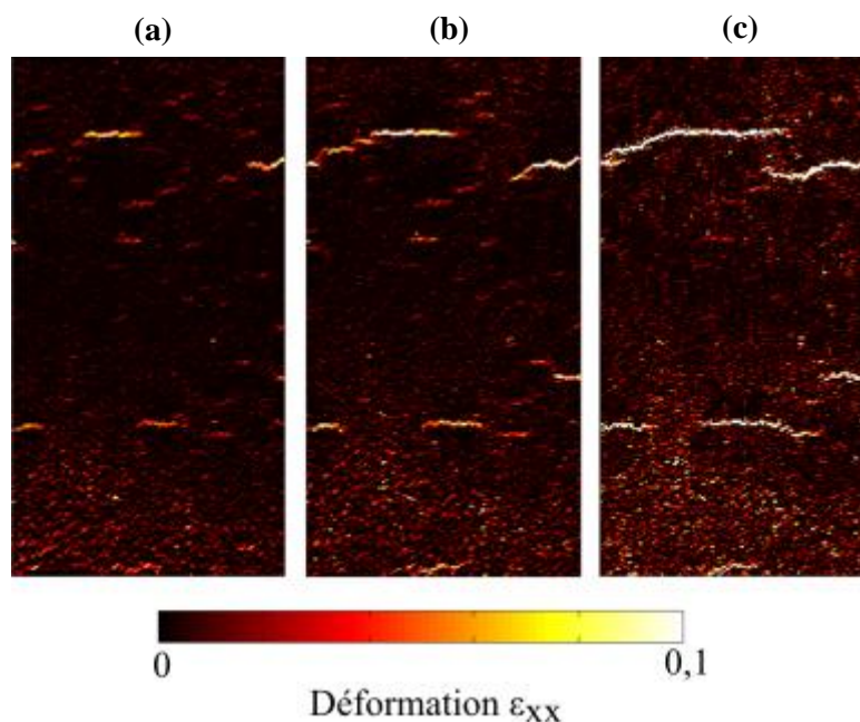
Figure I.40 : Coalescence des fissures dans un essai de fatigue à 190 MPa, à 3 instants du cyclage [Rupil 2012] : (a) 1.10^5 cycles, (b) 1,1.10^5 cycles et (c) 1,2.10^5 cycles
