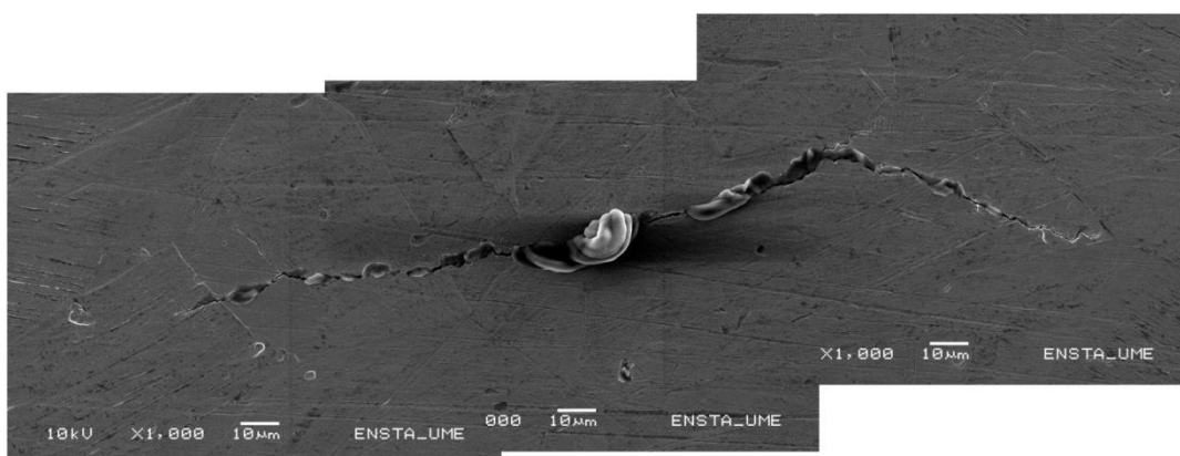
Figure IV.6 : La fissure la plus longue, observée après 6000 cycles à \Delta\varepsilon_t = \pm 0,45\%
