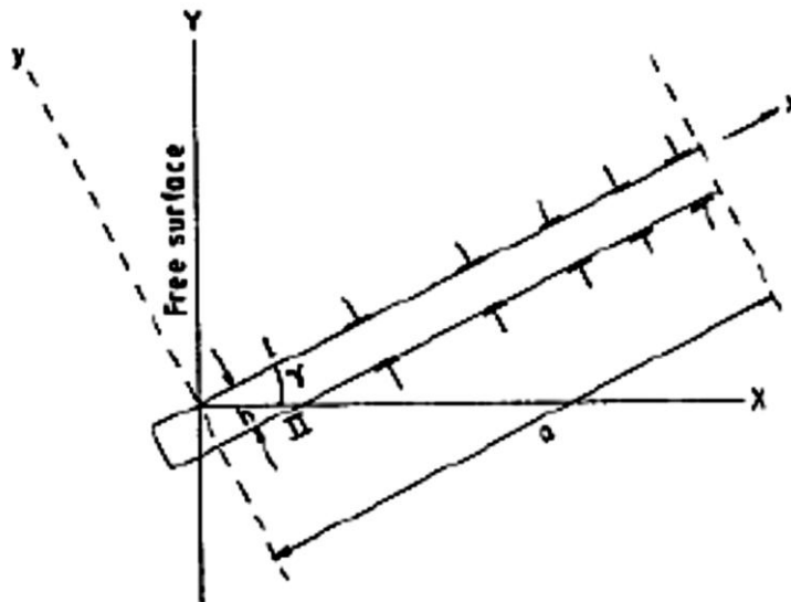
Figure I.32 : Diagramme schématisé d'une bande de glissement constituée de deux plans parallèles I et II, avec l'accumulation de dislocations polaires. [Mura 1994].
