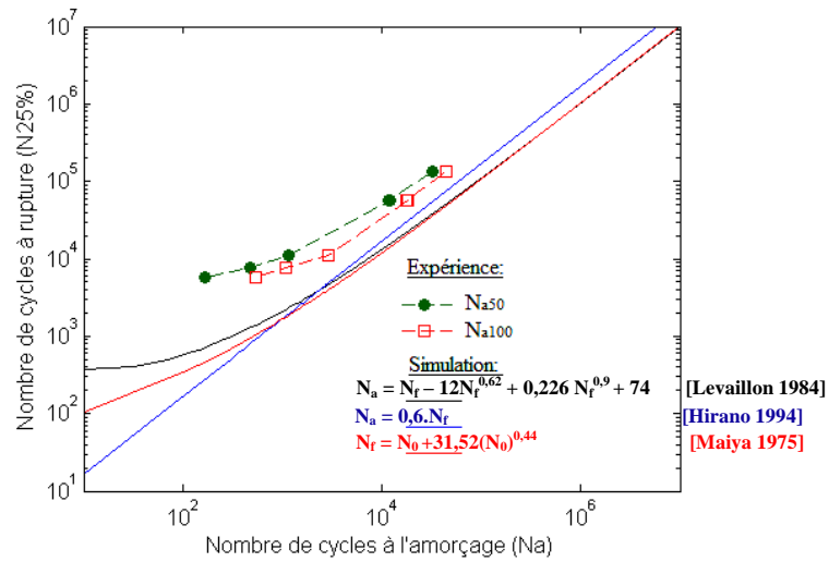
Figure IV.36 : Relation entre le nombre de cycles à rupture et celui à l'amorçage, comparée aux données de la littérature (relations I.2, I.3 et I.4 [Levailant 1984, Hirano 1994, Maiya 1975])
