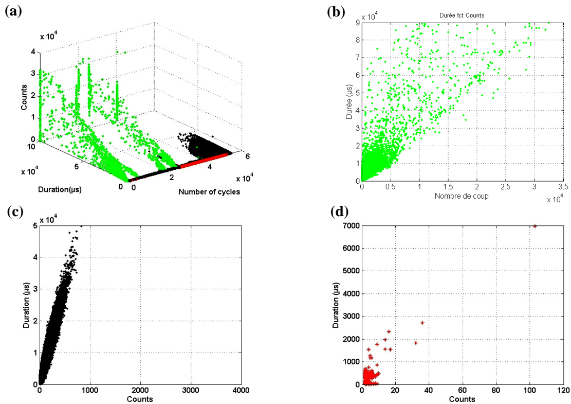
Figure IV.43 : Résultats de la segmentation des signaux acoustiques au cours d'un essai de fatigue à \Delta\varepsilon_t = \pm 0.3\% : (a) distribution de la durée et du nombre de coups des trois classes des signaux acoustiques segmentés par la méthode des k-moyennes et leurs évolutions au cours du cyclage. Et les paramètres caractéristiques de chaque classes (durée en fonction du nombre de coups) : (b) classe 1, (c) classe 2 et (d) classe 3
