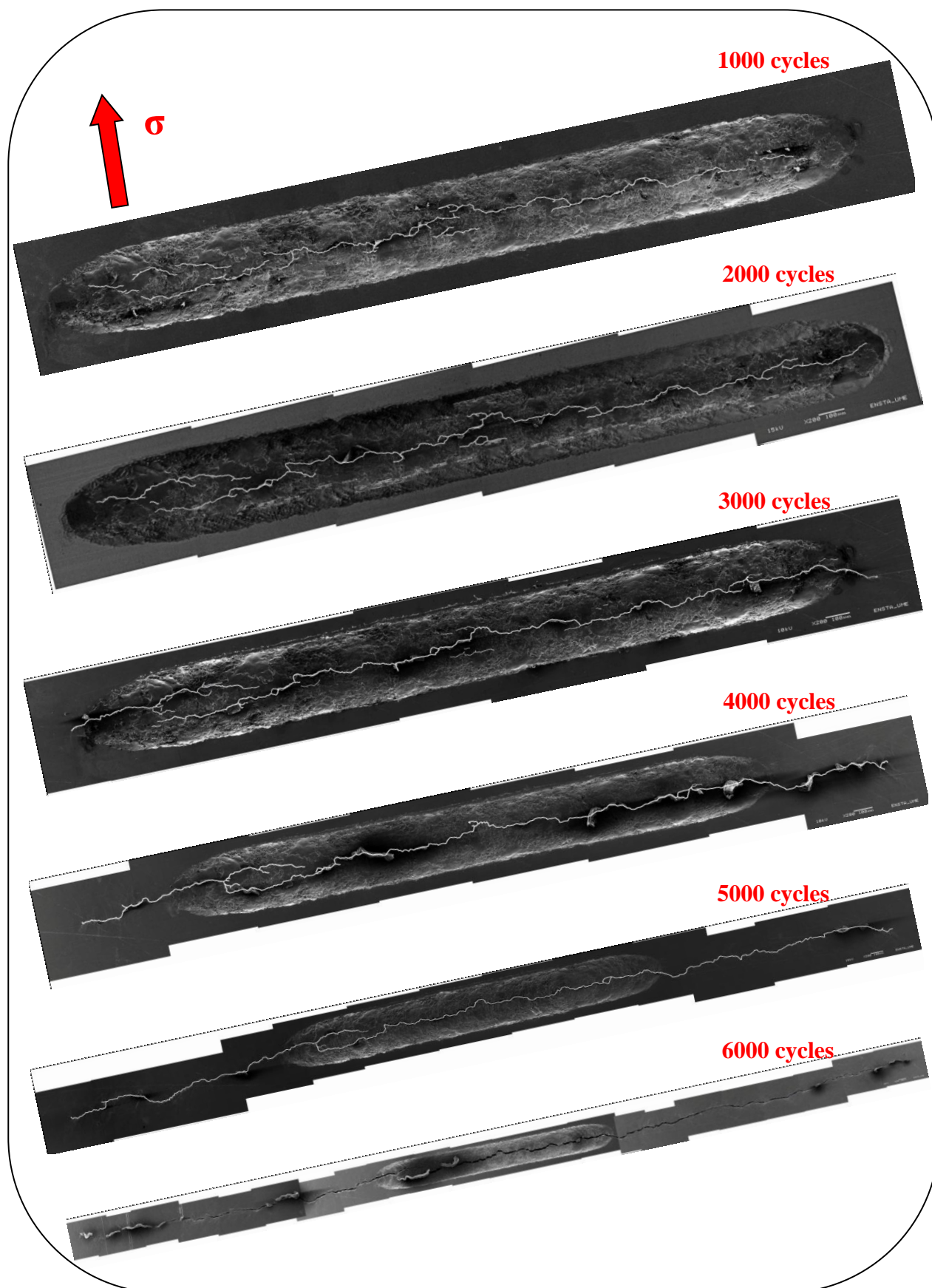
Figure A.3: Suivi de l'endommagement pour un essai de fatigue avec une éprouvette entaillée à \Delta\varepsilon/2 = \pm 0.3\%
