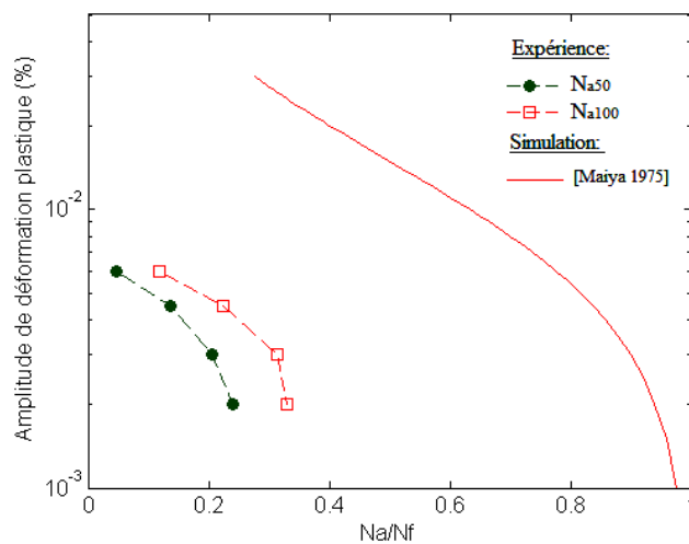
Figure IV.36 : Relation entre le nombre de cycles à rupture et celui à l'amorçage, comparée aux données de la littérature (relations I.2, I.3 et I.4 [Levailant 1984, Hirano 1994, Maiya 1975])
