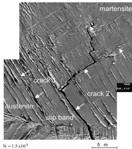
Figure I.16 : Transformation martensitique et microfissurations dans les bandes de glissement [Nebel 2003]
