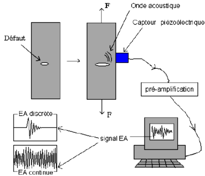
Figure II.10 : Schéma de la chaîne d'émission acoustique, de la création de l'onde mécanique à la visualisation du signal EA
