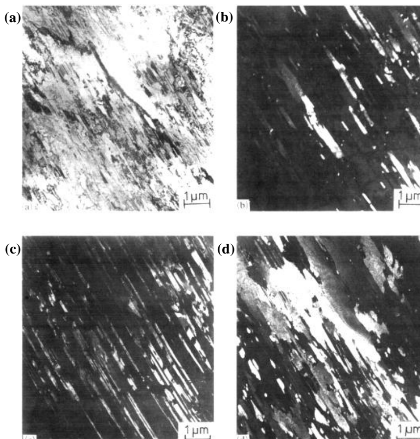
Figure I.14: Transformation martensitique par déformation sur un 304L à \Delta\varepsilon_p/2 = \pm 0,5\% , (a) champ clair, (b) champ sombre, martensite \alpha' , (c) champ sombre, martensite \varepsilon (d) champ sombre, austénite \gamma [Bayerlein 1989]
