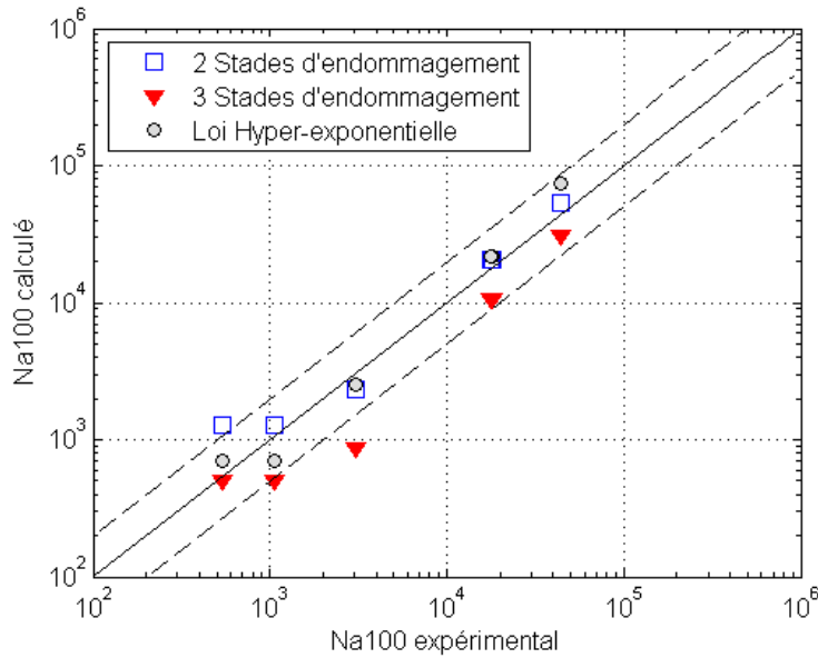
Figure IV.39: Comparaison entre le nombre de cycles à l'amorçage d'une fissure de 100 µm identifiée expérimentalement à celui estimé par différents critères d'endommagement
