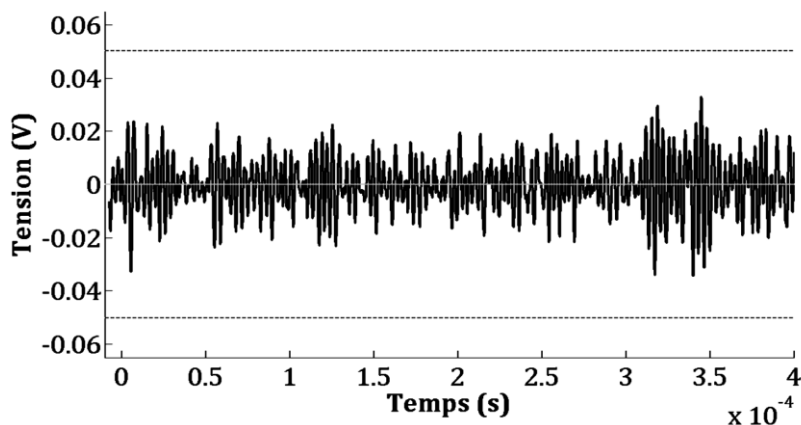
Figure II.12: Forme d'onde d'un signal d'EA continu.
