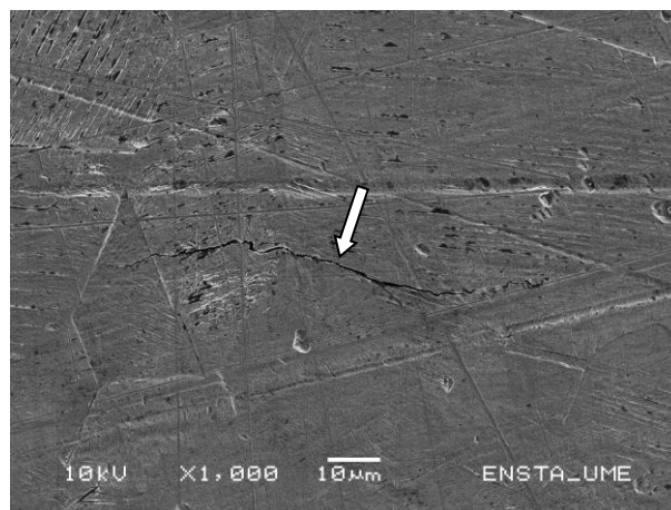
Figure IV.8 : La fissure la plus longue, observée après 20000 cycles à \Delta\varepsilon_t = \pm 0,3\%
