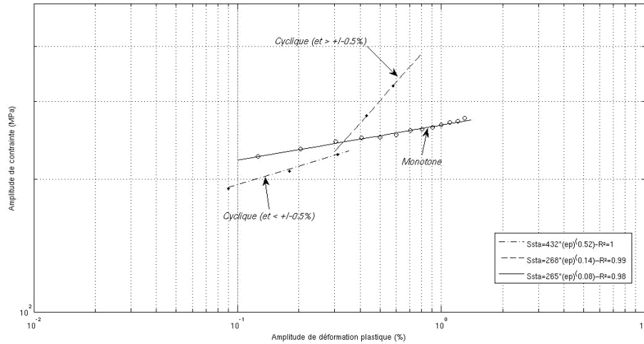
Figure III.7 : Courbes de consolidation cyclique et monotone de l'acier 304L
