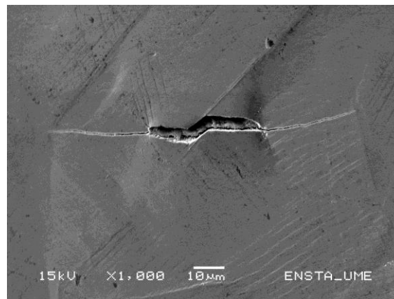
Figure IV.12 : fissure observée après 93000 cycles à \Delta\varepsilon_t = \pm 0,2\%
