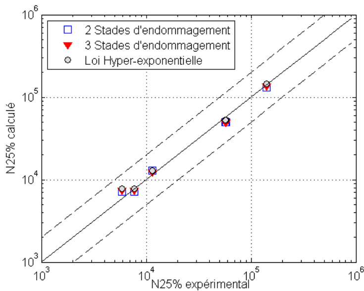
Figure IV.38: Comparaison entre les nombres de cycles à rupture obtenus expérimentalement et les nombres de cycles à rupture estimés par différents critères en termes d'endommagement
