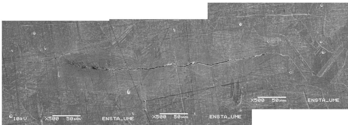
Figure IV.10 : La fissure la plus longue, observée après 32000 cycles à \Delta\epsilon_t = \pm 0,3\%
