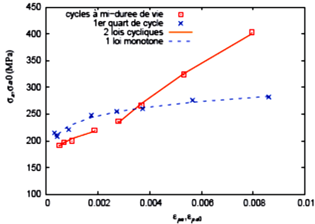
Figure I.6: Courbes d'érouissage cyclique et monotone à température ambiante d'un acier 304L [LePecheur 2008]
