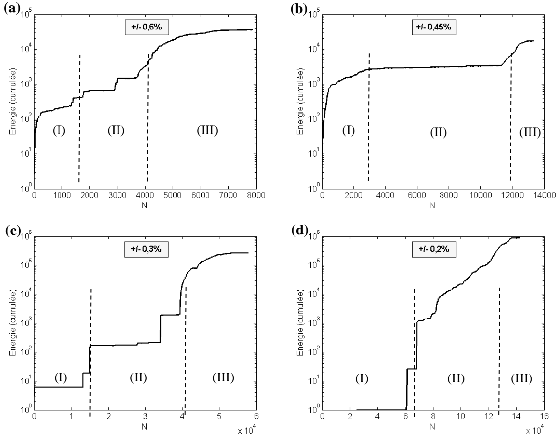
Figure IV.40 : Évolution de l'énergie cumulée des signaux acoustiques en fonction du nombre de cycles pour les différentes amplitudes de déformation (a) \Delta\varepsilon_t = \pm 0.6\% , (b) \Delta\varepsilon_t = \pm 0.45\% , (c) \Delta\varepsilon_t = \pm 0.3\% et (d) \Delta\varepsilon_t = \pm 0.2\%
