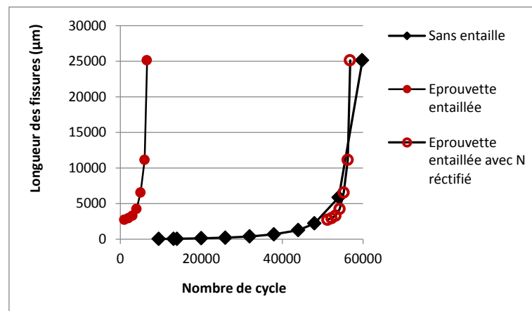
Figure A.5 : Comparaison entre l'évolution de la longueur de fissures de l'essai réalisé avec éprouvette entaillée et l'essai avec éprouvette sans entaille à déformation totale imposée similaire
