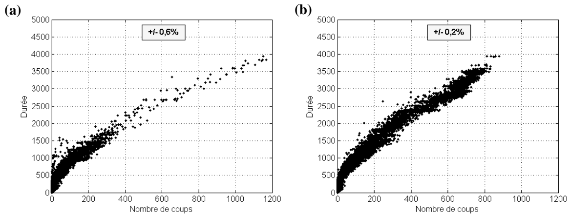
Figure IV.41 : Evolution de l'énergie cumulée des signaux acoustiques en fonction du nombre de cycles pour les différentes amplitudes de déformation (a) \Delta\varepsilon_t = \pm 0.6\% , (b) \Delta\varepsilon_t = \pm 0.2\%
