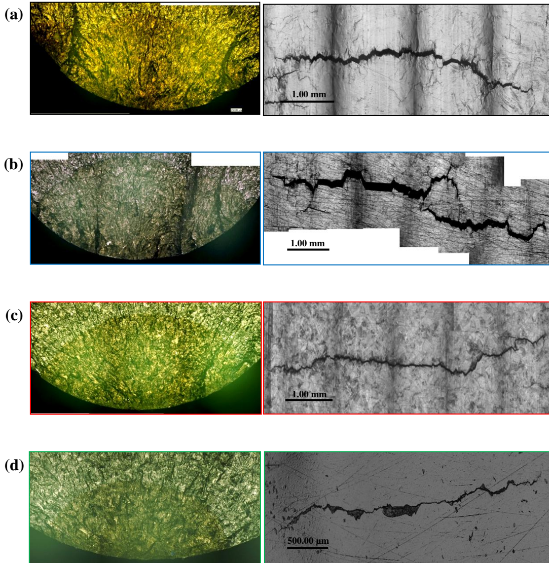
Figure IV.19 : Faciès de rupture des éprouvettes de l'acier 304L sollicitées en fatigue à différentes amplitudes de déformation totale imposées et les longueurs de la fissure principale lors du dernier arrêt avant la rupture :
