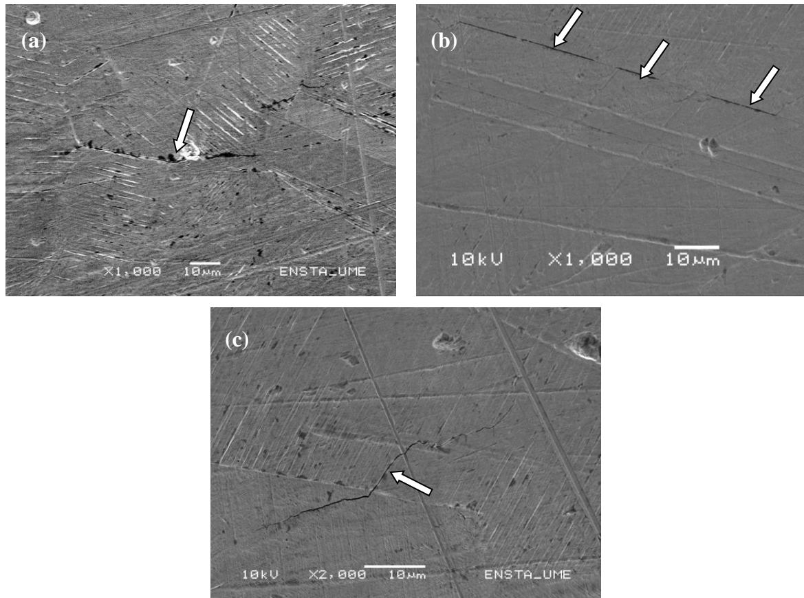
Figure IV.7 : Amorçage sur un joint de grain (a) sur un joint de macle (b) et sur une bande de glissement (c), observé après 20000 cycles à \Delta\varepsilon_t = \pm 0,3\%
