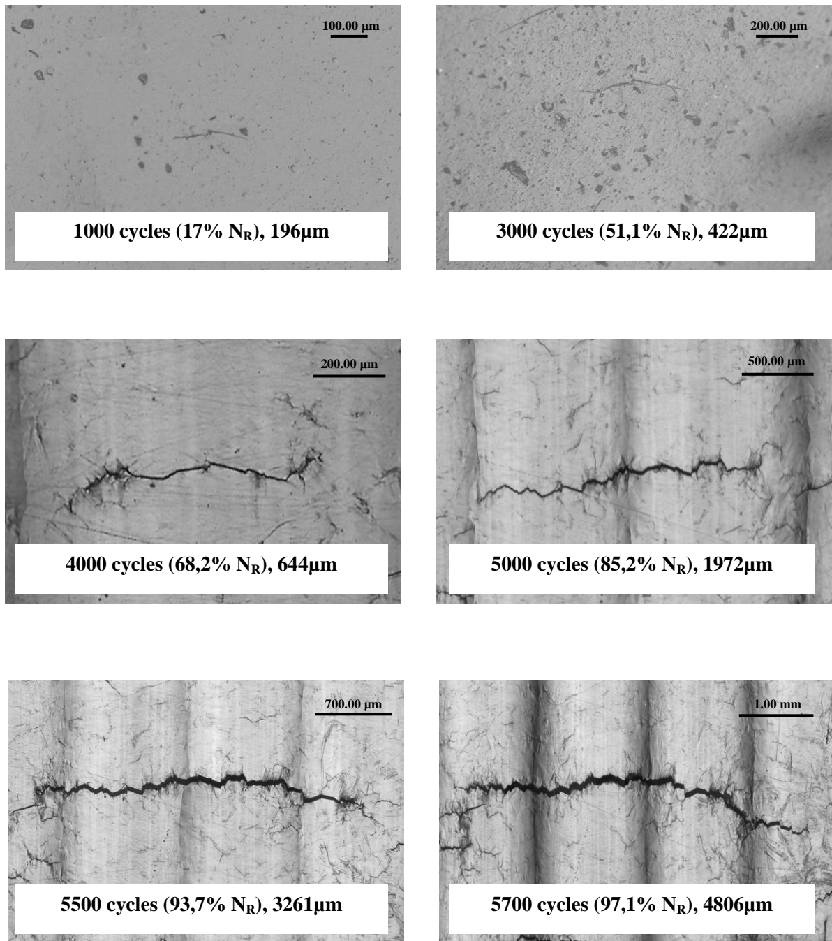
Figure IV.15 : Évolution de la fissure principale au cours du cyclage, pour l'essai à amplitude de déformation totale imposée de \Delta\varepsilon_t = \pm 0,6\% , N_f = 5867 cycles
