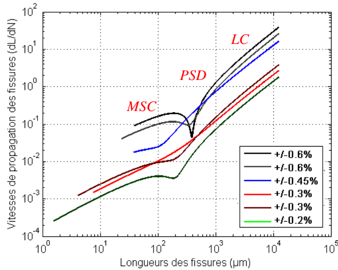
Figure IV.24 : Évolution de la vitesse de propagation des fissures en fonction de leurs longueurs en surface pour les différentes amplitudes de déformation totale imposées
