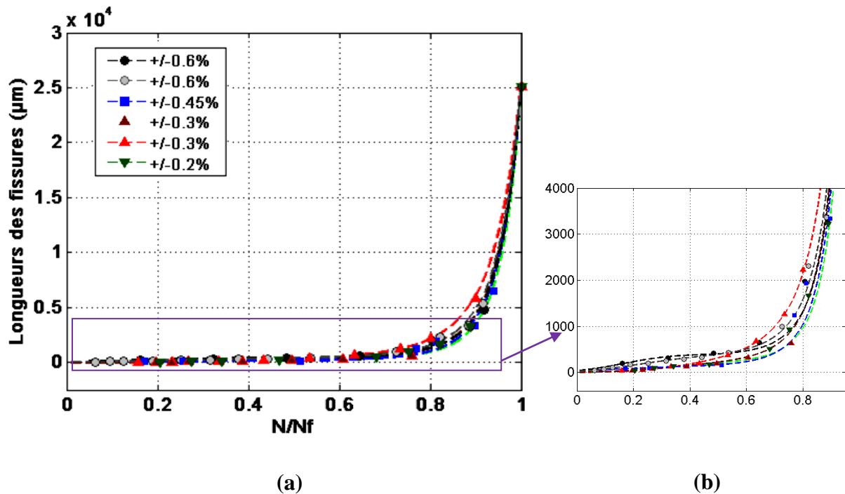
Figure IV.18 : Évolution de la longueur en surface de la fissure principale en fonction du nombre de cycles relatif à différentes amplitudes de déformation totale (a) jusqu'à rupture finale des éprouvettes (b) pendant la phase de faible croissance
