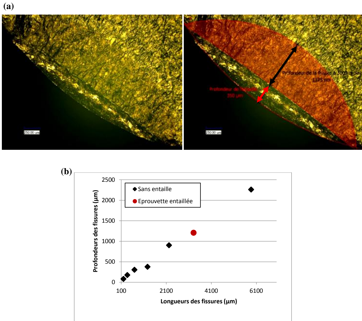
Figure A.4 : Faciès de rupture (a) et relation entre profondeur et leur longueur de la fissure formée (b) pour un essai de fatigue, à \Delta\varepsilon_t/2 = \pm 0.3\% , avec éprouvette entaillée
