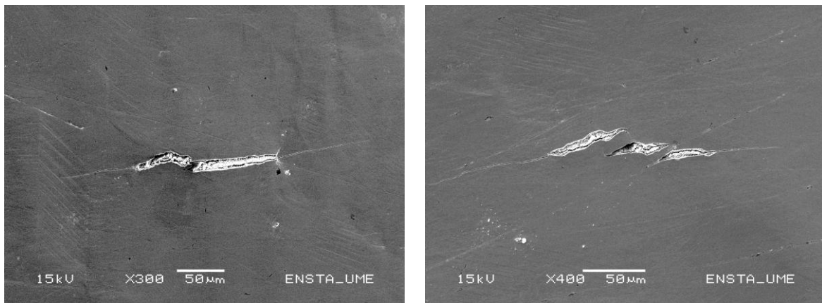
Figure IV.13 : Les fissures secondaires les plus longues, observées après 93000 cycles à \Delta\varepsilon_t = \pm 0,2\%
