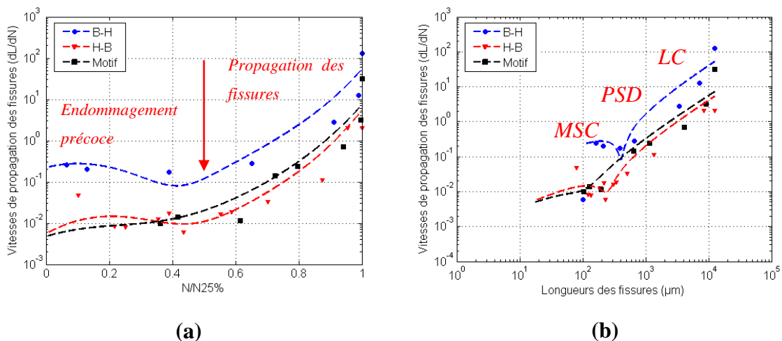
Figure V.14 : Evolution de la vitesse de propagation des fissures aux différentes configurations des essais de fatigue à amplitudes variables : (a) en fonction du nombre de cycles relative ( N/N_{25\%} ), (b) en fonction de leurs longueurs en surface
