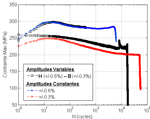
Figure V.3 : Réponse cyclique de l'acier 304L en fatigue à amplitudes variables - Configuration H-B
