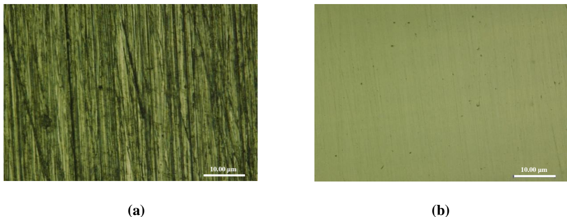
Figure II.6 : Micrographie de l'état de surface des éprouvettes, (a) à l'état brut et (b) à l'état poli
