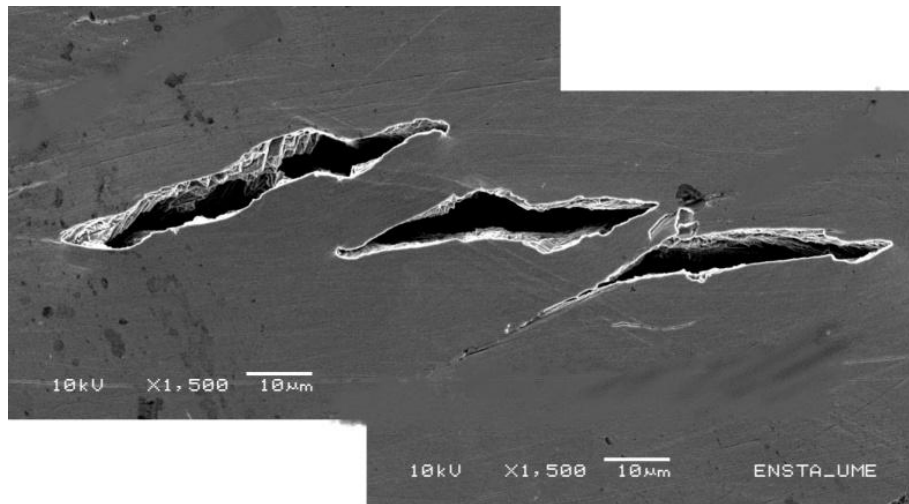
Figure IV.11 : Les fissures les plus longues, observées après 63000 cycles à \Delta\varepsilon_t = \pm 0,2\%
