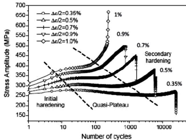
Figure I.5: Évolutions de l'amplitude de contrainte d'un acier 316L en fonction du nombre de cycles et de l'amplitude de déformation imposée [Lim 2005]
