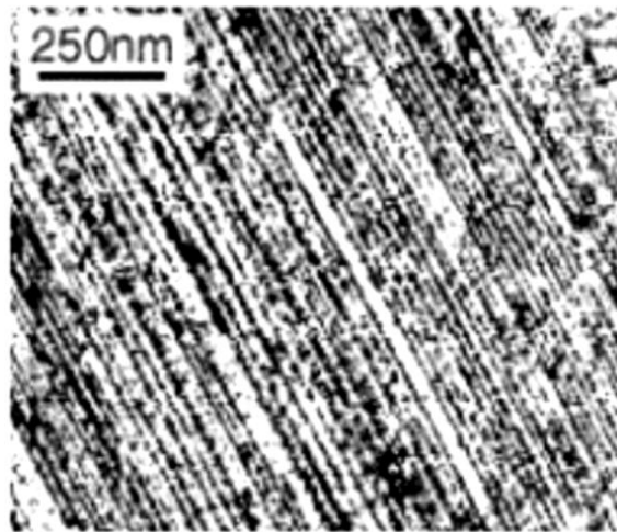
Figure I.13: Structures Corduroy formées lors d'un essai de fatigue piloté avec une amplitude de déformation de \Delta\varepsilon_p/2=0,2\% à 400 °C pour un acier 316L [Gerland 1997].
