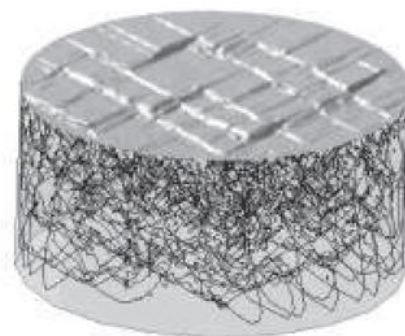
Figure I.21. Simulation des extrusions en surface en dynamique des dislocations [Déprès 2004]
