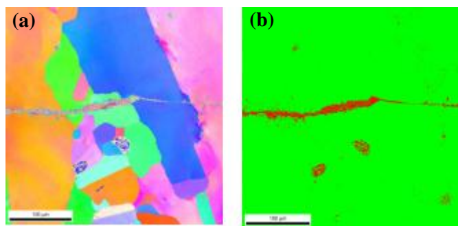
Figure I.17 : Propagation des fissures dans le "tunnel martensitique", dans une éprouvette CT sollicitée à une force supérieure à 900 N, R = 0,1: (a) distribution de l'orientation des grains austénitiques; (b) distribution de phases: (vert : austénite, rouge : martensite \alpha' ) [Stefan 2014]
