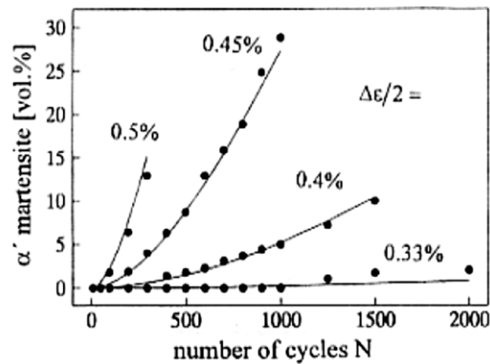
Figure I.15 : Taux de phase martensitique transformé en fonction du nombre de cycles, à différentes amplitude de déformation totale [Krupp 2001]
