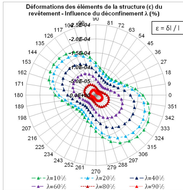
Figure 84. Représentation radiale des déformations des éléments (ε) de la structure du revêtement – Influence du déconfinement λ (%) avant la pose du revêtement.
