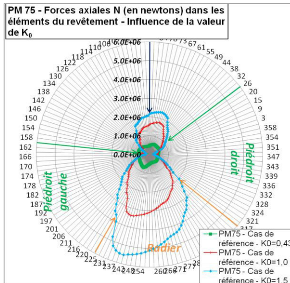
Figure 191. Représentation radiale des forces axiales internes N dans les éléments de la structure du revêtement pour le PM75 – Influence de la valeur du coefficient K_0 .
