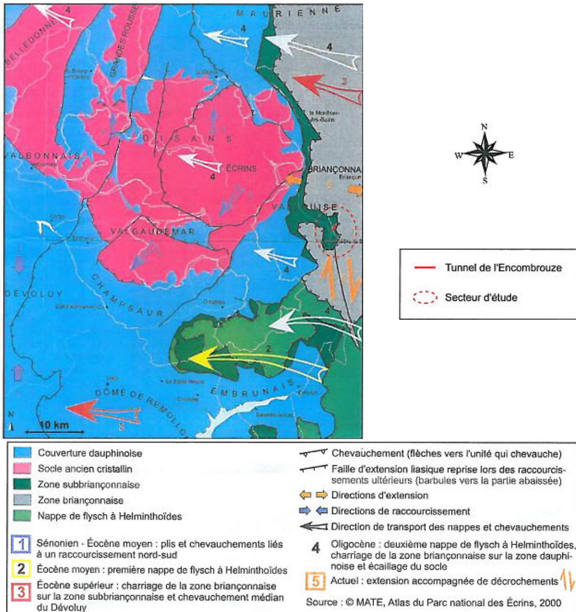
Figure 171. Contexte structural (Fenart, P., 2007).
