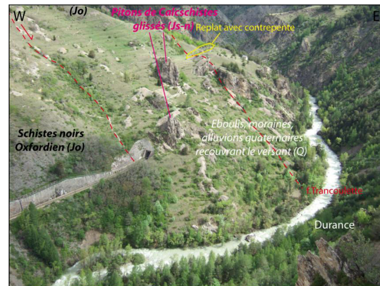
Figure 208. Panoramas illustrés du versant de la Vignette (d'après Gidon, M., 2014)
