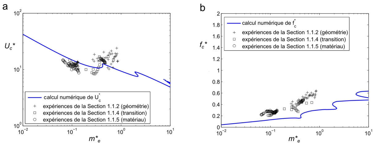
Figure 1.28 – Prédications au seuil de l'instabilité. a : Vitesse de vent critique adimensionnée en fonction de la masse ajoutée adimensionnée (approximation tridimensionnelle). L'échelle est logarithmique. b : Fréquence réduite critique f_c^* = f_c L / U_c en fonction de la masse ajoutée adimensionnée (approximation tridimensionnelle). L'échelle est semi-logarithmique.
