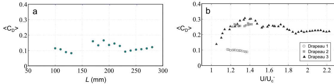
Figure 2.12 – Évolution du coefficient de traînée moyenne \langle C_D \rangle . a : En fonction de la longueur du drapeau, au seuil de l'instabilité ( U = U_c^- ). b : Pour une vitesse de vent croissante appliquée à Drapeau 1, Drapeau 2 et Drapeau 3 (Tableau 2.1).
