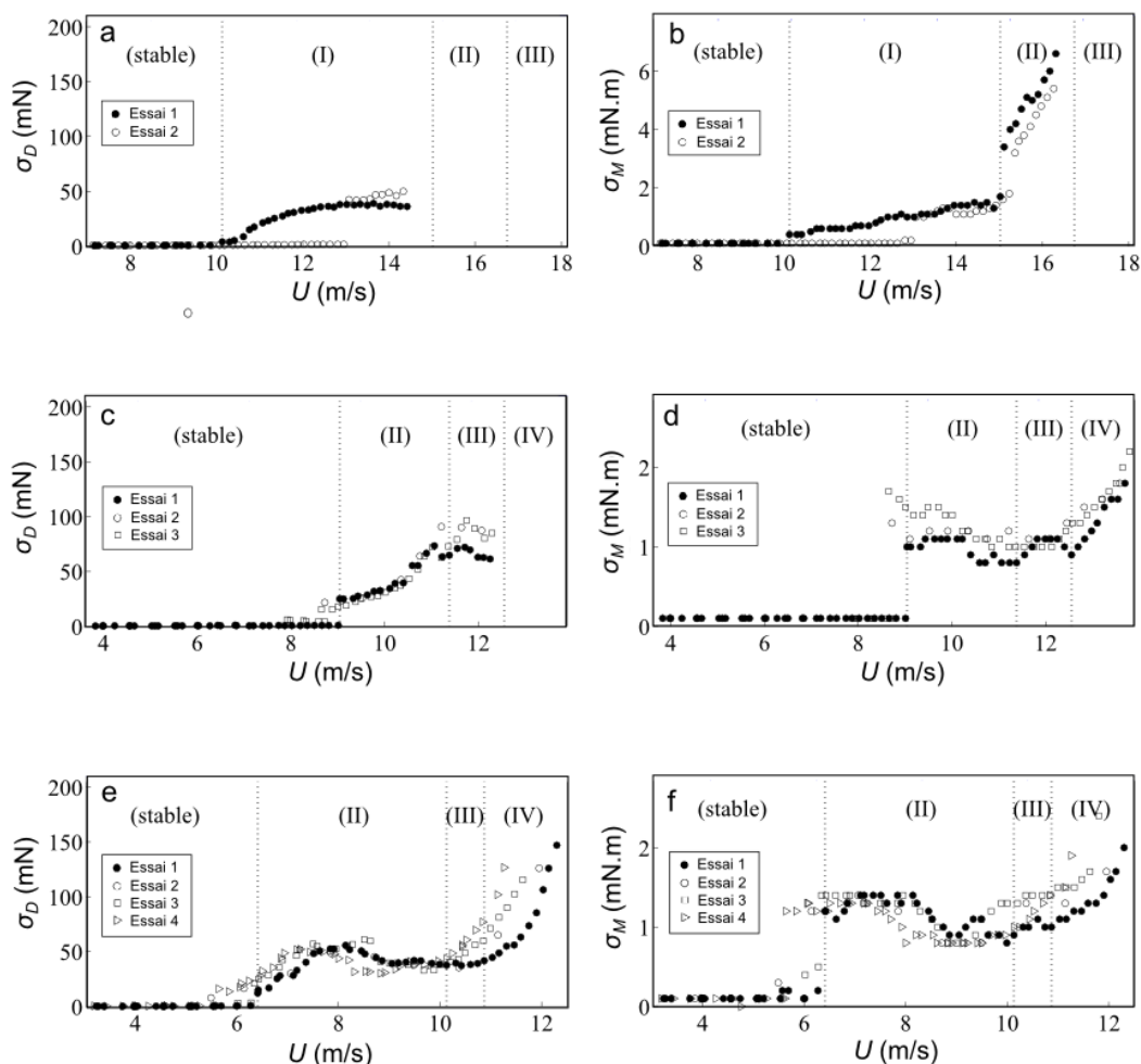
Figure 2.7 – Évolution des composantes stationnaires de la traînée D(t) et du moment M(t) , caractérisés par leur écart-type, lorsque la vitesse du vent augmente. a,b : Drapeau 1. c,d : Drapeau 2. e,f : Drapeau 3. Les symboles vides désignent des essais de reproductibilité. Les régimes (I), (II), (III) et (IV) correspondent respectivement à un, deux, trois et quatre nœuds de vibration.
