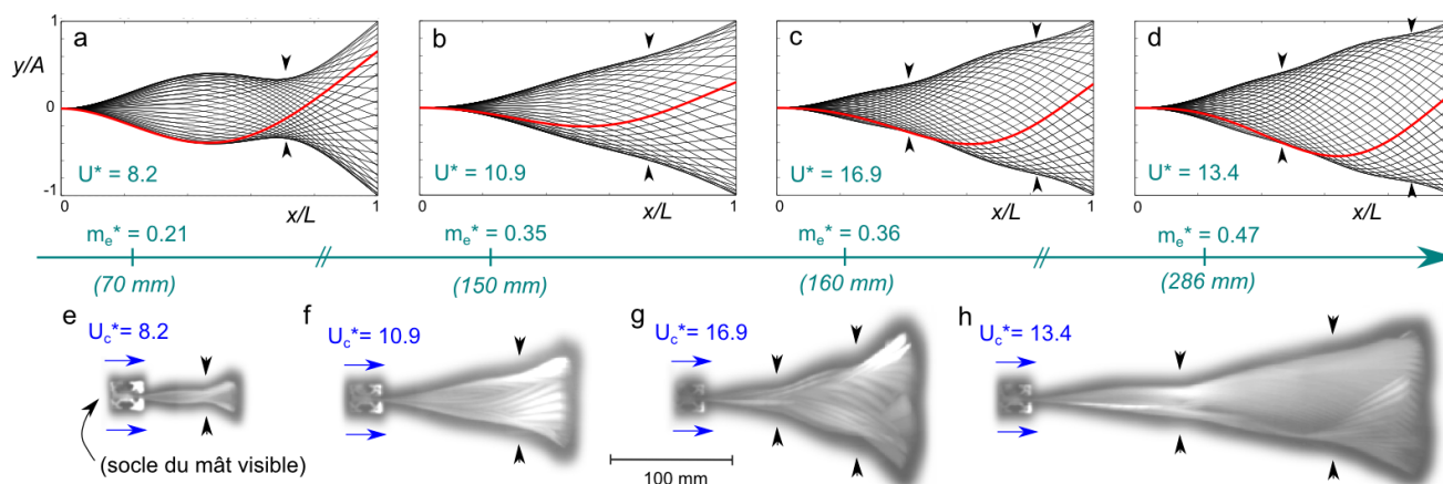
Figure 1.29 – Évolution de la superposition des déformées. Les nœuds sont indiqués par les flèches. a-d : Prédiction du modèle numérique, l'amplitude est définie à un coefficient multiplicatif près. e-h : Résultats expérimentaux de la Section 1.1.4.
