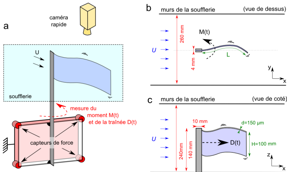
Figure 2.2 – Dispositif expérimental. a : Le drapeau et son mâte sont reliés à une balance aérodynamique destinée à mesurer les fluctuations de la traînée D(t) et du moment M(t) . b : Vue de dessus de la soufflerie et définition du moment M(t) . c : Vue de côté de la soufflerie et définition de la force de traînée D(t) .
