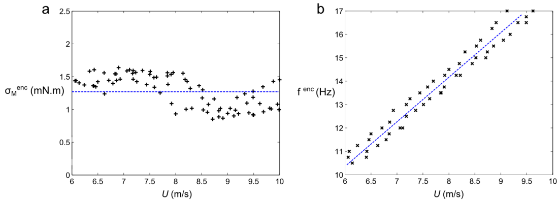
Figure 3.25 – Rappel des mesures effectuées au Chapitre 2 : superposition des résultats obtenus pour Drapeau 3. a : Sur la plage de vitesse de vent U = 6 - 10\text{ m/s} , l'écart-type du moment est bien approché par \sigma_M^{\text{enc}} \simeq 1.3\text{ mN.m} . b : Dans cette même plage de vitesse de vent, la fréquence peut être approchée par une fonction affine de U .
