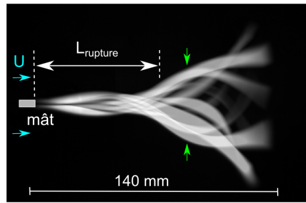
Figure D.4 – Superposition des déformées de Drapeau 1 ( L = 140 \text{ mm} ) à U = 15.0 \text{ m/s} proche de U_{rupture} . Les flèches vertes indiquent le lieu où les fluctuations de courbure sont les plus prononcées.
