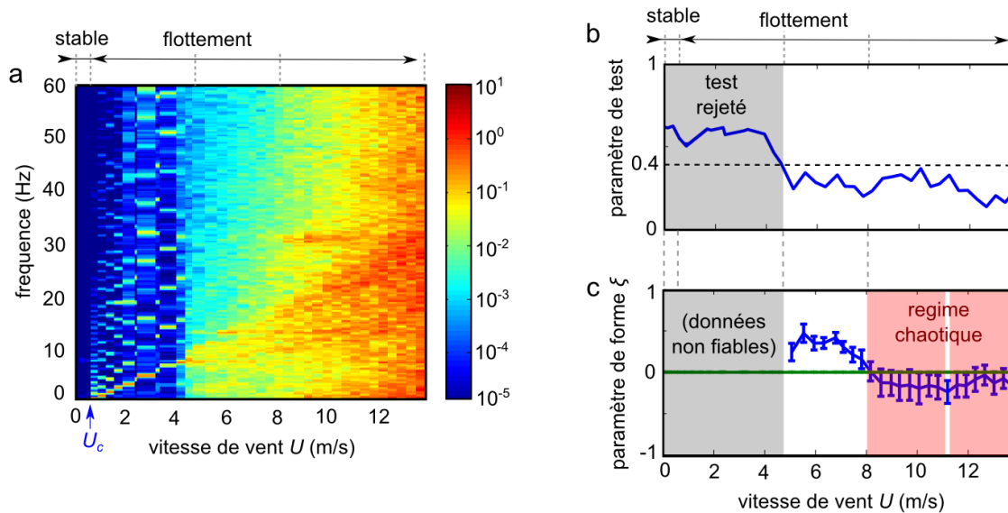
Figure E.3 – Détection du chaos. a : Évolution des densités spectrales de puissance de M(t) lorsque la vitesse du vent est augmentée. Le drapeau flotte à partir de U_c \approx 0.5 m/s. b : Résultats de l’algorithme de la Section E.3. La zone grise indique les données non fiables vis-à-vis du test de Lilliefors. c : Paramètre de forme \xi . La zone rose indique que la convergence vers une distribution de Gumbel est obtenue ( \xi \approx 0 ), c’est-à-dire que la dynamique est chaotique. Les barres d’erreurs correspondent à l’écart-type de \xi calculé pour 100 valeurs aléatoires de \zeta .
