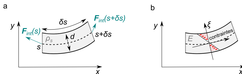
Figure 1.16 – Raisonnements sur une tranche infinitésimale de drapeau (vu dans l'épaisseur, tel que la largeur H soit dans la direction normale à la page). a : Bilan de forces internes. b : Hypothèse de contraintes variant linéairement dans l'épaisseur.
