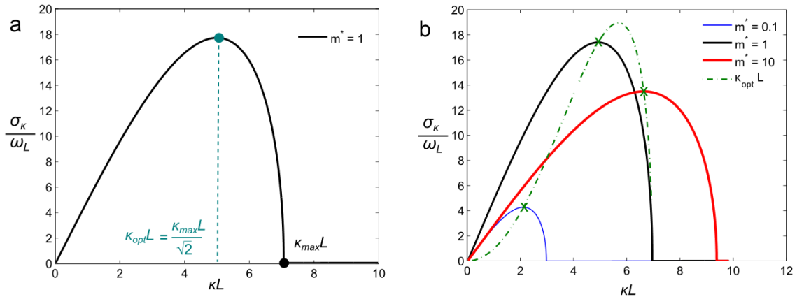
Figure 1.22 – Évolution du taux de croissance avec le nombre d'onde normalisé \kappa L . a : Présence d'un nombre d'onde limite \kappa_{\max}L et d'un taux de croissance optimum pour \kappa_{\text{opt}}L (droite verticale en pointillés). b : Allure du taux de croissance en fonction de m^* . La courbe en points-tirets précise la position de \kappa_{\text{opt}}L lorsque m^* varie entre 0 et 100.
