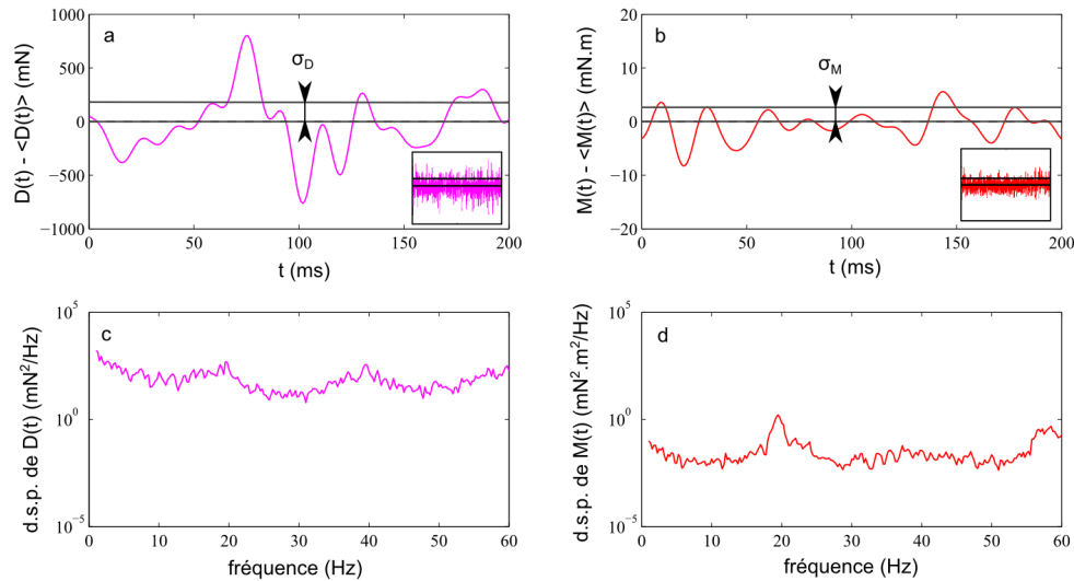
Figure 2.10 – Les claquements de drapeau illustrés dans le cas de Drapeau 3. La vitesse du vent en soufflerie est U = 12.3 m/s. a : Composante instationnaire de la traînée D(t) reconstruit sur 200 ms, caractérisée par son écart-type \sigma_D . Encart : Le signal complet de 14 s. b : Composante instationnaire du moment M(t) reconstruit sur 200 ms, caractérisée par son écart-type \sigma_M . Encart : Le signal complet de 14 s. c,d : Densités spectrales de puissance respectives des signaux de 14 s, en échelle semi-logarithmique.
