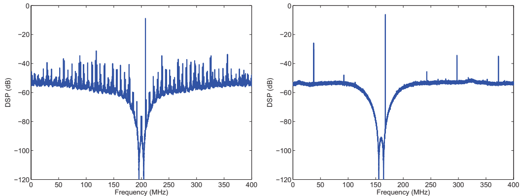
(a) Effets non linéaires dans les modulateurs F_s/4 (b) Réduction des effets non-linéaires pour les modulateurs non- F_s/4
