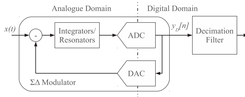
FIGURE 8 – Schéma de la structure générale d'un convertisseur \Sigma\Delta
