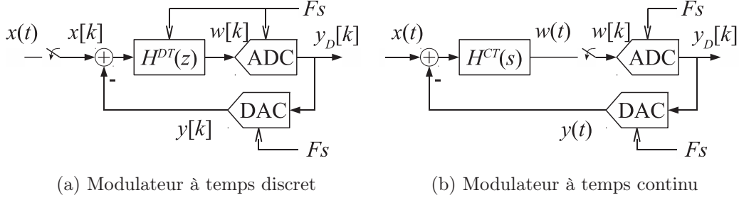
FIGURE 10 – Schéma des implémentations des modulateurs \Sigma\Delta
