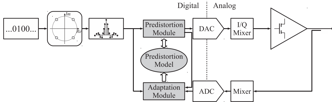
FIGURE 4 – Schéma détaillé de la prédistorsion numérique
