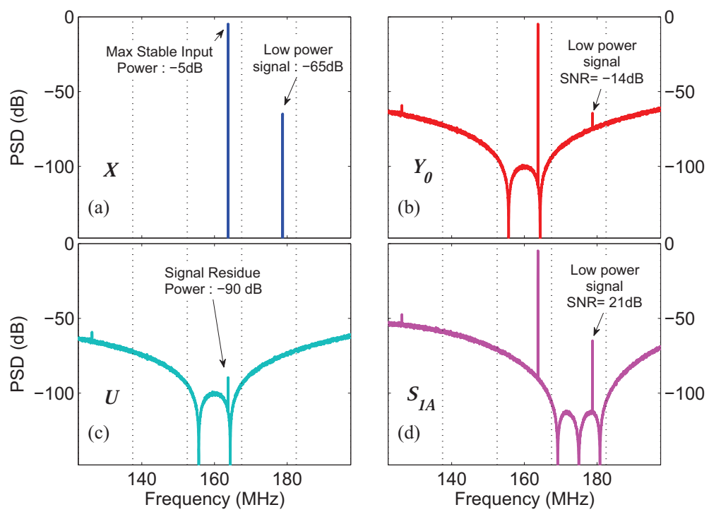
FIGURE 28 – Spectres dans la configuration choisie de convertisseur MSNBC
