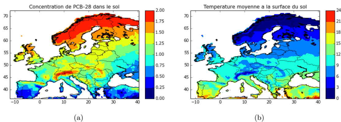
FIGURE 5.35 – Concentration de PCB28 dans le sol au bout de 10 ans avec le scénario sans émission (en \mu\text{g}\cdot\text{m}^{-3} ) et température moyenne annuelle à la surface du sol (en ^{\circ}\text{C} ).
