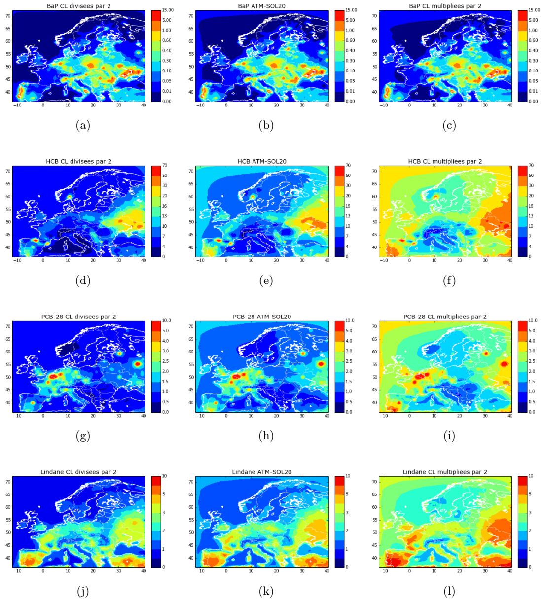
FIGURE 5.24 – Concentration annuelle dans l'air avec des conditions limites divisées (colonne de gauche) ou multipliées (colonne de droite) par 2 (en \text{ng}\cdot\text{m}^{-3} pour le BaP et en \text{pg}\cdot\text{m}^{-3} pour les autres POPs).
