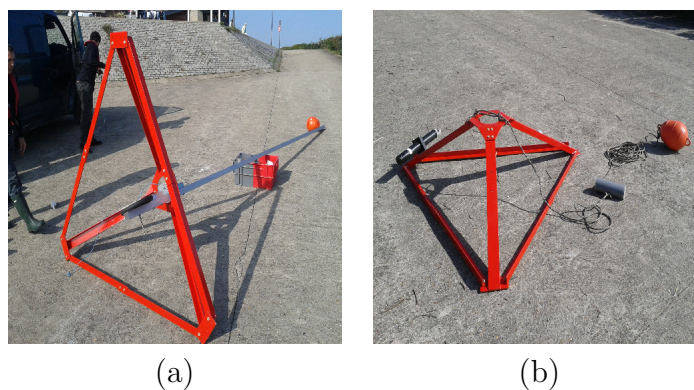
FIGURE 2.14: (a) : Mât fixé sur un trépied sur lequel les appareils de mesure de courant sont fixés, (b) : Trépieds sur lequel l'ADCP peut être placé
