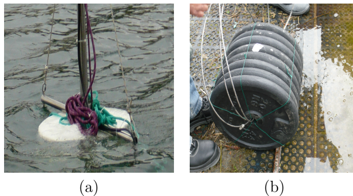
FIGURE 2.13: (a) : Flotteur sur le quel la station météo à été fixée, (b) : Poids de 160 kg pour stabiliser la chaîne de capteurs
