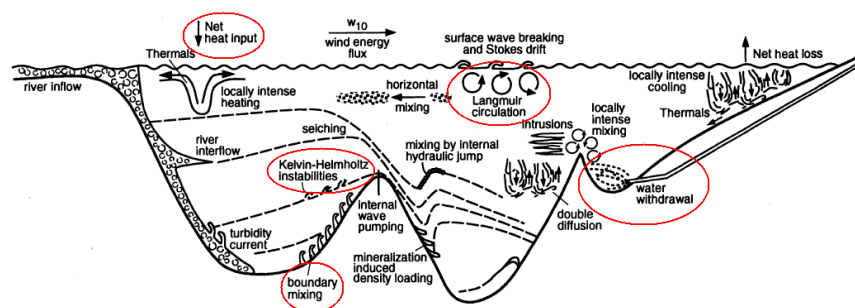
FIGURE 1.2: Schéma des différents forçages météorologiques sur un plan d'eau Lerman and Gat (1995)
