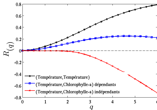
FIGURE 4.12: Comparaison des R(q) obtenus pour différentes combinaisons de : en noir (Température,Température), en rouge (Température,Chlorophylle-a) indépendants, en bleu (Température,Chlorophylle-a) dépendants
