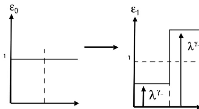
FIGURE 3.11: Schéma du \alpha -modèle. A chaque étape de la cascade le champs est divisé en 2 et multiplié soit par \gamma+ ou \gamma- , d'après Fitton (2013)
