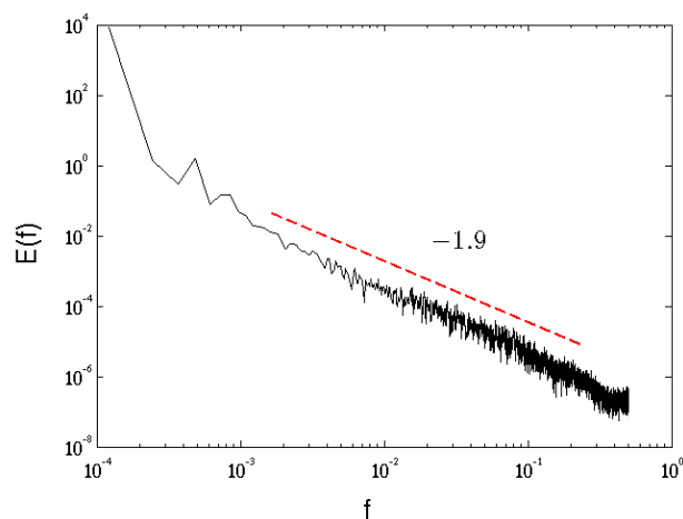
FIGURE 2.31: Spectre de densité d'énergie de l'oxygène dissous dans le lac de Créteil, (1 unité en fréquence = 0.03 Hz)
