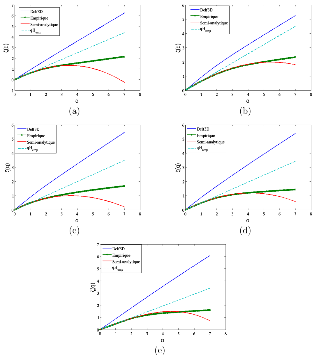
FIGURE 4.30: Exposant de la fonction de structure \zeta(q) du champ de température (simulée et mesurée) à différentes profondeurs : (a) : 0.5m, (b) : 1.5m, (c) : 2.5m, (d) : 3.5m, (e) : 4.5m
