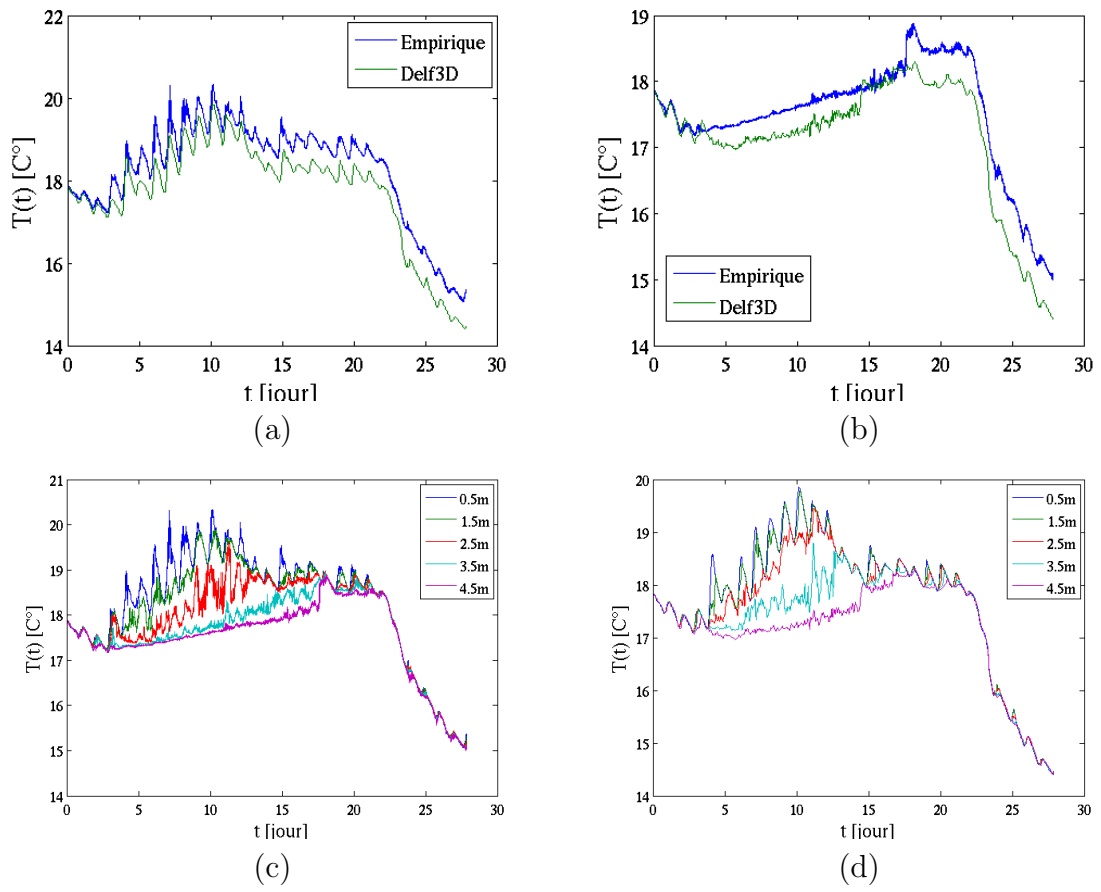
FIGURE 4.27: Séries temporelles de température (simulées et mesurées) pour différentes profondeurs, (a) : champ de température à 0.5m,(b) : champ de température à 1.5m, (c) : champs de température mesurées sur le lac, (d) : champs de température simulées
