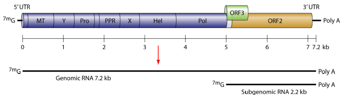
Figure 15 : Structure du génome du VHE (Kamar et al., 2014)
