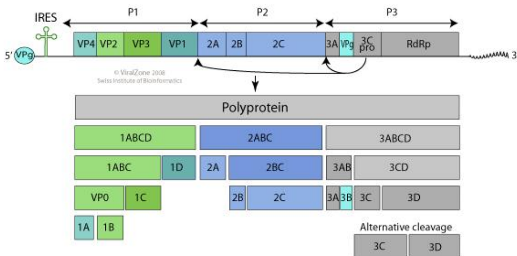
Figure 11 : Organisation génomique de VHA (ViralZone)
