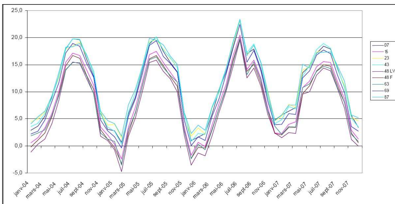
Figure 6.1 : Courbe des températures relevées sur neuf sites d'essai (source : Météo France)
