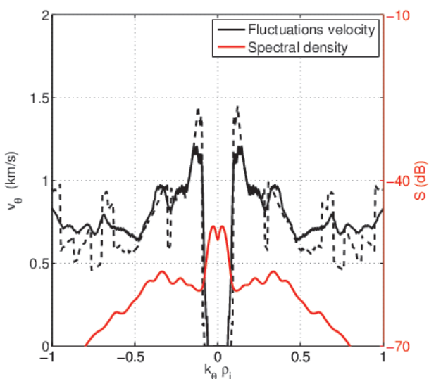
(d) Vitesse des fluctuations et énergie spectrale dans la zone TOP.
