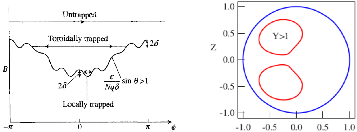
(a) Variation toroïdale du champ magnétique, montrant la différence entre particules passantes, piégées toroïdalement (particules banane) et piégées localement. Seules les zones avec \varepsilon \sin(\theta) / Nq\delta < 1 ont des puits ripple [Wes04].
