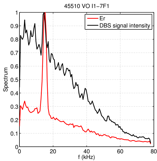
(c) Visée verticale mode O à \rho \sim 0.82 moyenne entre les déclenches 1 à 7
