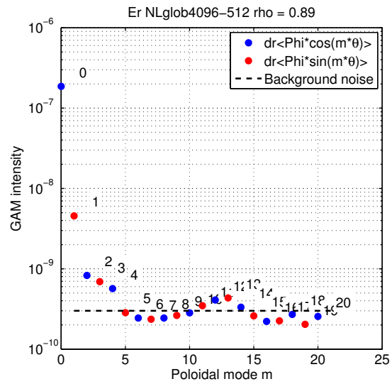
(d) Répartition de l'énergie GAM entre composantes (régime turbulent)
