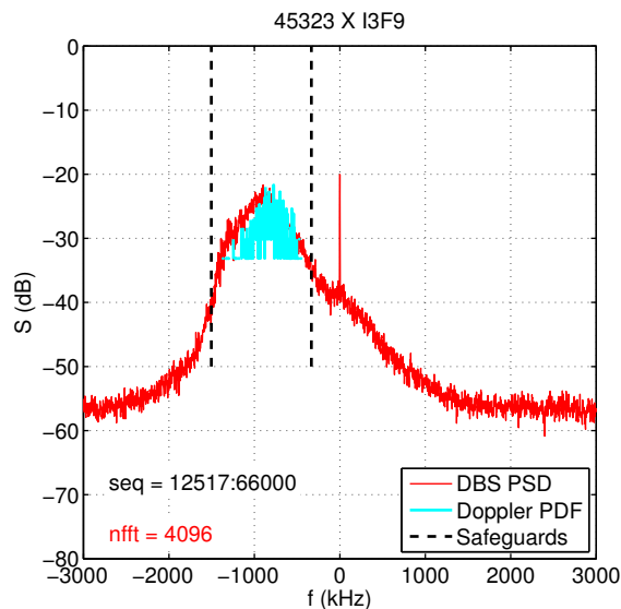
FIGURE 4.5 – Aligement de la densité spectrale de puissance (PSD) du signal d’acquisition avec la distribution (PDF) de la série de décalages Doppler obtenue avec la méthode MUSIC.
