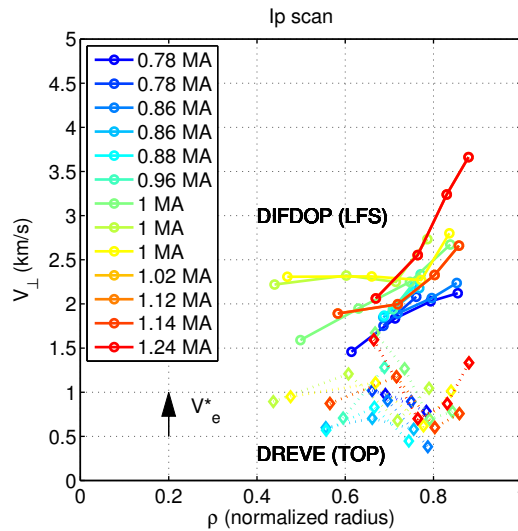
FIGURE 3.1 – Illustration du résultat principal pour la série de plasmas du tableau 3.1 à B_0 = 3.87 T , et P_{ICRH} = 2 MW , où I_p varie entre 0.78 et 1.24 MA : V_{\perp} est plus intense côté bas champ qu'en haut de la machine. Dans les conventions adoptées, V_{\perp} > 0 correspond au sens diamagnétique électronique, soit vers le haut côté bas champ de la machine.
