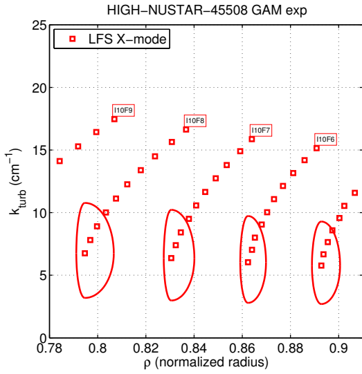
(a) Localisation de certaines mesures mode X du choc 45508.
