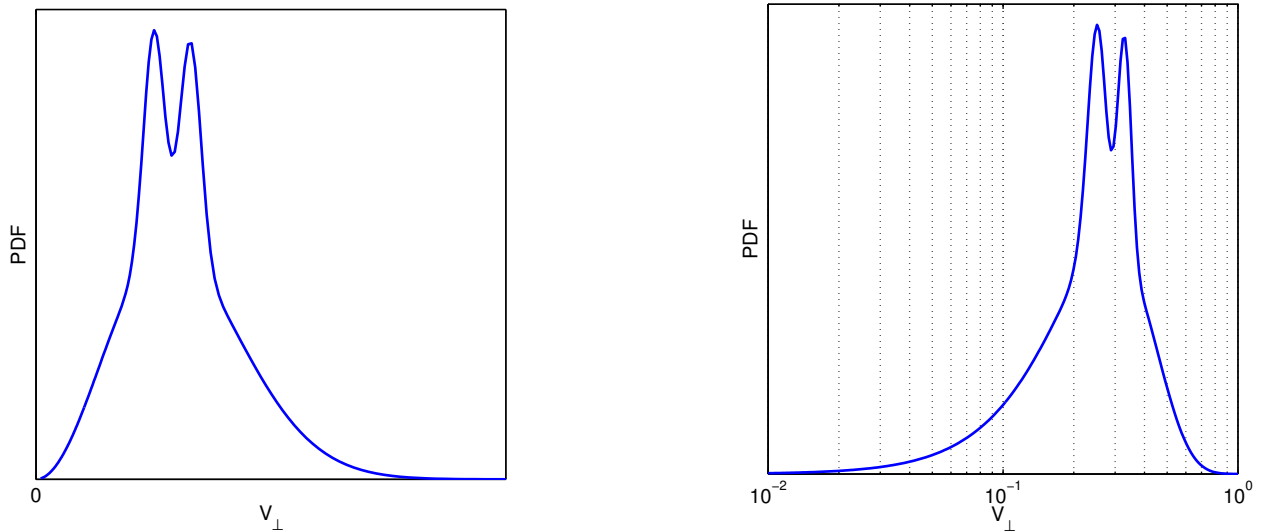
(b) Illustration d'une PDF hypothétique modifiée par la présence d'oscillations prédateur-proie raisonnablement nettes, stationnaires et harmoniques.
