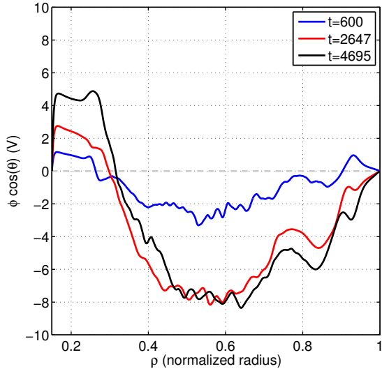
(b) Composante \langle \phi \cos \theta \rangle à trois instants
