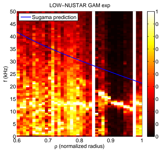
(a) Cas bas v^* .
