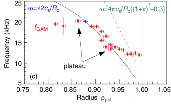
FIGURE 5.19 – Observation de paliers de fréquence GAM sur ASDEX (petit rayon a = 0.5 m , grand rayon R_0 = 1.65 m , vitesse du son c_s = \sqrt{(T_e + T_i)/m_i} , facteur de sécurité q_{95} = 3.66 et élongation \kappa_b = 1.09 ) (adapté de [CTS + 08]).
