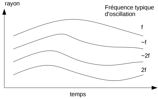
(b) Illustration de la variation radiale de la fréquence GAM, d'un facteur 2, de part et d'autre d'un saut de phase.
