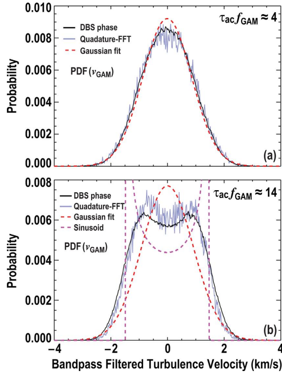
FIGURE 5.44 – Dans deux plasmas de DIII-D, distribution de V_{\perp,GAM} montrant en (a) un GAM relativement peu cohérent dans un plasma chauffé additionnellement à 2.7 MW et en (b) un GAM très cohérent dans un plasma chauffé additionnellement à 4.7 MW. La distribution du cas (a) est la mieux représentée par une gaussienne (tirets rouges) tandis que la distribution du cas (b) est intermédiaire entre la gaussienne et la densité de probabilité d’une sinusoïde (tirets roses), typique d’une oscillation harmonique et stationnaire de V_{\perp,GAM} [HPC + 12].
