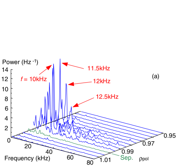
(a) Observation de multiples pics GAM à proximité de la séparatrice dans ASDEX [CSS + 05].
