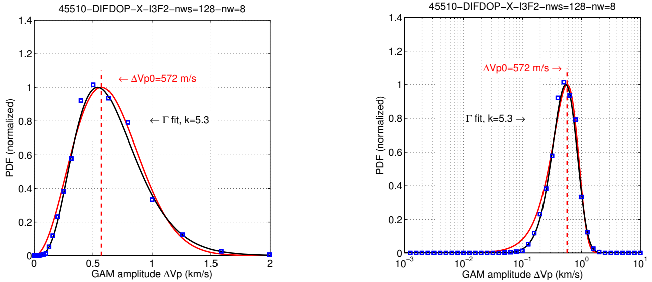
(a) Exemple de PDF obtenue expérimentalement dans le choc 45510, haut v^* (échelle linéaire à gauche, logarithmique à droite).
