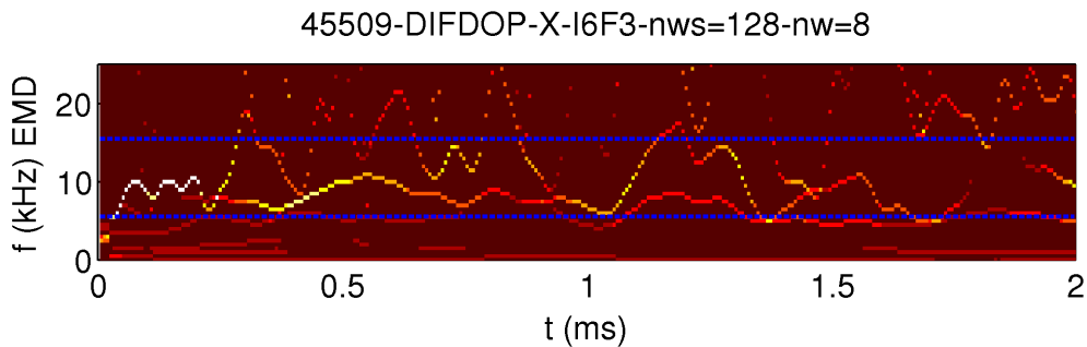
(a) Algorithme de Rilling
