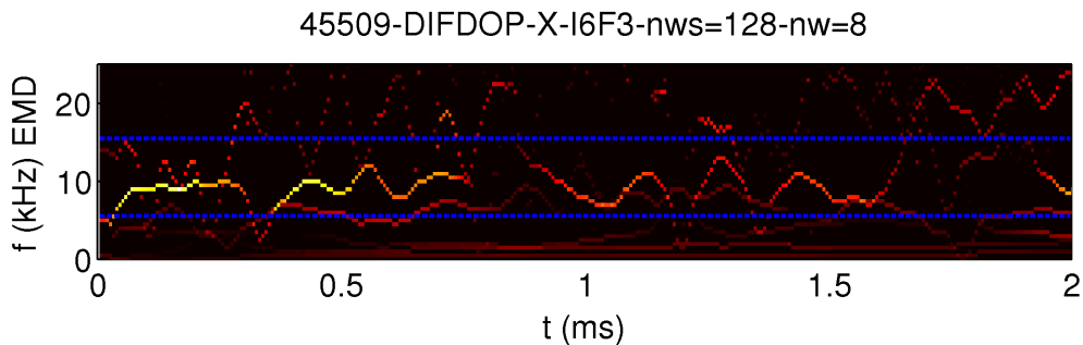
(b) Algorithme CEEMDAN (méthode d'analyse assistée par le bruit)
