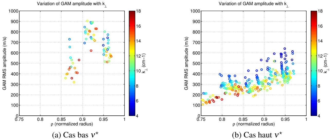
FIGURE 5.39 – Intensité des GAMs en fonction du rayon et de l'échelle de mesure k_{\perp} ( cm^{-1} ).
