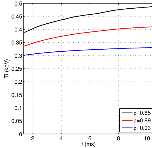
FIGURE 5.35 – Variation temporelle de la température dans la simulation à trois rayons.
