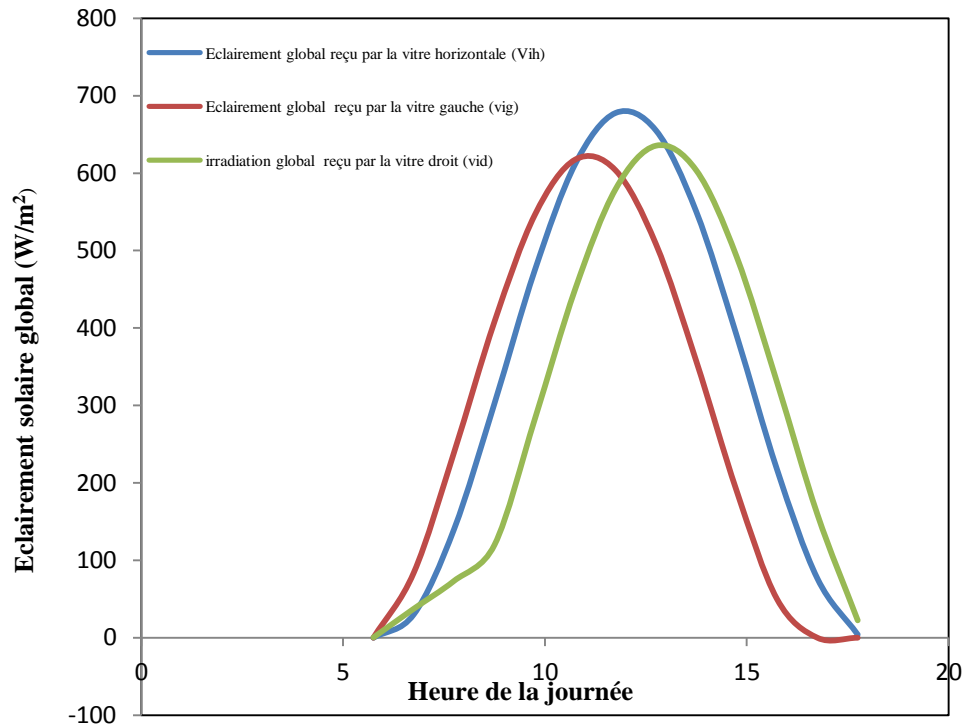
Fig. 3.16 Simulation de l'évolution de l'éclairage solaire global sur les trois vitres du séchoir solaire de Kilichi pour la journée du 27 Août dans la localité de N'gaoundéré.
