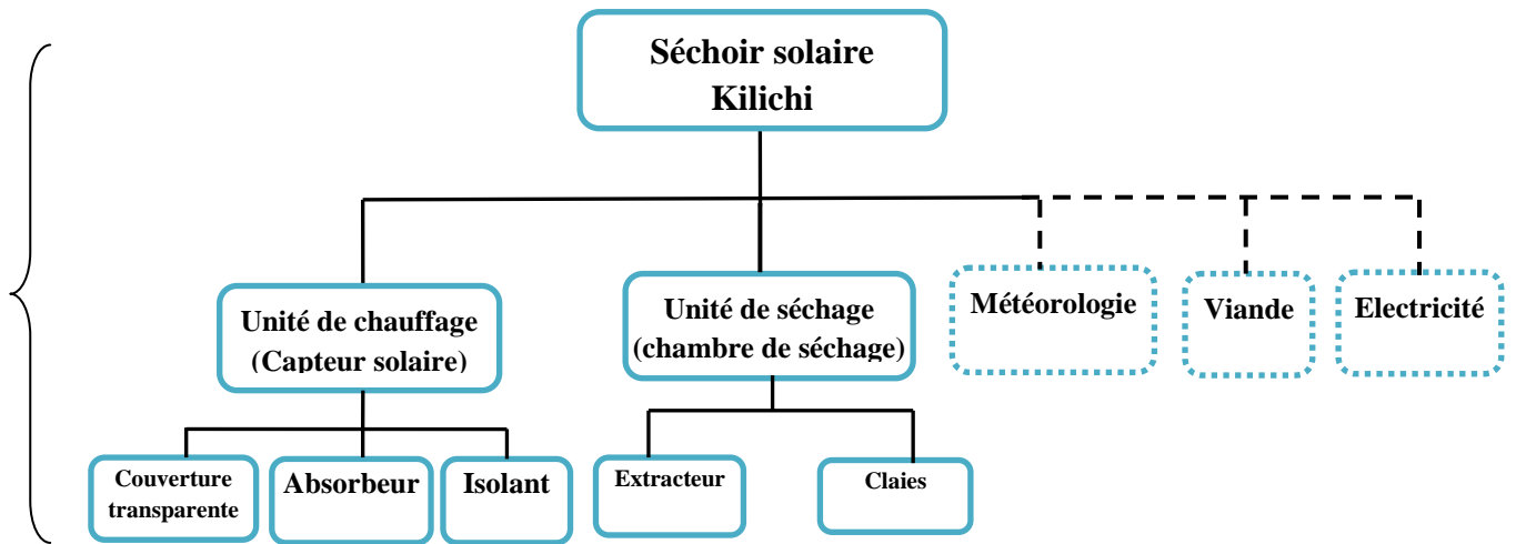
Fig. 3.6 Organigramme Technique (OTé) de niveau 3 du séchoir solaire de Kilichi .
