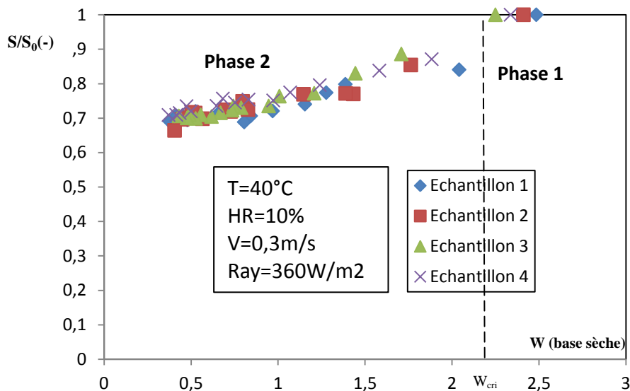
Fig. 5.18 Evolution de la surface relative de quatre échantillons de viande séchés dans les mêmes conditions.
