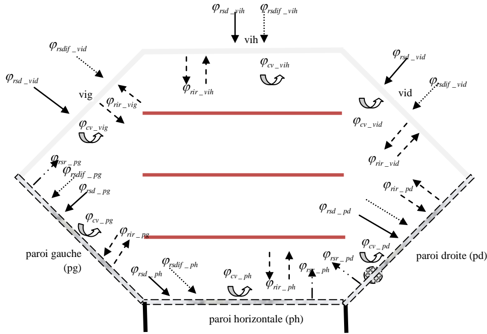
Fig. 4.8 Bilan d'énergie sur les vitres et parois du séchoir de Kilichi : → rayonnement solaire direct, ..... → rayonnement solaire diffus - - - → rayonnement solaire infrarouge, ↻ convection, ← → rayonnement solaire réfléchi.
