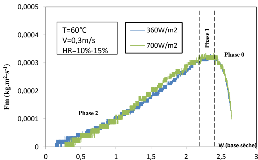
Fig. 5.14 Evolution du flux masse F_m en fonction de la teneur en eau W pour deux valeurs d'intensités de rayonnement solaire ( 360 \text{ W/m}^2 et 700 \text{ W/m}^2 ).
