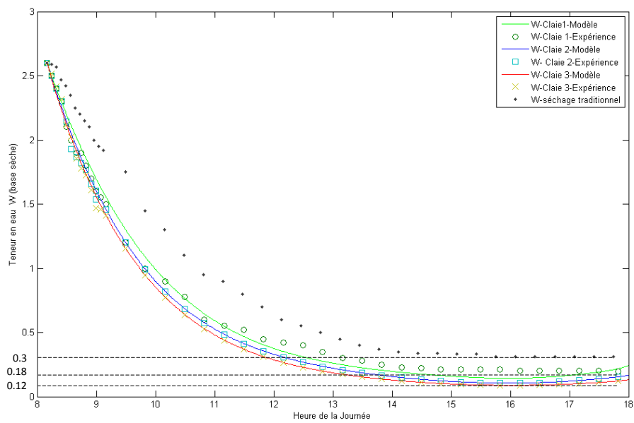
Fig. 4.30 Evolution de la teneur en eau W en fonction des heures de la journée, dans le séchoir et à l'air libre (séchage traditionnel) : valeurs expérimentales et modélisées pour la journée du 22 Avril 2014.
