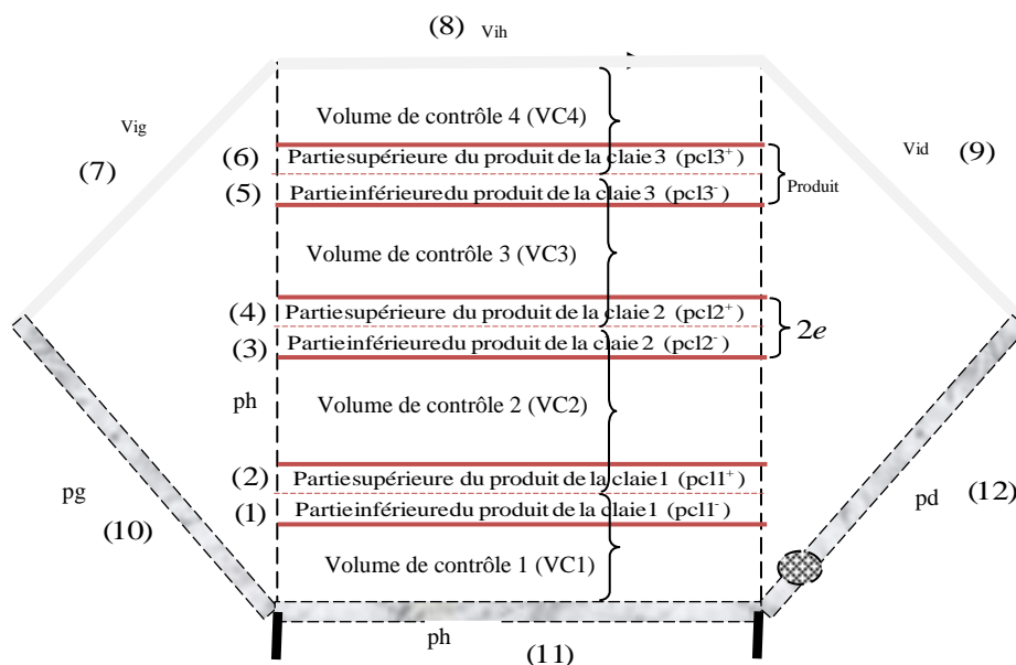
Fig. 4.2 Vue de face intérieure du séchoir solaire de Kilichi : décomposition des surfaces du séchoir.
