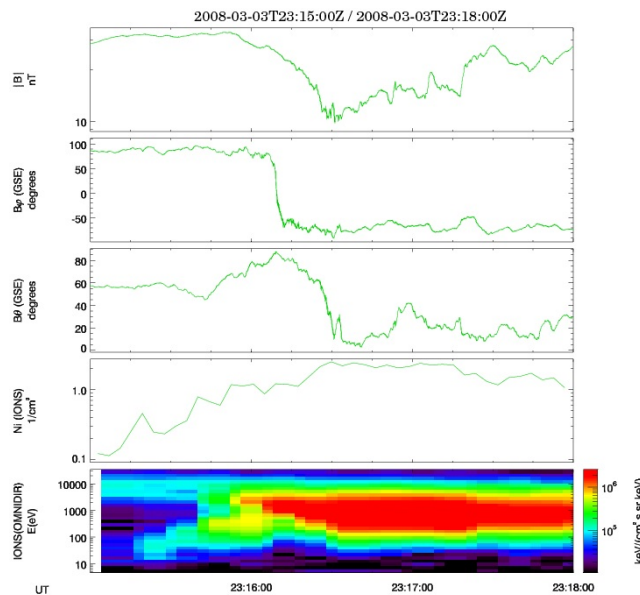
FIGURE 2.1 – Densité, spectrogramme d'énergie et champ magnétique observés par Cluster (C3) le 03 mars 2008 autour de 23 :15. Le changement de composition du plasma, les transitions en densité et en champ magnétique marquent la traversée de la frontière
