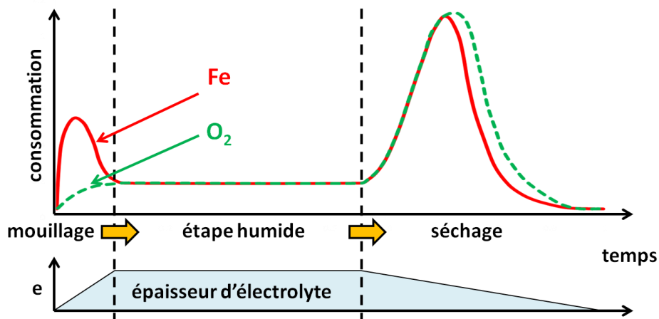
figure 26 : Évolutions de l'épaisseur de l'électrolyte en surface de la couche de produits de corrosion, et des consommations de fer et d'oxygène au cours d'un cycle de corrosion, selon Stratmann [138].
