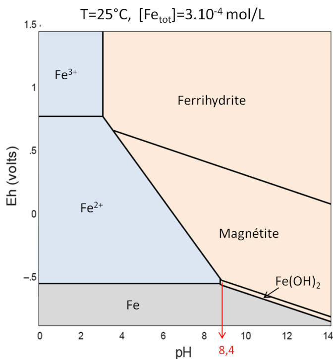
figure 112 : Diagramme de Pourbaix du système fer-eau à 25°C, avec [\text{Fe}]_{\text{tot}} = 3 \cdot 10^{-4} mol/L. Les domaines de stabilité de la goéthite et de la lépidocrocite ont été masqués pour faire apparaître celui de la ferrihydrite.
