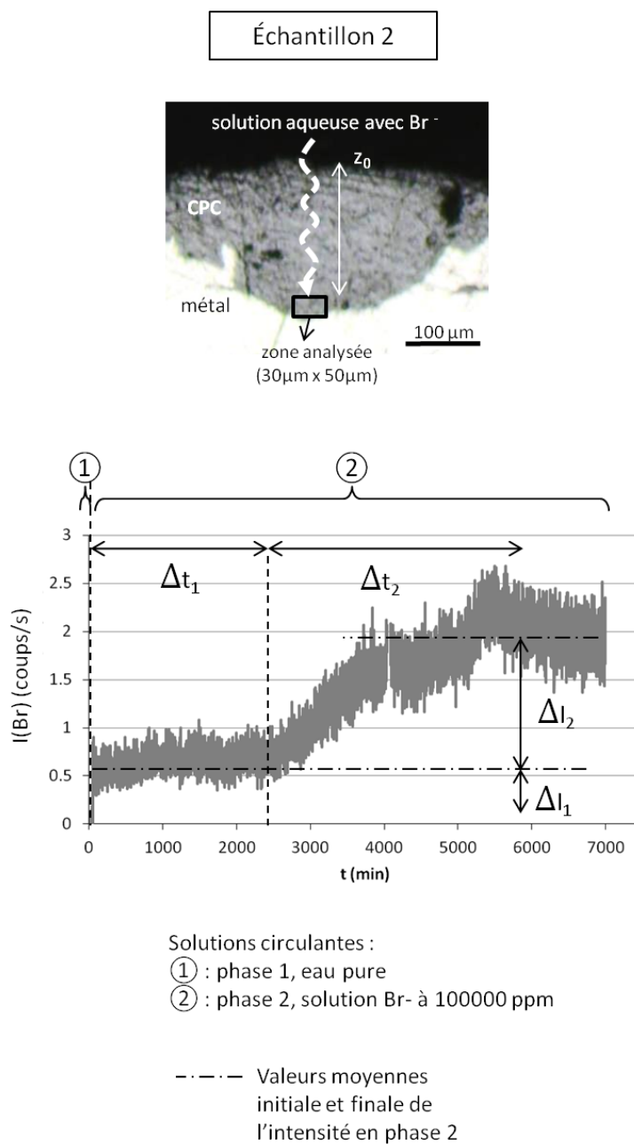
figure 121 : Micrographie de la zone sondée sur l'échantillon 3, et courbe correspondante de l'intensité du spectre de fluorescence intégrée sur la région correspondant au pic K\alpha du brome ( I(\text{Br}) ) en fonction du temps. Phase 1 : mesure du bruit de fond de I(\text{Br}) sur la couche de produits de corrosion (CPC) lorsque la solution circulante est de l'eau pure. Phase 2 : la solution circulante est la solution de KBr ; on observe une 1 ère phase de pénétration du brome dans la CPC avec une montée instantanée de I(\text{Br}) et un pseudo-plateau de durée \Delta t_1 , puis une 2 ème phase de pénétration du brome dans la CPC avec une montée de I(\text{Br}) lente, de durée \Delta t_2 , et l'atteinte d'une nouvelle valeur moyenne maximale de I(\text{Br}) . Les paramètres \Delta t_1 , \Delta t_2 , \Delta I_1 et \Delta I_2 sont donnés dans le tableau 17 (cf. Chap.3-C.1).
