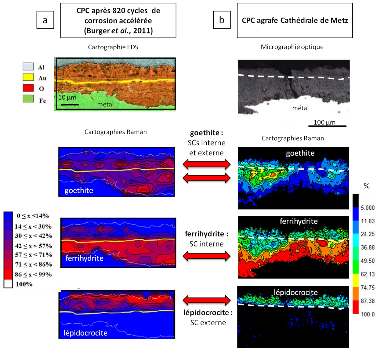
figure 105 : Comparaison de la structure en deux sous-couche et de la répartition des phases (cartographies en microspectroscopie Raman) constituant les couches de produits de corrosion (CPC) de deux systèmes. a : CPC formée sur un coupon de fer après 820 cycles de corrosion accélérée, d'après Burger et al. [125] ; b : CPC d'une agrafe de la cathédrale de Metz (500 ans). L'abréviation SC correspond à la locution "Sous-Couche".
