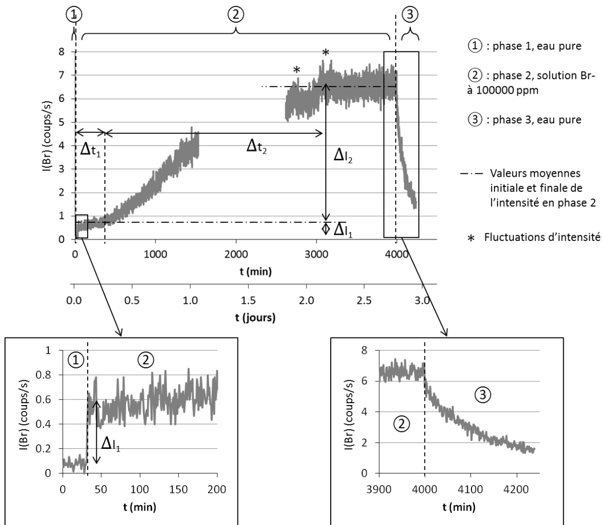
figure 84 : Courbe de l'intensité du spectre de fluorescence intégrée sur la région correspondant au pic \text{K}\alpha du brome ( I(\text{Br}) ) en fonction du temps. La zone sondée est celle représentée sur la figure 83 (échantillon 1). Phase 1 : mesure du bruit de fond de I(\text{Br}) sur la couche de produits de corrosion (CPC) lorsque la solution circulante est de l'eau pure. Phase 2 : la solution circulante est la solution de KBr ; on observe une 1 ère phase de pénétration du brome dans la CPC avec une montée instantanée de I(\text{Br}) et un pseudo-plateau de durée \Delta t_1 , puis une 2 ème phase de pénétration du brome dans la CPC avec une montée de I(\text{Br}) lente, de durée \Delta t_2 , et l'atteinte d'une nouvelle valeur moyenne maximale de I(\text{Br}) ; l'interruption de la courbe est due à un problème technique. Phase 3 : la solution de KBr est remplacée par de l'eau pure ; la CPC se vide rapidement du brome. Les paramètres \Delta t_1 , \Delta t_2 , \Delta I_1 et \Delta I_2 sont donnés dans le tableau 17 pour les 3 échantillons sur lesquels des expériences de transport ont été menées.
