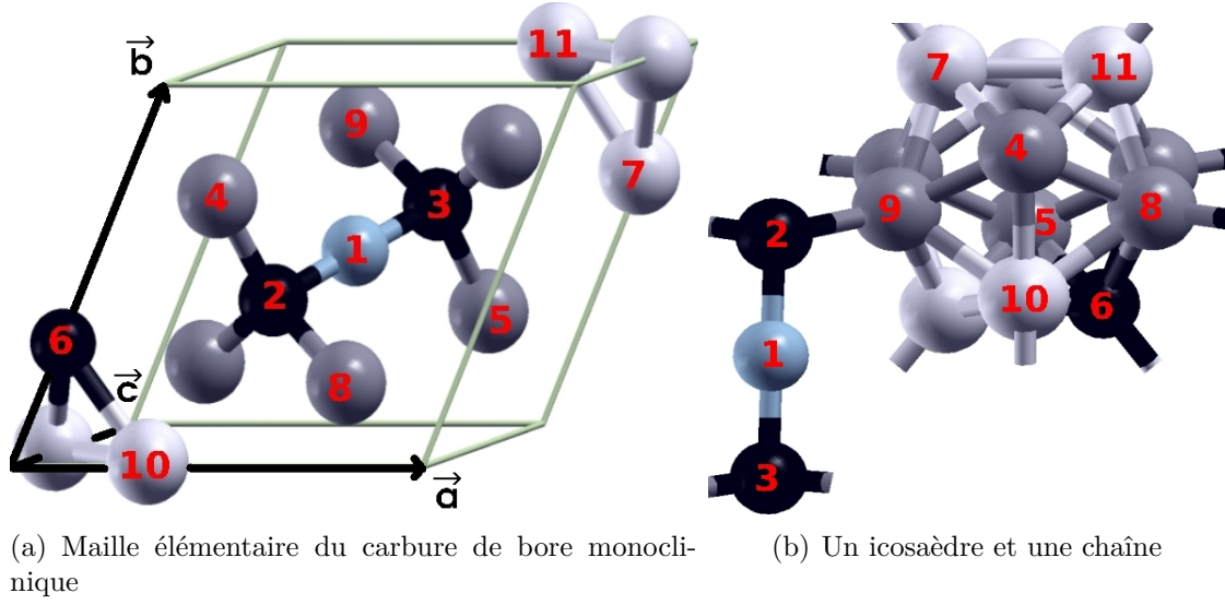
FIG. A.1 – Maille élémentaire du carbure de bore monoclinique base-centrée. Boule bleue (1) : atome bore de centre de chaîne. Boule noire (2,3,6) : atome carbone à une extrémité de chaîne ou en site polaire de l'icosaèdre. Boule blanche (7,10,11) : atome de bore en site polaire. Boule grise (4,5,8,9) : atome de bore en site équatorial.
