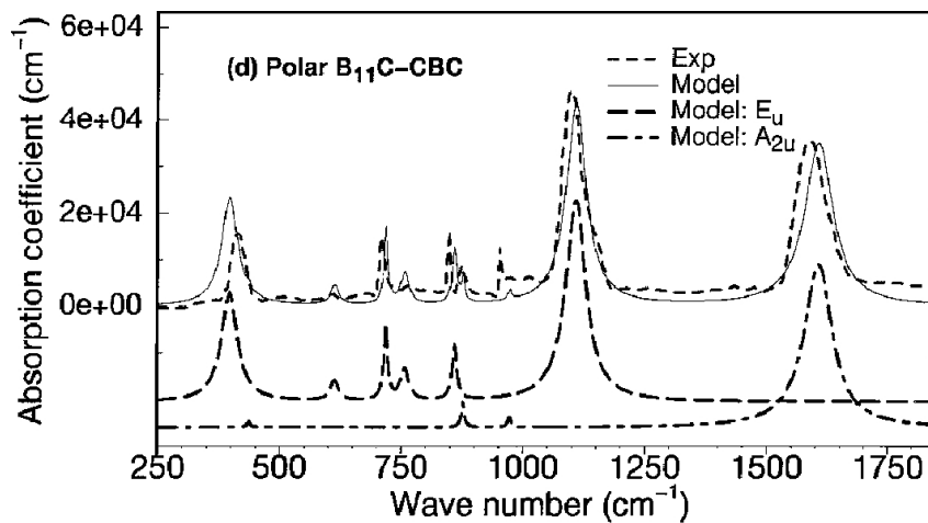
FIG. 2.12 – Spectre d'absorption infrarouge expérimental de B_{4.3}C [223] et spectre théorique de (B_{11}C^p)C-B-C [4, 209] obtenu en DFT-LDA.
