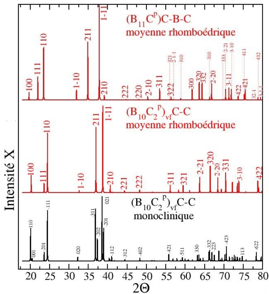
FIG. B.4 – Spectres de diffraction des rayons X du carbure de bore B_4C et du matériau monoclinique (B_{10}C_2^p)_{vf}C-C ainsi que sa moyenne rhomboédrique. Les valeurs des angles et des intensités sont données Tab. B.14.
