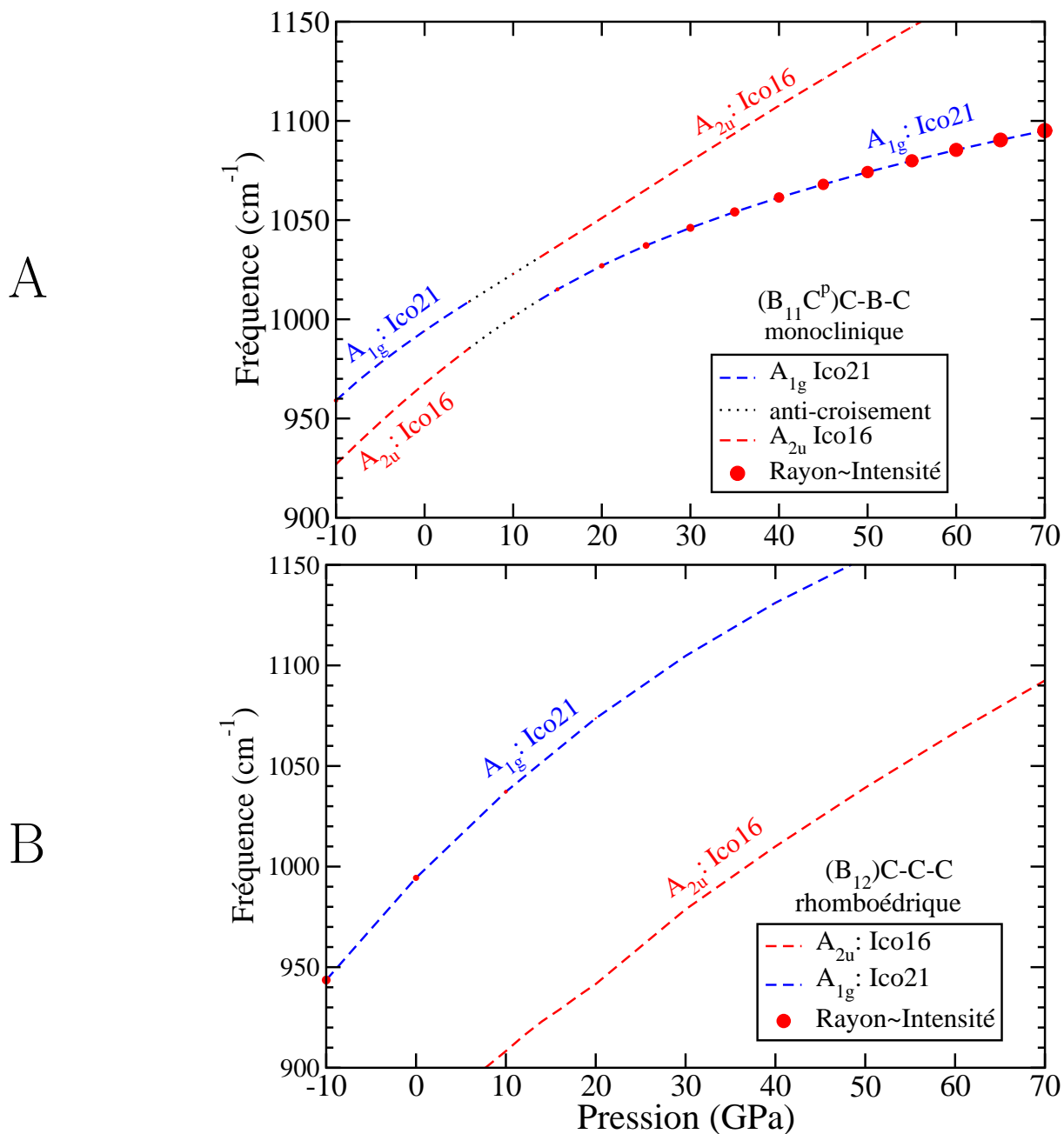
FIG. 4.12 – Apparition de mode. de ( B_{11}C^p )C-B-C en fonction de la pression pour le mode de respiration de l'hexagone équatorial Ico21 . Panel A : anti-croisement (en pointillé) des modes Ico21 et Ico16 en symétrie monoclinique. Panel B : comportement sous pression des modes Ico21 et Ico16 en symétrie rhomboédrique.
