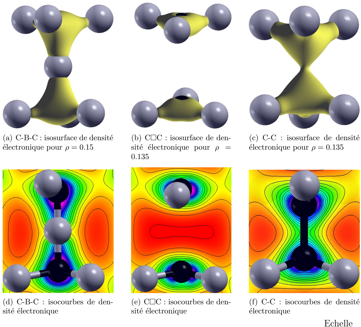
FIG. 1.12 – Densité électronique des chaînes C-B-C, des chaînes C-C et des arrangements C□C. Boules noires : atomes de carbone. Boules grises : atomes de bore localisés sur un site équatorial. Dans cet exemple, les chaînes et arrangements proviennent des mailles rhomboédriques (B_{12})C-B-C , (B_{12})C-C et (B_{12})C□C .
