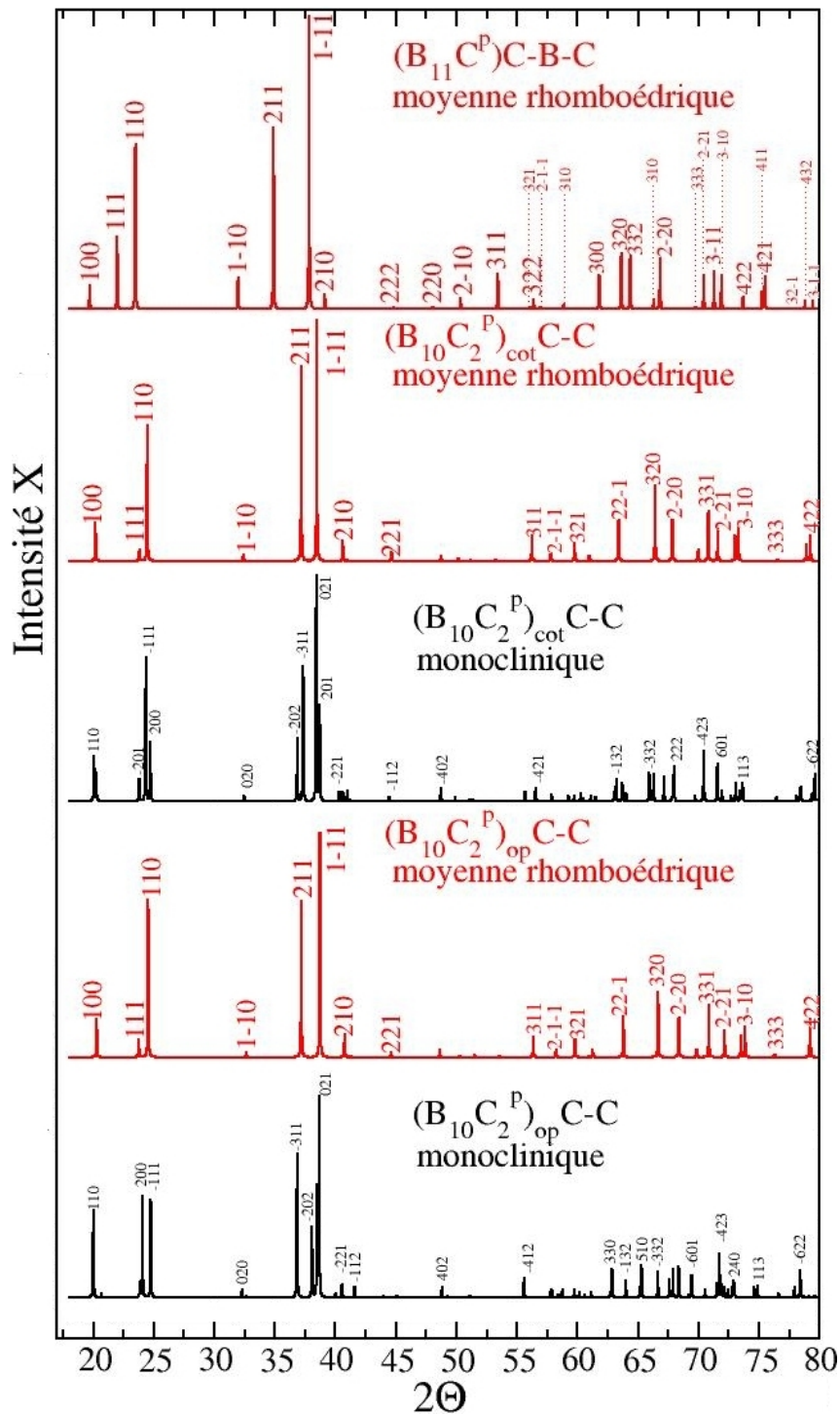
FIG. B.3 – Spectres de diffraction des rayons X du carbure de bore B_4C et des matériaux monocliniques (B_{10}C_2^p)_{cot}C-C et (B_{10}C_2^p)_{op}C-C ainsi que leur moyenne rhomboédrique. Les valeurs des angles et des intensités sont données Tab. B.14.
