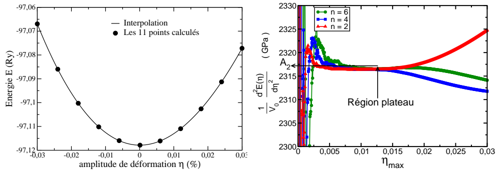
(a) Variation de l'énergie en fonction de l'amplitude de déformation. Les onze points noirs correspondent aux calculs en DFT-GGA. La courbe est l'interpolation par la « cubic spline ». (b) Variation des termes d'ordre 2 ( A_2 ) des polynômes approximateurs d'ordre n en fonction de l'amplitude maximale de déformation imposée. La région plateau est indiquée.
