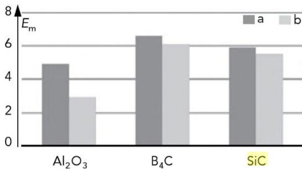
FIG. 1.4 – Efficacité balistique des céramiques. a) Vis-à-vis d’un projectile 7,62 à noyau en acier dur. b) Vis-à-vis d’un projectile 7,62 à noyau en carbure de tungstène. Origine : Réf. [21]
