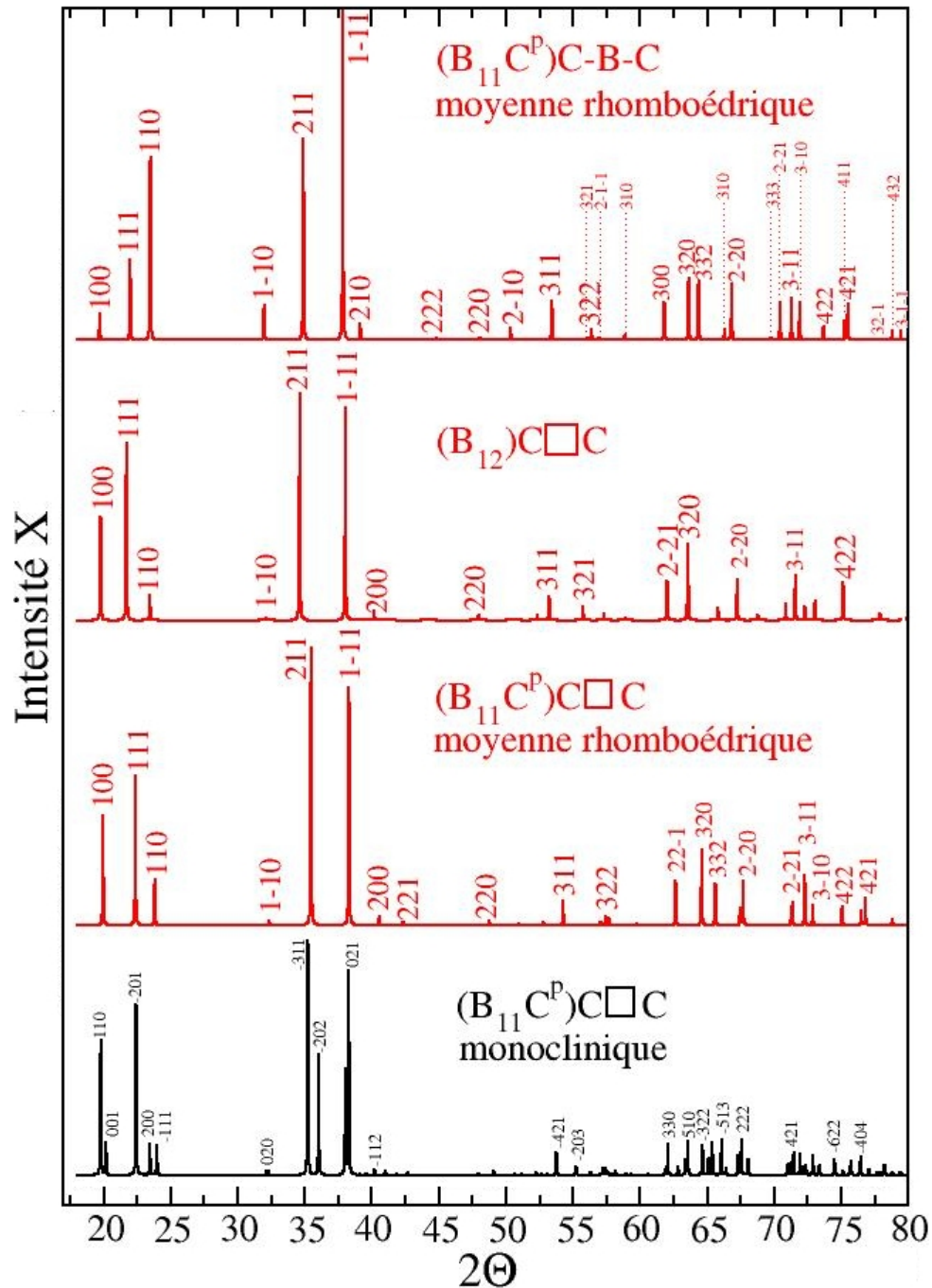
FIG. B.1 – Spectres de diffraction des rayons X du carbure de bore et des matériaux concurrents à arrangements C\Box C (B_{12})C\Box C et (B_{11}C^p)C\Box C ainsi que de sa moyenne rhomboédrique. Les valeurs des angles et des intensités sont données Tab. B.13.
