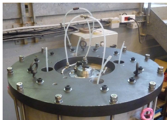
Figure 2-28 – Vue du couvercle de la chambre d'étalonnage installé sur l'enceinte de confinement
