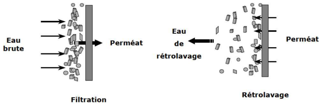
Figure 1-28 – Représentation schématisée des procédés de filtration et de rétrolavage (Rémize, 2006)
