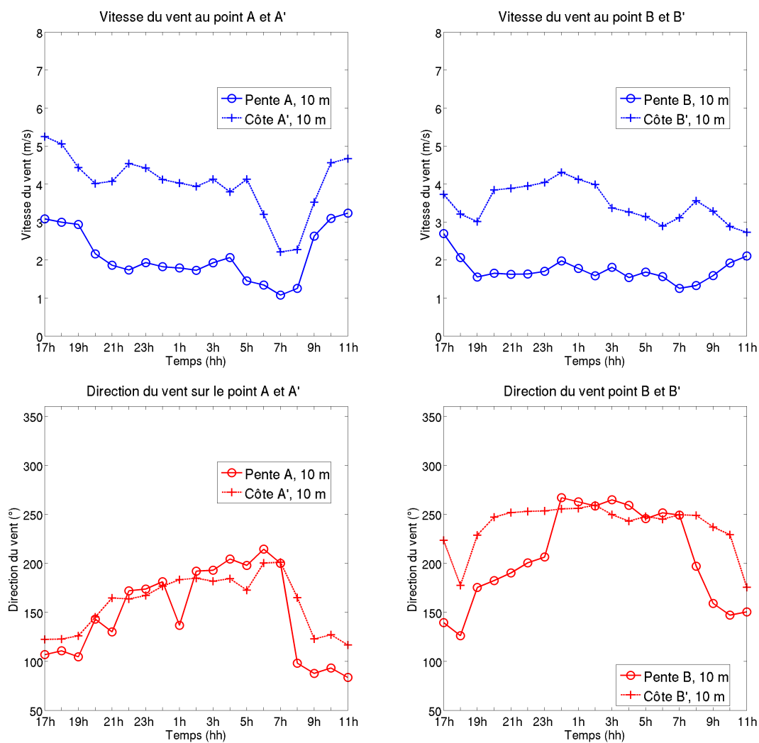
FIGURE 7.13 : (a) Cycle diurne de la vitesse du vent en m/s à 10 m au Nord sur les pentes (point A) et sur la côte (point A') et à l'Est sur les pentes (point B) et sur la côte (point B') (b) de même pour le cycle diurne de la direction du vent à 10 m (°). Cas du 07/01/2012.
