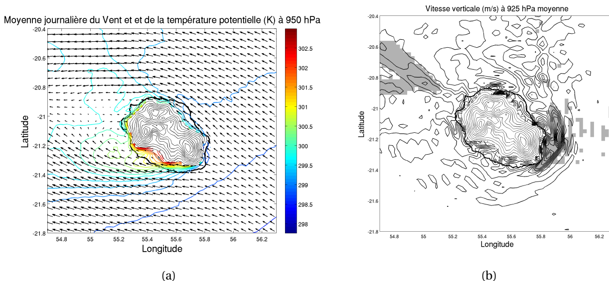
FIGURE 8.18 : (a) Champ du vent horizontal moyen sur la journée et de la température potentielle (K) moyenne à 950 hPa, (b) Vitesse verticale moyenne sur la journée à 925 hPa représentée par les contours noirs de 0,025 m/s. Les zones grisées correspondent aux zones de soulèvement de la couche limite atmosphérique en moyenne sur la journée : Le 07/01/2012. La topographie est représentée par un contour avec un intervalle de 250 m.
