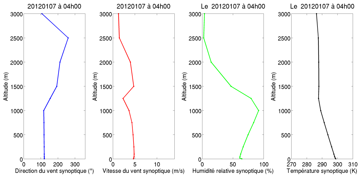
FIGURE 7.11 : De gauche à droite : profil de la direction du vent ( ^{\circ} ), profil de la vitesse du vent (m/s), profil d'humidité relative (%) et profil de température (K) calculés sur le domaine 1. Cas du 07/01/2012.
