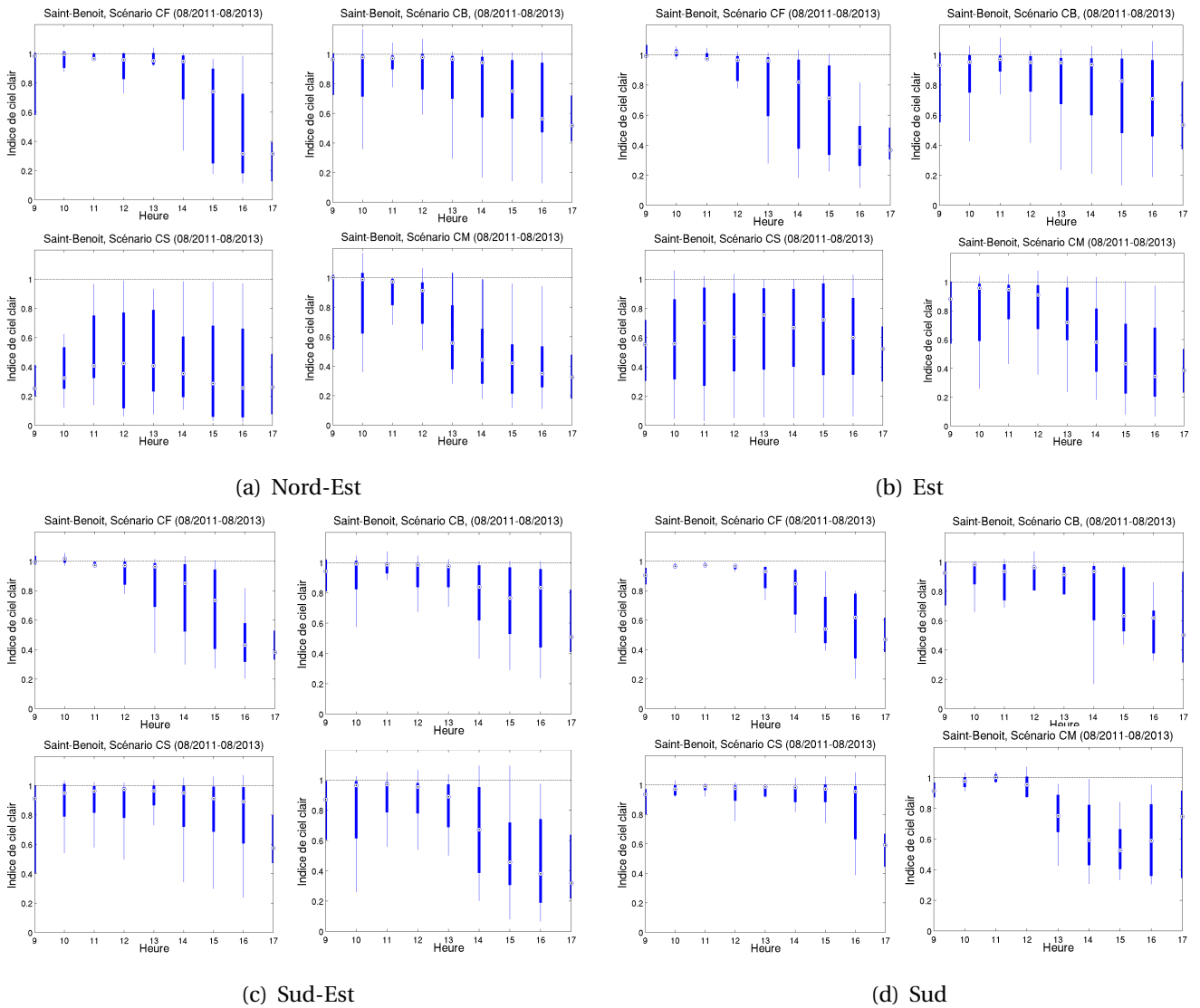
FIGURE 8.8 : Variabilité du cycle diurne de K_{t_{obs}} sur la station de Saint-Benoît pour les différents régimes d'ennuagement de nuit, CF, CB, CS, CM pour des régimes de vent de (a) Nord-Est, (b) d'Est, (c) de Sud-Est et (d) de Sud. Le point représente le 50 e centile, la barre épaisse représente le 25 e et 75 e centile et la barre fine le 5 e et 95 e centile.
