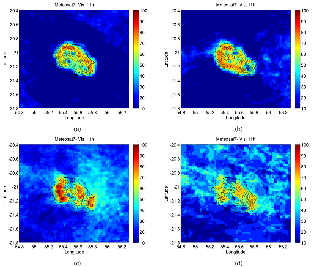
FIGURE 8.28 : Fréquence de Kt_{sat} à 11h00 pour (a) des vitesses de vents synoptiques faibles ( v < 4 m/s à 1000 hPa et de même à 900 hPa), (b) des vitesses de vents synoptiques moyens ( 5 m/s \leq v < 7 m/s à 1000 hPa et de même à 900 hPa), (c) des vitesses de vents synoptiques forts ( 8 \leq v < 10 m/s à 1000 hPa et de même à 900 hPa) et (d) des vitesses de vents synoptiques très forts ( v > 10 m/s à 1000 hPa et de même à 900 hPa). Les vitesses sont prises à partir des réanalyses ERA-Interim. La topographie est représentée par un contour avec un intervalle de 250 m.
