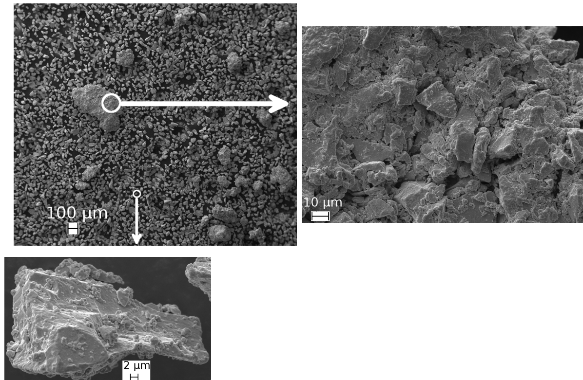
FIGURE VI.13 – Vues au MEB de la poudre revêtue, à différents agrandissements.
