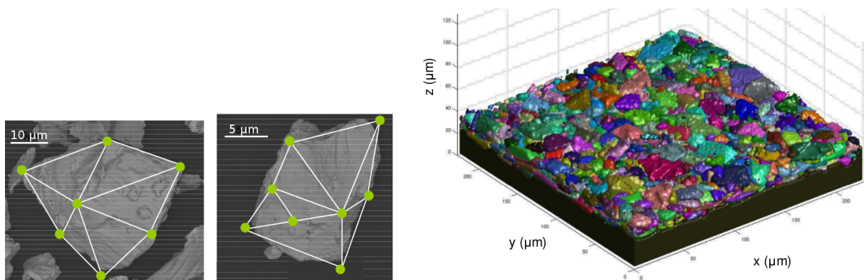
FIGURE I.18 – A gauche, modélisation des particules par individuation des sommets et triangulation. A droite, exemple d'un dépôt obtenu par simulation numérique (24 couches, taux de rebonds de 33 %) (tirées de [45]).
