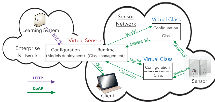
Figure 6.14: Concept d'architecture du Capteur Virtuel et de ses Classes Virtuelles avec les informations échangées durant l'exécution.
