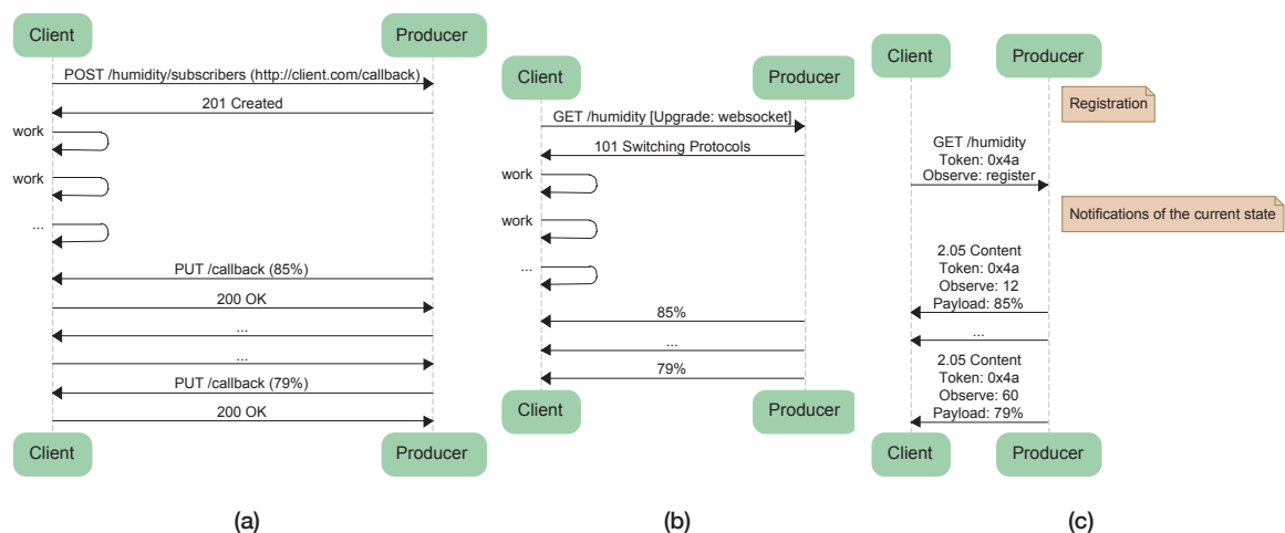
Figure 6.6: Diagrammes de séquences utilisant HTTP et CoAP. (a) le HTTP callback transforme le client en un serveur exposant une ressource de rappel. (b) HTTP est uniquement utilisé pour initier une WebSocket qui va se transformer en une connexion TCP bi-directionnelle. (c) les clients peuvent observer et être notifiés par une réponse CoAP contenant la nouvelle représentation.
