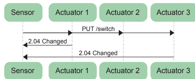
Figure 6.5: Avec la communication de groupe offerte par CoAP, un client peut interagir simultanément avec plusieurs ressources. Le capteur dans cet exemple est captable de contrôler les actionneurs 1 et 3 appartenant au même groupe. Les dispositifs ne faisant pas partie du groupe ne considèrent pas les messages (actionneur 2).
