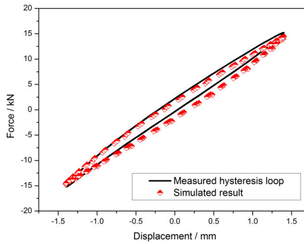
(b) f=2\text{Hz} A=1.4\text{mm}
