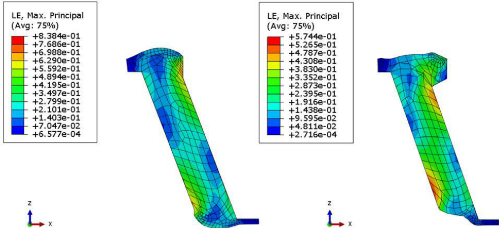
(d) The maximum principle strain (LE, Max. Principal)
