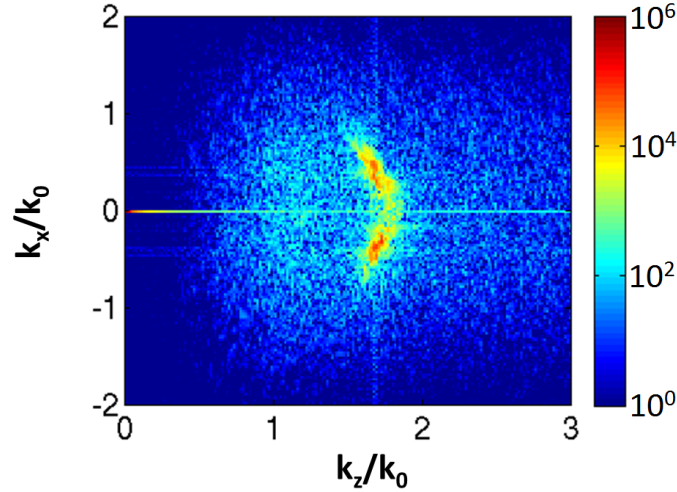
FIGURE V.3.11 – Spectre dans le plan k_z - k_x des fluctuations électroniques |n_e|^2 intégrées sur la portion z=[32; 96]\mu\text{m} et x=[-28; -12]\mu\text{m} à t=1.48 ps correspondant au maximum de l'instabilité Raman du speckle fort. On observe la présence de modes transverses dus au bowing de l'EPW.
