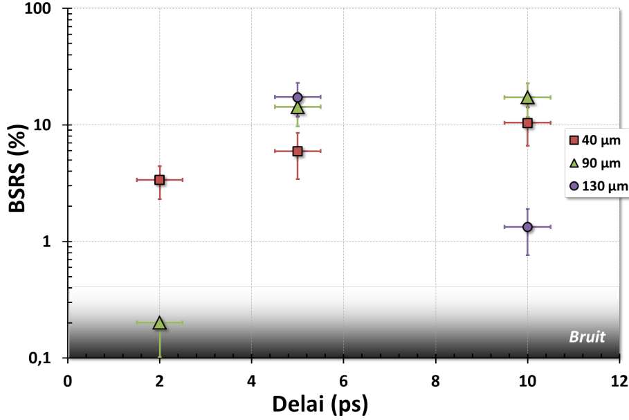
FIGURE V.4.2 – Courbe de réflectivité du speckle faible en configuration bispeckle polarisations croisées pour plusieurs espacements latéraux.
