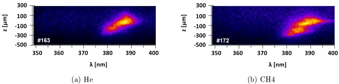
FIGURE VI.1.2 – Spectres Thomson résolus longitudinalement en configuration lissée par RPP pour les deux gaz à la même intensité.
