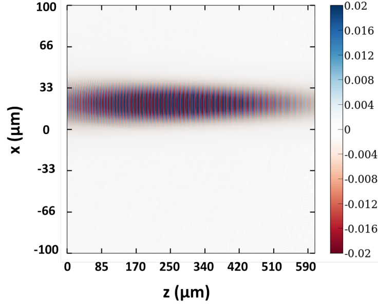
FIGURE V.3.4 – Champ E_y associé au speckle faible mesurée à 4.15 ps. L'onde laser du speckle faible se propage dans le plasma sans perturbation majeure.
