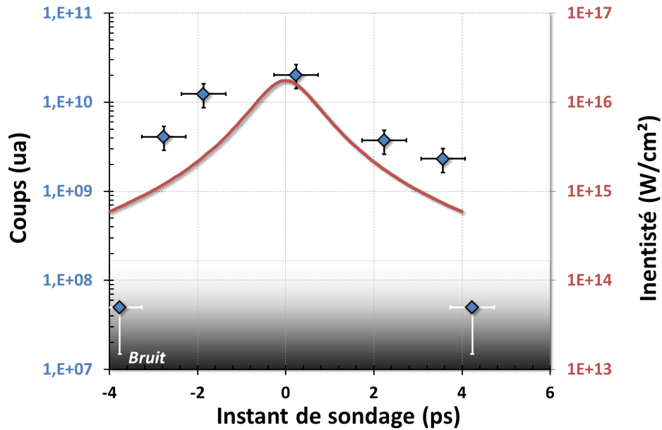
FIGURE IV.1.3 – Évolution de l'instabilité Raman (points bleus) et de l'impulsion d'interaction (courbe rouge) en fonction du temps.
