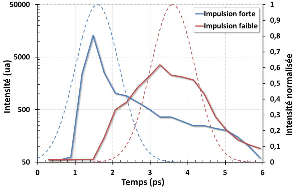
FIGURE V.3.19 – Intensité du spectre en k_z associée au Raman des deux speckles au cours du temps, mesurée à la position z = [32; 96] \mu\text{m} , intégrée sur l'intervalle [1.2; 1.9] k_0 et \Delta x = 10 \mu\text{m} de part et d'autre du centre respectif de chacun des speckles. Les courbes en pointillés présentent l'évolution des deux impulsions laser au cours du temps.
