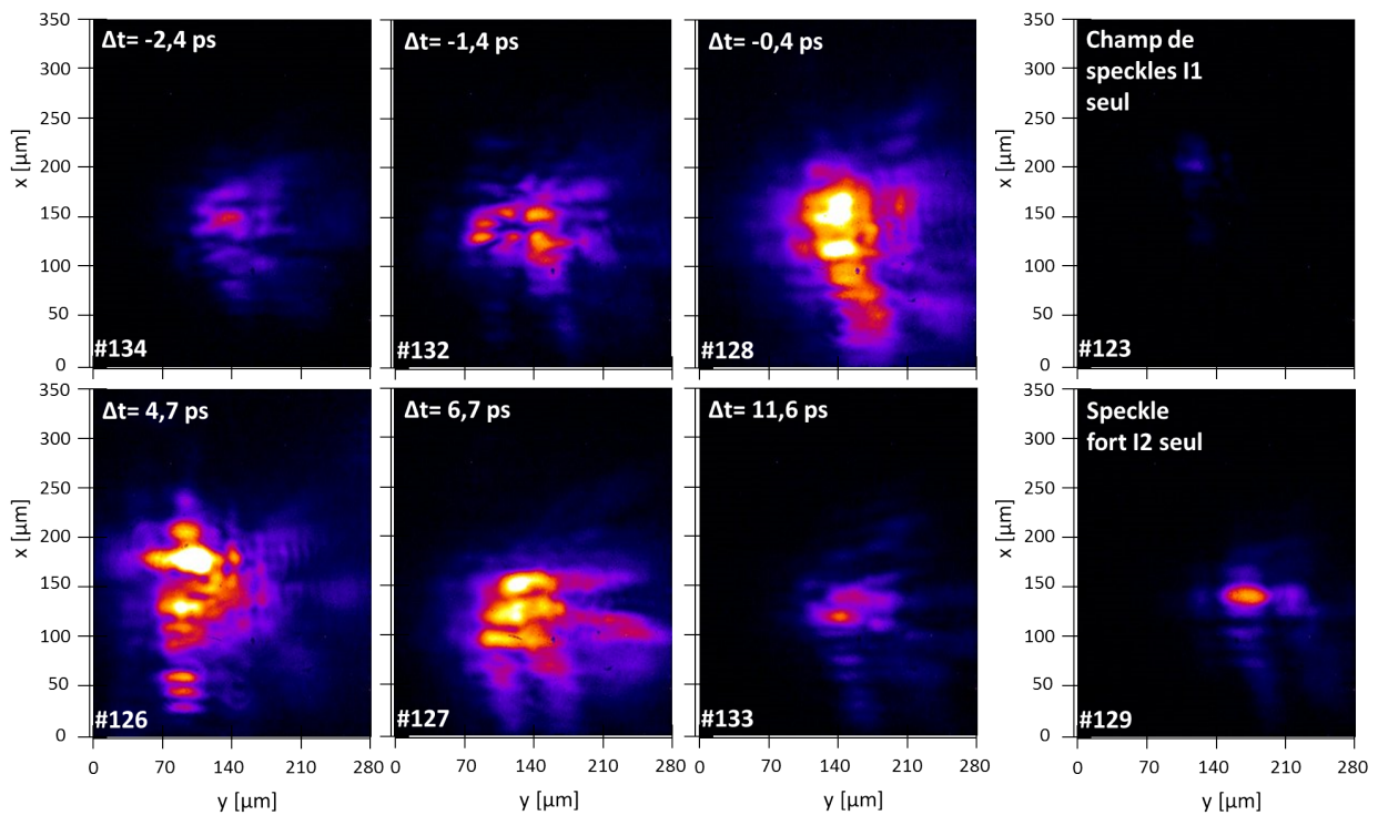
FIGURE VI.2.2 – Images de rétrodiffusion d'un speckle fort focalisé dans un champ de speckles faibles et images de référence.
