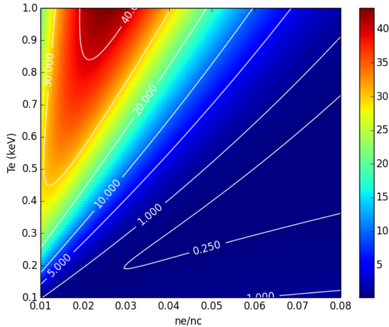
FIGURE V.2.5 – Amortissement des ondes plasma électroniques \nu_2 = \nu_L + \nu_{ei}/2 en \text{ps}^{-1} selon la densité et la température électronique.
