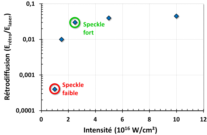
FIGURE II.3.4 – Courbe de réflectivité monospeckle en fonction de son intensité (Yin et al., 2012) obtenue à l'aide de simulations 2D d'ouverture f/4 , \lambda_0 = 351 nm, k_2\lambda_D = 0.34 . Les intensités des deux speckles utilisés dans la configuration bispeckle sont également indiquées.
