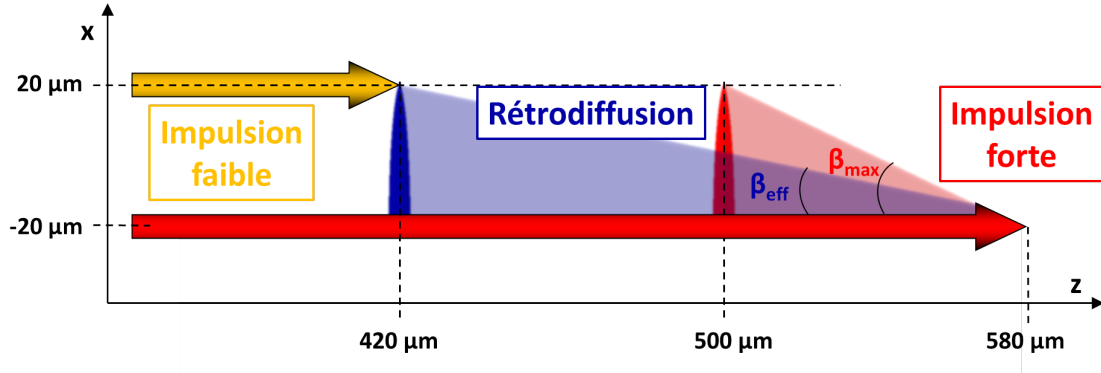
FIGURE V.3.18 – Représentation schématique de la rétrodiffusion de l’impulsion forte dans la simulation CALDER, avec la présence d’un cône de rétrodiffusion contenant la majorité de l’énergie rétrodiffusée et un cône contenant les ondes minoritaires diffusées à grand angle avec le bowing de l’EPW.
