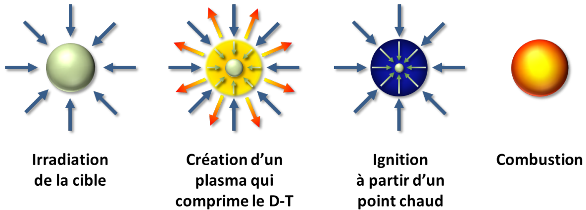
FIGURE I.2.1 – Schéma du principe de la fusion par confinement inertiel.
