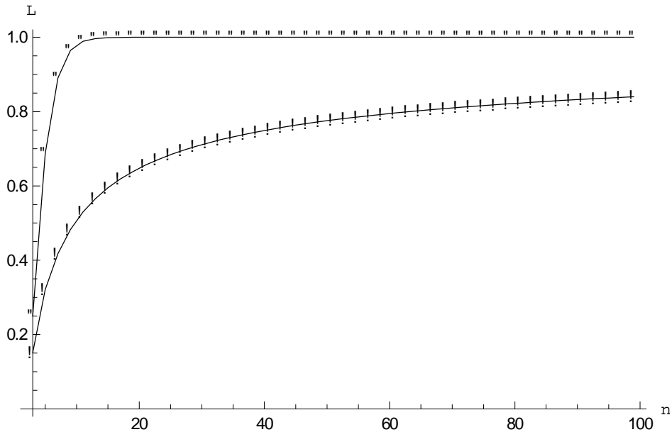
FIGURE 3: Comparaison de la violation de L (75) par jS(n, \frac{n}{2})_i ( n ) et jW_n_i ( l ) en fonction de n (le nombre de parties).
