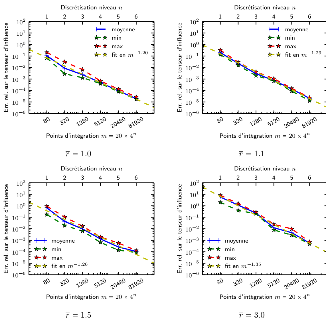
FIGURE 2.4 – Erreur relative sur le tenseur d'influence de deux sphères
