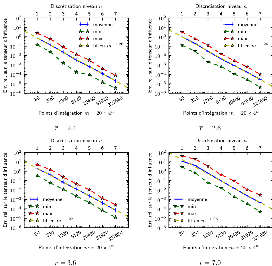
FIGURE 2.5 – Erreur relative sur le tenseur d'influence de deux ellipsoïdes allongés
