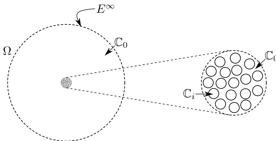
FIGURE 1.3 – Schéma de la microstructure considérée pour le calcul aux éléments finis.
