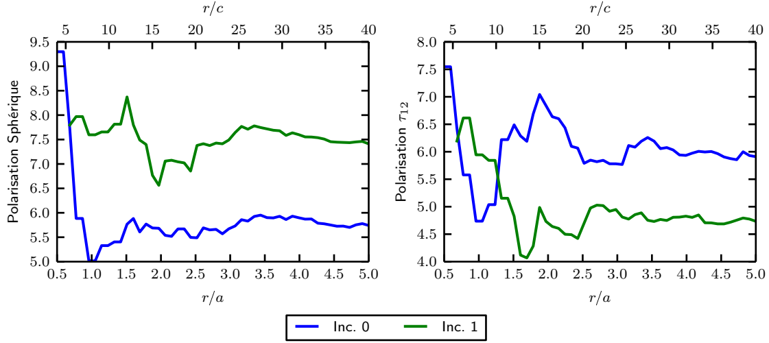
FIGURE 2.17 – Polarisations sphériques \tau_{ii}/3 sous chargement sphérique \mathbf{E} = \underline{e}_i \otimes \underline{e}_i (gauche) et déviatorique \tau_{12} sous chargement \mathbf{E} = \underline{e}_1 \otimes^s \underline{e}_2 (droite) en fonction de la taille du voisinage r . Les courbes sont relatives aux deux inclusions (0) et (1) les plus proches du centre de l’amas. Les chargement et les résultats sont définis dans le repère global. La distance de transition est : r_0 = 4a .
