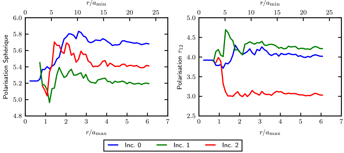
FIGURE 2.11 – Polarisations sphériques \tau_{ii}/3 sous chargement sphérique \mathbf{E} = \underline{e}_i \otimes \underline{e}_i (gauche) et déviatorique \tau_{12} sous chargement \mathbf{E} = \underline{e}_1 \otimes^s \underline{e}_2 (droite) en fonction de la taille du voisinage r . Les courbes sont relatives à l'inclusion centrale (0) et les deux inclusions les plus proches (1) et (2).
