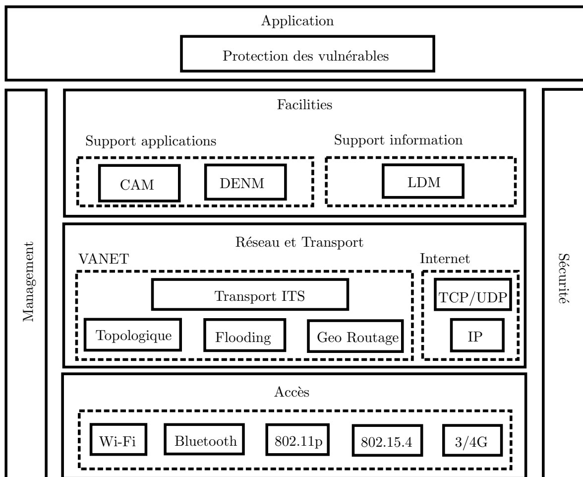
FIGURE 4.1: Architecture du système de communication véhiculaire
