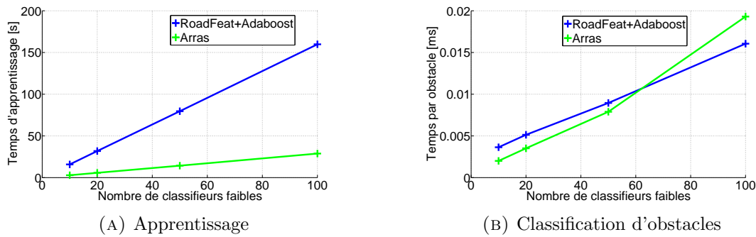
FIGURE 6.5: Temps de traitement
