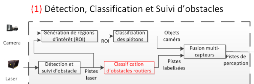
FIGURE 3.6: Architecture du système de perception des usagers vulnérables
