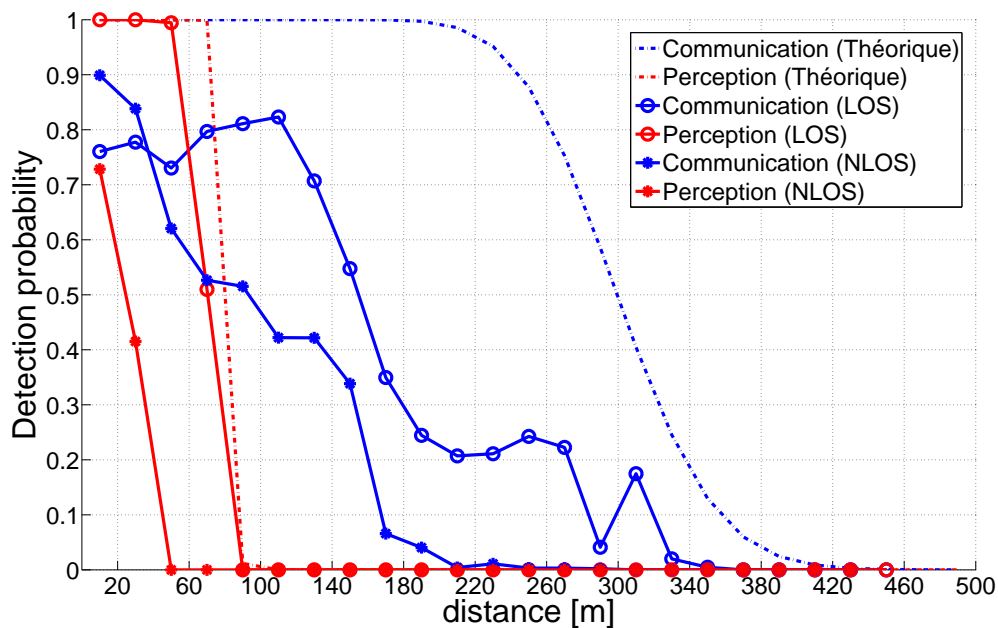
FIGURE 6.15: Capacité de détection des systèmes de perception et de communication dans des conditions LOS et NLOS.
