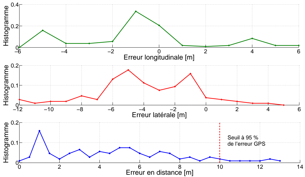
FIGURE 6.12: Histogramme des erreurs GPS en position longitudinale et latérale, et en distance
