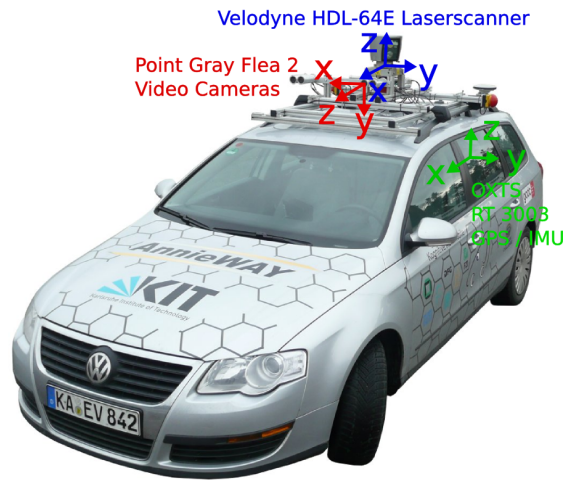
FIGURE 6.1: Illustration du véhicule employé pour l'acquisition des données de la base Kitti
