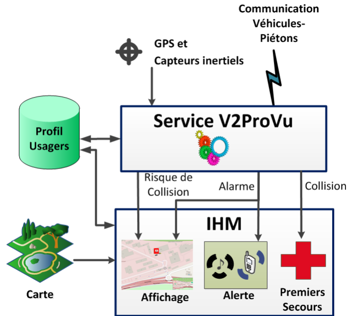
FIGURE 5.10: Description de l'application V2ProVu
