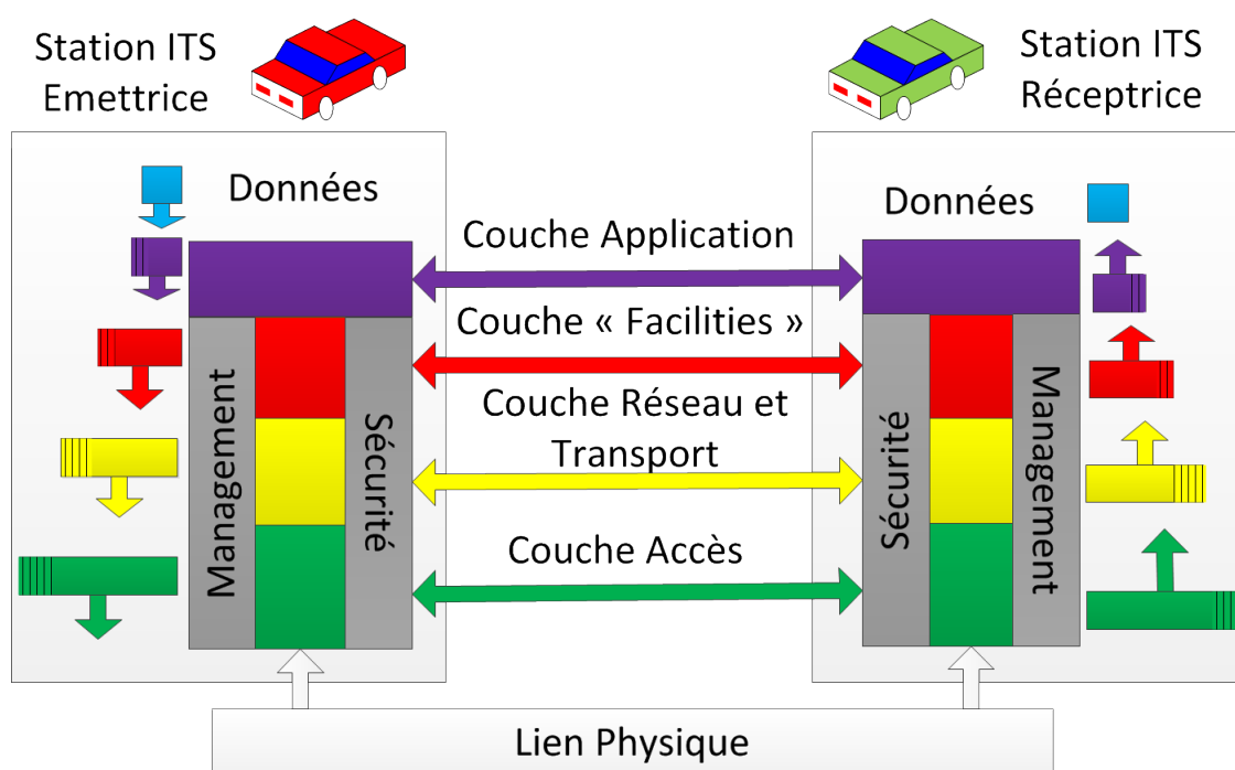
FIGURE 2.6: Modèle en couches pour la communication véhiculaire
