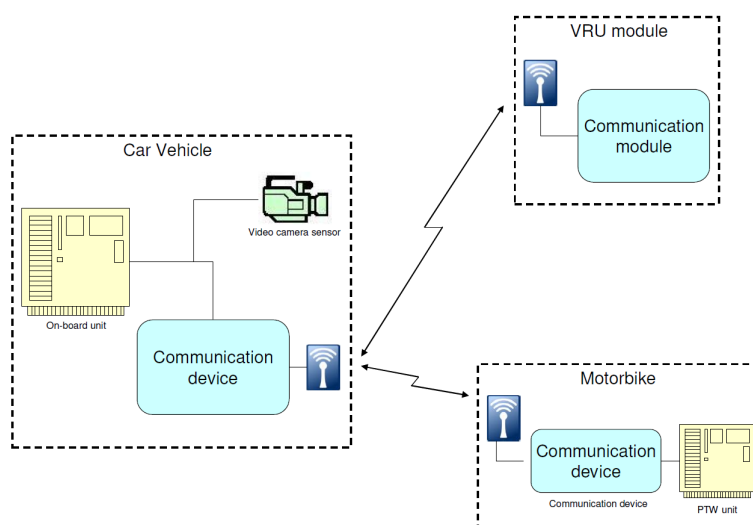
FIGURE 2.9: Architecture générale du projet WATCH-OVER
