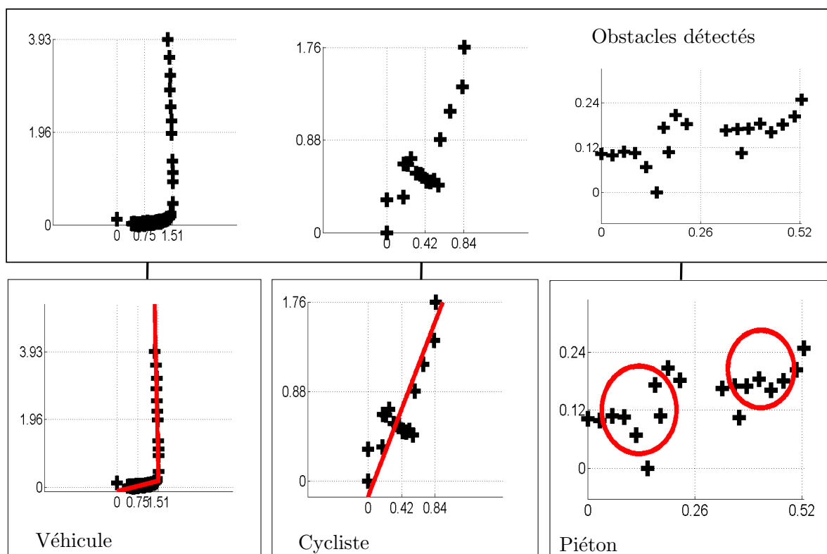
FIGURE 3.13: Illustration des caractéristiques des objets détectés par laser
