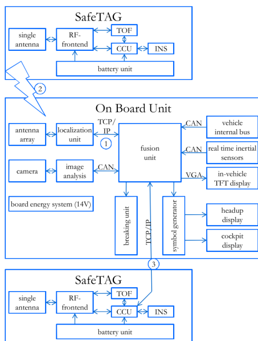
FIGURE 2.10: Architecture générale du projet Ko-TAG
