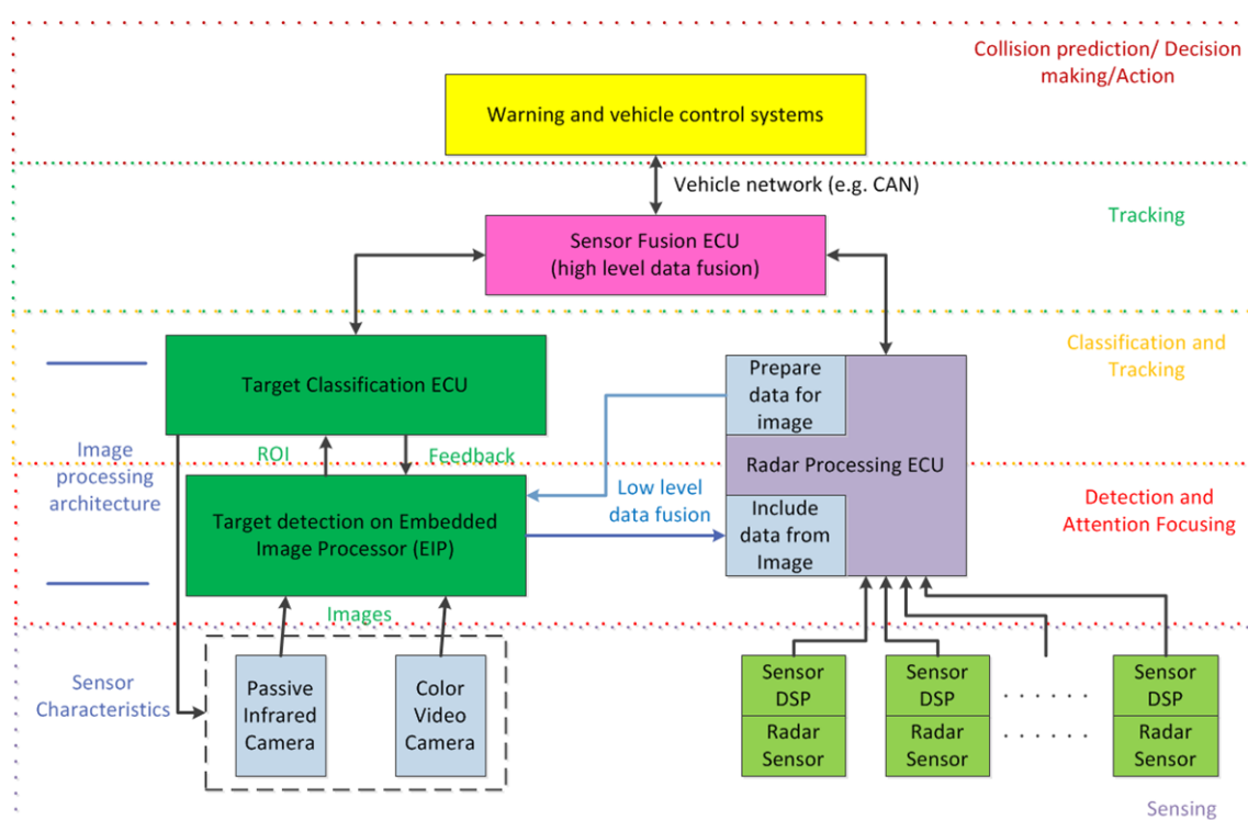
FIGURE 2.8: Architecture générale du projet SAVE-U
