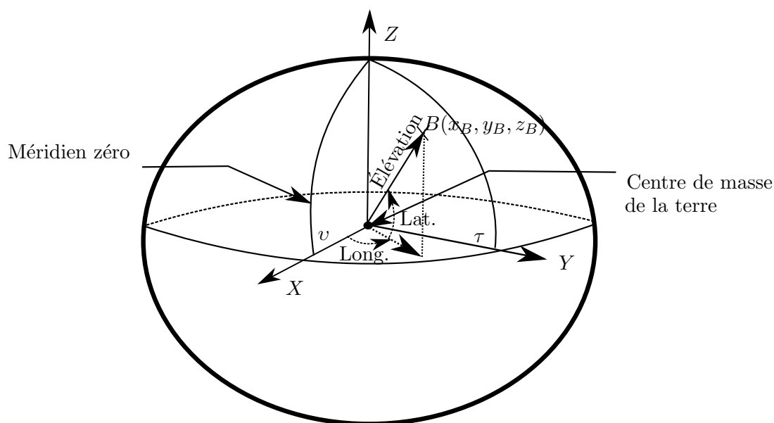
FIGURE 5.1: Système géodésique mondial
