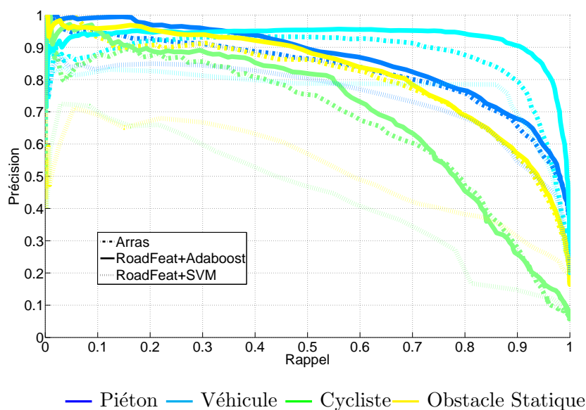
FIGURE 6.6: Précision-Rappel
