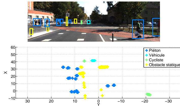
FIGURE 6.4: Exemple de scan laser 2D annoté. Les impacts laser ainsi que les boîtes englobantes des objets sont projetés dans l'image correspondante à la scène.
