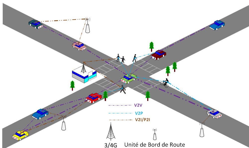
FIGURE 2.5: Scénario de communication véhiculaire
