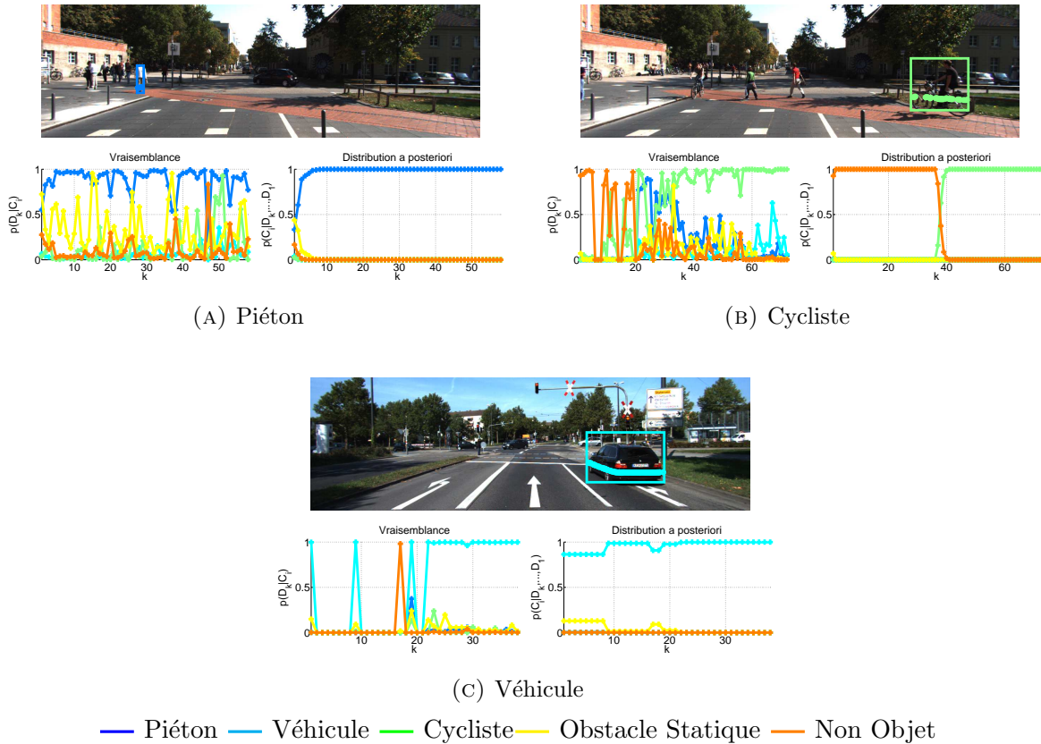
FIGURE 3.14: Exemples de classification de pistes
