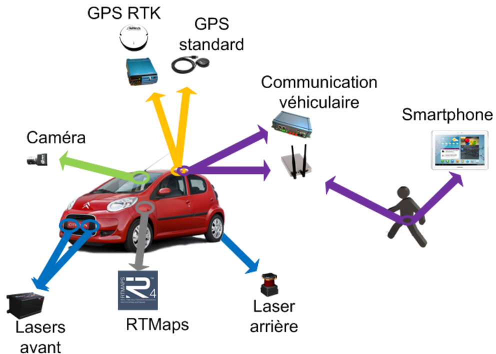
FIGURE 6.2: Illustration de la plateforme INRIA et de l'équipement porté par le piéton
