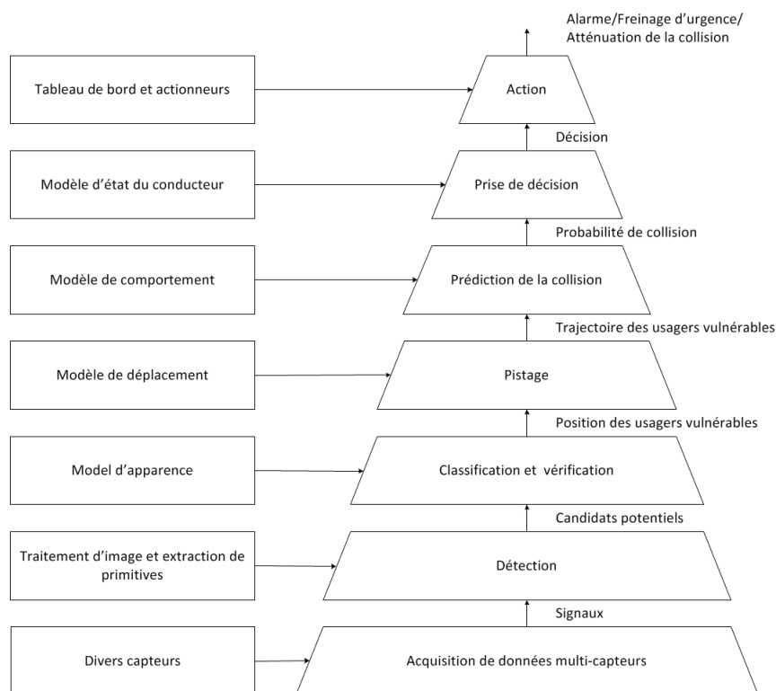
FIGURE 3.1: Système de protection des usagers vulnérables basé sur la perception
