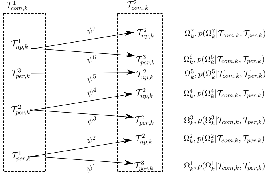
FIGURE 5.6: Hypothèses d'association établies depuis la Figure 5.5
