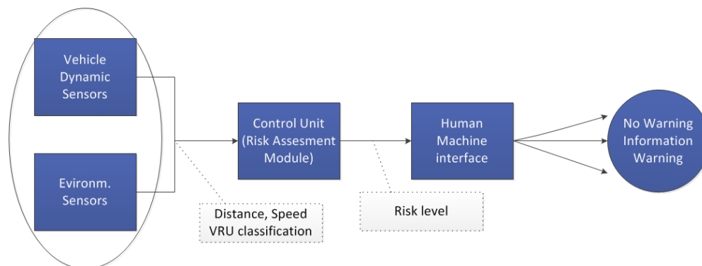
FIGURE 2.7: Architecture générale du projet PROTECTOR
