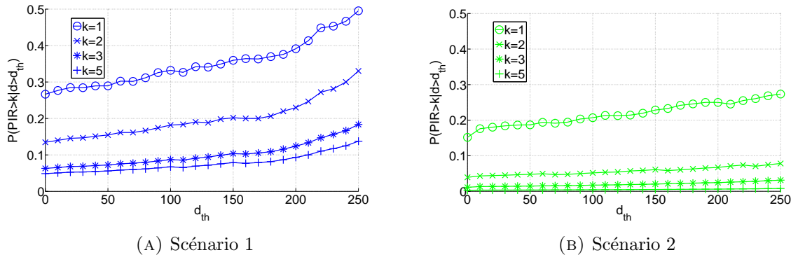
FIGURE 6.11: Probabilité de ne pas recevoir plus de k paquets consécutifs
