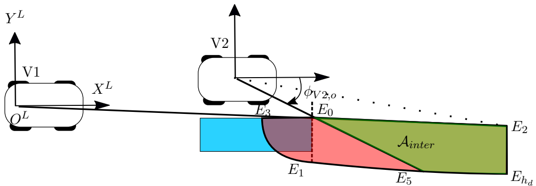
FIGURE 4.8: Illustration du calcul du minuteur pour le routage géographique
