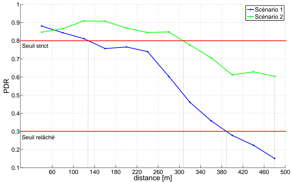
FIGURE 6.10: Taux de réception correcte des paquets (PDR)
