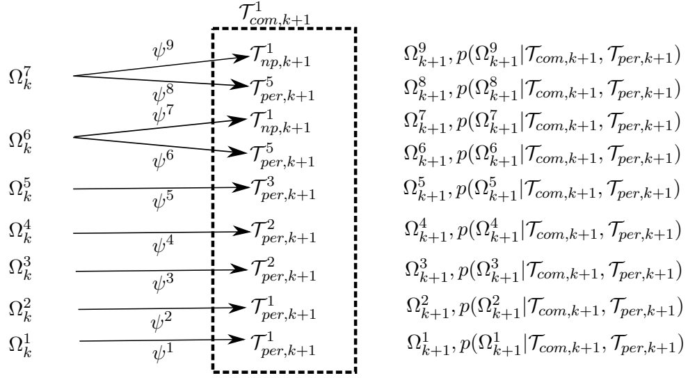
FIGURE 5.8: Evolution temporelle des hypothèses d'association
