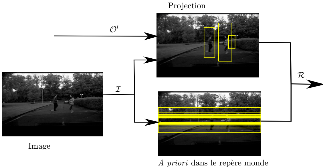
FIGURE 3.8: Génération de ROIs pour la classification de piétons
