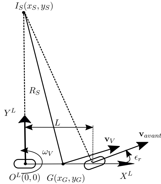
FIGURE 4.4: Modèle bicyclette
