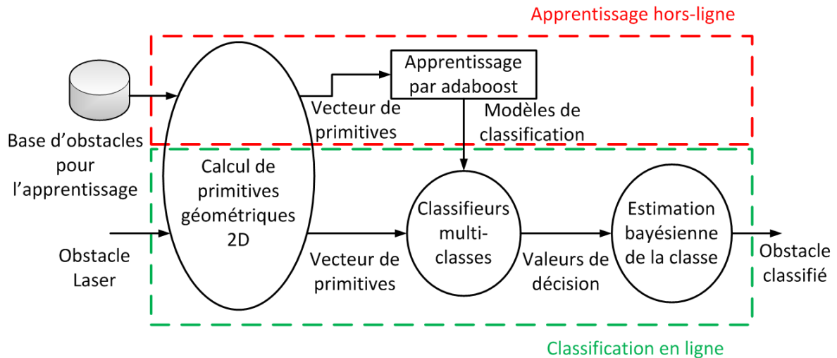
FIGURE 3.12: Classification multi-classes d'obstacles routiers par capteur laser
