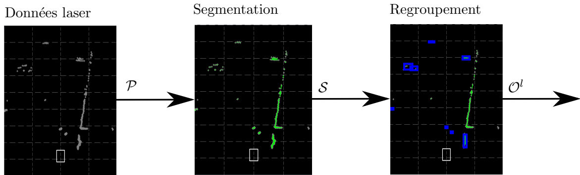
FIGURE 3.7: Détection d'obstacles par capteur laser
