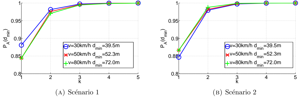
FIGURE 6.13: Probabilité d'être informé à la distance d_{min}
