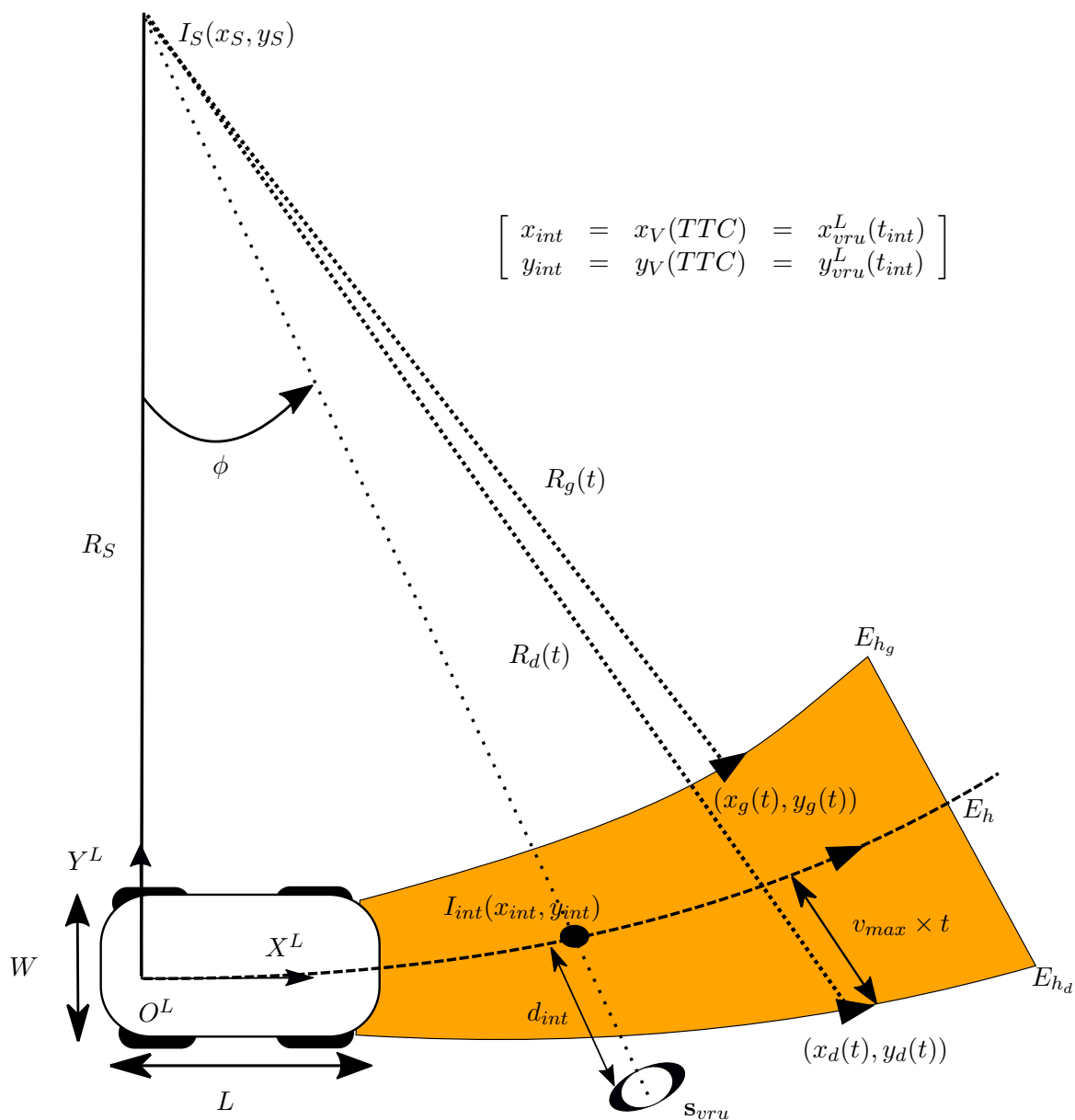
FIGURE 4.6: Définition de la GDA
