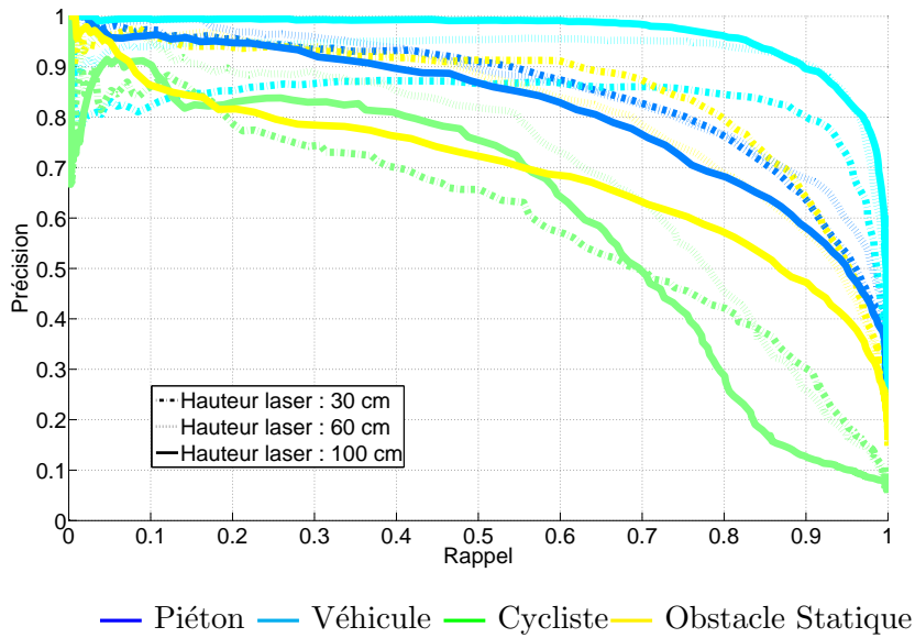
FIGURE 6.8: Précision-Rappel en fonction de la hauteur du laser
