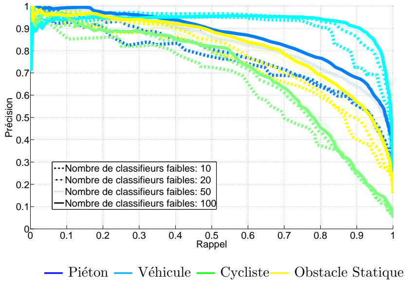
FIGURE 6.7: Précision-Rappel en fonction du nombre de classifieurs faibles
