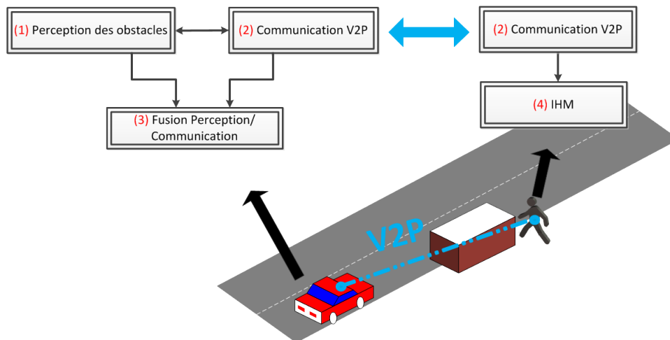
FIGURE 1.3: Schéma des contributions et de leurs interactions
