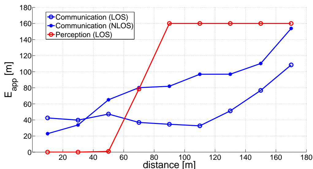
FIGURE 6.17: Évaluation de l'erreur d'application.
