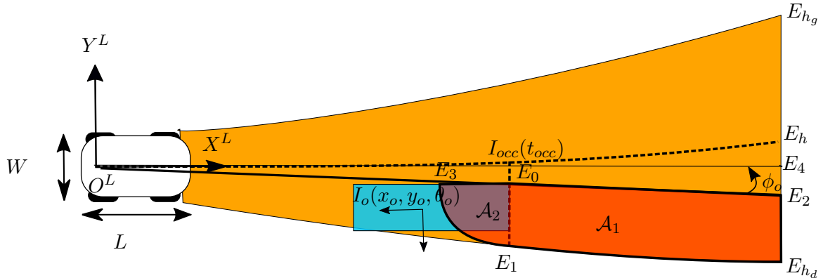
FIGURE 4.7: Définition de la Geo-Area
