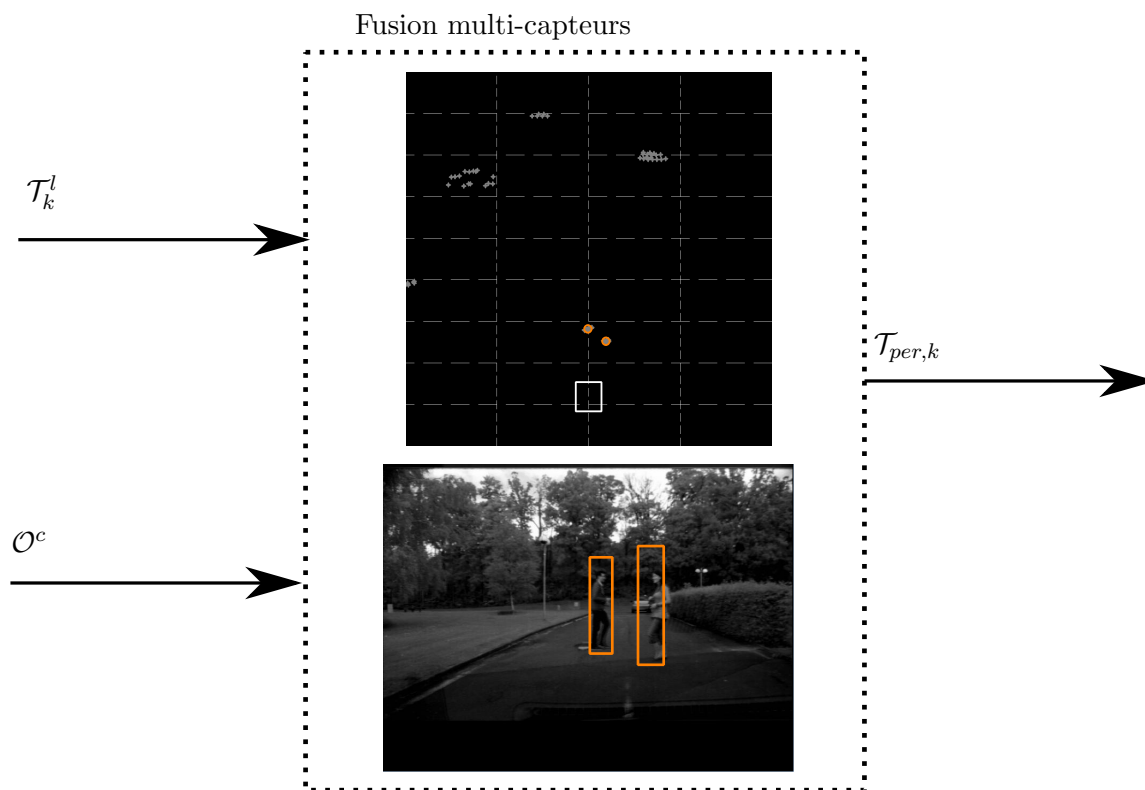
FIGURE 3.11: Fusion multi-capteurs
