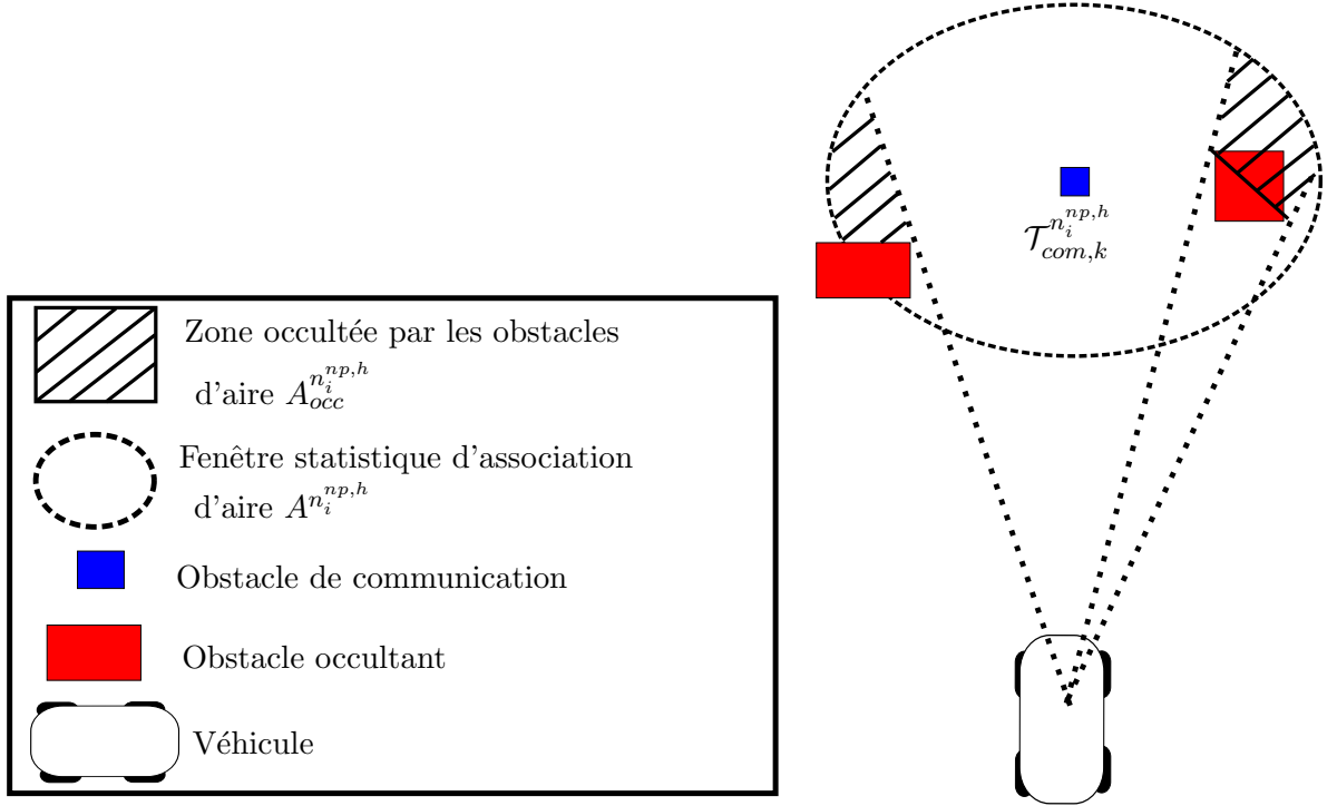
FIGURE 5.9: Aire occultée par les obstacles perçus pour une piste de communication
