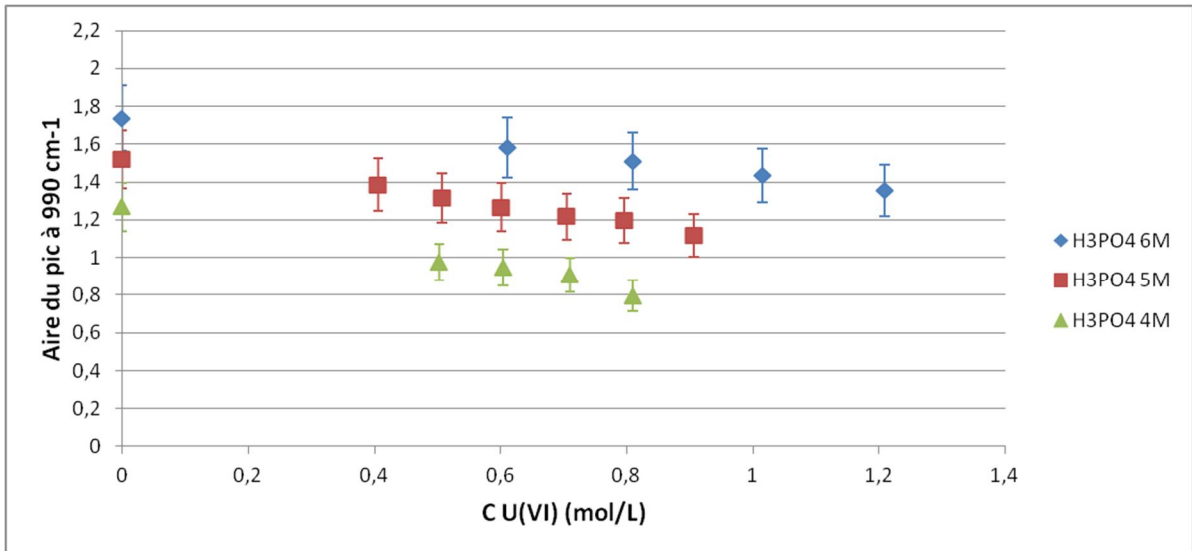
Figure 14 : Evolution de l'aire du pic à 990\text{ cm}^{-1} avec la concentration en uranium(VI) pour des solutions d'acide à 4, 5 et 6 mol/L
