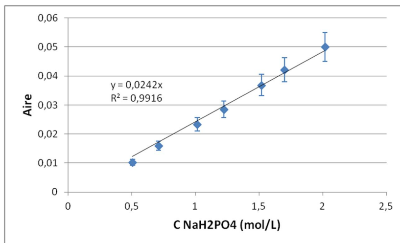
Figure 7 : Evolution de l'aire du pic à 889 cm -1 avec la concentration en dihydrogénophosphate de sodium
