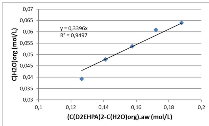
Figure 42 : Courbe [\overline{H_2O}] en fonction de \left([\overline{(H_2L_2)}]_0 - [\overline{H_2O}]\right) \cdot a_w pour le D2EHPA à 0,51 mol/L
