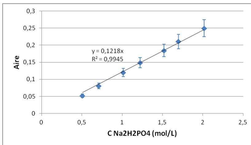
Figure 8 : Evolution de l'aire du pic à 990 cm -1 avec la concentration en dihydrogénophosphate de sodium
