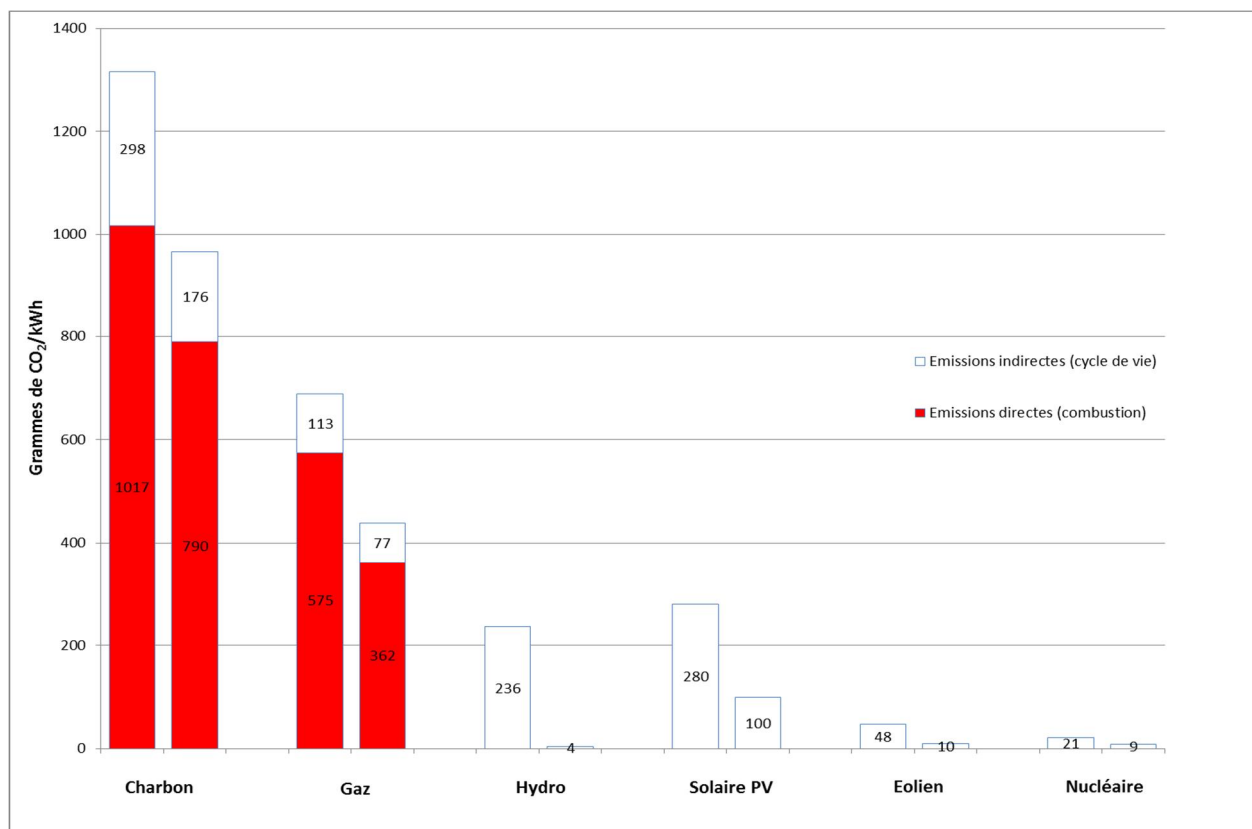
Figure 2 : Masses de CO 2 rejetées par kWh d'électricité produit par les technologies les plus répandues en 2000 [3] (les barres doubles indiquent la gamme)
