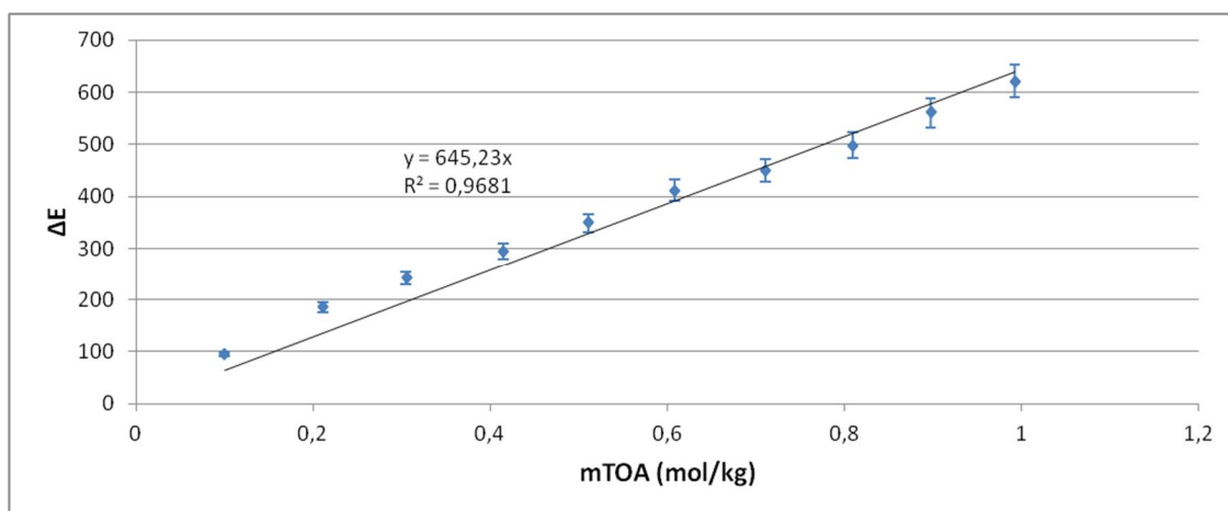
Figure 18 : Evolution du signal VPO avec la molalité en TOA dans le pentane à 25°C
