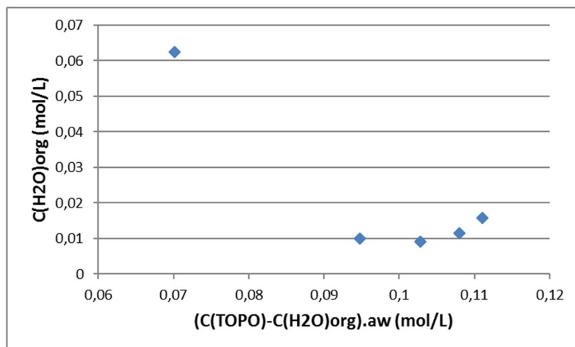
Figure 44 : Courbe \overline{[H_2O]} en fonction de \left(\overline{[H_2L_2]}\right)_0 - \overline{[H_2O]} pour le TOPO
