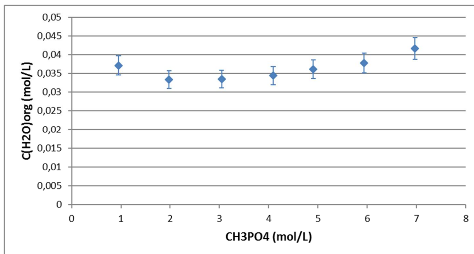
Figure 45: Evolution de la concentration en eau dans la phase organique (0,51 mol/L de D2EHPA) avec la concentration en acide phosphorique de la phase aqueuse
