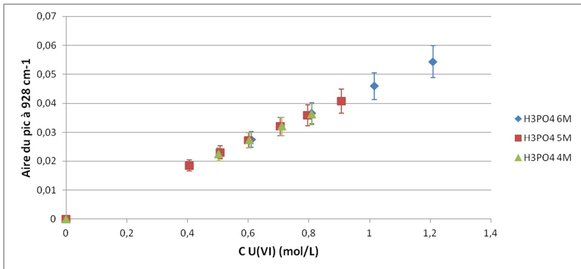
Figure 15 : Evolution de l'aire du pic à 928\text{ cm}^{-1} avec la concentration en uranium(VI) pour des solutions d'acide à 4, 5 et 6 mol/L
