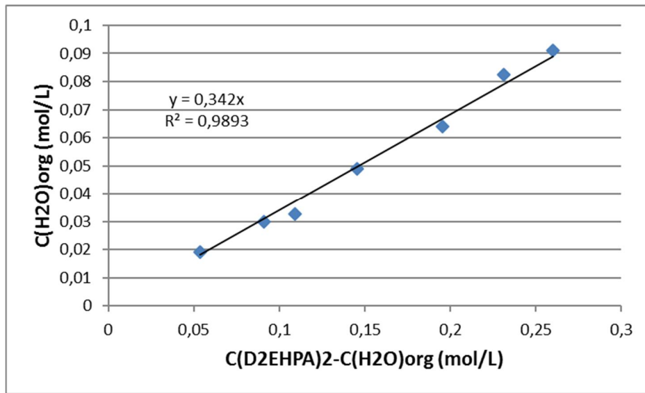
Figure 38 : Courbe \overline{[H_2O]} en fonction de [(H_2L_2)]_0 - \overline{[H_2O]}
