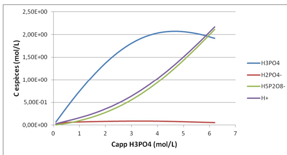
Figure 2 : Diagramme de spéciation du système \text{H}_3\text{PO}_4\text{-H}_2\text{O}
