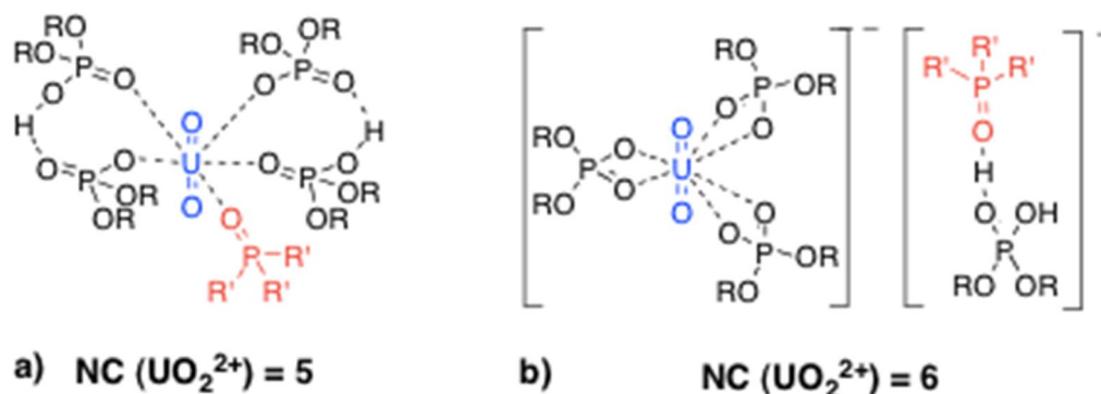
Figure 11 : Structures du complexe uranium(VI)-D2EHPA-TOPO selon a) Baes [153] et b) Zangen [160]
