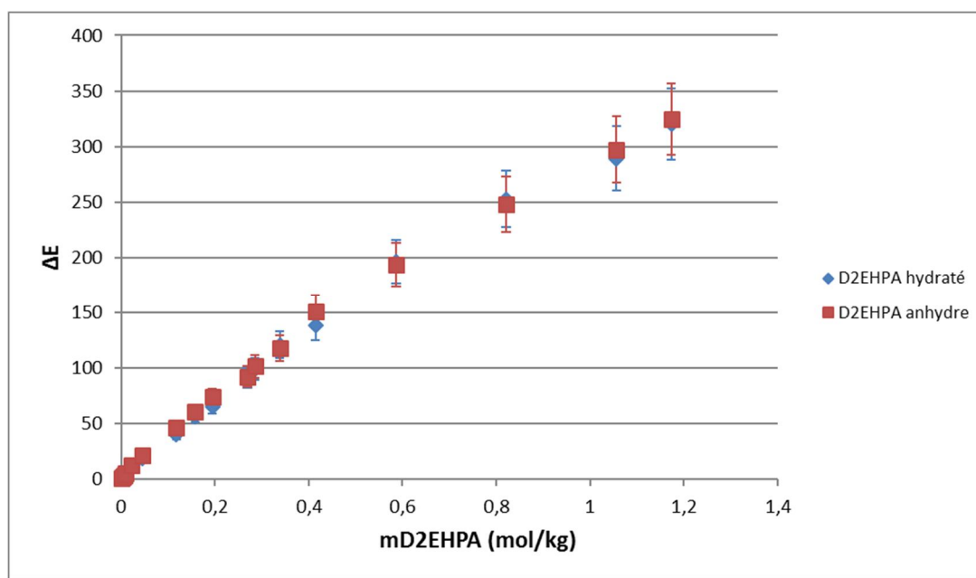
Figure 24 : Evolution du signal VPO avec la molarité en D2EHPA dans du pentane anhydre et saturé d'eau à 25^\circ\text{C}
