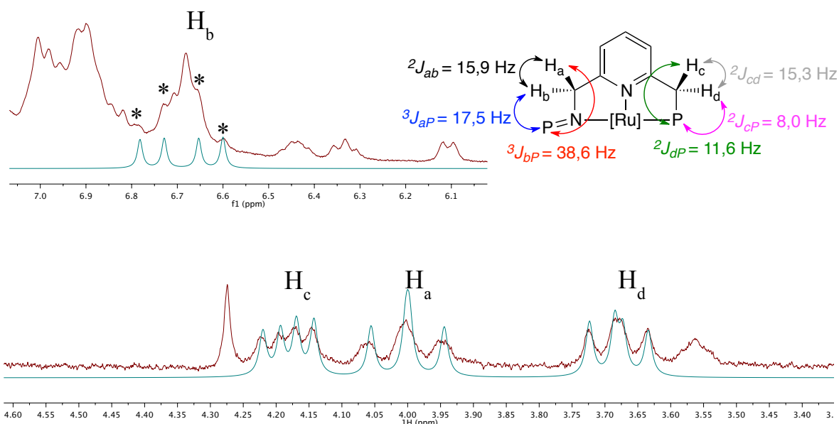
Figure 84 - Spectres (rouge) et simulations (turquoise) des deux systèmes AMX de [L^{13}RuCl(PPh_3)]
