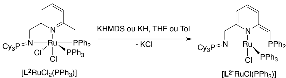
Schéma 199 - Déaromatation du complexe [L^2RuCl_2(PPh_3)]
