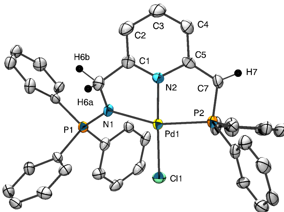
Figure 68 - ORTEP de [L^{1*}PdCl] – Les atomes d'hydrogènes, hormis benzyliques ont été omis pour plus de clarté. Longueurs de liaisons (Å) et angles (°) sélectionnés : N1-P1 1,595(5), N1-Pd1 2,124(5), P2-Pd1 2,218(2), N2-Pd1 1,994(5), Cl1-Pd1 2,313(2), C7-P2 1,742(7), N2-C1 1,358(8), C1-C2 1,37(1), C2-C3 1,43(1), C3-C4 1,34(1), C4-C5 1,44(1), C5-N2 1,389(8), C1-C6 1,50(1), C5-C7 1,38(1), C7-H7 0,87(8), C6-H6A 0,90(7), C6-H6B 1,08(7); N1-Pd1-P2 161,8(1), N2-Pd1-Cl1 176,1(2), N1-Pd1-N2 79,8(2), P2-Pd1-N2 84,4(2), N1-Pd1-Cl1 102,8(1), P2-Pd1-Cl1 93,46(6).
