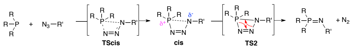
Schéma 17 - Mécanisme général de la réaction de Staudinger
