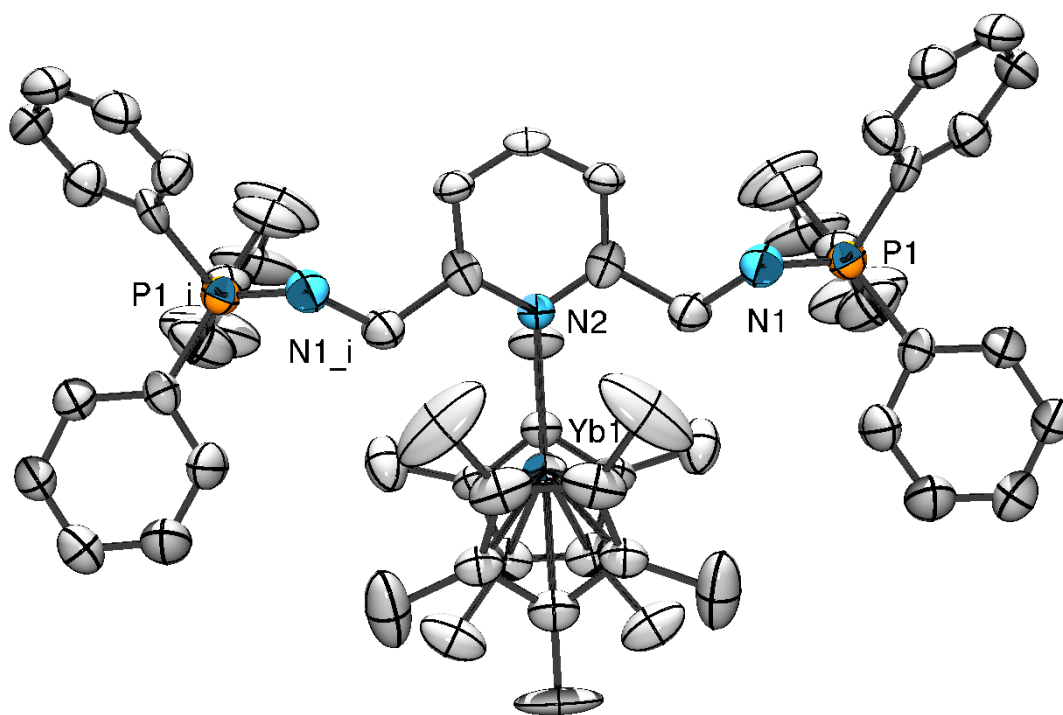
Figure 45 - ORTEP de [\text{L}^{\text{Ph}}\text{YbCp}^*_2] – Les atomes d'hydrogènes ont été omis pour plus de clarté, Cp désigne un centroïde. Longueurs de liaisons (Å) et angles (°) sélectionnés : N1-P1 1,562(8), N2-Yb1 2,53, Yb1-Cp1 2,43 ; N2-Yb1-Cp1 111,2.
