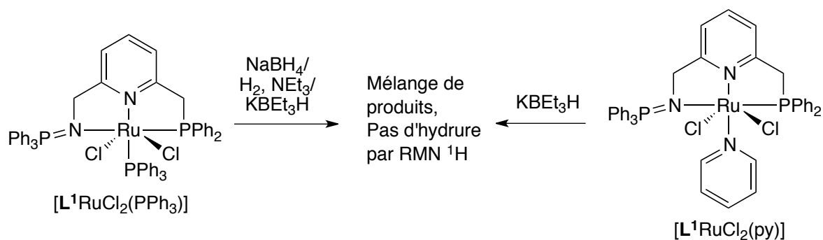
Schéma 202 - Tentatives d'introduction d'un hydrure
