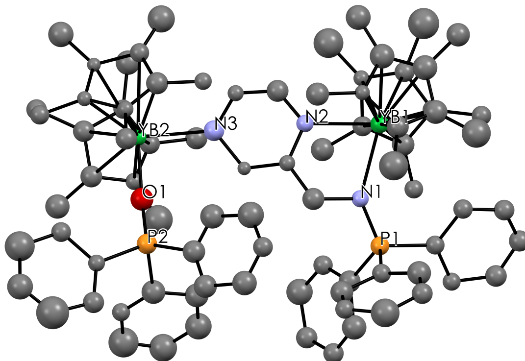
Figure 54 - Représentation isotrope du complexe [Cp^*_2Yb(OPPh_3)L^{Pyra}Cp^*_2Yb]
