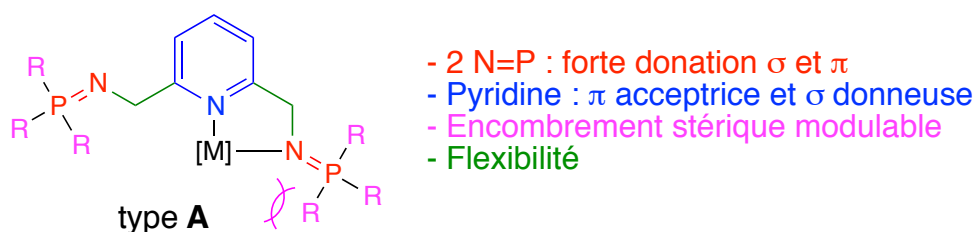
Schéma 80 - Propriétés désirées pour un ligand pinceur iminophosphorane symétrique
