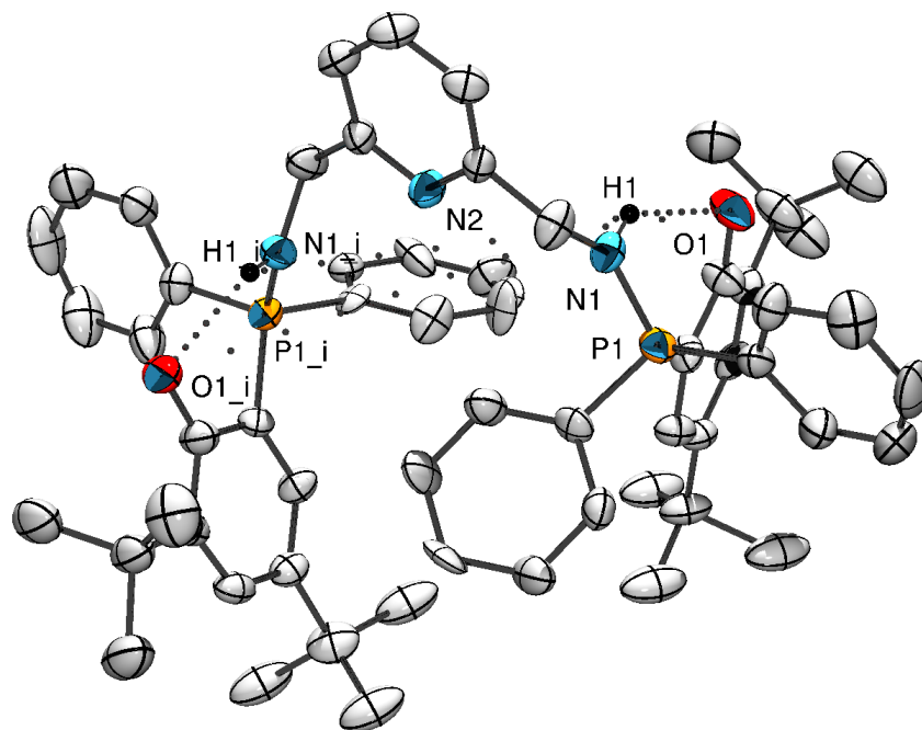
Figure 93 - ORTEP de L^{PyPsalen}H_2 – Les atomes d'hydrogènes sauf H1 ont été omis pour plus de clarté. Longueurs de liaisons (Å) et angles (°) sélectionnés : N1-P1 1,617(5), N1-H1 0,85(7), H1-O1 2,07(7) ; P1-N1-C4 127,2(4), P1-N1-H1 110(5), N1-H1-O1 135(6).
