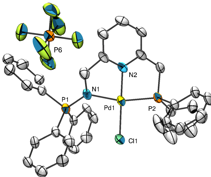
Figure 72 - ORTEP de [L^1PdCl]PF_6 – Une seule des deux molécules co-cristallisées est présentée, une molécule de THF et les atomes d'hydrogènes ont été omis pour plus de clarté. Longueurs de liaisons (Å) et angles (°) sélectionnés : N1-P1 1,617(6), N1-Pd1 2,074(6), P2-Pd1 2,207(2), N2-Pd1 2,001(6), Cl1-Pd1 2,295(2) ; N1-Pd1-P2 164,1(2), N2-Pd1-Cl1 175,8(2), N1-Pd1-N2 80,2(3), P2-Pd1-N2 83,9(2), N1-Pd1-Cl1 99,7(2), P2-Pd1-Cl1 96,23(8).
