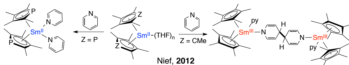
Schéma 130 - Modulation de la réactivité du samarium divalent
