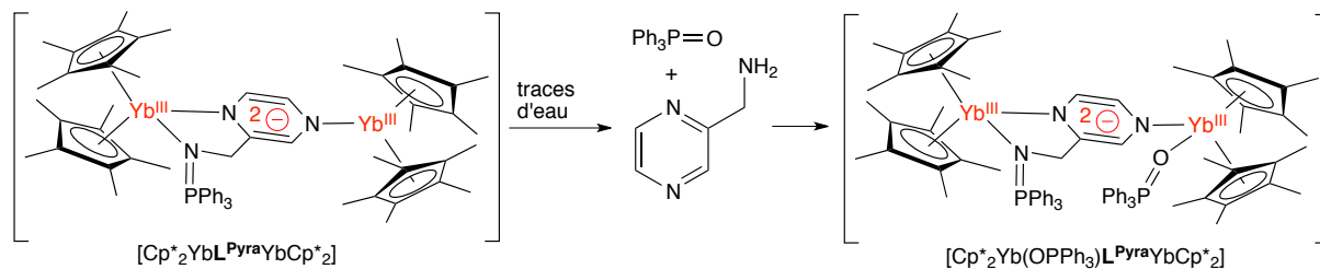
Schéma 157 - Formation de [Cp^*_2Yb(OPPh_3)L^{Pyra}Cp^*_2Yb] par hydrolyse du ligand
