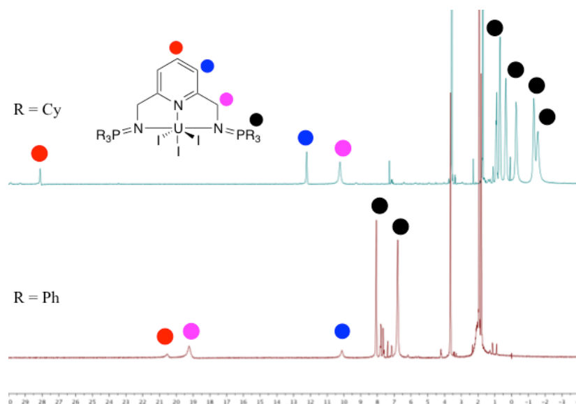
Figure 40 - Spectres protons des composés [L^{Ph}U\text{I}_3] et [L^{Cy}U\text{I}_3]
