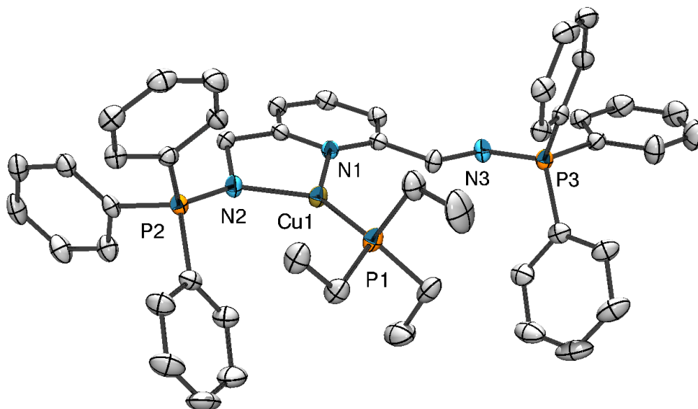
Figure 28 - ORTEP de [\text{L}^{\text{Ph}}\text{CuPEt}_3](\text{PF}_6) – Les atomes d'hydrogènes et l'anion \text{PF}_6^- ont été omis pour plus de clarté. Longueurs de liaisons (Å) et angles ( ^\circ ) sélectionnés : N2-P2 1,591(2), N3-P3 1,580(2), N2-Cu1 1,990(2), N1-Cu1 2,066(2), P1-Cu1 2,174(1) ; N1-Cu1-N2 83,1(1), N2-Cu1-P1 138,66(7), N1-Cu1-P1 138,25(7).
