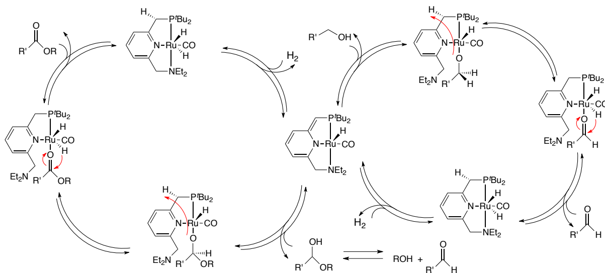
Schéma 56 - Mécanisme simplifié de l(a)' (dés)hydrogénation
