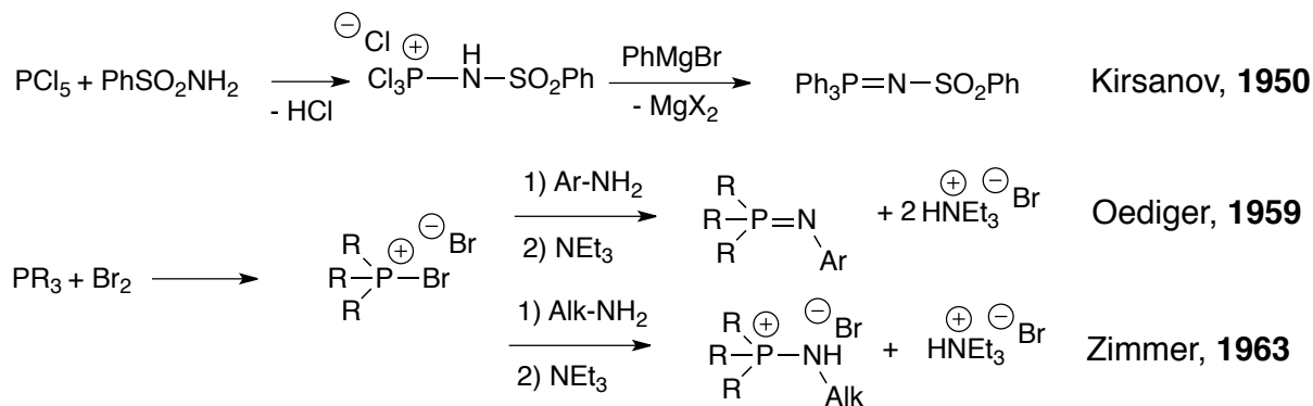
Schéma 20 - Réaction originale de Kirsanov, variation de Oediger et constatation de Zimmer
