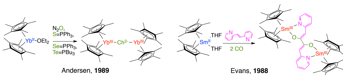
Schéma 127 - Réactivités des lanthanides divalents vis-à-vis des chalcogènes et du monoxyde de carbone
