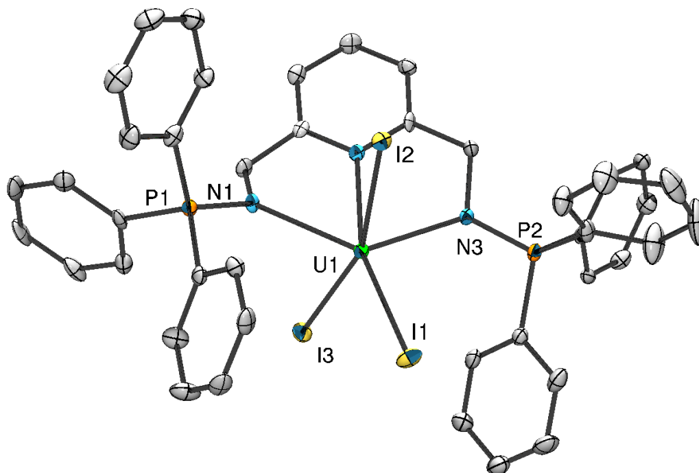
Figure 42 - ORTEP de [L^{Ph}UI_3] – Trois molécules de THF co-cristallisées et les atomes d'hydrogènes ont été omis pour plus de clarté. Longueurs de liaisons (Å) et angles ( ^\circ ) sélectionnés : N1-P1 1,597(3), N3-P2 1,617(3), N1-U1 2,494(4), N3-U1 2,528(3), N2-U1 2,540(2), I1-U1 3,1042(6), I2-U1 3,1406(4) I3-Yb1 3,1692(5) ; N1-U1-N3 130,2(1), N2-U1-I1 162,30(8), I2-U1-I3 161,92(2), N1-U1-N2 65,3(1), N3-U1-N2 65,0(1), N1-U1-I1 128,58(8), N3-U1-I1 100,38(8), N1-U1-I2 84,47(8), N3-U1-I2 87,65(8), N2-U1-I2 79,96(8), I1-U1-I2 89,94(1), I2-U1-I3 102,37(2).
