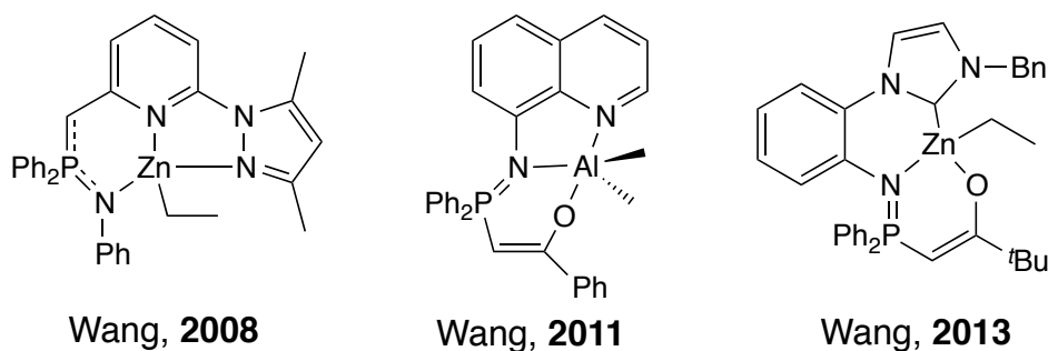
Schéma 67 - Ligands iminophosphoranes appliqués à la polymérisation
