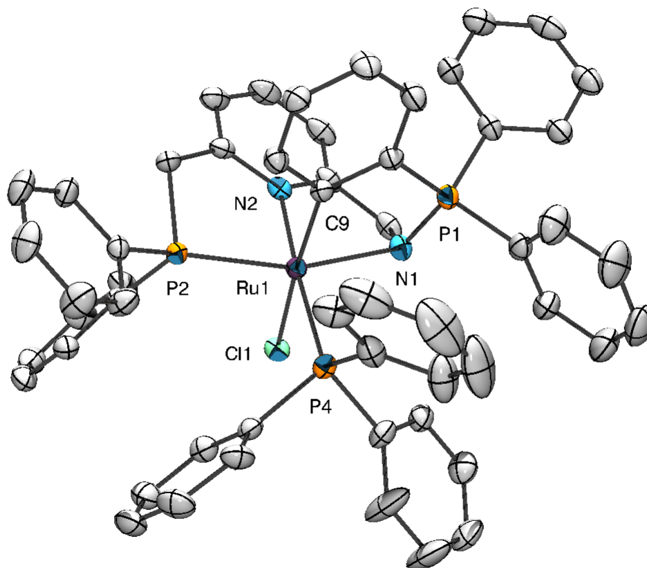
Figure 83 - ORTEP de [L^1RuCl(PPh_3)] – Une molécule et demi de benzène et les atomes d'hydrogènes ont été omis pour plus de clarté. Longueurs de liaisons (Å) et angles ( ^\circ ) sélectionnés : N1-P1 1,612(2), N1-Ru1 2,193(2), P2-Ru1 2,2821(8), N2-Ru1 2,094(2), P4-Ru1 2,3087(8), Cl1-Ru1 2,5412(7), C9-Ru1 2,072(3) ; N1-Ru1-P2 157,49(7), N2-Ru1-P4 173,08(7), C9-Ru1-Cl1 172,69(8), N1-Ru1-N2 76,6(1), P2-Ru1-N2 80,94(7), P2-Ru1-P4 104,23(3), N1-Ru1-P4 98,26(7), Cl1-Ru1-N1 88,08(7), Cl1-Ru1-P2 91,65(3), Cl1-Ru1-N2 86,35(7), Cl1-Ru1-P4 88,88(3), C9-Ru1-N2 88,9(1), C9-Ru1-N1 85,4(1), C9-Ru1-P4 95,34(8), C9-Ru1-P2 80,94(7).
