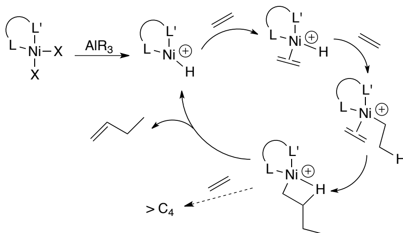
Schéma 220 - Mécanisme de Cossee simplifié
