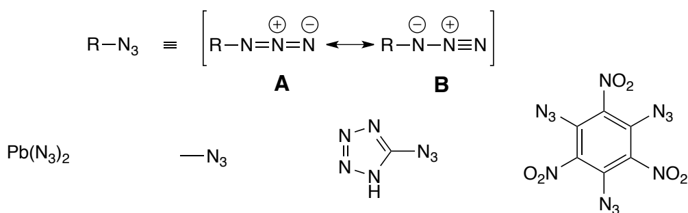
Schéma 12 - Formes de résonance d'un azoture et exemples d'azotures explosifs
