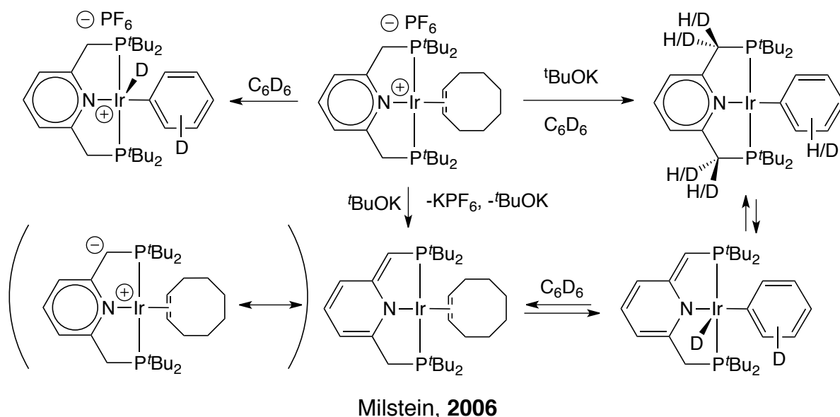
Schéma 54 - Coopération métal-ligand par aromatisation/déaromatisation
