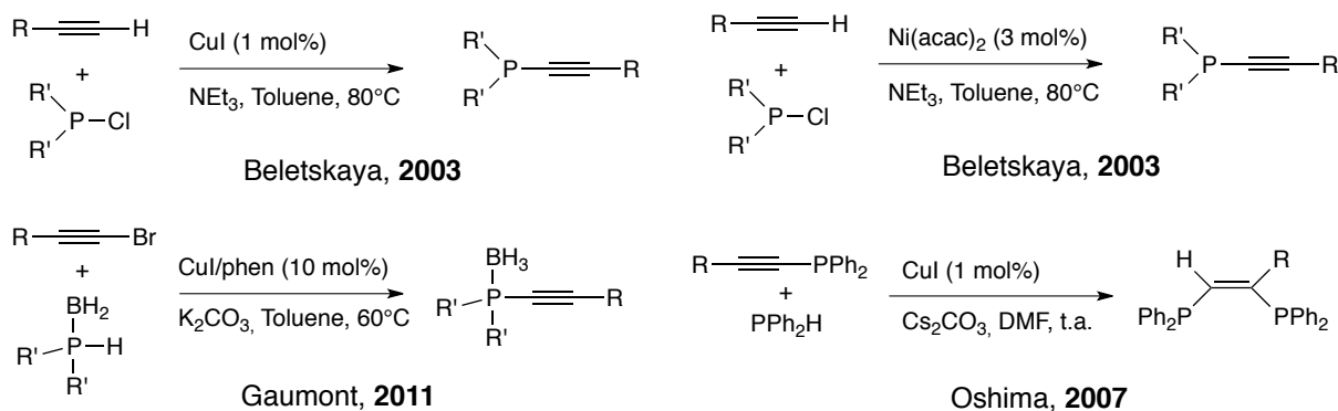
Schéma 114 - Synthèse et réactivité d'alcynes-phosphine par catalyse homogène
