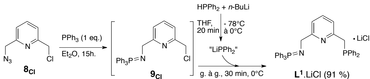
Schéma 175 - Synthèse "one pot" de L^1.LiCl
