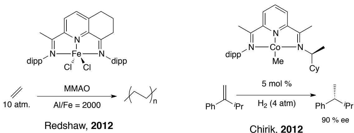
Schéma 31 - Applications des ligands bis(imino)pyridines à la catalyse
