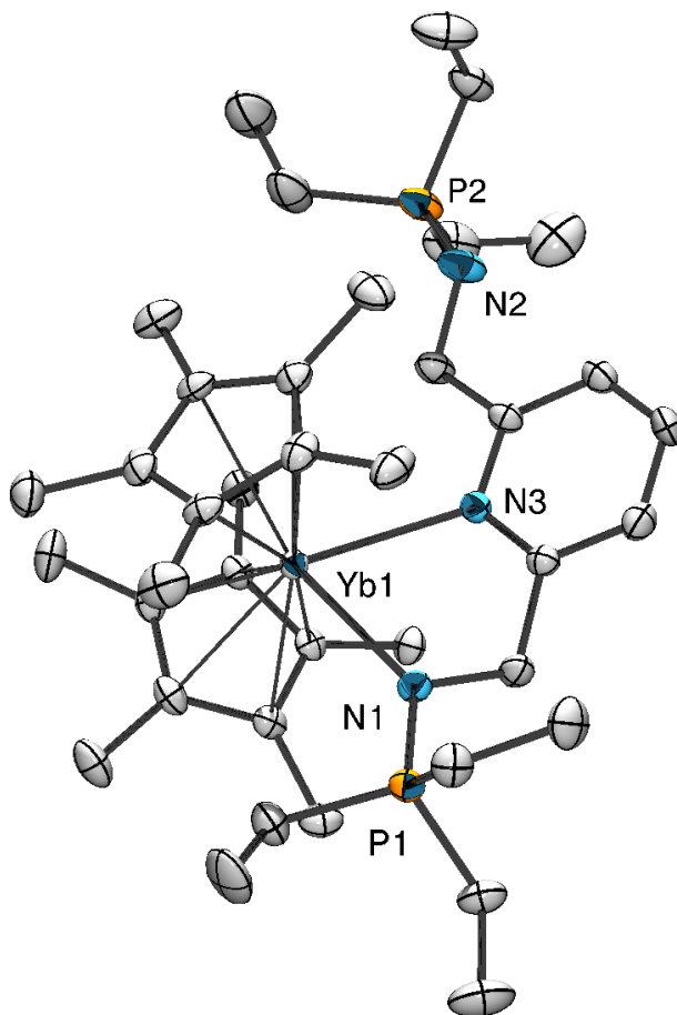
Figure 44 - ORTEP de [\mathbf{L}^{\text{Et}}\text{YbCp}^*_2] – Les atomes d'hydrogènes ont été omis pour plus de clarté, Cp désigne un centroïde. Longueurs de liaisons (Å) et angles (°) sélectionnés : N1-P1 1,593(3), N2-P2 1,561(4), N1-Yb1 2,511(3), N3-Yb1 2,562(3), Yb1-Cp1 2,49, Yb1-Cp2 2,50 ; N1-Yb1-N3 72,1(1), N3-Yb1-Cp1 108,3, N3-Yb1-Cp2 105,1.
