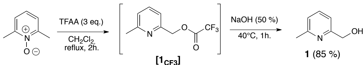
Schéma 167 - Désymétrisation de la lutidine N-oxyle
