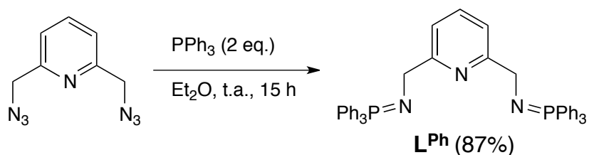
Schéma 85 - Synthèse de L^{Ph}
