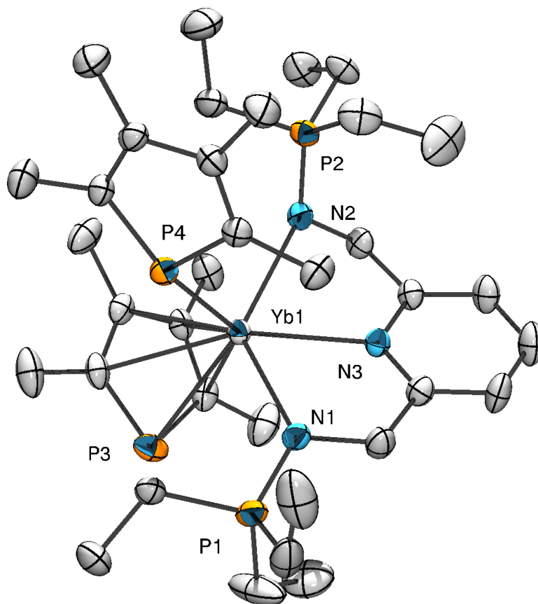
Figure 49 - ORTEP de [\text{L}^{\text{Et}}\text{Yb}(\text{tmp})_2] – Les atomes d'hydrogènes ont été omis pour plus de clarté, tmp désigne un centroïde. Longueurs de liaisons (Å) et angles (°) sélectionnés : N1-P1 1,597(3), N2-P2 1,594(3), N1-Yb1 2,512(2), N2-Yb1 2,533(2), N3-Yb1 2,493(2), Yb1-P3 3,027(1), Yb1-P4 2,9723(8), Yb1-tmp1 2,573 ; N1-Yb1-N3 65,58(8), N2-Yb1-N3 66,92(8), N3-Yb1-tmp1 123,9, P4-Yb1-tmp1 115,5.
