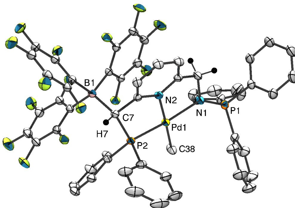
Figure 74 - ORTEP de [\text{L}^{\text{B}}\text{PdMe}] – Les atomes d'hydrogènes, hormis H7 ont été omis pour plus de clarté. Longueurs de liaisons (Å) et angles ( ^\circ ) sélectionnés : N1-P1 1,597(2), N1-Pd1 2,136(2), P2-Pd1 2,2078(6), N2-Pd1 2,073(2), C38-Pd1 2,056(2), C5-C7 1,515(3), C7-P2 1,868(2), C7-B1 1,710(3), C7-H7 0,94(3) ; N1-Pd1-P2 159,60(6), N2-Pd1-C38 177,6(1), N1-Pd1-N2 80,11(7), P2-Pd1-N2 81,95(5), N1-Pd1-C38 101,9(1), P2-Pd1-C38 95,81(7), P2-C7-B1 122,9(1), C5-C7-B1 108,0(2), B1-C7-H7 104(2).
