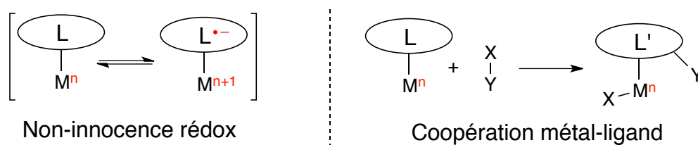
Schéma 46 - Différence entre non-innocence rédox et coopération métal-ligand
