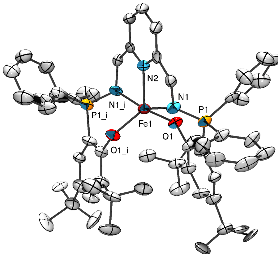
Figure 95 - ORTEP de [\mathbf{L}^{\text{PyPsalen}}\text{Fe}] – Les atomes d'hydrogènes ont été omis pour plus de clarté. Longueurs de liaisons (Å) et angles (°) sélectionnés : N1-P1 1,588(8), N1-Fe1 2,148(7), N2-Fe1 2,11(1), O1-Fe1 2,017(6) ; N1-Fe1-N1i 153,9(4), O1-Fe1-O1i 120,8(3), O1-Fe1-N2 119,6(2), N1-Fe1-N2 76,9(2), N1-Fe1-O1 89,2(3).
