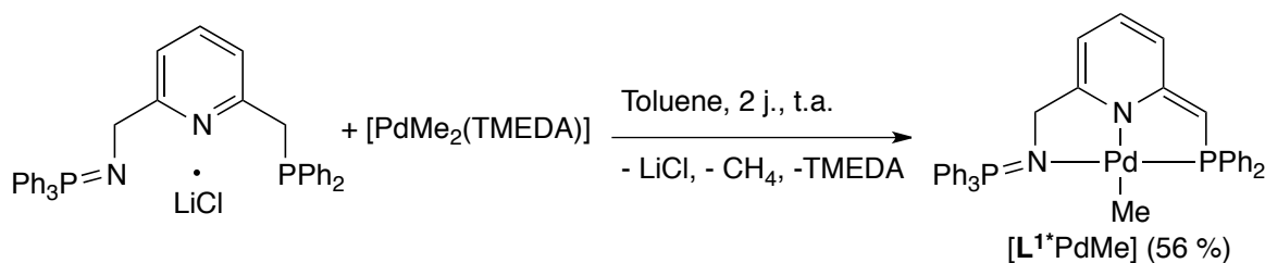
Schéma 186 - Formation d'un complexe palladium-alkyle déaromatisé
