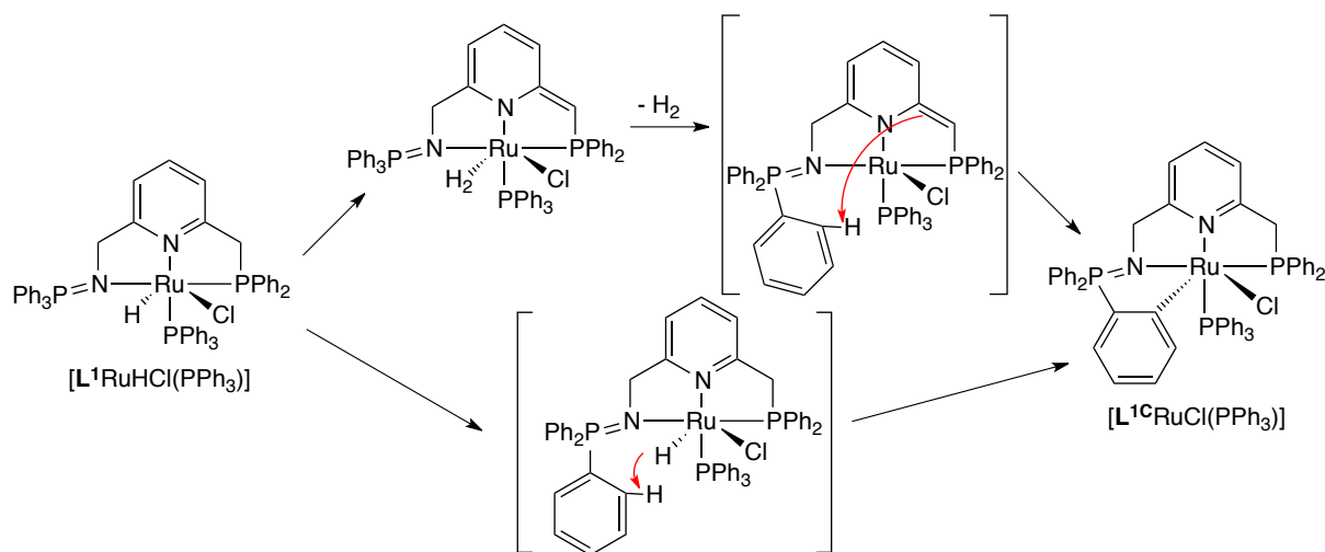
Schéma 205 - Mécanismes possibles pour la cycloméatallation
