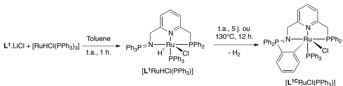
Schéma 203 - Formation d'un complexe hydrure et activation C-H
