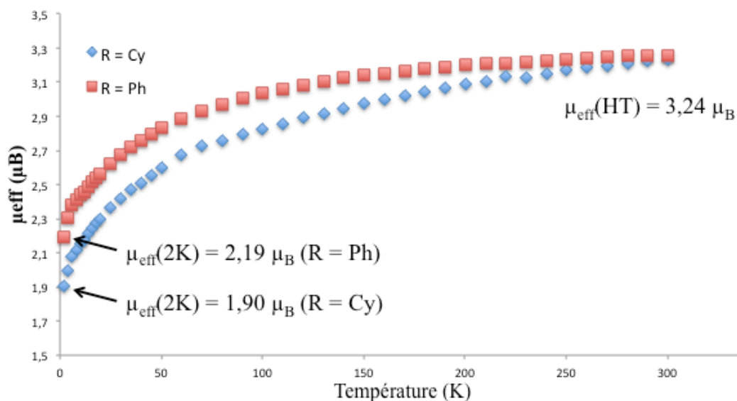
Figure 41 - Moments effectifs en fonction de la température pour les complexes [L^{\text{Ph}}\text{UI}_3] et [L^{\text{Cy}}\text{UI}_3]
