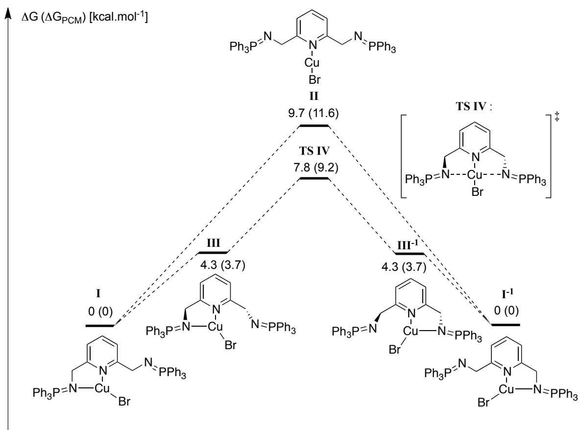
Schéma 104 - Profils énergétiques calculés pour le processus d'échange dans [\text{L}^{\text{Ph}}\text{CuBr}]
