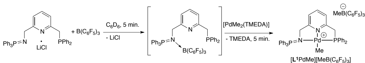
Schéma 193 - Formation de [L^1PdMe][MeB(C_6F_5)_3]
