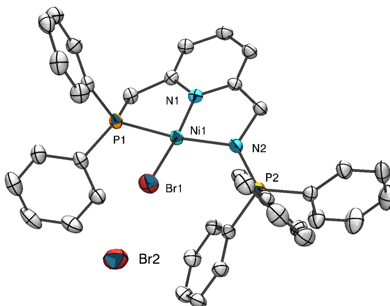
Figure 63 - ORTEP de [L^1NiBr]Br – Les atomes d'hydrogènes et deux molécules de dichlorométhane co-cristallisées ont été omis pour plus de clarté ainsi qu'un désordre chlore/brome sur la position Br1. Longueurs de liaisons (Å) et angles (°) sélectionnés : N2-P2 1,605(3), N2-Ni1 1,941(3), P1-Ni1 2,1459(8), N1-Ni1 1,880(2), Br1-Ni1 2,224(7) ; N2-Ni1-P1 169,61(8), N1-Ni1-Br1 173,4(2), N2-Ni1-N1 83,6(1), P1-Ni1-N1 86,08(8), N2-Ni1-Br1 99,9(2), P1-Ni1-Br1 90,5(2).
