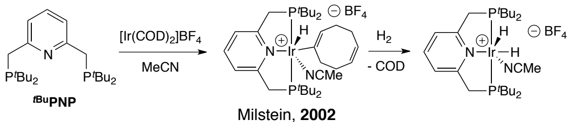
Schéma 36 - C-H activation et réaction avec le dihydrogène d'un pinceur PNP
