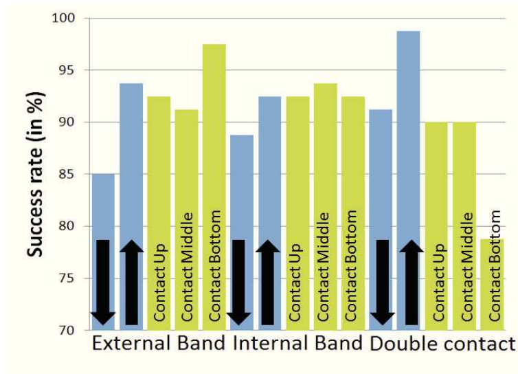
FIGURE 8.20 – Taux de réussite moyen pour chaque geste de notre vocabulaire.
