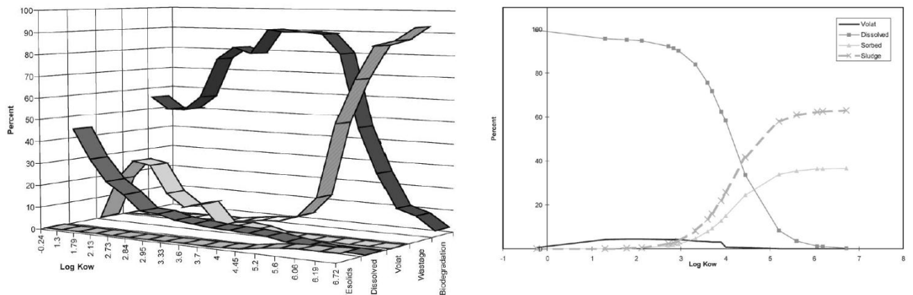
Figure I-9 : Répartition des différents mécanismes d'abattement d'un procédé à boues activées en fonction de l'hydrophobicité (Byrns 2001)
