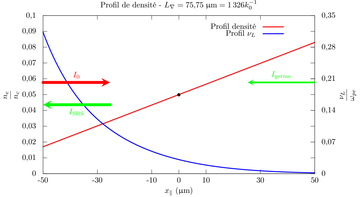
FIGURE 5.1 – Coupe sur l’axe central du profil de densité linéaire L_{\nabla} = 75,75 \mu\text{m} = 1326k_0^{-1} . La pompe entre par le côté gauche et se propage vers la droite, tandis que le germe entre du côté droit et se propage vers la gauche. Ces deux faisceaux se croisent au centre de la boîte, là où le système est accordé, à 5% de la densité critique. Ce point particulier est représenté par le point noir sur la figure. La réflectivité, I_{\text{SRS}} , est l’intégrale sur le bord gauche du signal sortant.
