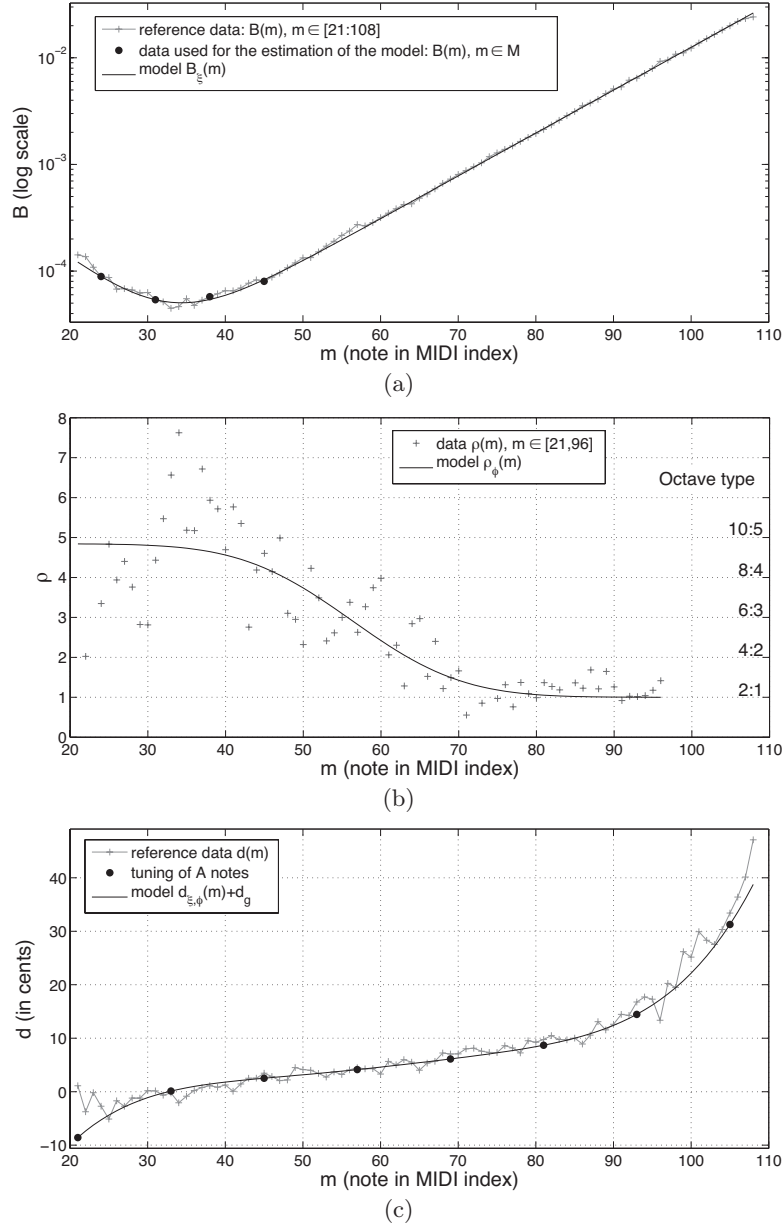
Figure E.14: Piano   queue RWC3. (a) Coefficient d'inharmonicit  B , (b) param tre de type d'octave \rho , (c) d viation de l'accord par rapport au temp r ment  gal le long de la tessiture.
